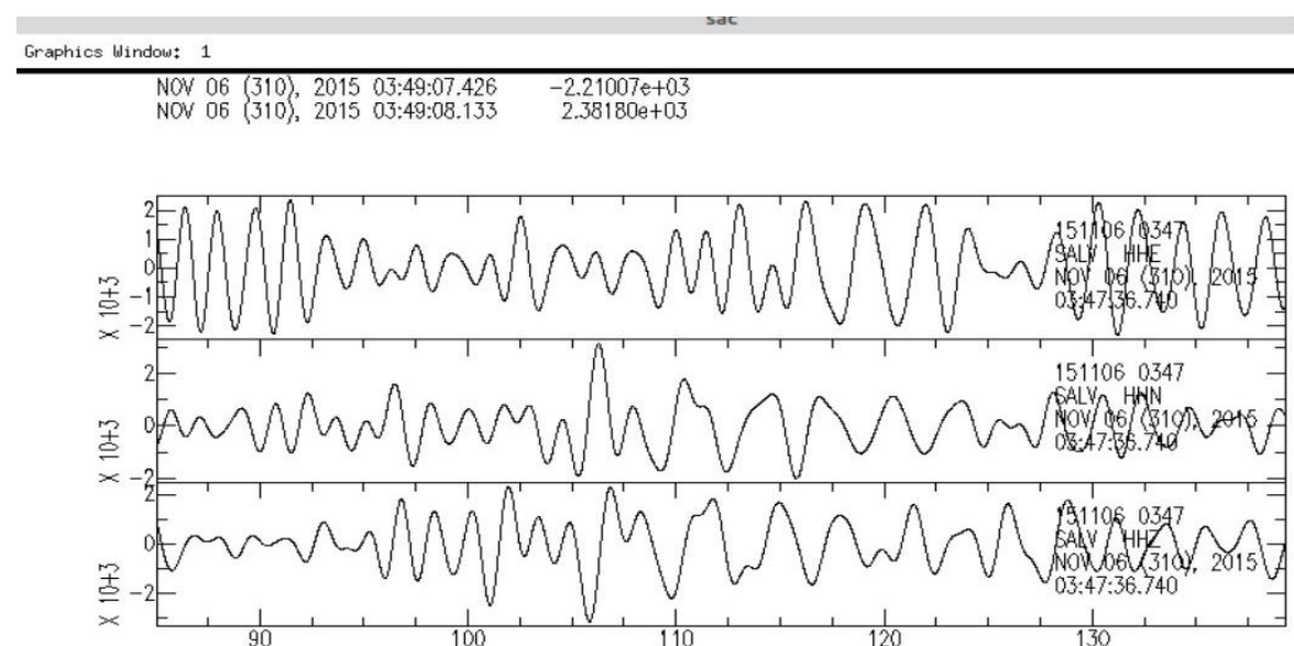
Figura 6.12 - Aceleração de onda sísmica registrado pela estação SALV.
