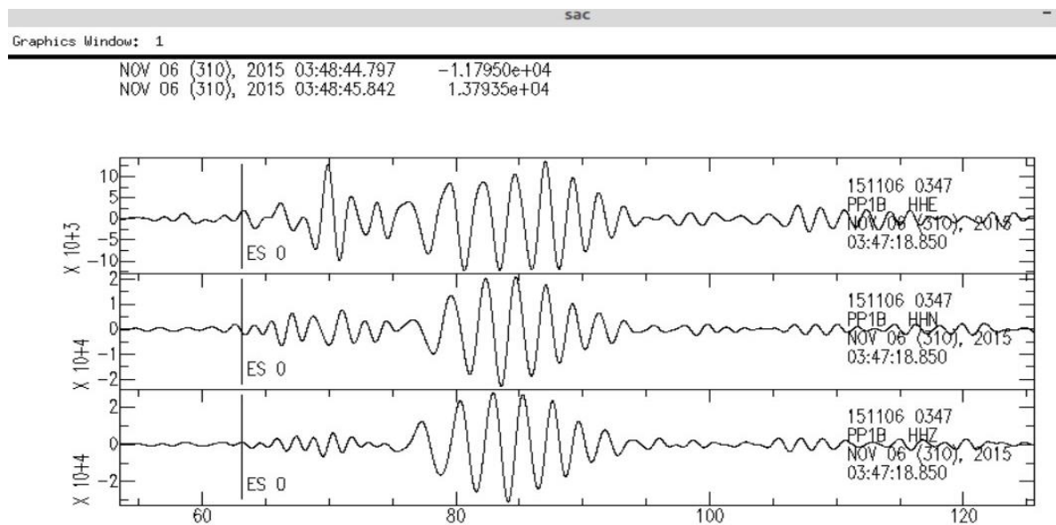
Figura 6.9 - Aceleração de onda sísmica registrado pela estação PP1B.
