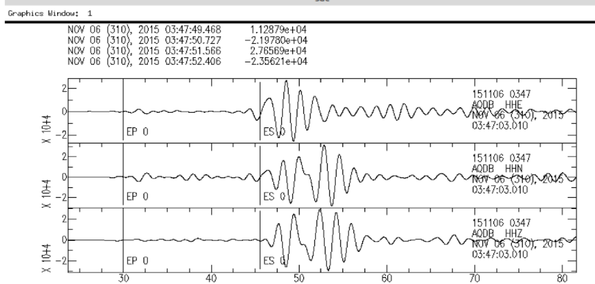
Figura 6.6 - Aceleração de onda sísmica registrado pela estação AQDB.
