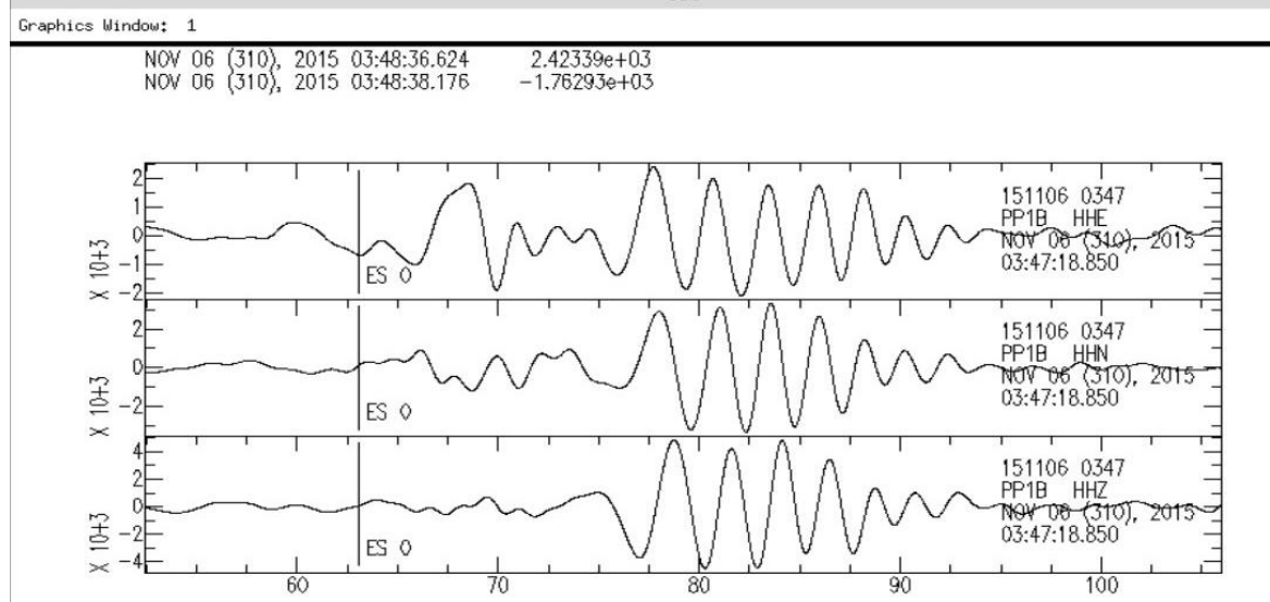
Figura 6.7 - Deslocamento de onda sísmica registrado pela estação PP1B.
