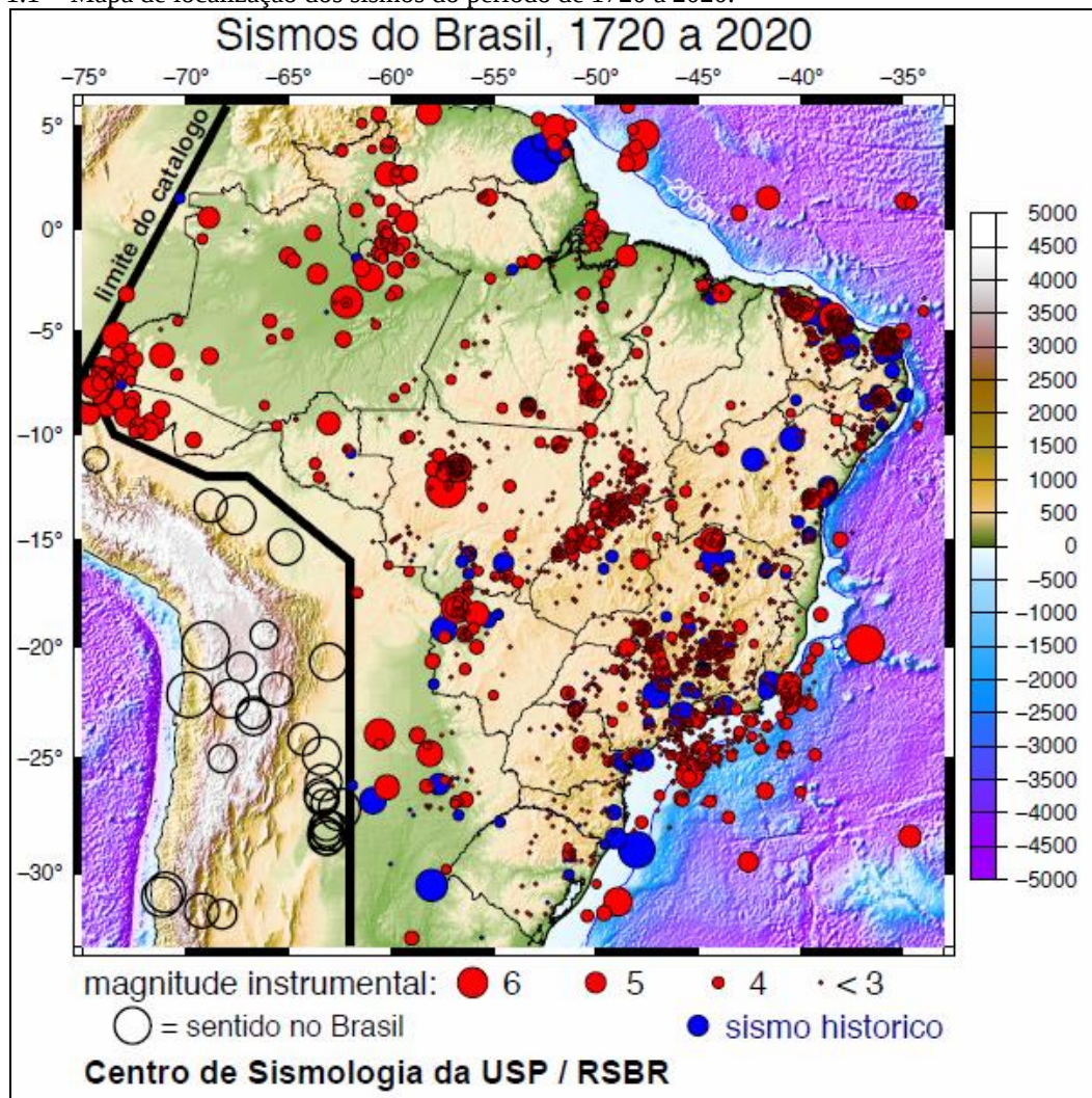
Figura 1.1 - Mapa de localização dos sismos do período de 1720 à 2020.
