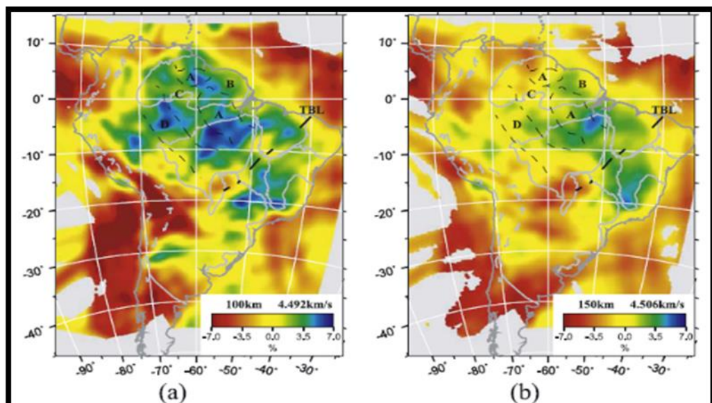
Figura 4.14- Fatias horizontais do modelo de velocidade S obtido a 100, 150, 200 e 300 km.
