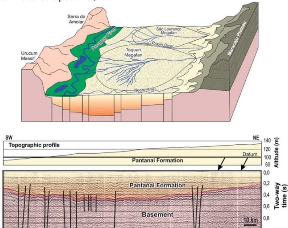
Figura 4.11- Bacia estruturada por falhas. (a) Diagrama de bloco esquemático que ilustra a geometria da bacia. (b) Desenho de linha sobre a seção sísmica,
