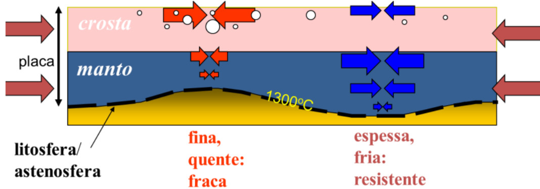
Figura 4.13- Modelo de regiões de maior sismicidade, o qual apresenta zonas de baixa velocidade para as ondas sísmicas, podendo estar associado ao afinamento litosférico e como consequência soerguimento da astenosfera,
