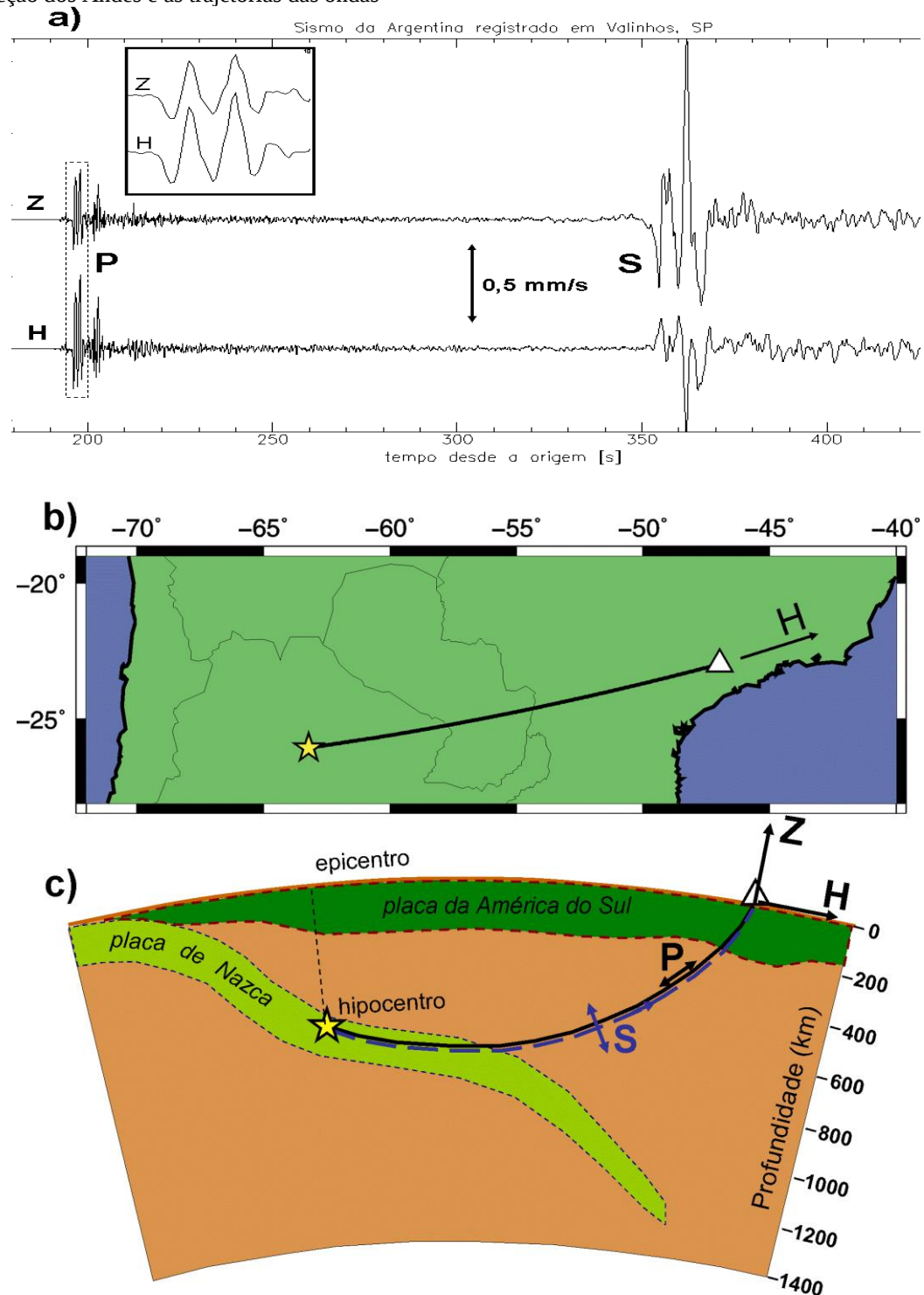
Figura 4.1- (a) Registro do sismo da Argentina de 13/11/2006 na estação sismográfica de Valinhos (SP); (b) Localização do epicentro (estrela) e a estação de Valinhos, SP (triângulo). (c) Perfil com o hipocentro na zona de subducção dos Andes e as trajetórias das ondas
