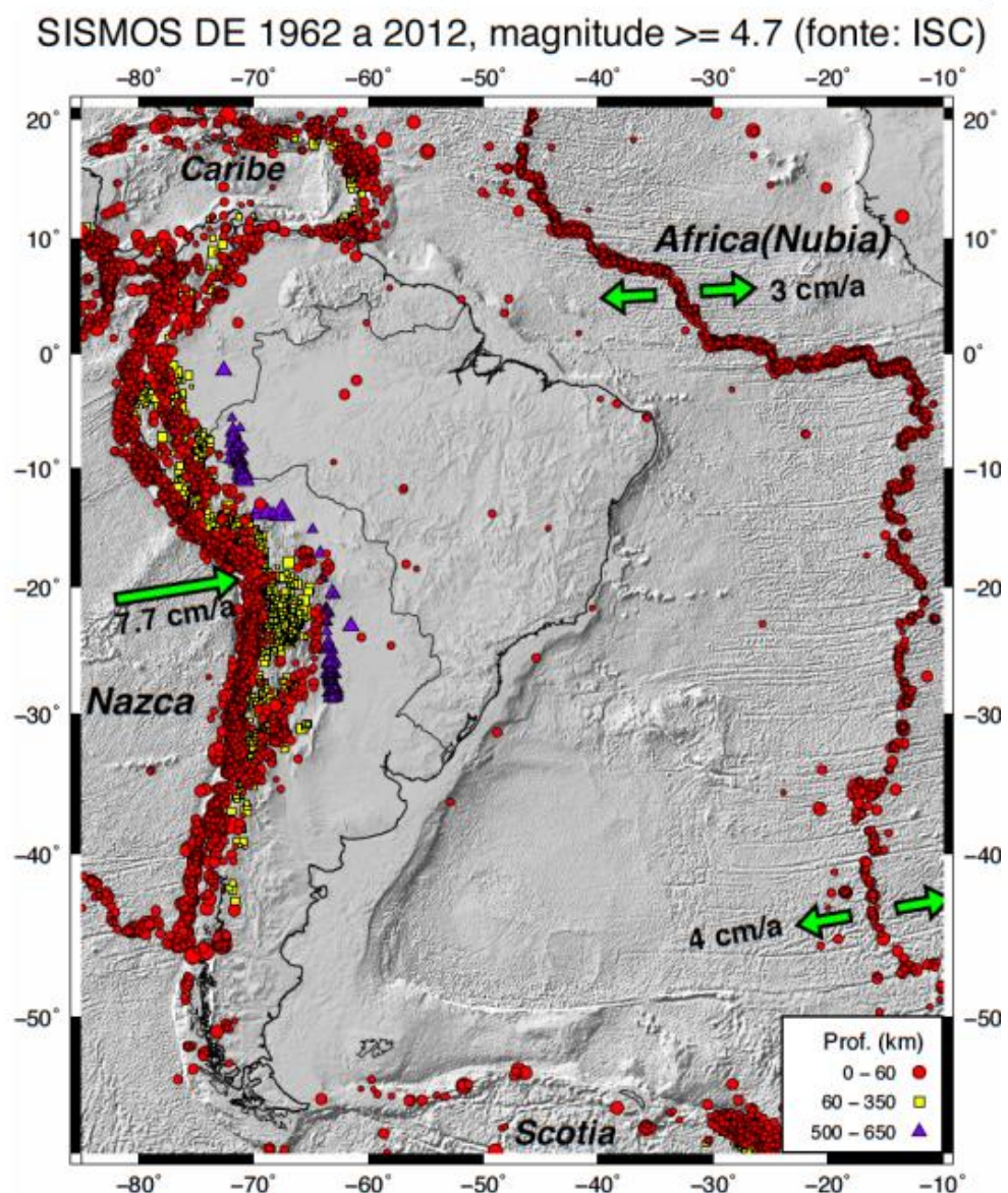
Figura 4.8 - Sismos na placa da América do Sul (1962-2012) com magnitudes acima de 4.7 na Escala Richter.
