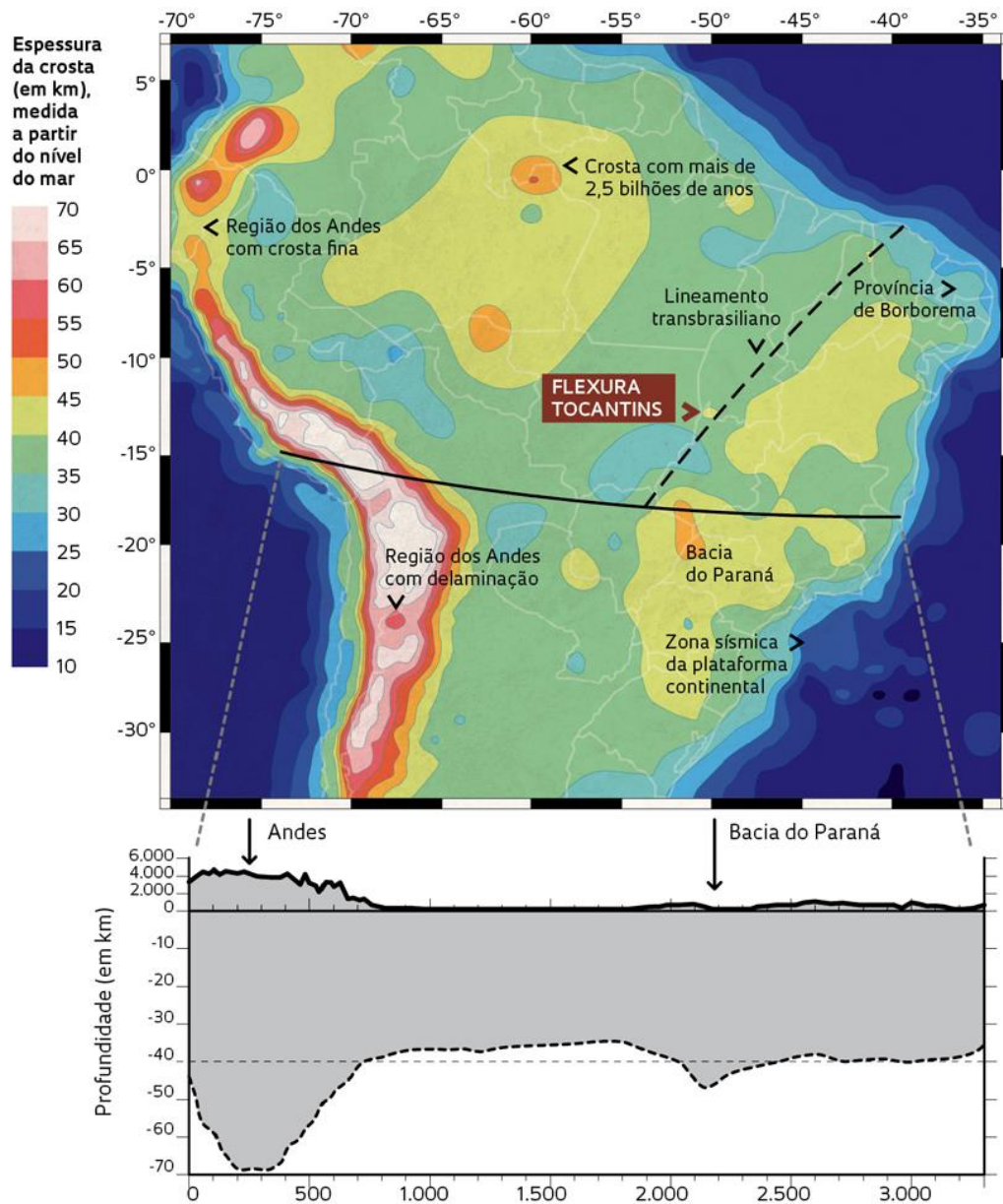
Figura 4.7 - Sob a terra. Levantamento mostra a diferença de espessura da crosta terrestre no Brasil e na cordilheira dos Andes (distância em Km).
