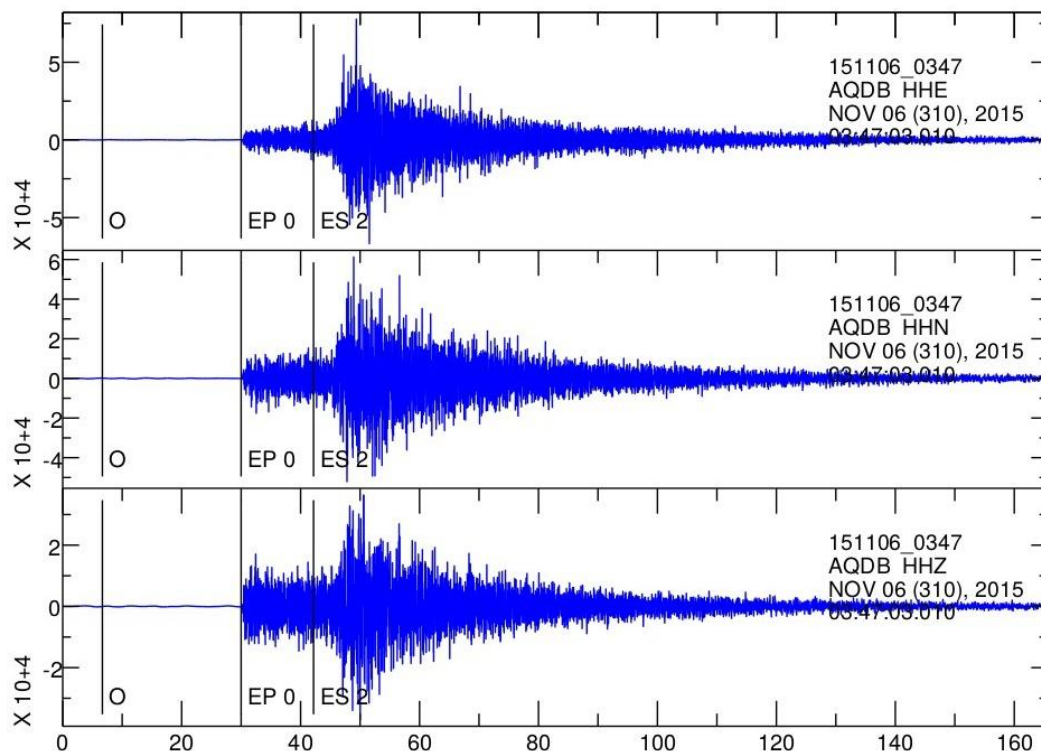
Figura 4.4 - Registro típico de um sismo realçando os tempos de chegada de uma onda P, onda S, o intervalo de tempo entre elas e a chegada posterior de uma onda Love. Na onda S é destacada a medida de sua amplitude, parâmetro para alguns cálculos de magnitude.
