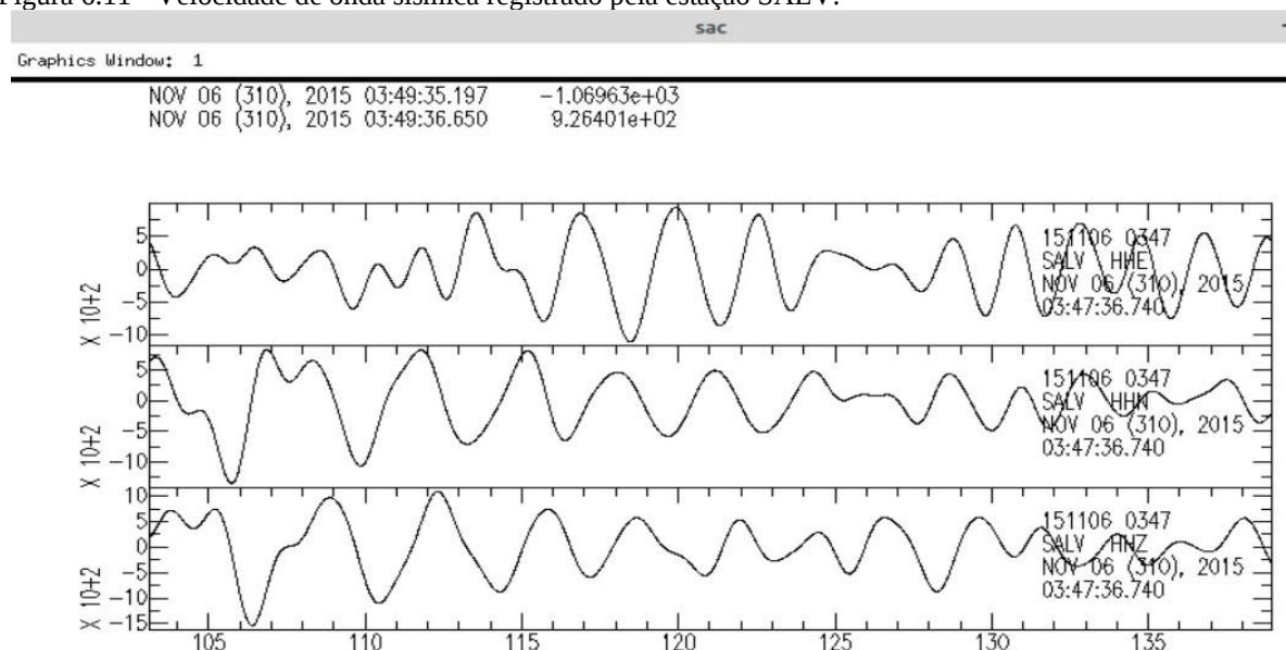
Figura 6.11 - Velocidade de onda sísmica registrado pela estação SALV.
