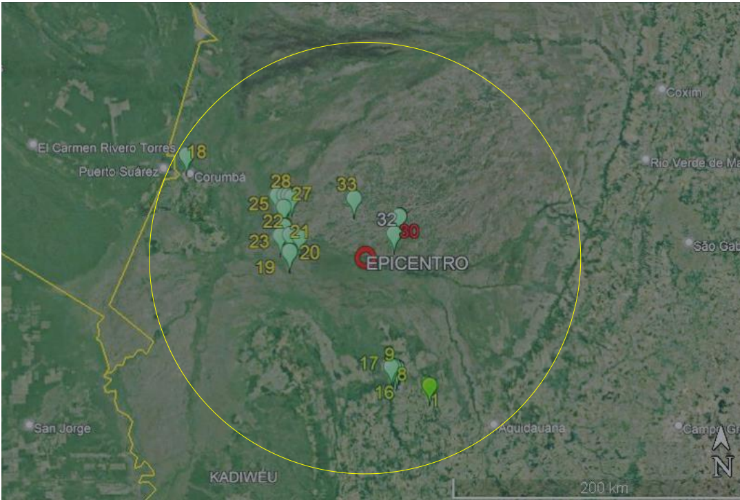
Figura 6.14 - Identificação da região macrossísmica atingida pelo sismo de 6 de novembro de 2015.
