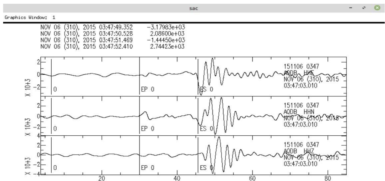
Figura 6.4 - Deslocamento de onda sísmica registrado pela estação AQDB.
