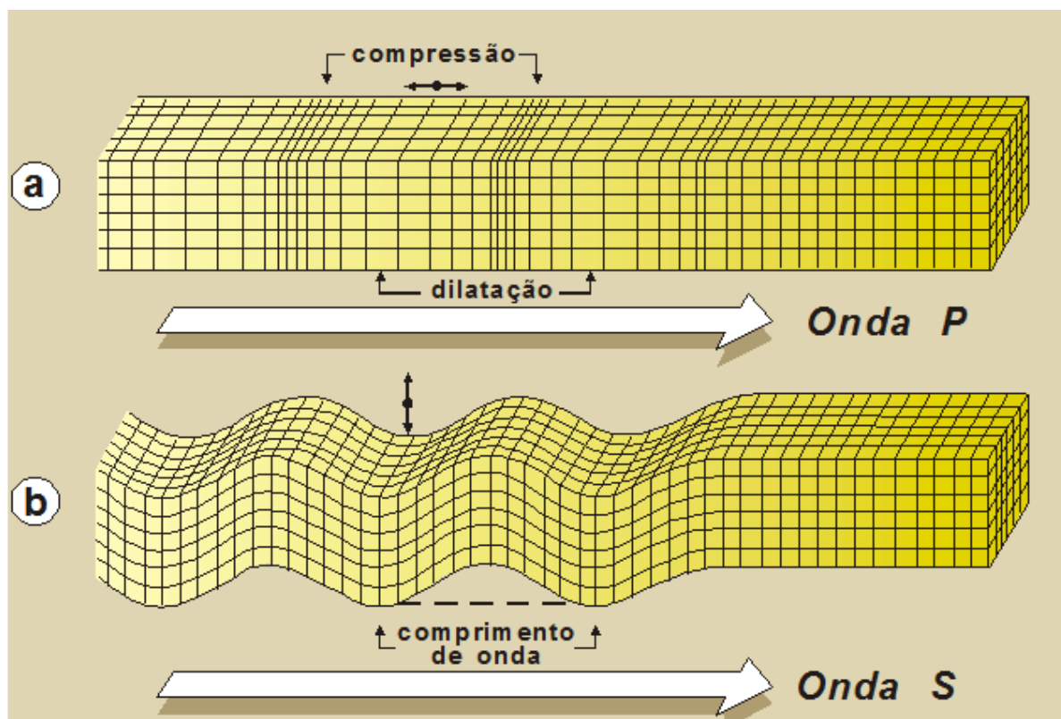
Figura 4.2 - a) Ondas P (longitudinais). b) Ondas S (transversais).
