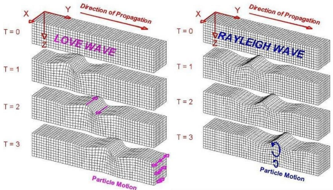
Figura 4.3 - Ondas de superfície Rayleigh e Love. “Y” e a direção radial, ou direção de propagação da onda. “X” e a direção transversal, ou direção horizontal perpendicular a propagação. A oscilação da partícula na onda Rayleigh acontece nos eixos “X” e “Z” sendo uma elipse retrograda no plano vertical radial. A vibração da partícula na onda Love e na direção “X”.
