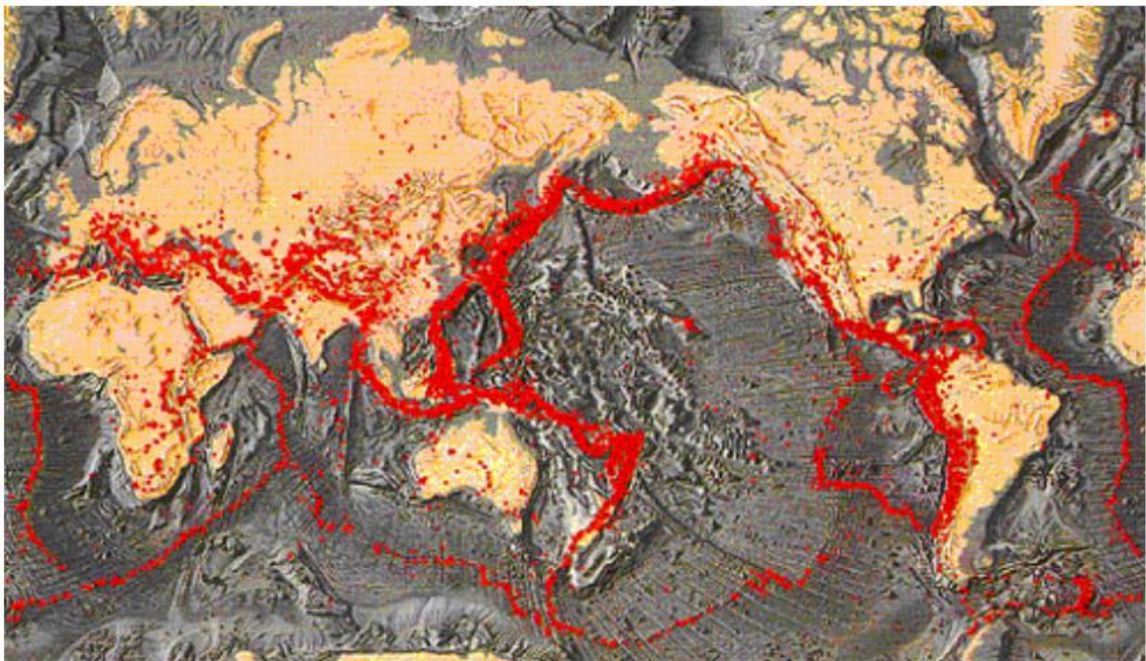
Figura 4.5- Mapa de distribuição dos sismos no mundo, destacados em vermelho e a configuração das placas litosféricas litosféricas.
