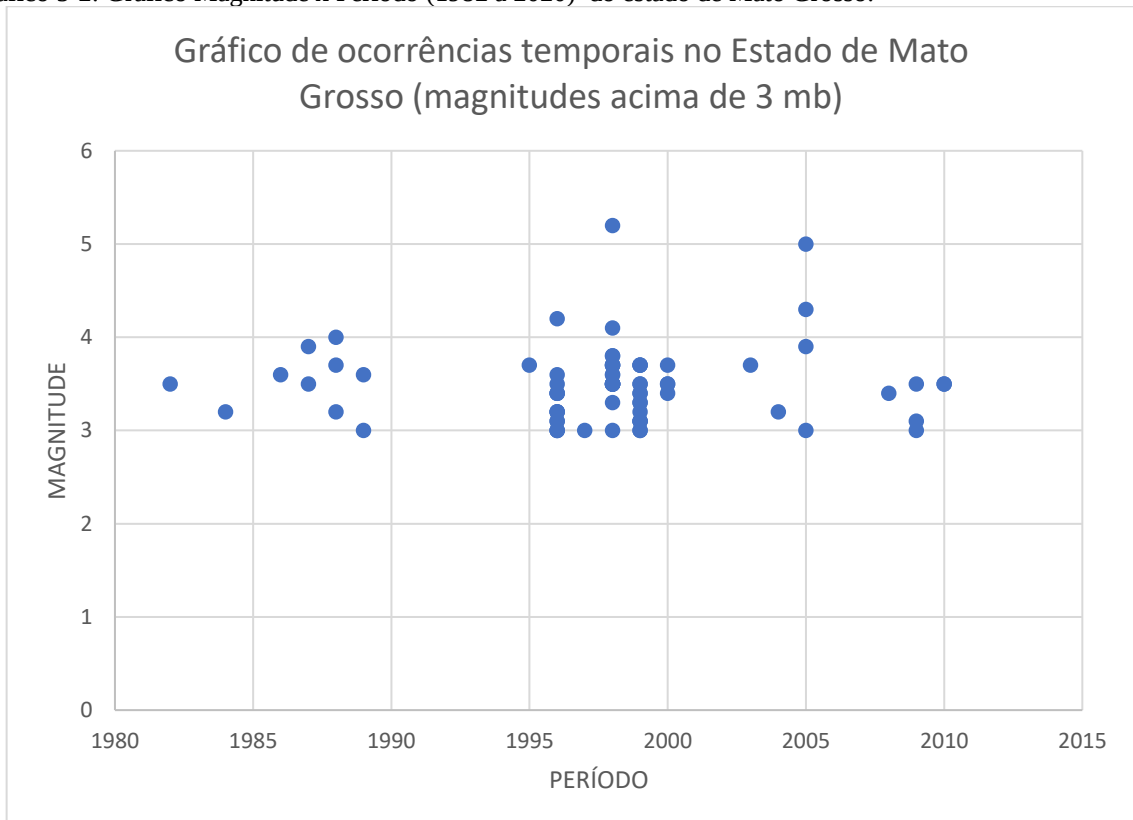
Gráfico 5-2: Gráfico Magnitude x Período (1982 a 2020) do estado de Mato Grosso.
