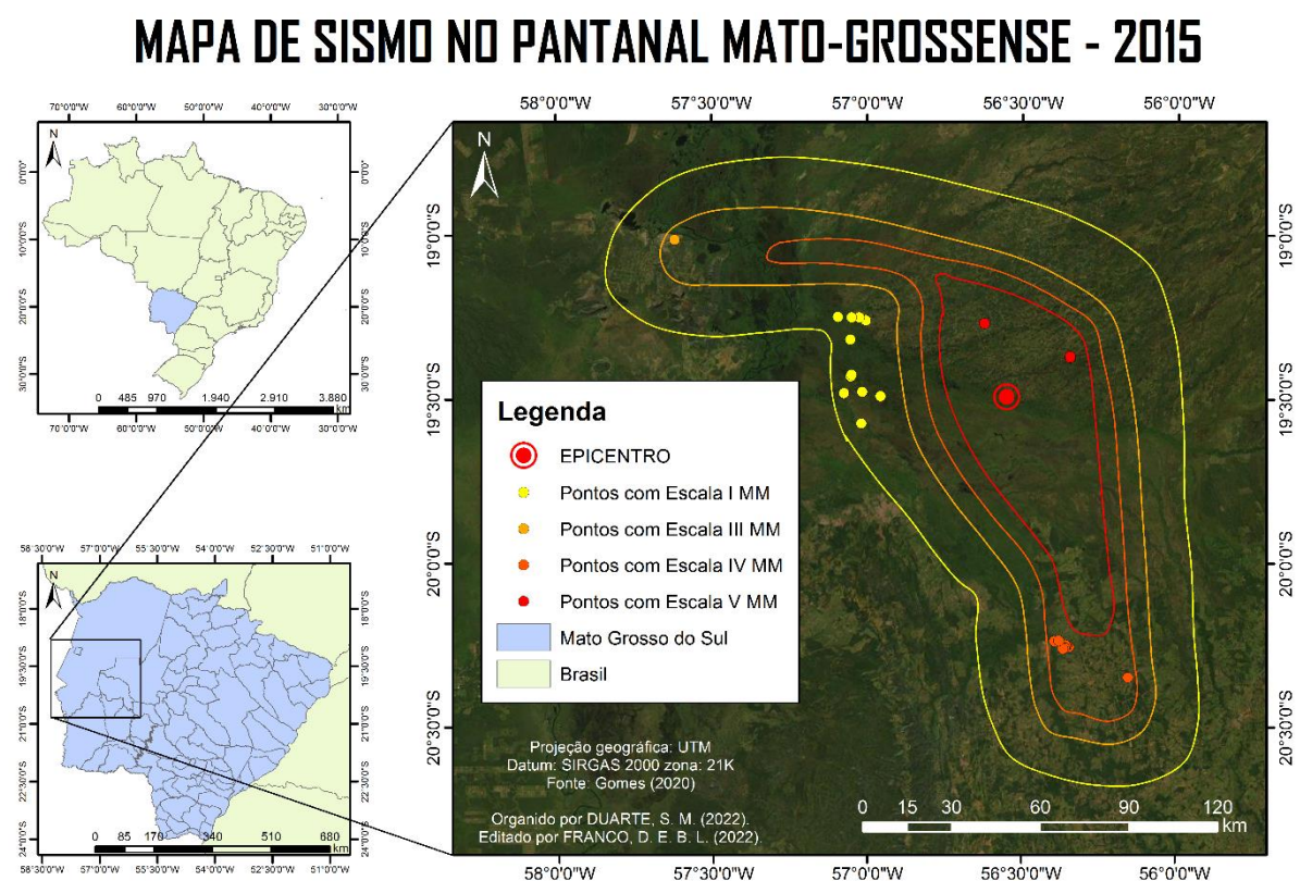
Figura 6.15 - Identificação das regiões de intensidades atingida pelo sismo de 6 de novembro de 2015.
