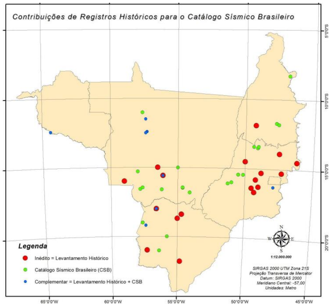
Figura 4.16- Contribuições com o Catálogo Sísmico Brasileiro, após a realização do levantamento de registros históricos da atividade sísmica na região Centro-Oeste do Brasil, segundo Silva 2017-A.
