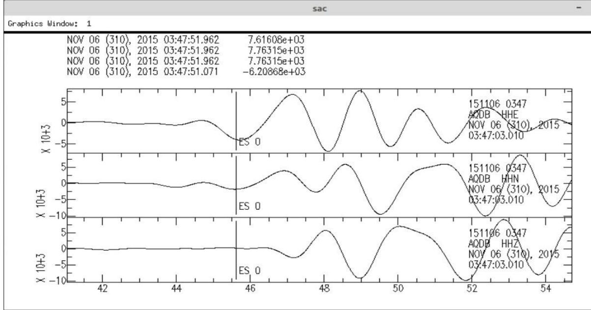
Figura 6.5 - Velocidade de onda sísmica registrado pela estação AQDB.
