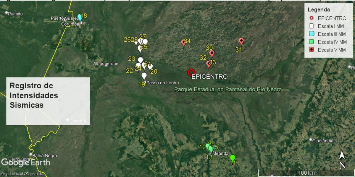
Figura 6.13 - Registros de marcação dos pontos de Intensidade Sísmica, coletados na pesquisa de campo.
