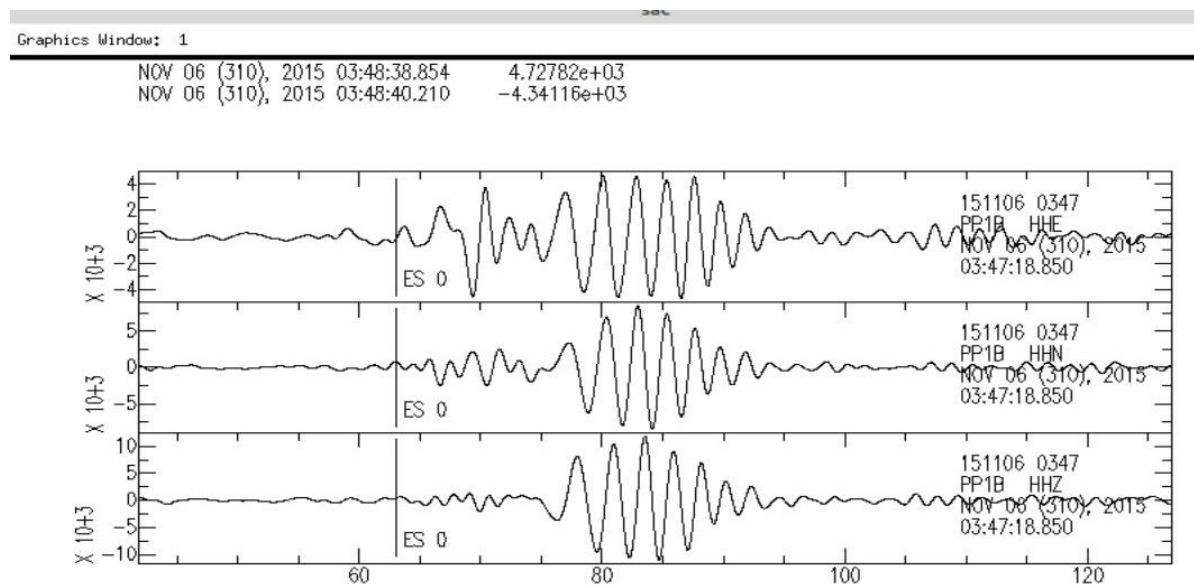
Figura 6.8 - Velocidade de onda sísmica registrado pela estação PP1B
