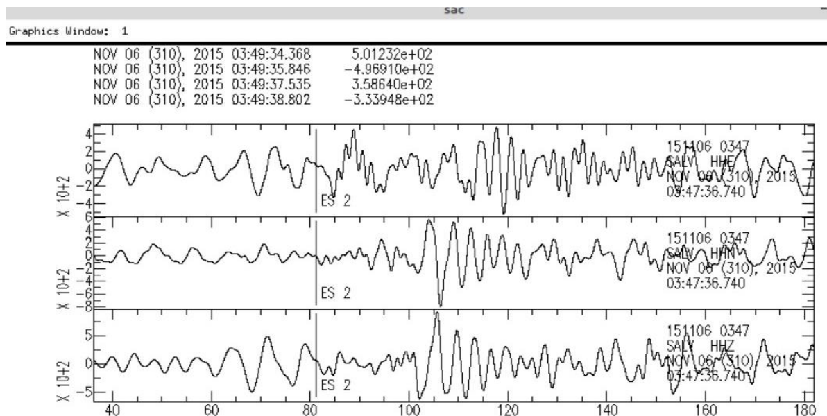
Figura 6.10 - Deslocamento de onda sísmica registrado pela estação SALV.
