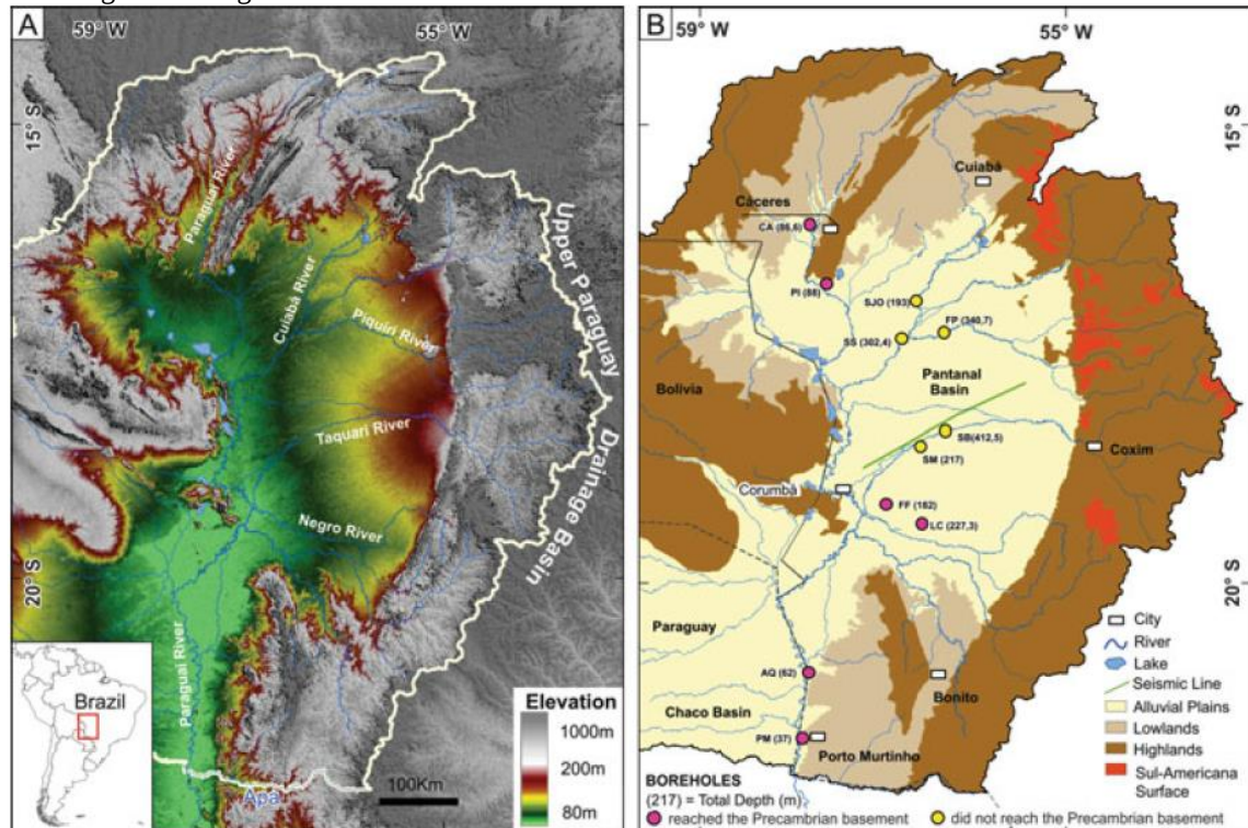
Figura 3.8 - Bacia hidrográfica do Alto Rio Paraguai: A) Modelo digital de elevação (MDE) SRTM (90 m); B) Províncias geomorfológicas da BAP.
