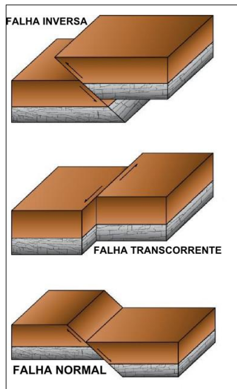
Figura 4.9- Os principais tipos de falhas: normal, inversa e transcorrente.
