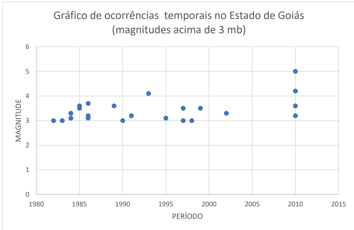
Gráfico 5-3: Gráfico Magnitude x Período (1982 a 2020) do estado de Goiás.
