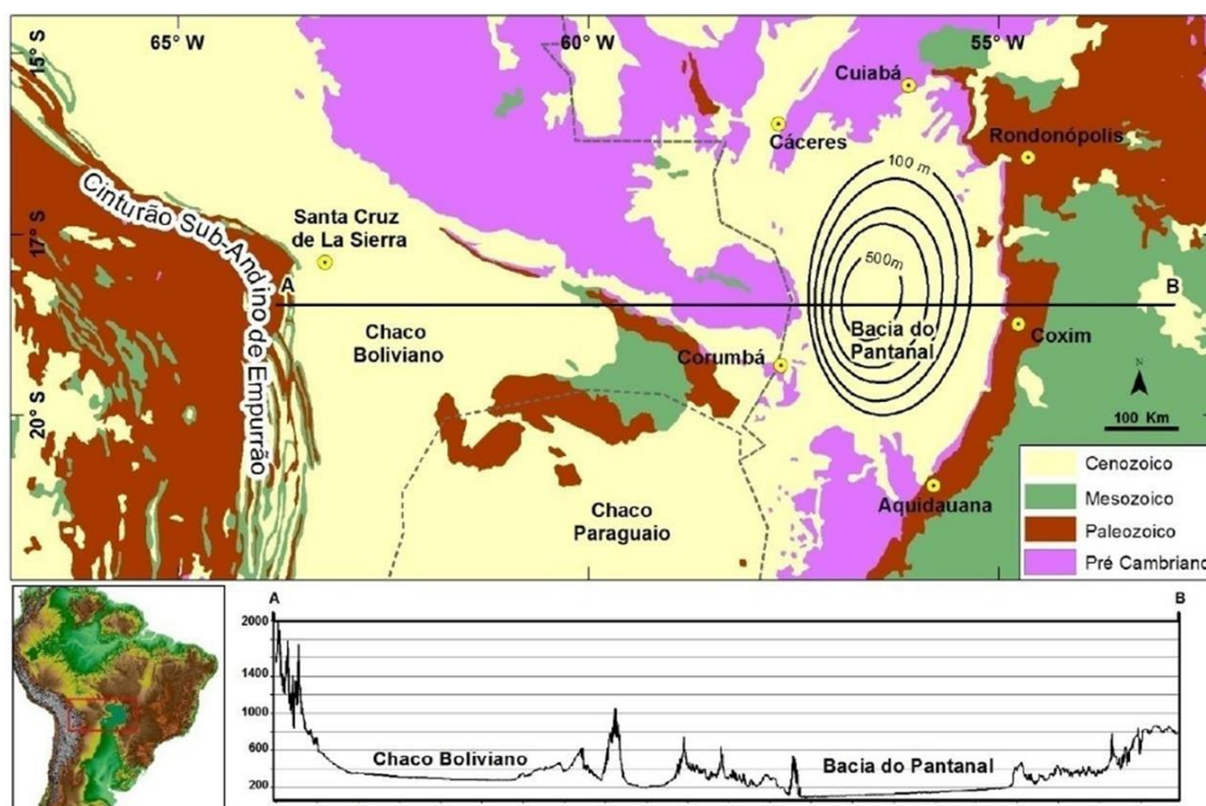
Figura 3.7 - Geologia regional da Bacia do Pantanal e adjacências
