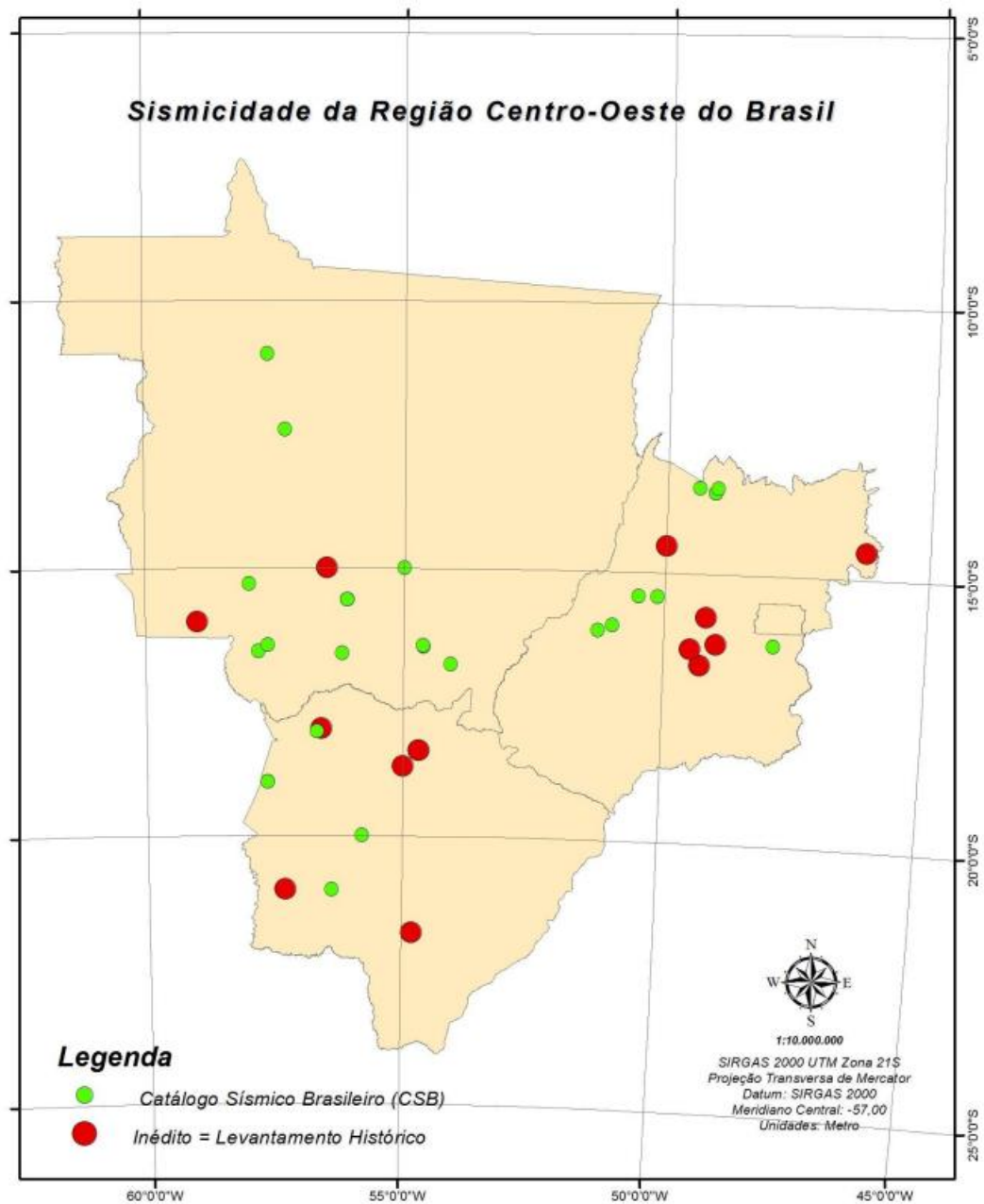
Figura 4.17- Atualização dos registros históricos sobre a sismicidade da Região Centro-Oeste do Brasil. Silva, 2017-A.
