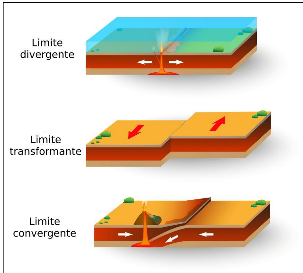
Figura 4.6- Os três tipos de limites de placas tectônicas.
