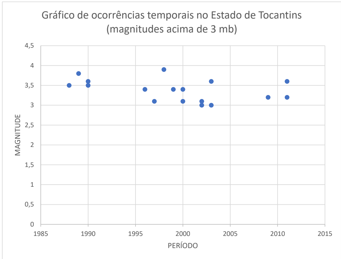
Gráfico 5-1: Gráfico Magnitude x Período (1982 à 2020) do estado de Tocantins.
