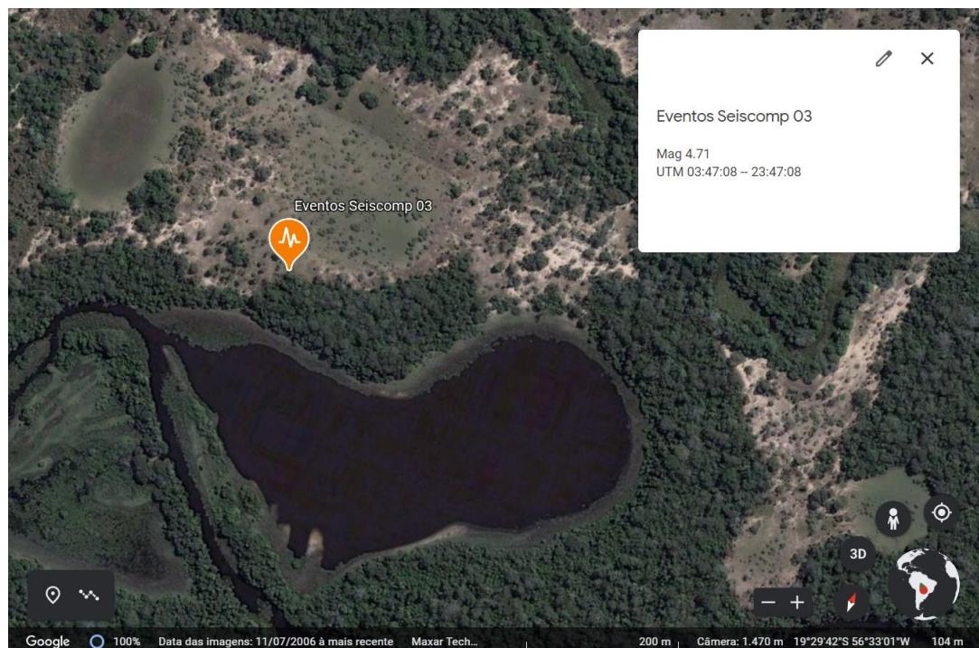
Figura 6.2 - Evento registrado no Seiscomp3 em Miranda-MS.
