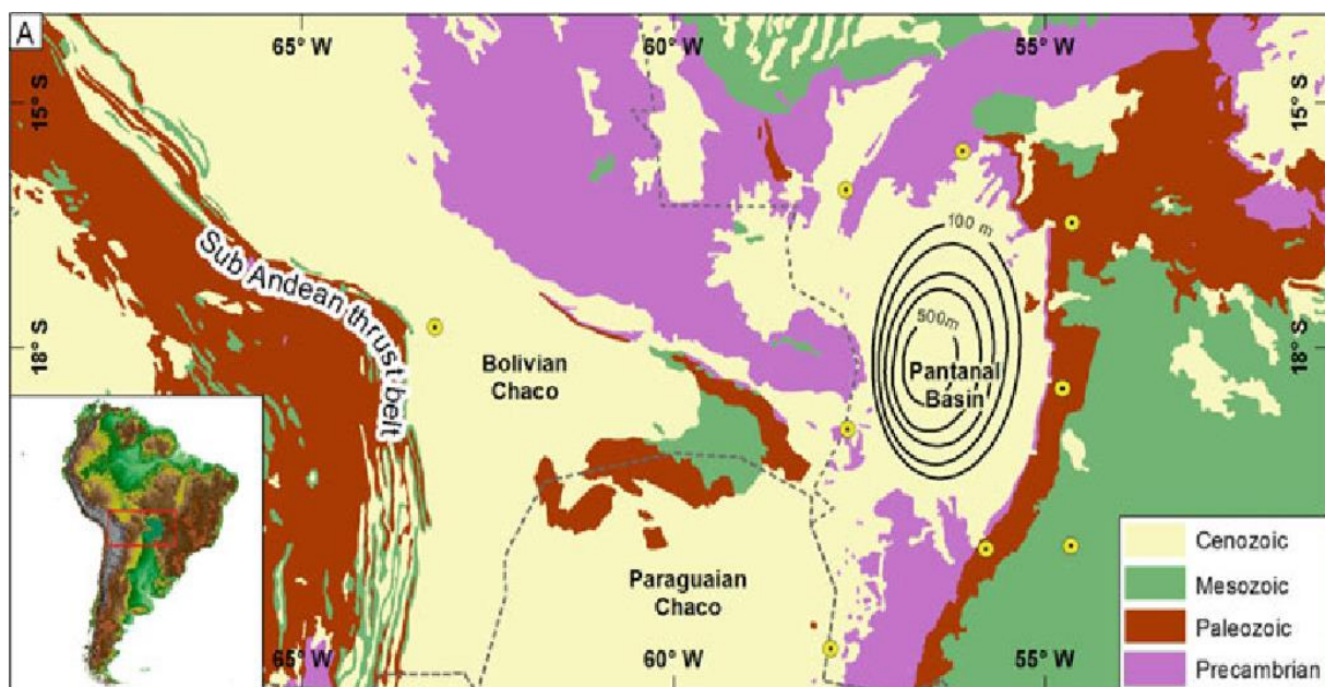
4.10- Localização da Bacia Sedimentar do Pantanal.
