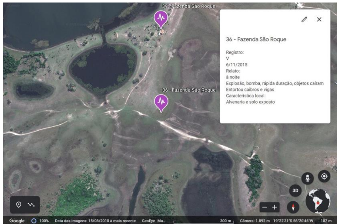
Figura 6.1 - Identificação do local de relato de evento sísmico em Miranda-MS.
