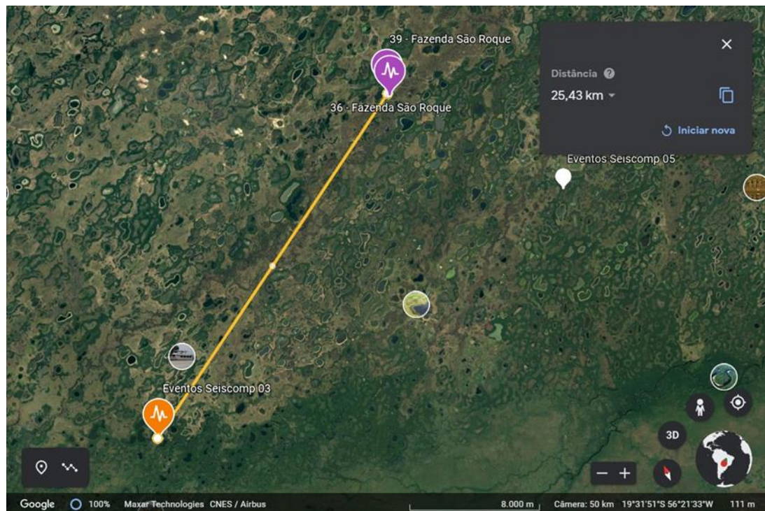
Figura 6.3 - Distância entre os registros de evento na região de Miranda-MS.
