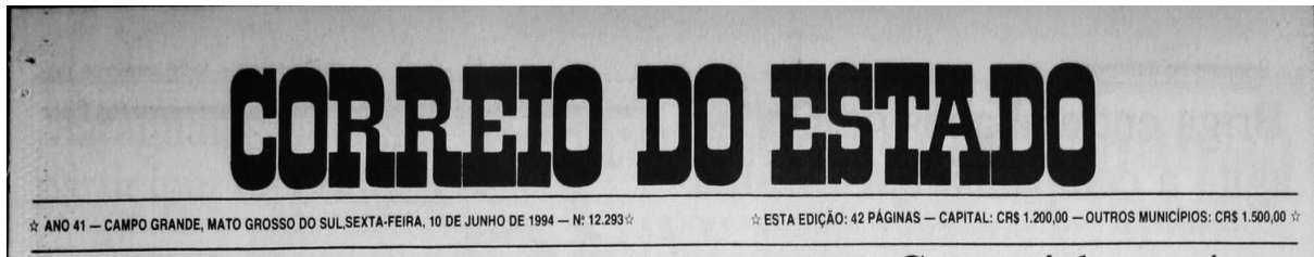
Figura 5.2 - Notícias sobre o temor de terra ocorrido na Bolívia, em 9 de junho 1994 e noticiado no dia 10 de junho de 1994. a) página de capa; b), c), d) e f) estão noticiados nas páginas 09 e 10.
