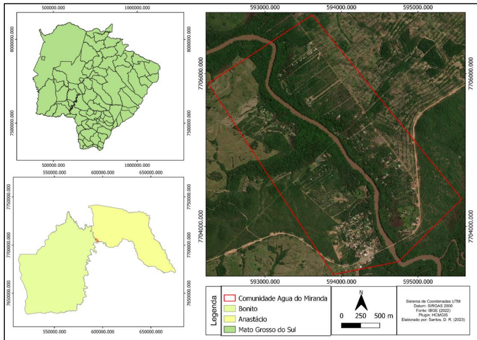
Figura 6: Delimitação da área do distrito de Bonito e Anastácio
