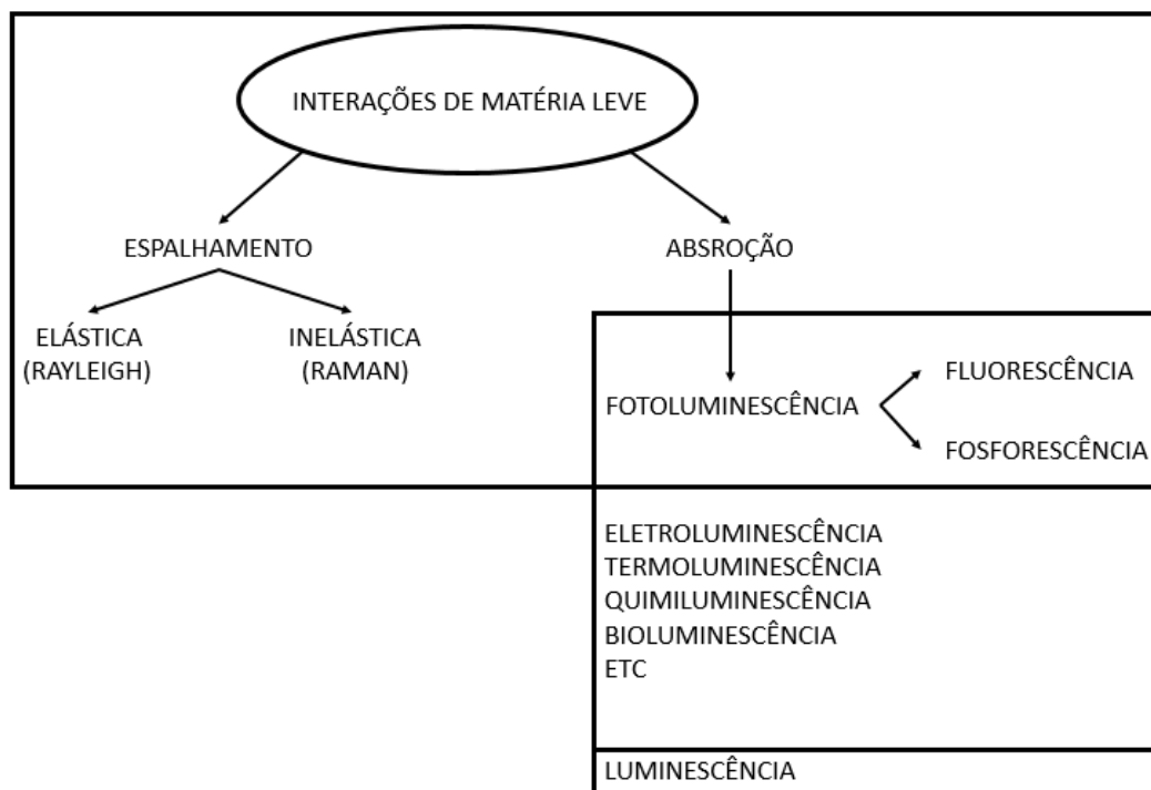
Figura 1 – Posição da Fluorescência e Fosforescência no quadro de Interações de Luz-Matéria. (Valeur et. al. 2001).
