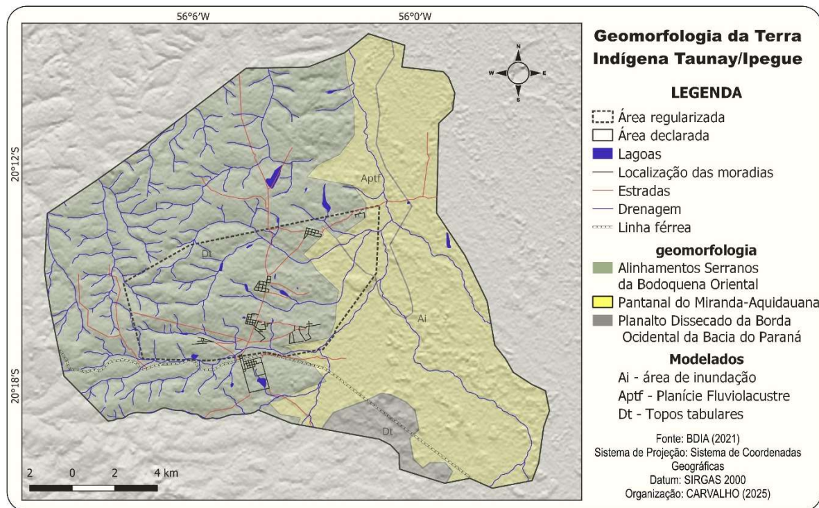
Figura 9 – Mapa de geomorfologia da Terra Indígena Taunay/Ipegue
