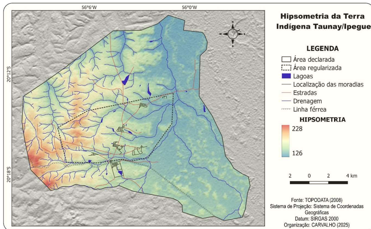
Figura 4 – Mapa hipsométrico da Terra Indígena Taunay/ Ipegue
