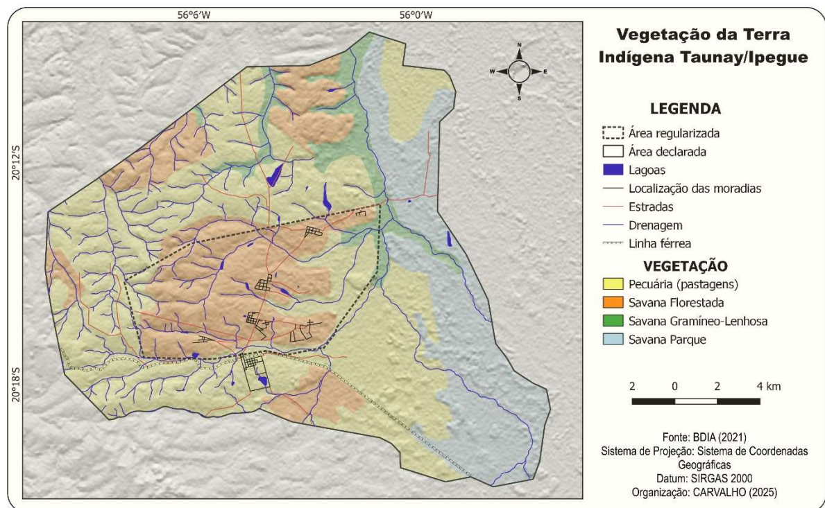
Figura 12 – Mapa de vegetação da Terra Indígena Taunay/Ipegue
