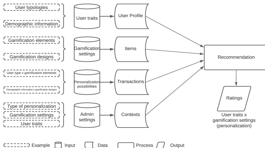
Fig. 2 Framework ReGammend V2. Fonte: Do autor
