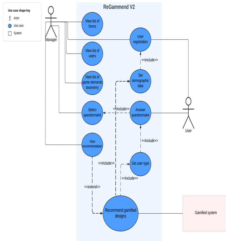
Fig. 5 Casos de Uso. Fonte: Do autor
