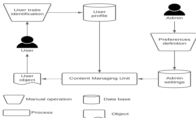
Fig. 3 Architecture ReGammend V2. Fonte: Do autor
