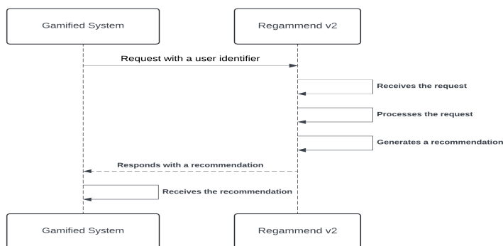
Fig. 1 Fluxo ReGammend V2. Fonte: Do autor
