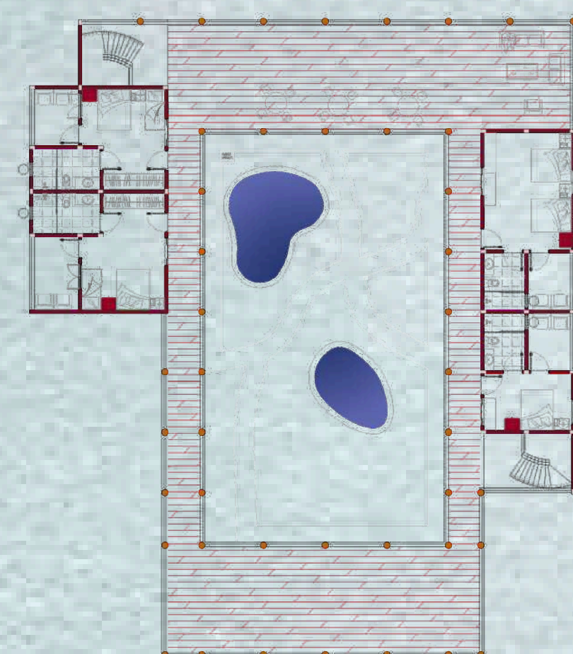
PLANTA BAIXA 1 PAV. - POUSADA
