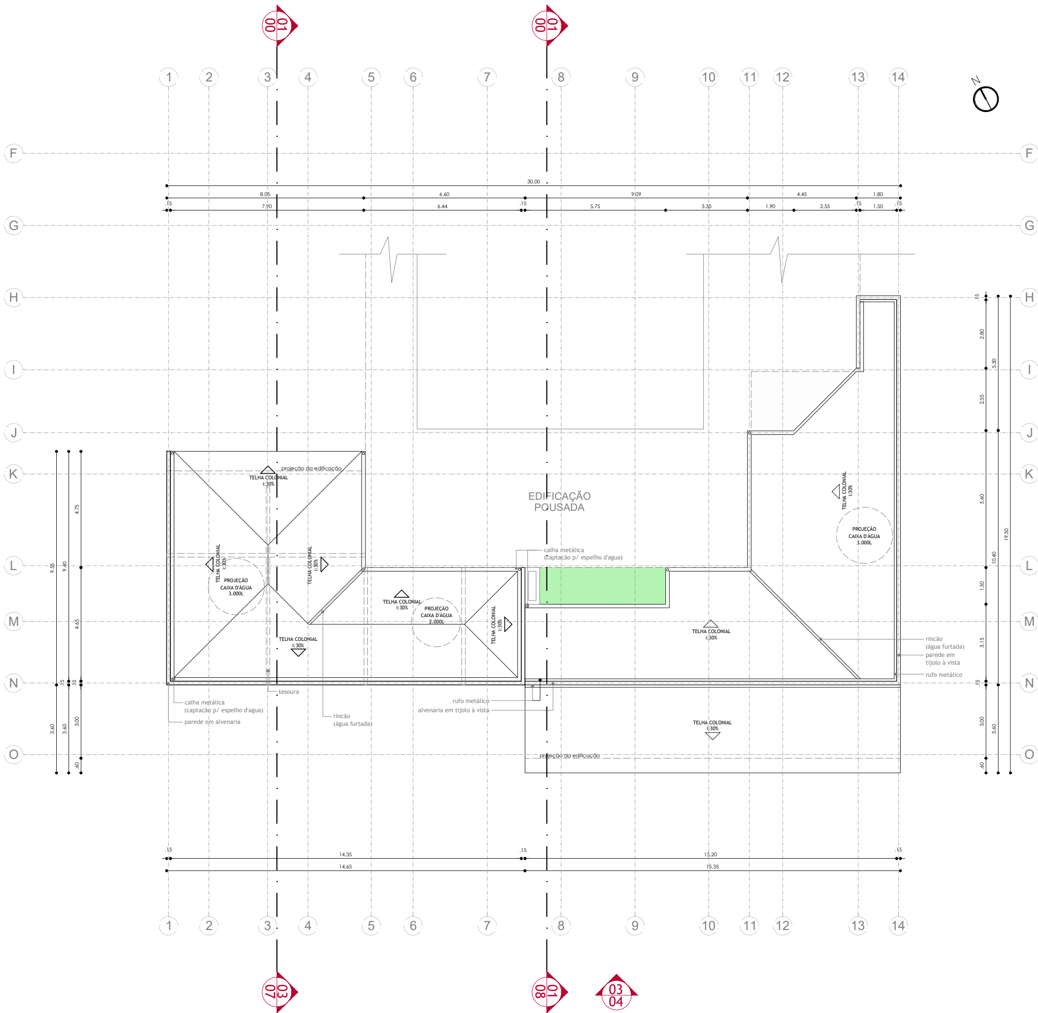
1 PLANTA DE COBERTURA TÉRREA - POUSADA
