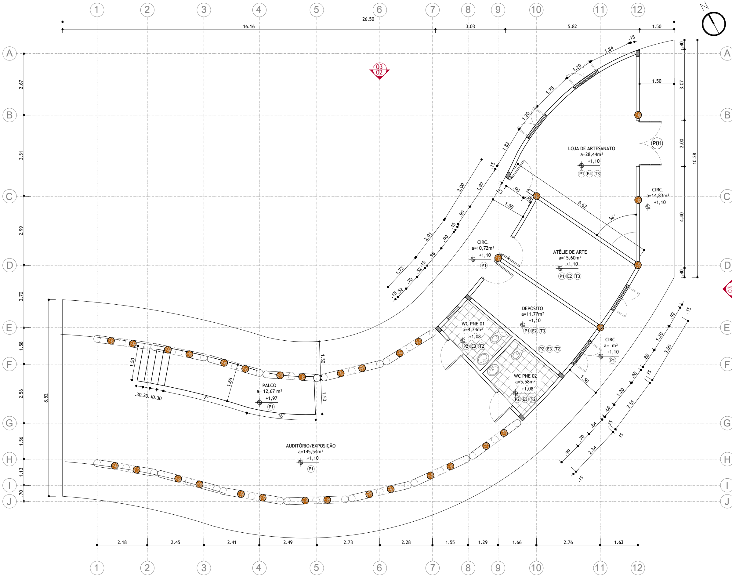
2 PLANTA BAIXA - PAV. EXPOSIÇÃO esc. 1:100
