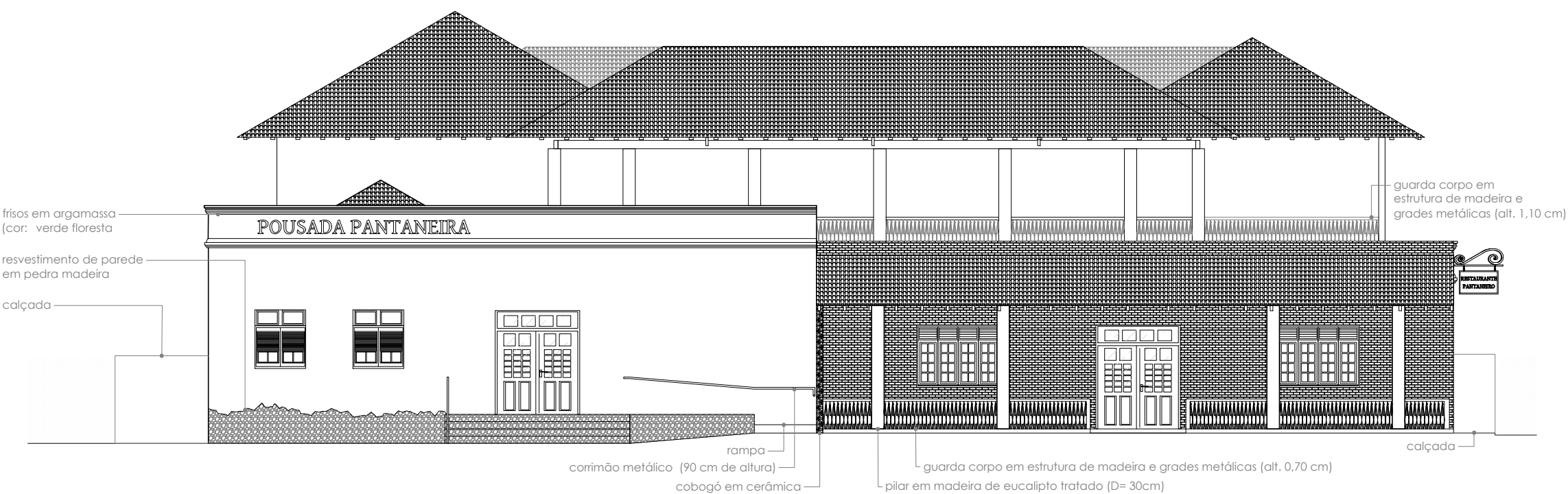
3 FACHADA FRONTAL - POUSADA esc. 1:125
