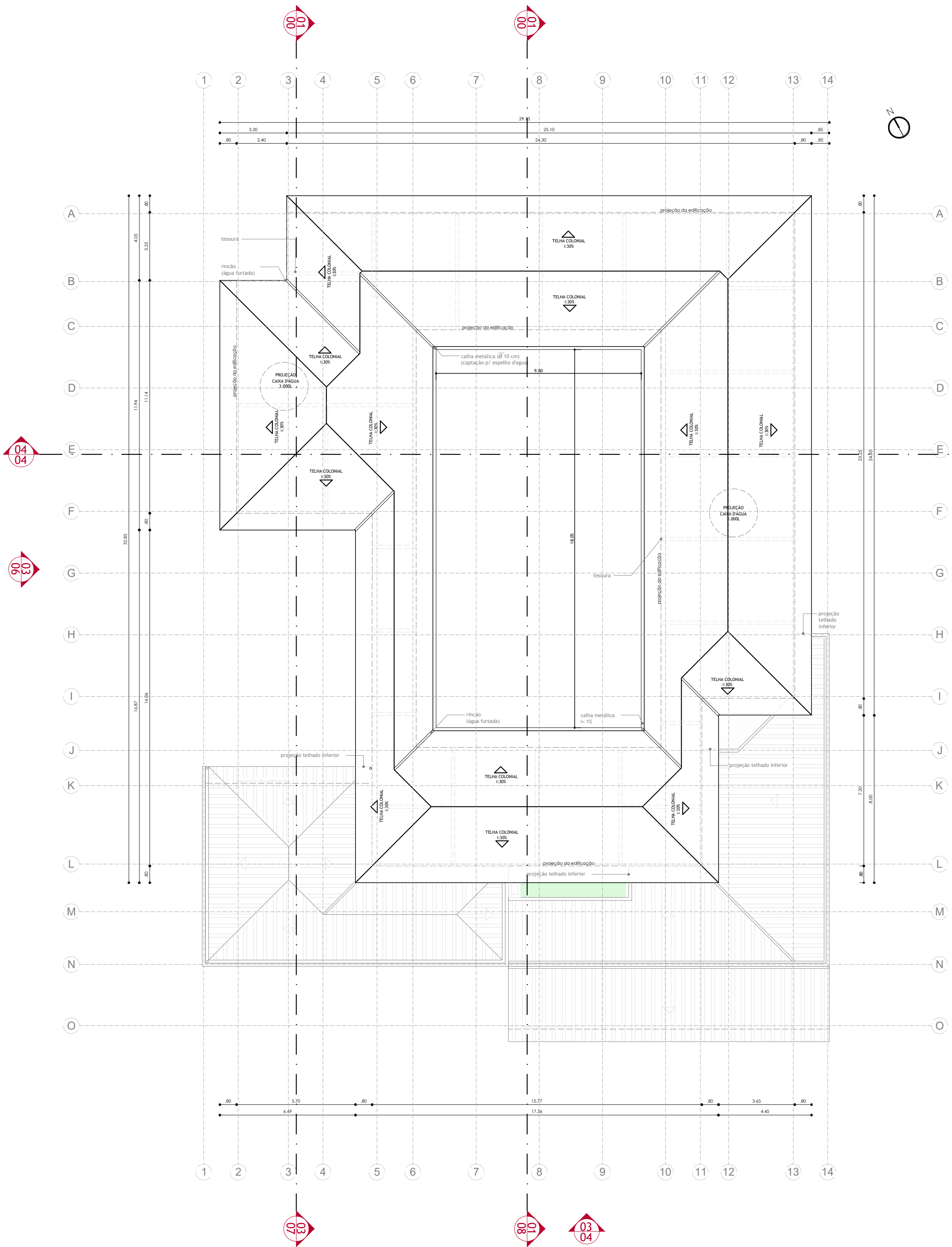
2 PLANTA DE COBERTURA 1 PAV - POUSADA
