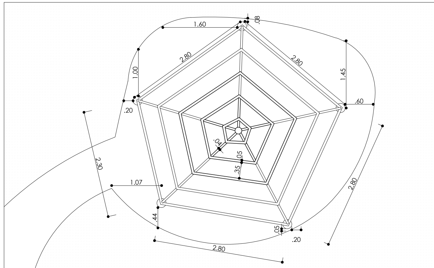
02 PLANTA DE LOCAÇÃO - PERGOLADO
