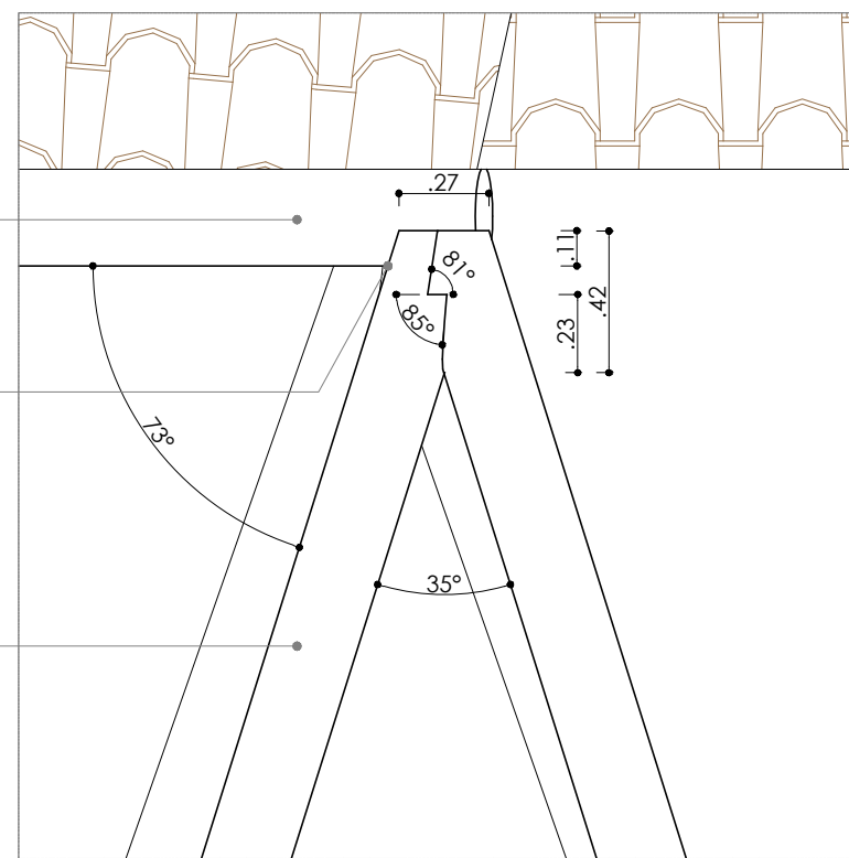
04 DETALHAMENTO - PILAR esc 1:25
