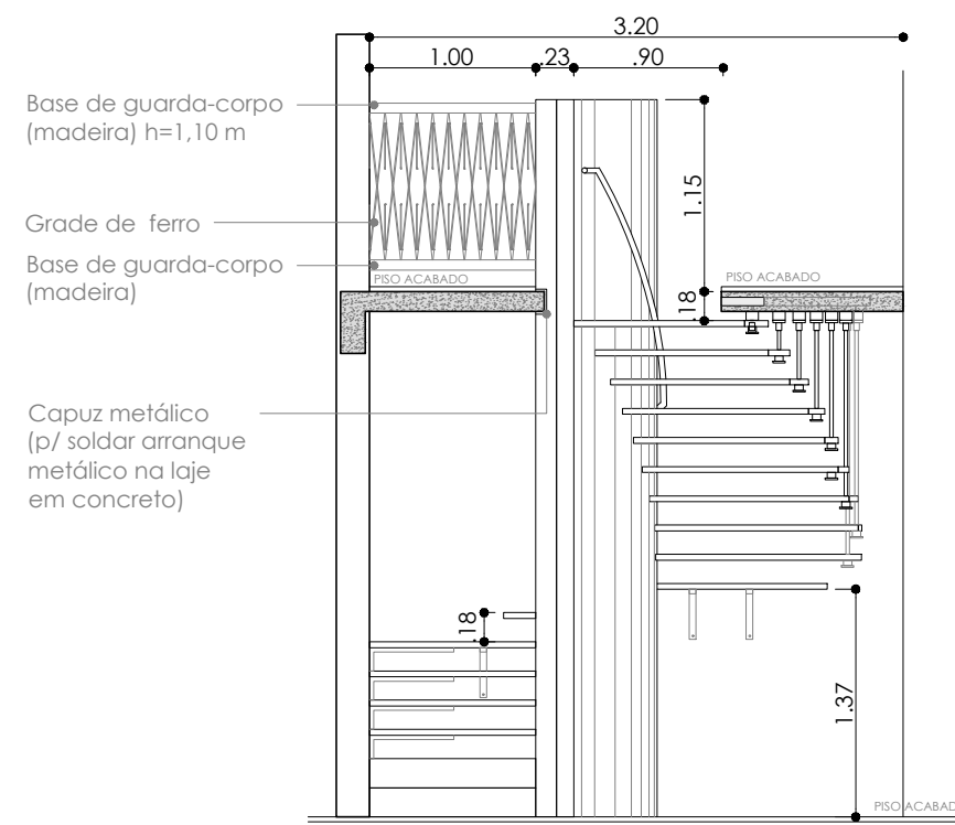
06 ELEVACÃO 01- ESCADA 01
