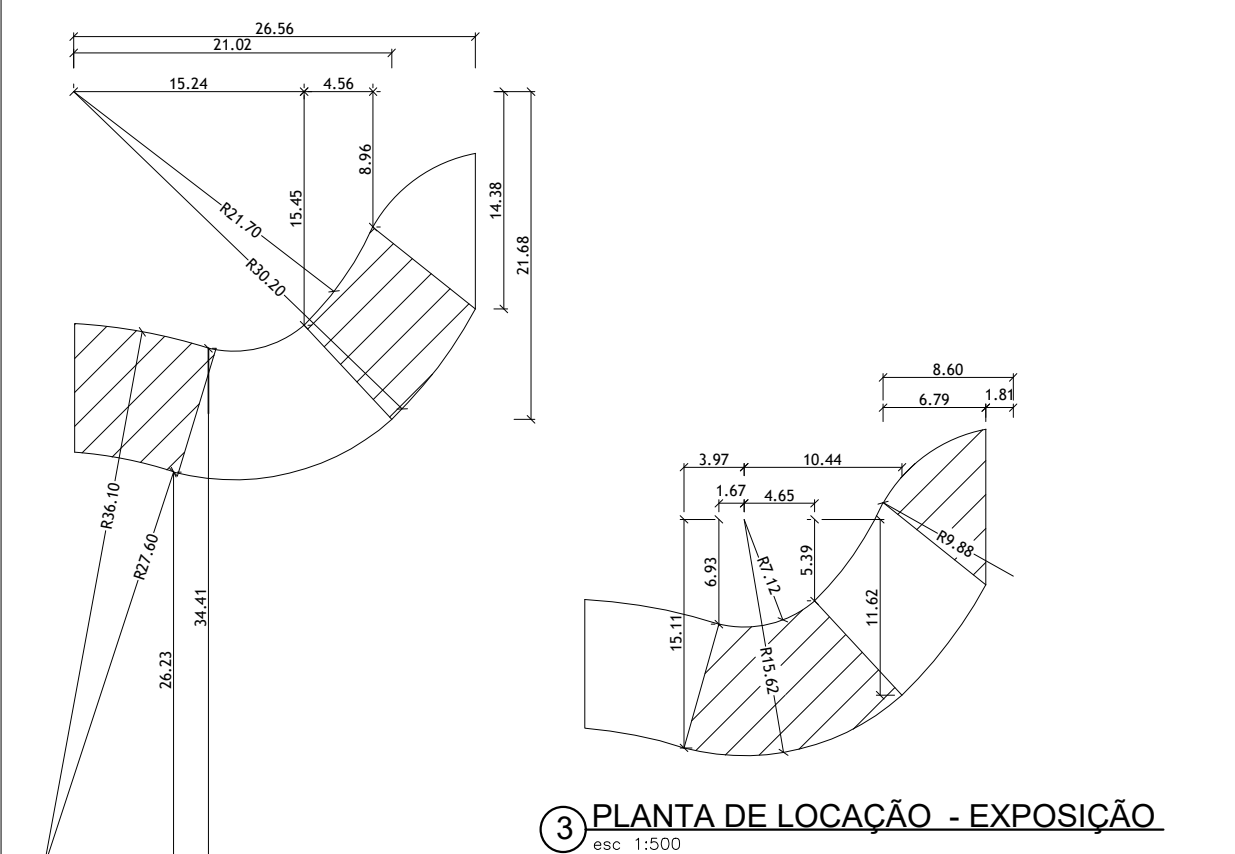
4 PLANTA DE LOCAÇÃO - EXPOSIÇÃO esc 1:500
