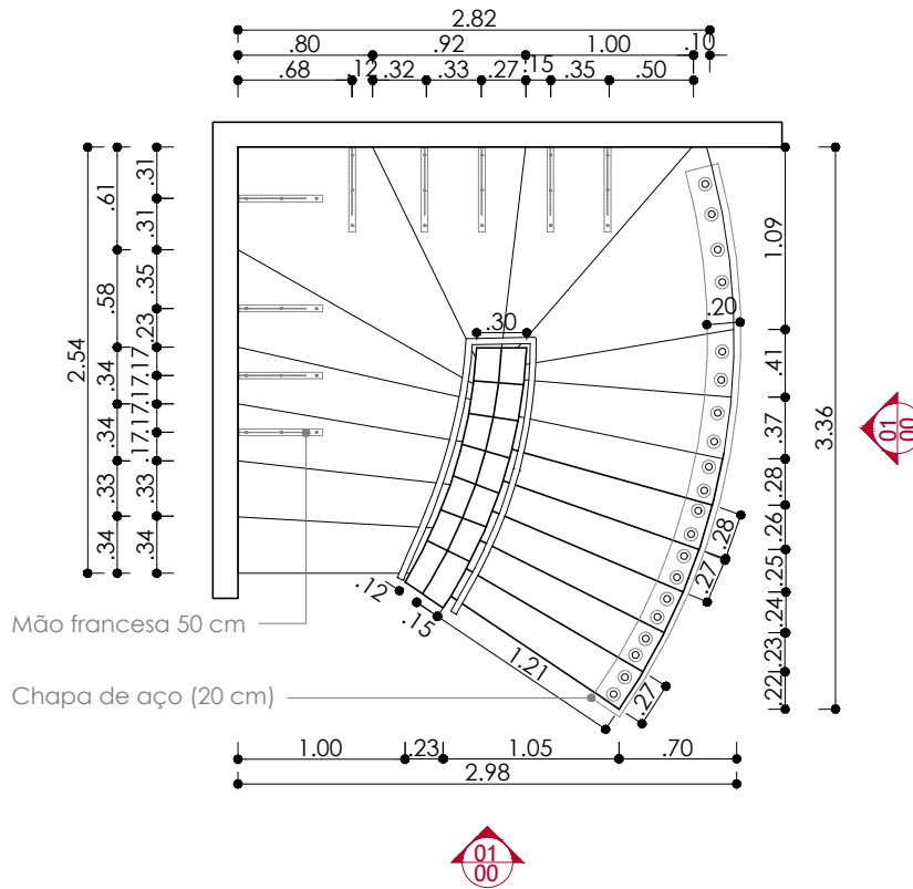
04 PLANTA BAIXA - ESCADA 01
