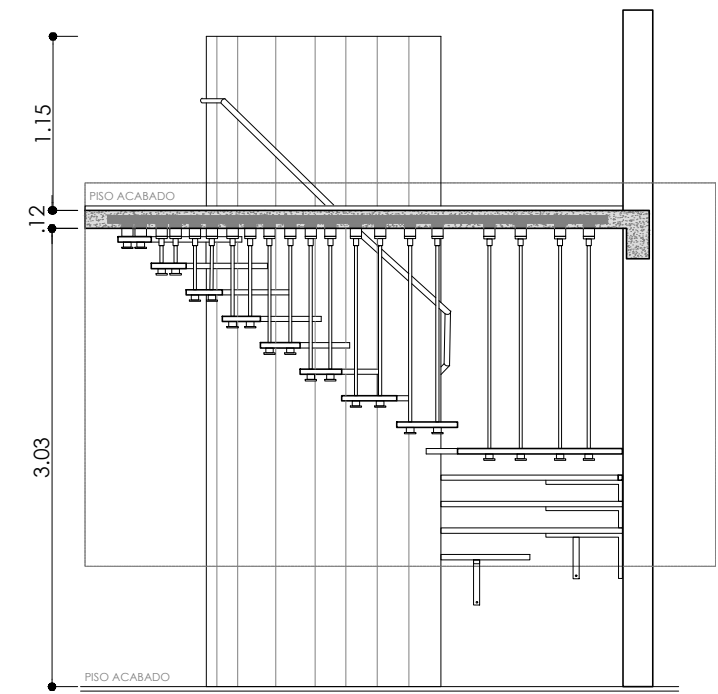
07 ELEVACÃO 02 - ESCADA 01
