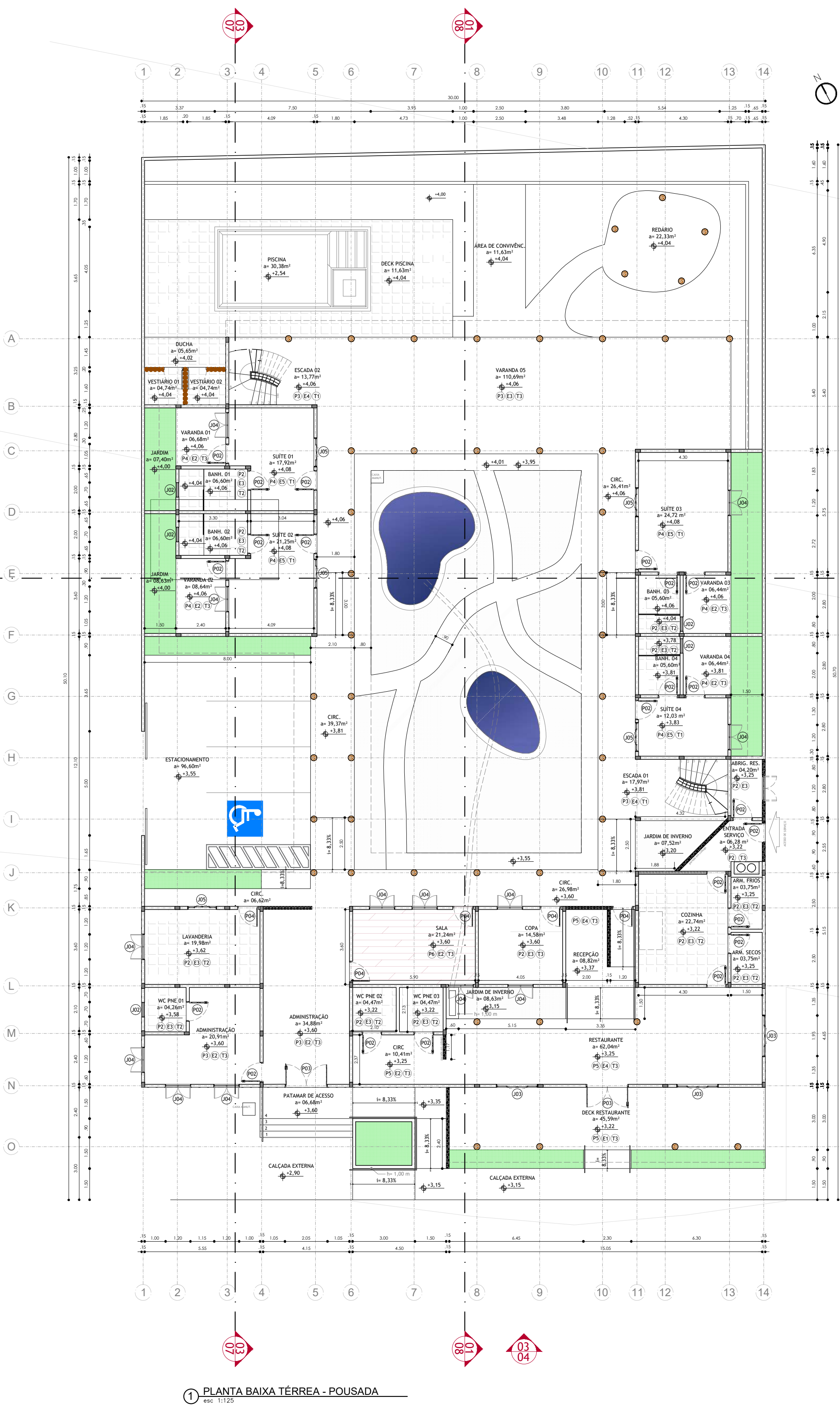
1 PLANTA BAIXA TÉRREA - POUSADA
