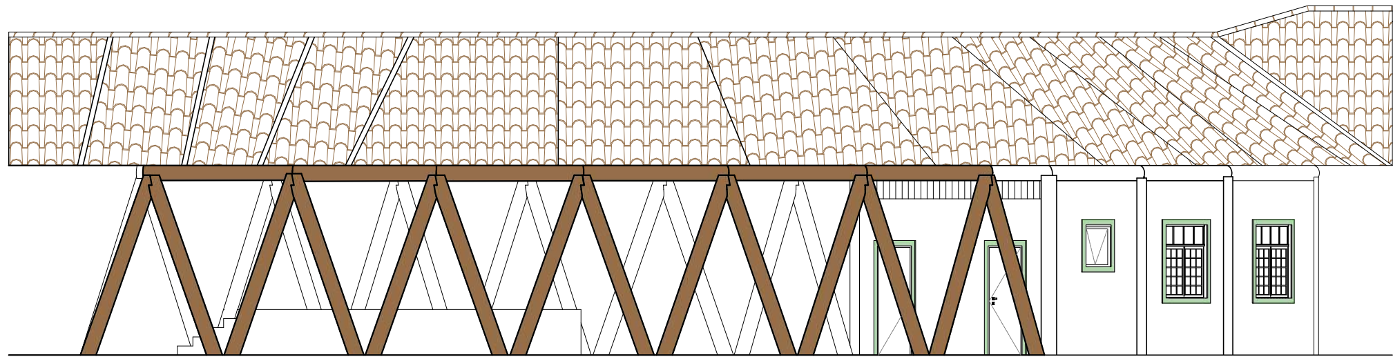
1 FACHADA FRONTAL - PAV ESPOSIÇÃO esc 1:100
