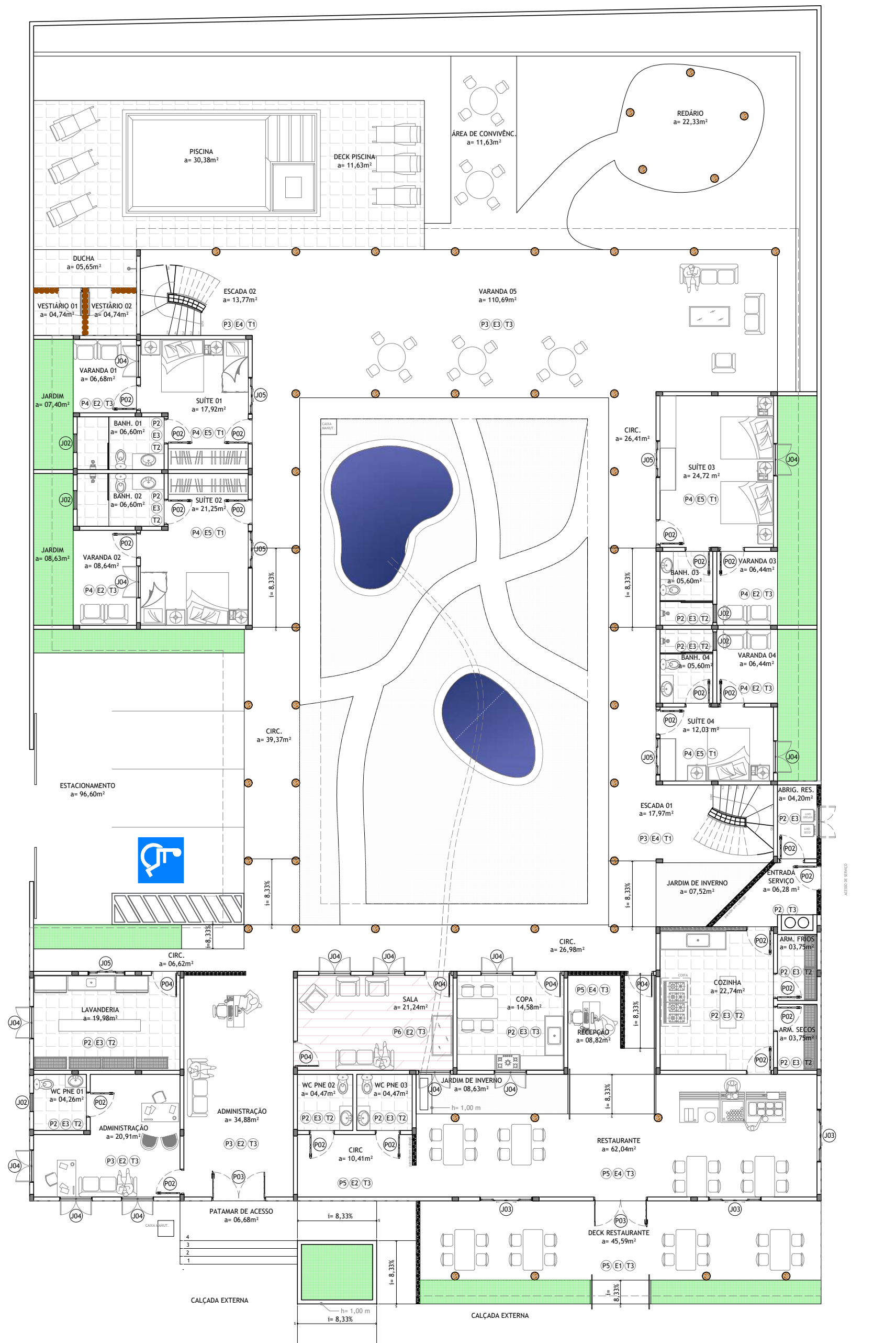
1 PLANTA DE LAYOUT TÉRREA - POUSADA esc. 1:125
