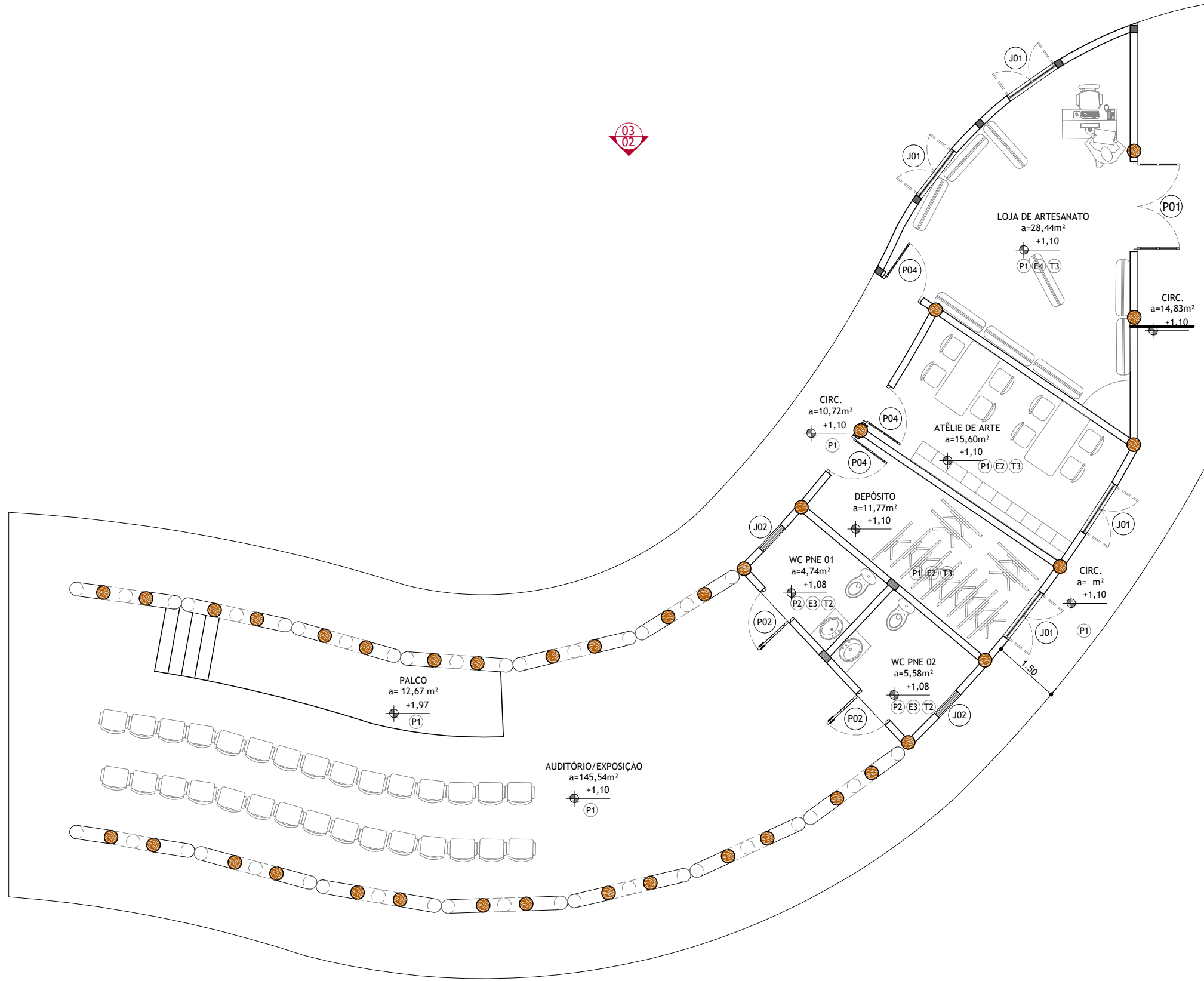
1 PLANTA DE LAYOUT - PAV. EXPOSIÇÃO esc. 1:100
