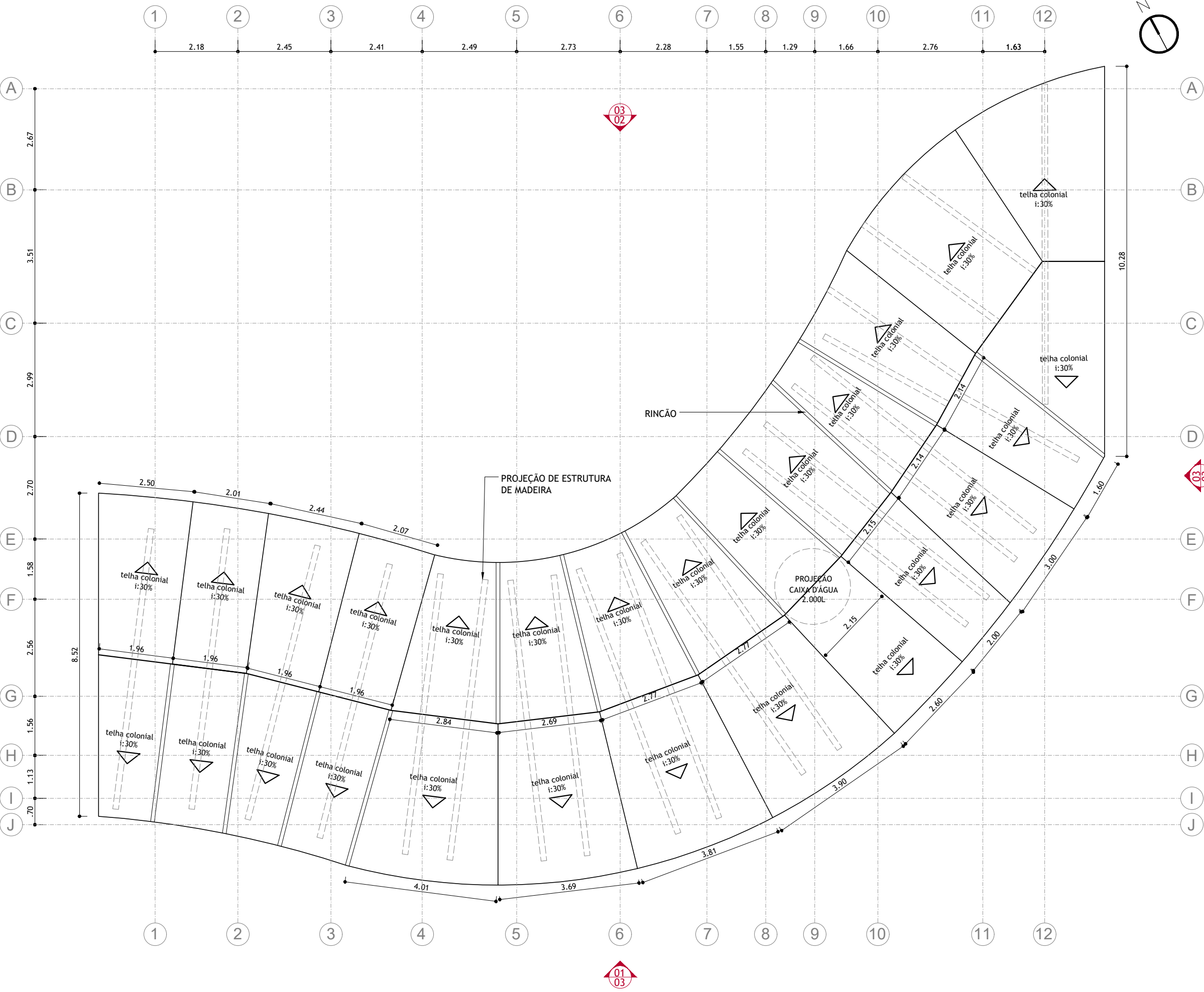
4 PLANTA DE COBERTURA - PAV. EXPOSIÇÃO esc. 1:100
