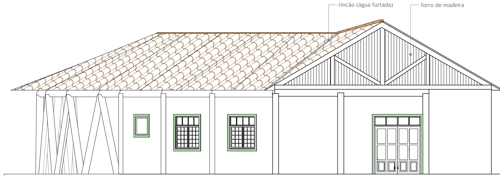
3 FACHADA LAT. DIREITA - PAV ESPOSIÇÃO esc 1:100
