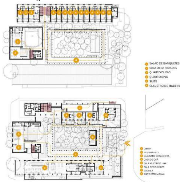
Figura 18: Planta com estudo de fluxos
