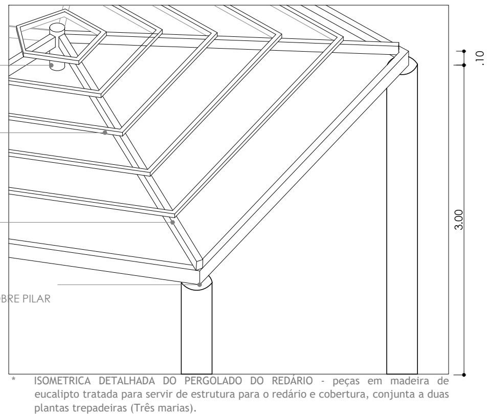
03 DETALHAMENTO ISOMETRICO - PERGOLADO
