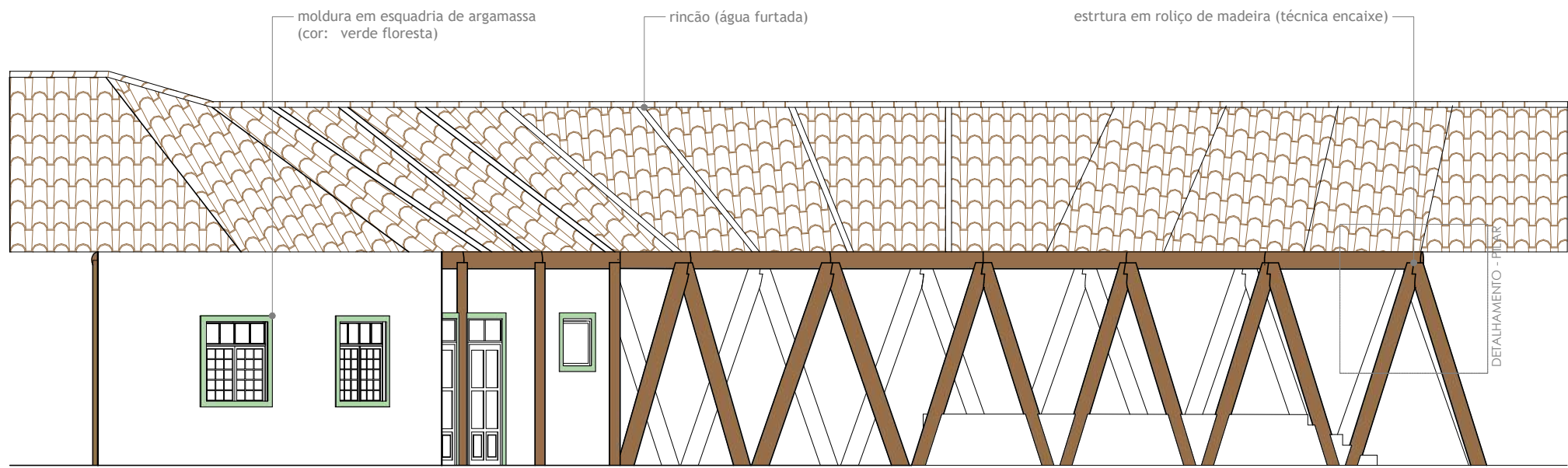
2 FACHADA POSTERIOR - PAV ESPOSIÇÃO esc 1:100
