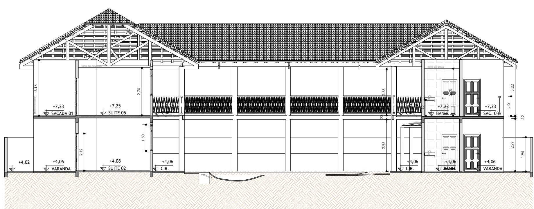
4 CORTE 04 - POUSADA esc. 1:125
