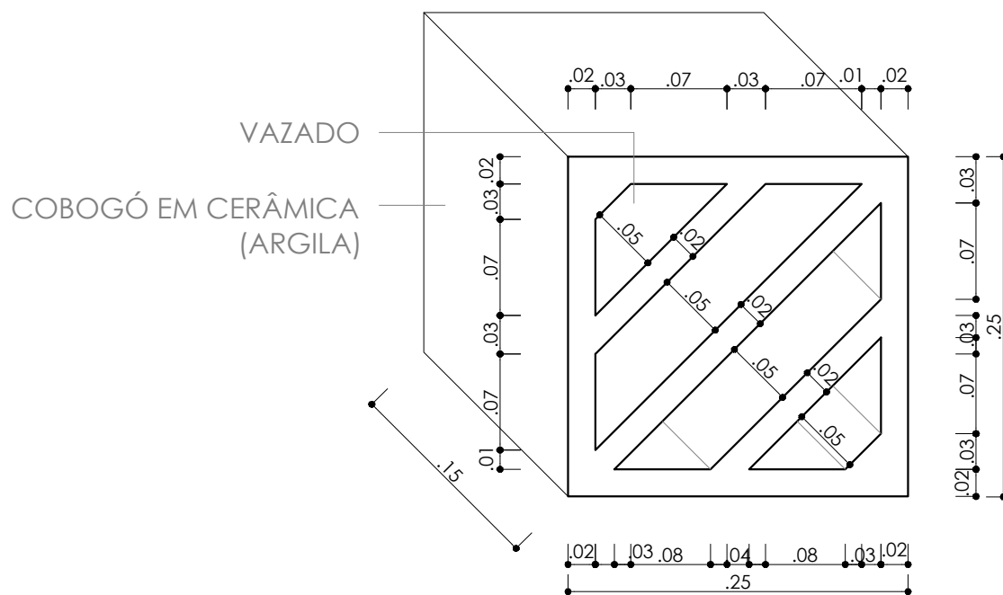
08 DETALHAMENTO COBOGÓ
