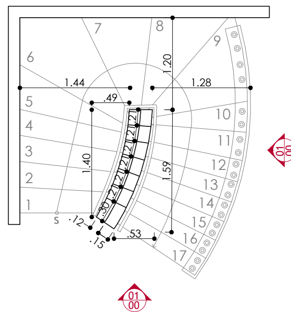
05 PLANTA BAIXA - ESCADA 01
