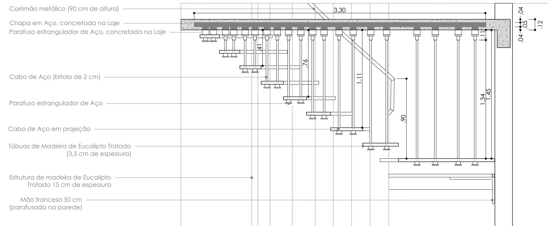
09 DETALHAMENTO - ESCADA 01
