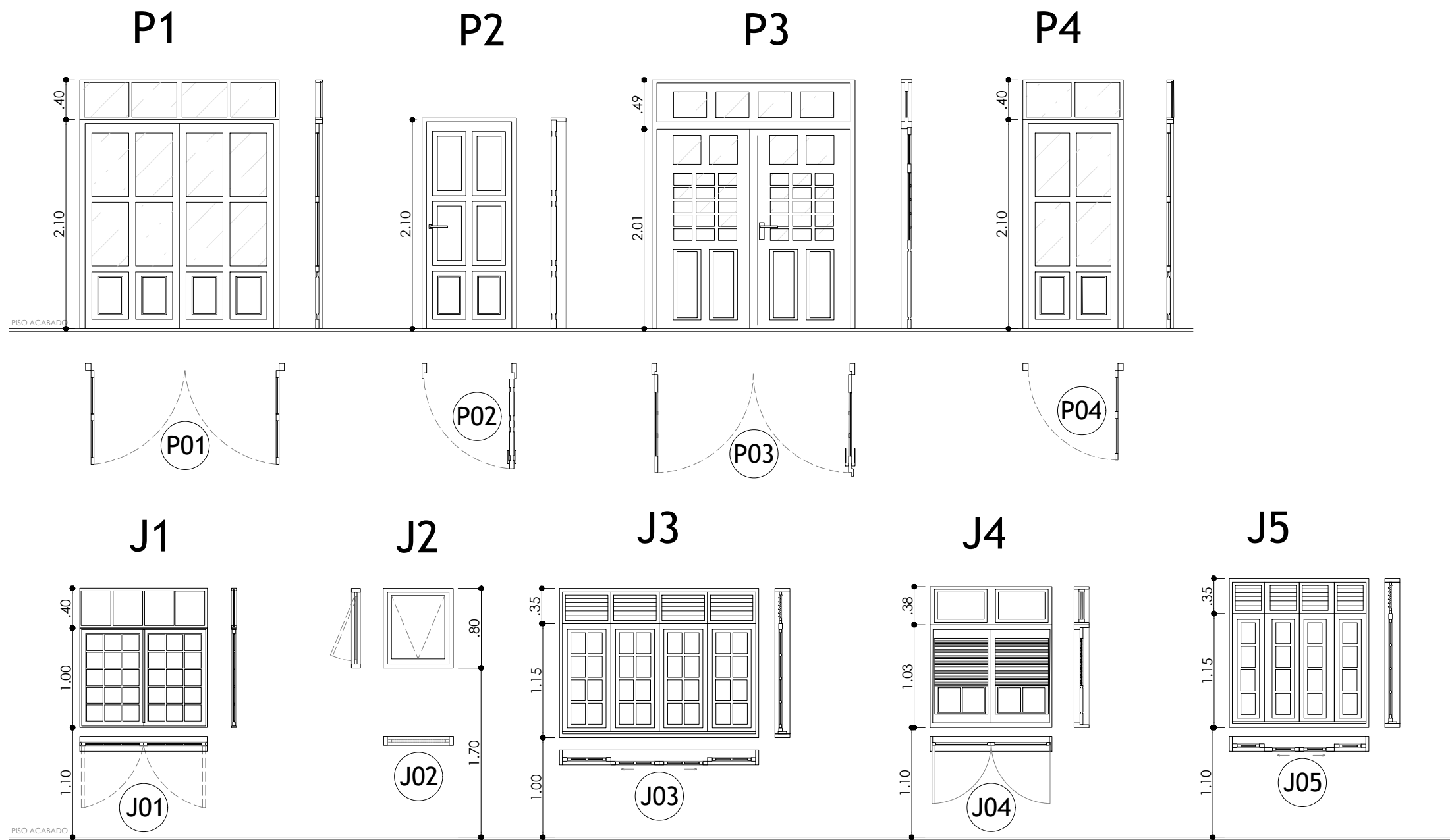
01 DETALHAMENTO ESQUADRIAS esc 1:50
