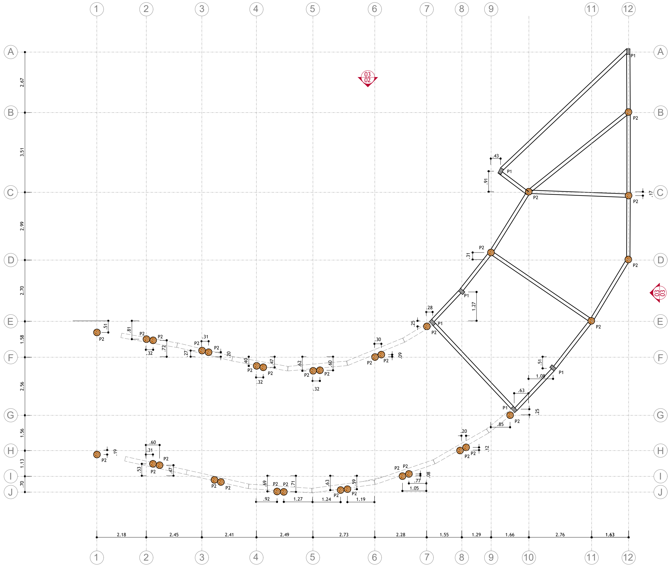
3 PLANTA DE LOCAÇÃO DE PILARES - PAV. EXPOSIÇÃO esc. 1:100
