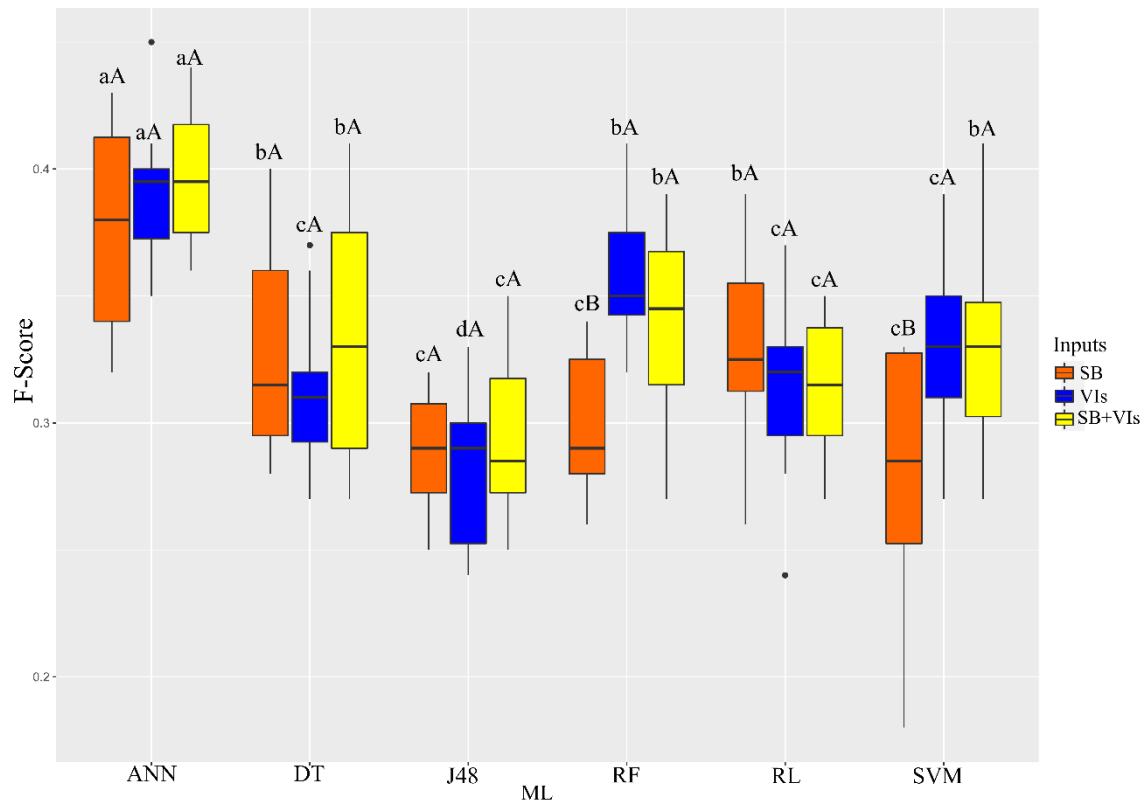
Figura 4. Boxplot para porcentagem de F-Score para a interação significativa entre os modelos de aprendizagem de máquinas e os inputs testados.
