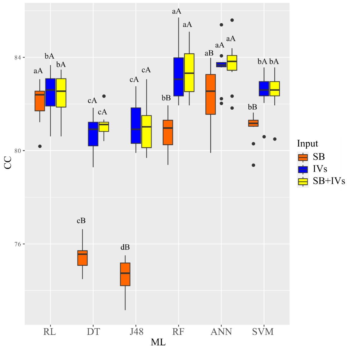
Figura 4. Boxplot para porcentagem de classificação correta (CC) considerando a interação significativa entre os algoritmos de ML e as entradas testadas.
