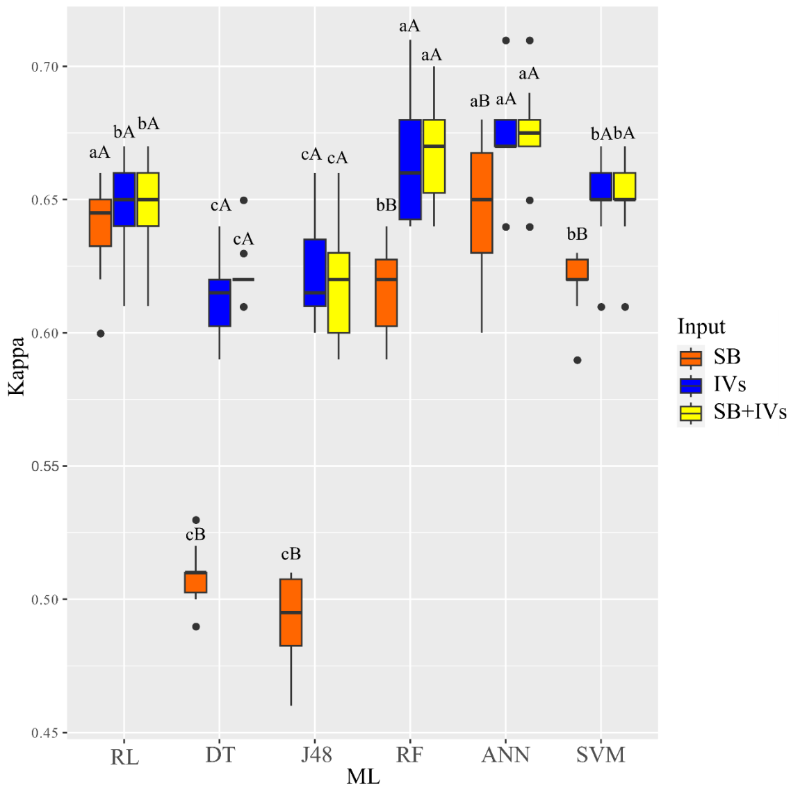
Figura 6. Boxplot para coeficiente Kappa considerando a interação significativa entre os algoritmos de ML e as entradas testadas.
