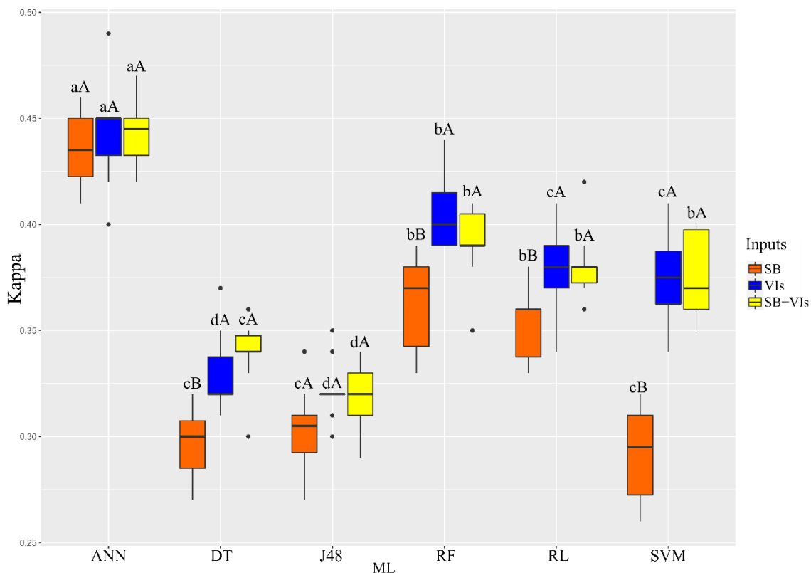
Figura 5. Boxplot para porcentagem de Kappa para a interação significativa entre os modelos de aprendizagem de máquinas e os inputs testados.
