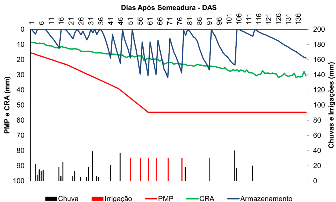
Figura 2. Balanço hídrico irrigado no decorrer da segunda safra 2021/2022.
