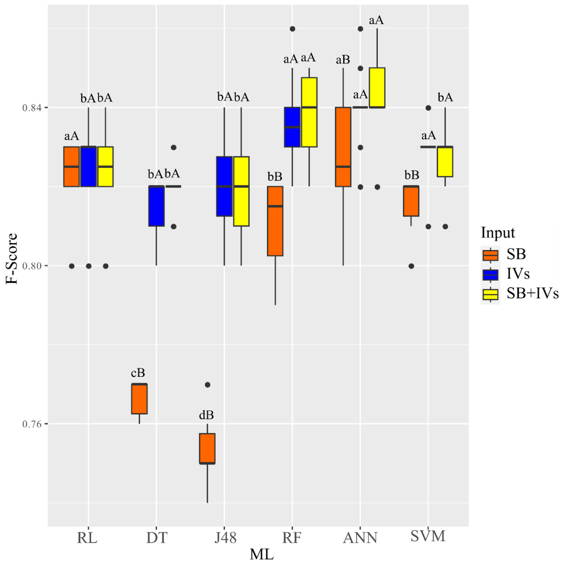
Figura 5. Boxplot para F-Score considerando a interação significativa entre os algoritmos de ML e as entradas testadas.
