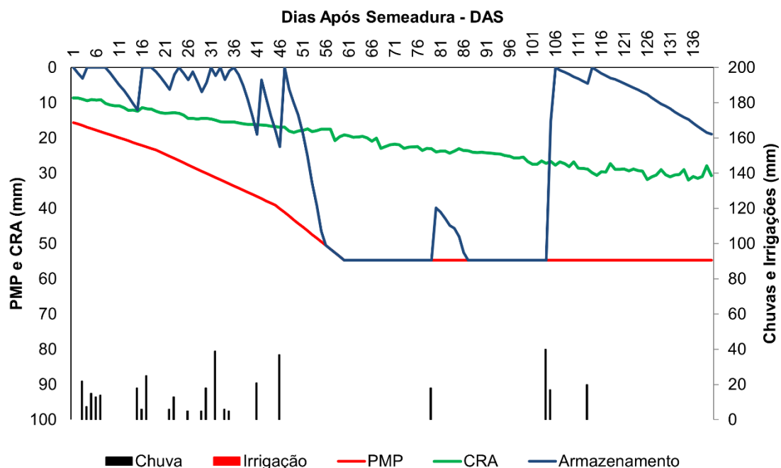
Figura 1. Balanço hídrico sequeiro no decorrer da segunda safra 2021/2022.
