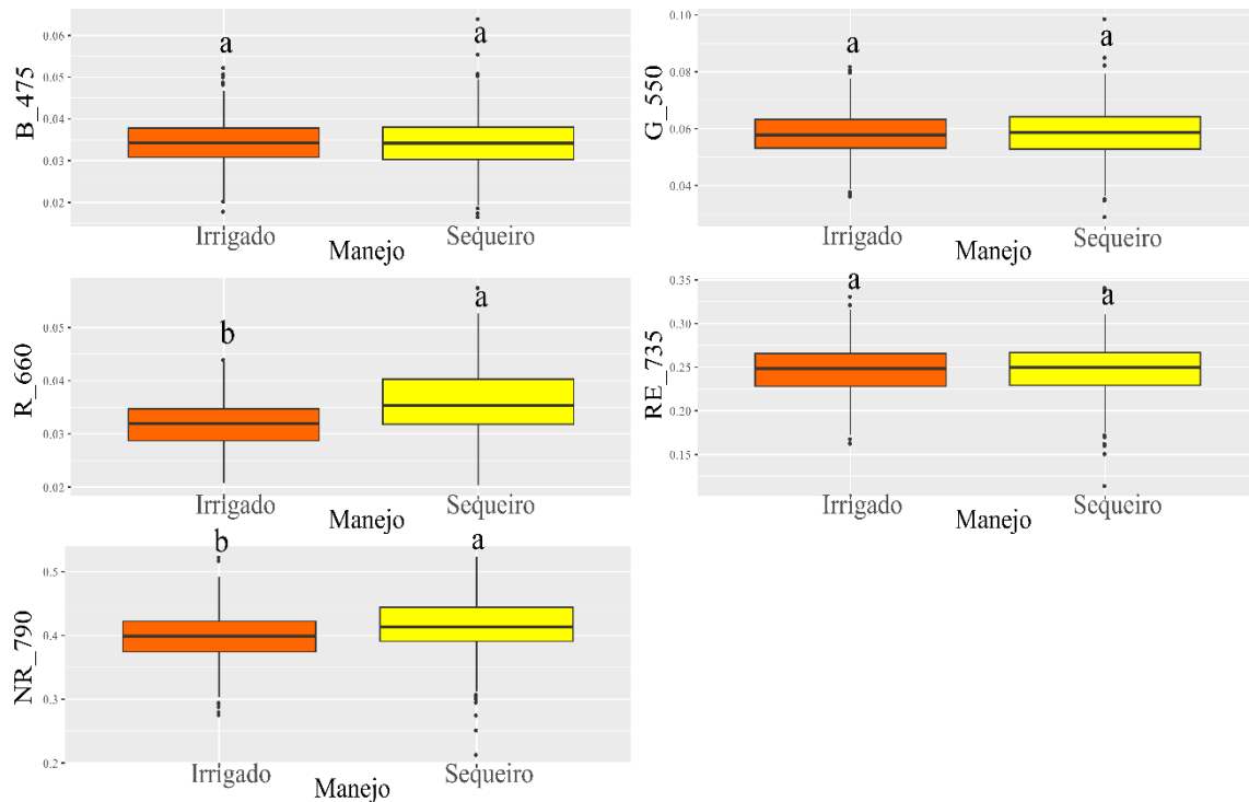
Figura 3. Boxplot para as médias de reflectância nos comprimentos de onda azul (B, 475 nm), verde (G, 550 nm), vermelho (R, 660 nm), borda do vermelho (RE, 735 nm) e NIR (790 nm) em milho sob manejo de irrigação e sequeiro.
