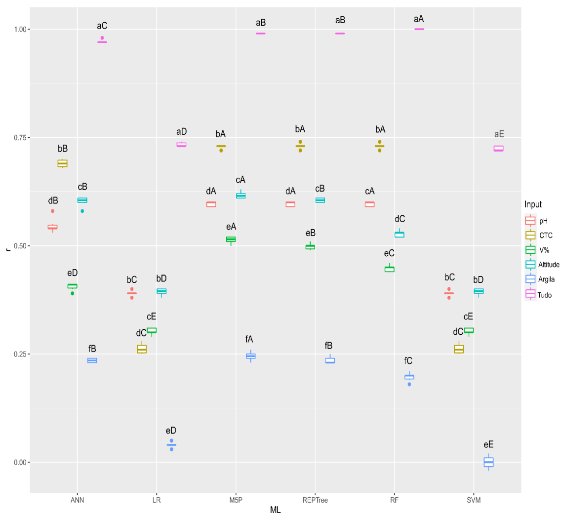
Figura 3. Boxplot para coeficiente de correlação ( r ) para o agrupamento de médias entre os inputs (pH, CTC, V%, altitude, argila e todas as informações) dos algoritmos (ANN, LR, M5P, REPTree, RF e SVM) na predição de produtividade de grãos de soja. Letras maiúsculas comparam as médias dos algoritmos de aprendizagem de máquina, enquanto letras minúsculas comparam os inputs pelo teste de Scott-Knott a 5% de probabilidade.
