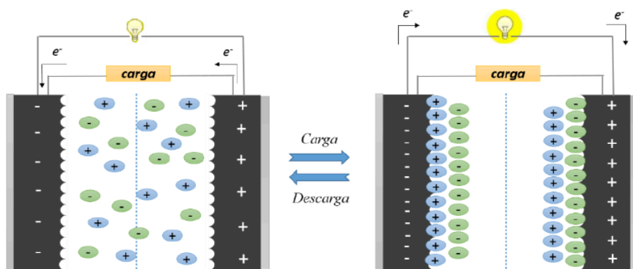
Figura 2 – Esquema de supercapacitor de dupla camada elétrica. Lado esquerdo mostra o supercapacitor descarregado e lado direito carregado.
