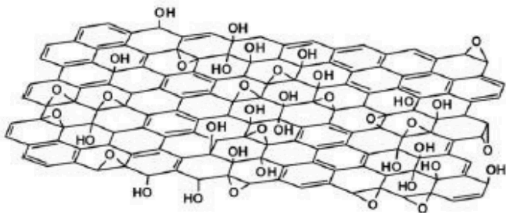
Figura 7 – Lamela do GO e grupos funcionais.
