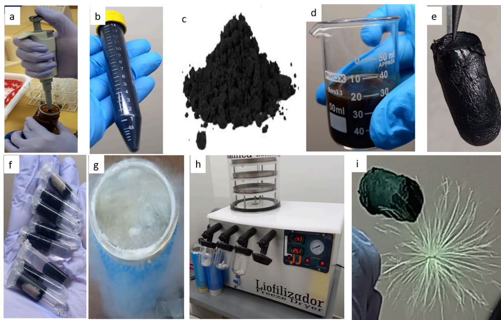
Figura 13 - Etapas da adição do carbon Black à síntese: a) GO, na concentração 2 mg/L, b) carbon black, c) CB (pó), d) solução homogeneizada, e) esponja, f) esponjas no eppendorf, g) amostras no nitrogênio, h) amostras no liofilizador, i) aerografeno dopado de carbon black.
