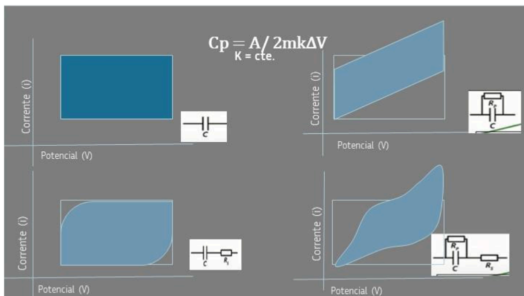
Figura 22 - Curvas típicas de voltametria cíclica e seus respectivos circuitos equivalentes. a) Capacitor, b) Capacitor e resistor em paralelo, c) Capacitor e resistor em série e d) Capacitor em paralelo com um resistor e este conjunto em série com um resistor.
