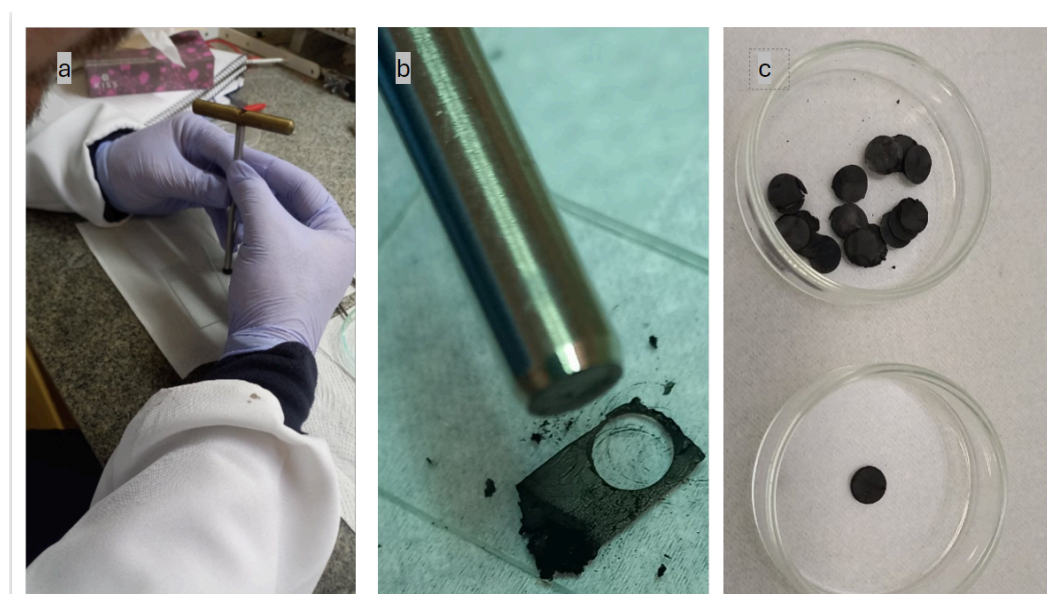
Figura 16 Corte e molde de amostras: a) Haste posicionada para corte, b) Amostra moldada c) Amostras padronizadas.
