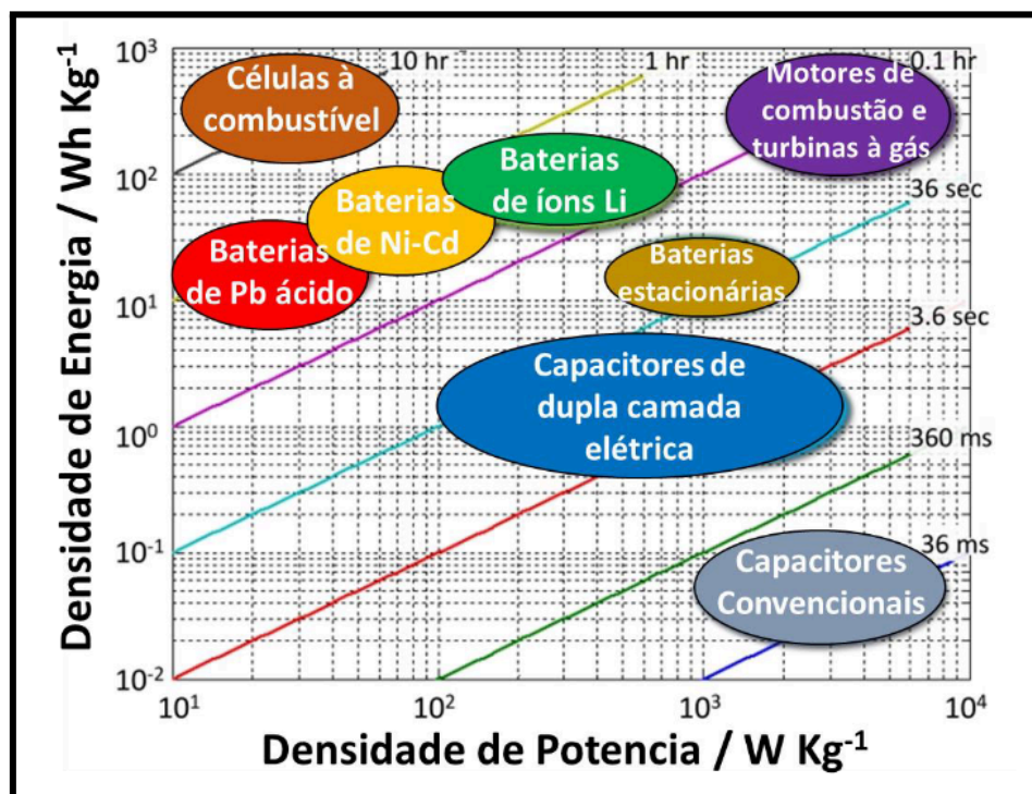
Figura 1 – Diagrama de Ragone apresenta comparação de dispositivos, levando em consideração a densidade de energia de diversos dispositivos de armazenamento. Nele, são representados os capacitores convencionais, os de dupla camada, baterias, células combustíveis, motores de combustão e turbinas à gás. Fonte: Da Silva et al., 2020.
