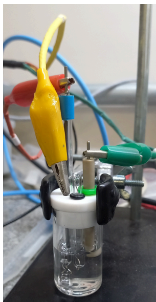
Figura 21- Célula eletroquímica de 3 eletrodos
