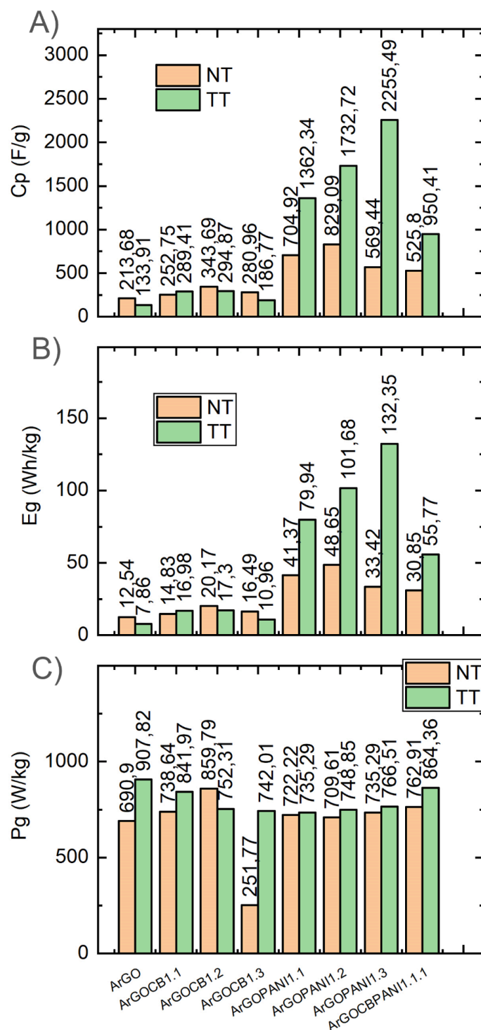
Figura 27 - Comparação de todas as amostras antes e após o tratamento térmico; A) Capacitância específica; B) Densidade de Energia e; C) Densidade de Potência.
