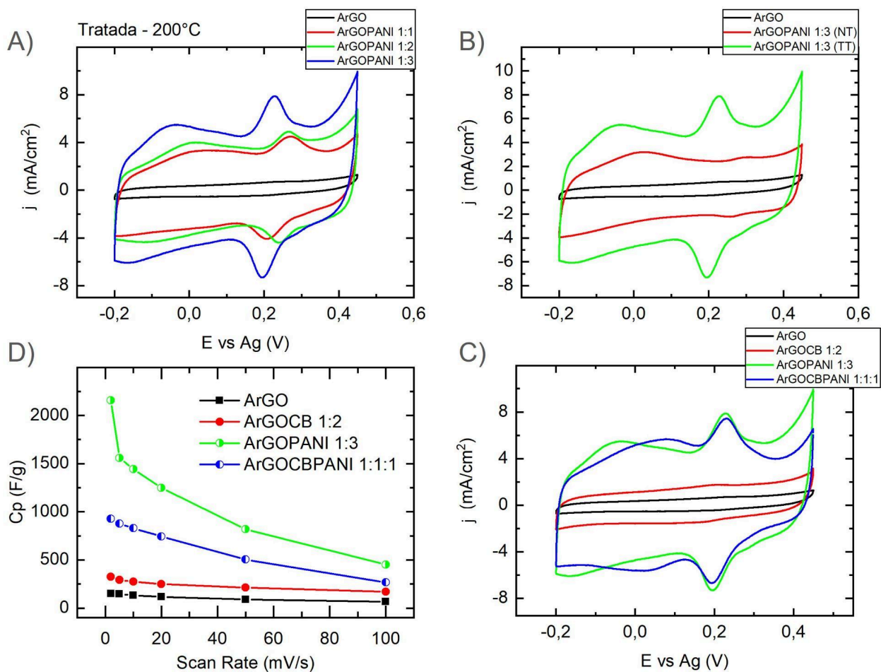
Figura 25 - Voltametria cíclica das amostras . A) e B) voltamogramas comparando as amostras ArGOPANI com diferentes proporções e diferenças após tratamento térmico, respectivamente. C) Compara as maiores áreas de cada amostra e D) Compara as capacitâncias específicas em função das velocidades de varredura.
