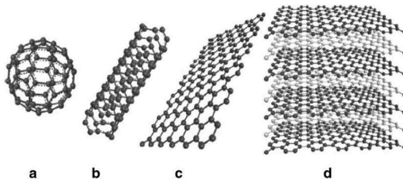
Figura 6– Formas alotrópicas do carbono: a) fulereno, b) nanotubo de carbono, c) grafeno, d) grafite
