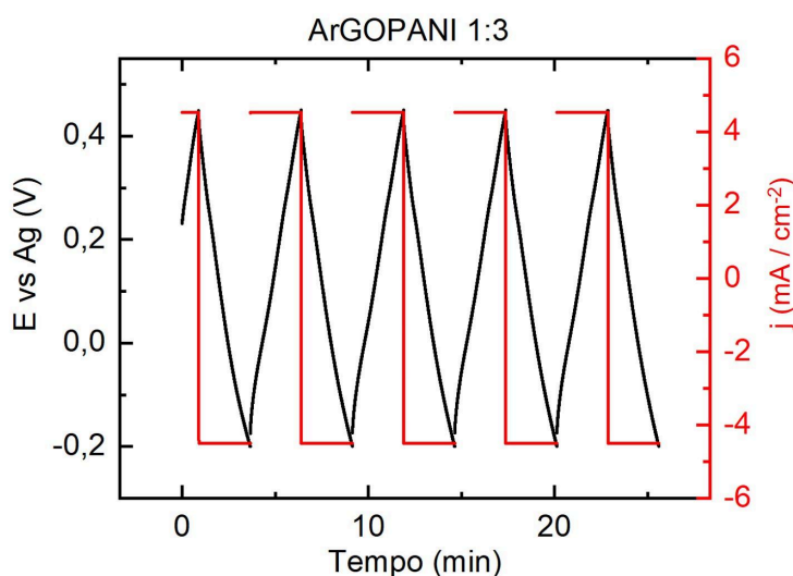
Figura 26- Gráfico de carga e descarga associada à densidade de corrente aplicada.
