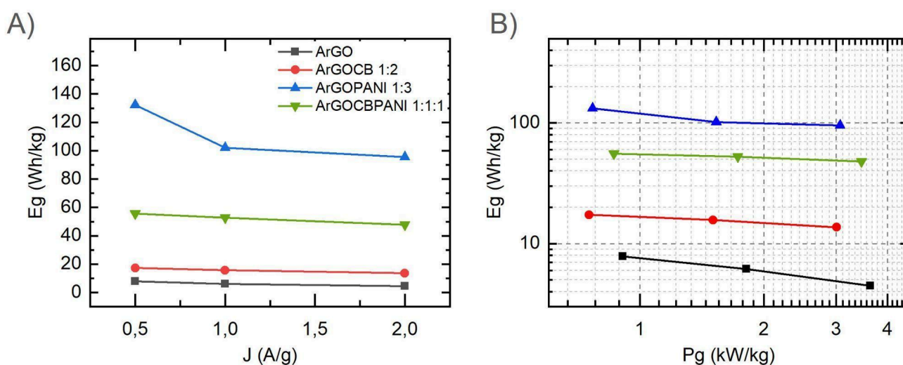
Figura 28- Gráfico da densidade de energia; A) em função da densidade de corrente e B) Em função da densidade de potência.
