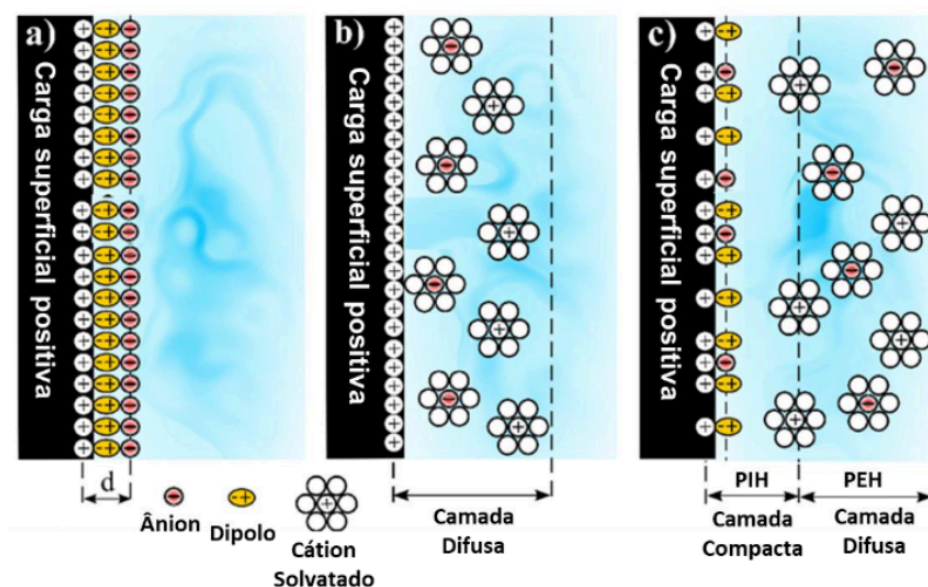
Figura 3 – Modelos de concepções de dupla camada elétrica. A) modelo de placas proposto por Helmholtz, b) Modelo de camada volumétrica difusa proposto por Gouy, e c) modelo de junção de camadas rígidas e camadas difusas proposto por Stern.
