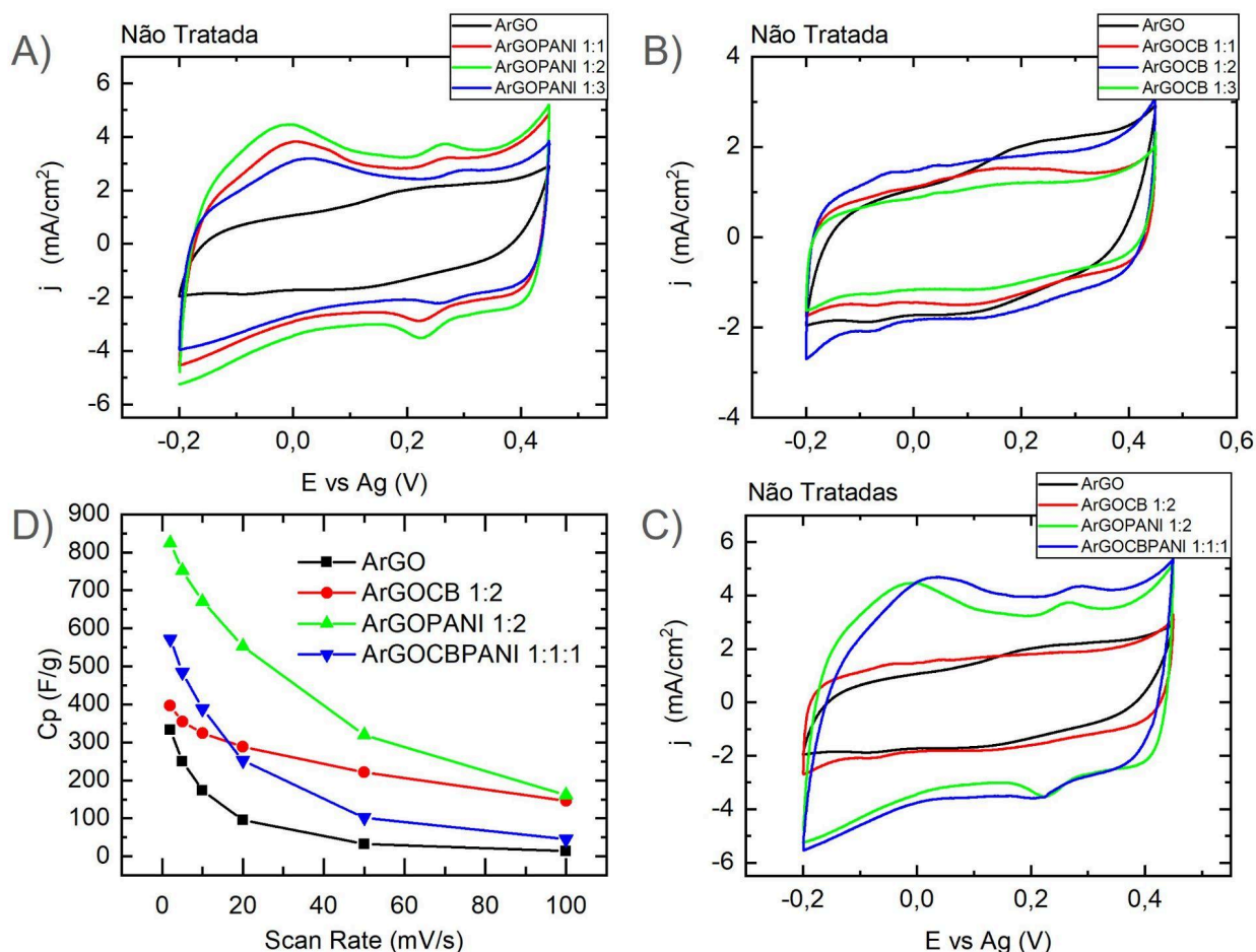
Figura 24 - Voltametria cíclica e capacitância específica das amostras “não tratadas termicamente”. A) e B) voltamogramas comparando as amostras ArGOPANI e ArGOCPB com diferentes proporções, respectivamente. C) Compara as maiores áreas de cada amostra e D) Compara as capacitâncias específicas em função das velocidades de varredura.
