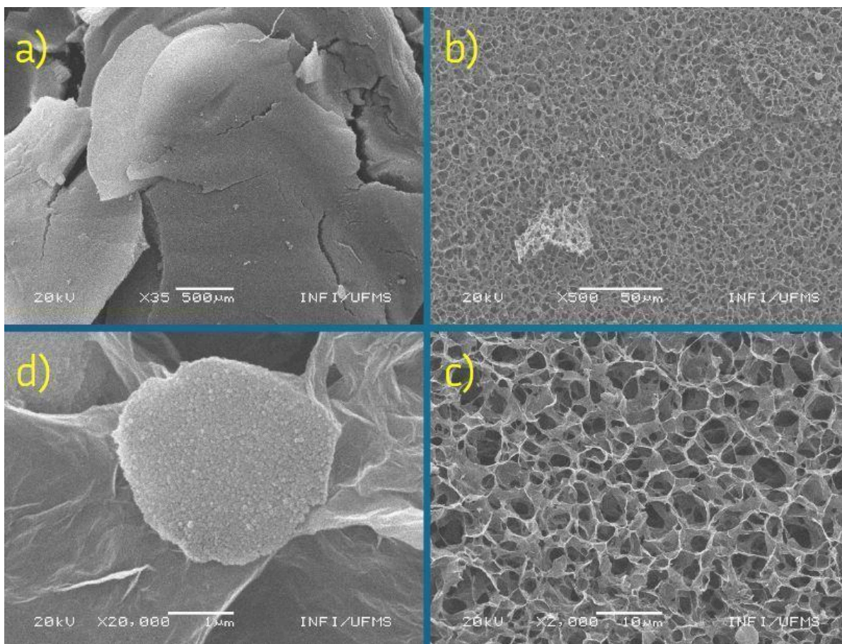
Figura 23- Imagens MEV do ArGOCB com magnificações de 35, 500 e 2000 vezes em a), b) e c), respectivamente. d) mostra um aglomerado de carbon black sobre o ArGO.
