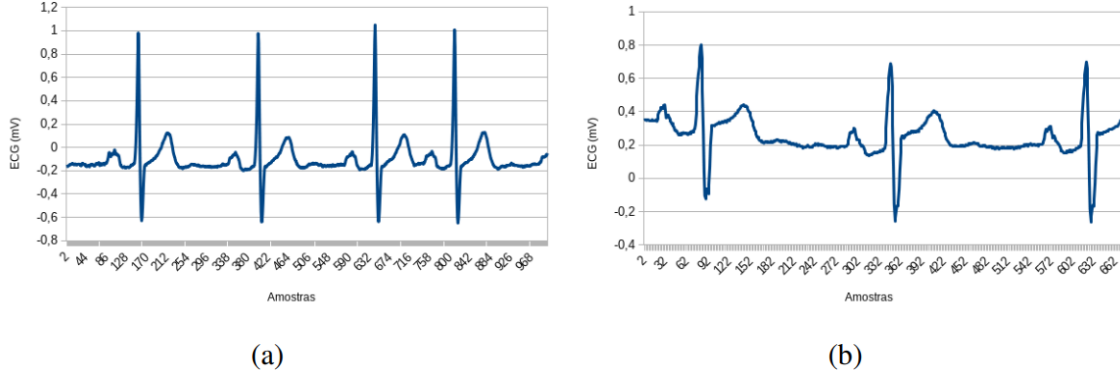
Figura 16: ECG (derivação DII) registrado em um indivíduo normal (a), e ECG registrado com os eletrodos afastados 12 cm (b)
