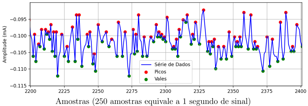
Figura 15: Segmento do registro reg11, utilizado para verificar o ruído intrínseco do dispositivo.
