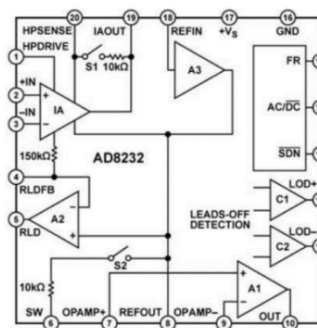
Figura 6: Arquitetura interna do circuito integrado do AD8232.
