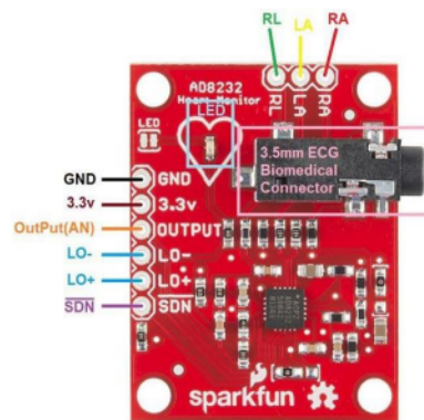
Figura 5: Imagem do módulo AD8232. Suas dimensões são 3 x 3 x 3 mm Fonte: https://www.sparkfun.com/
