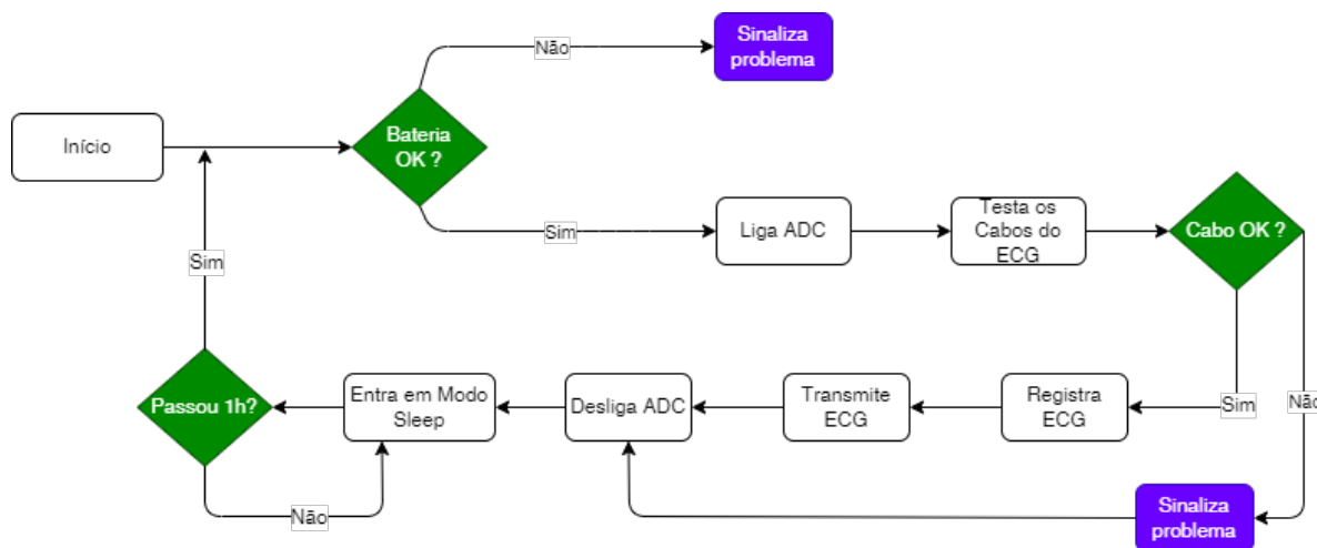
Figura 9: Fluxograma da Firmware desenvolvida para o dispositivo. Fonte: Elaboração própria.
