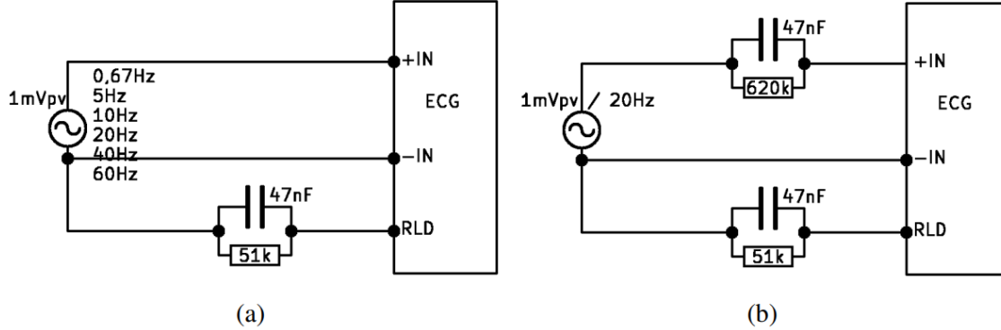
Figura 13: Circuito utilizado para verificar a resposta em frequência, ajustando a frequência da fonte CA para diferentes valores (a); e circuito utilizado para obter o registro reg8, usado na verificação da impedância de entrada (b).
