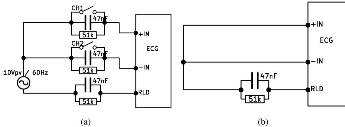
Figura 14: Circuito para obter os registros utilizados na verificação da rejeição em modo comum (CMRR), considerando situações de desequilíbrio na impedância de entrada: reg12 (CH1-ON e CH2-ON), reg13 (CH1-OFF e CH2-ON), e reg14 (CH1-ON e CH2-OFF) (a); e circuito utilizado para obter o registro reg11 e verificar o ruído intrínseco do dispositivo (b).
