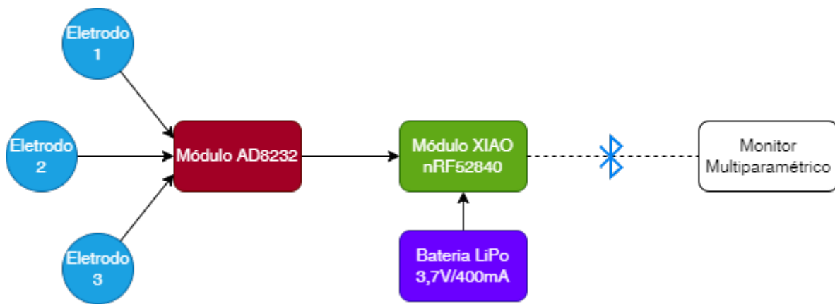
Figura 4: Arquitetura do hardware do dispositivo construído. Fonte: Elaboração própria.
