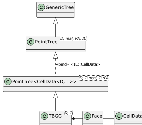
Figura 3.4: Diagrama de classes UML da hierarquia das classes que modela a Tree Based Graded Grid , que adiciona faces à árvore e as associa às células da estrutura.
