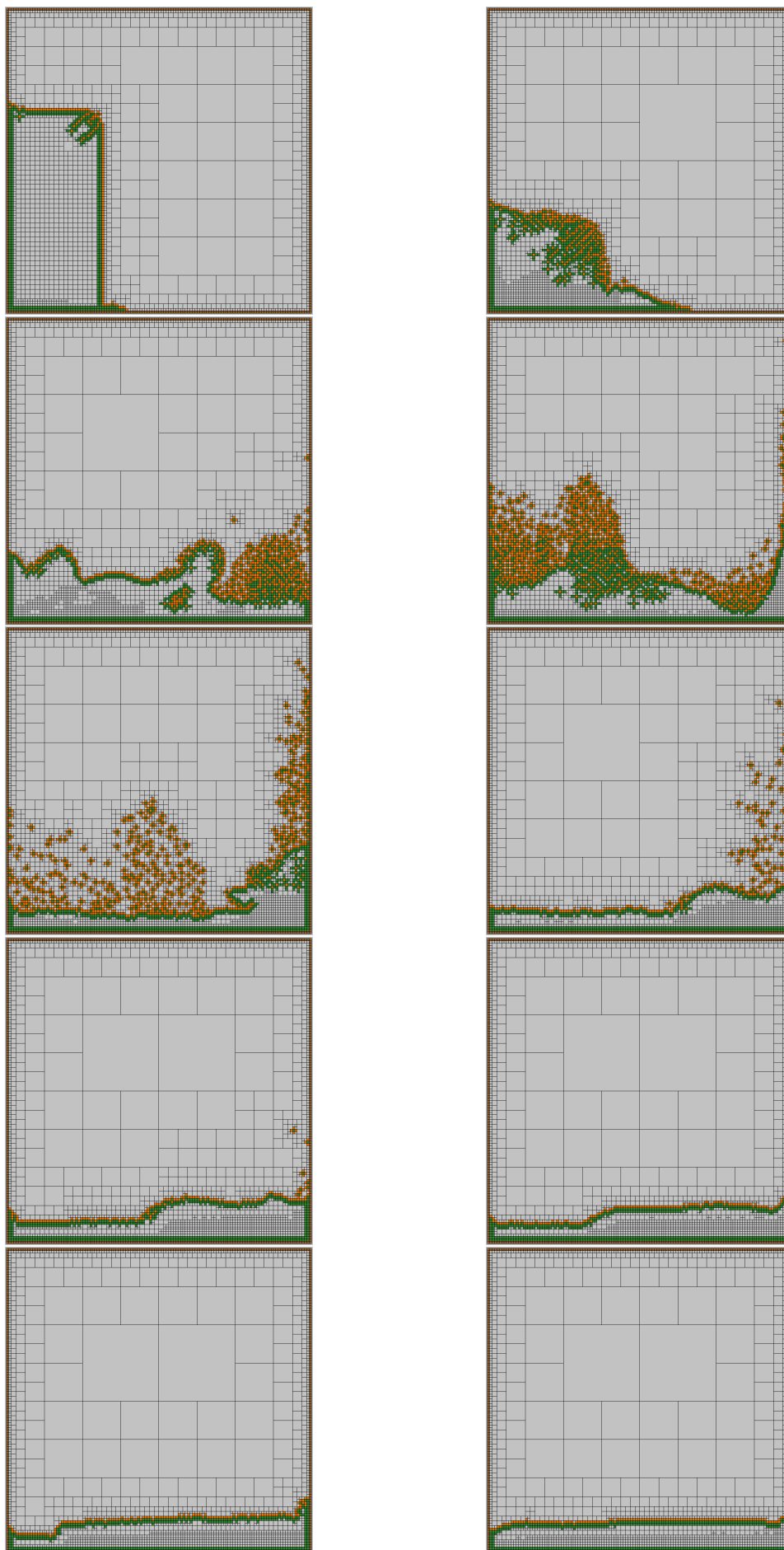
Figura 4.2: Simulação dam break para corpos granulares, ilustrada por 10 passos, escolhidos a cada 100 passos, iniciando no passo 100.
