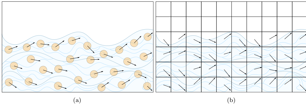
Figura 1.1: Exemplos de uma simulação Lagrangeana e Euleriana. (b) Uma simulação baseada em partículas. (a) Uma simulação baseada em grade. (Adaptado de Liu et al. [32].)
