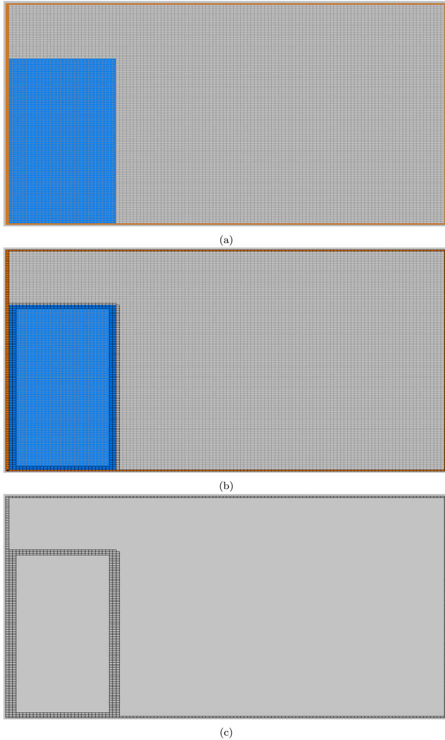
Figura 4.9: Processo de refinamento da TBGG. (a) Grade totalmente refinada pra classificar as células em fluido (células azuis) ou sólido (células laranjas). (b) Árvore construída e refinada com base na grade. (c) Árvore obtida após o refinamento.
