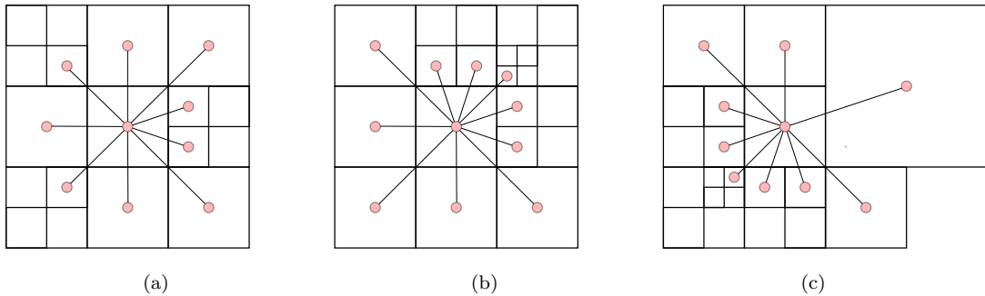
Figura 3.1: Exemplos de estênceis para o cálculo do Laplaciano em uma quadtree balanceada.
