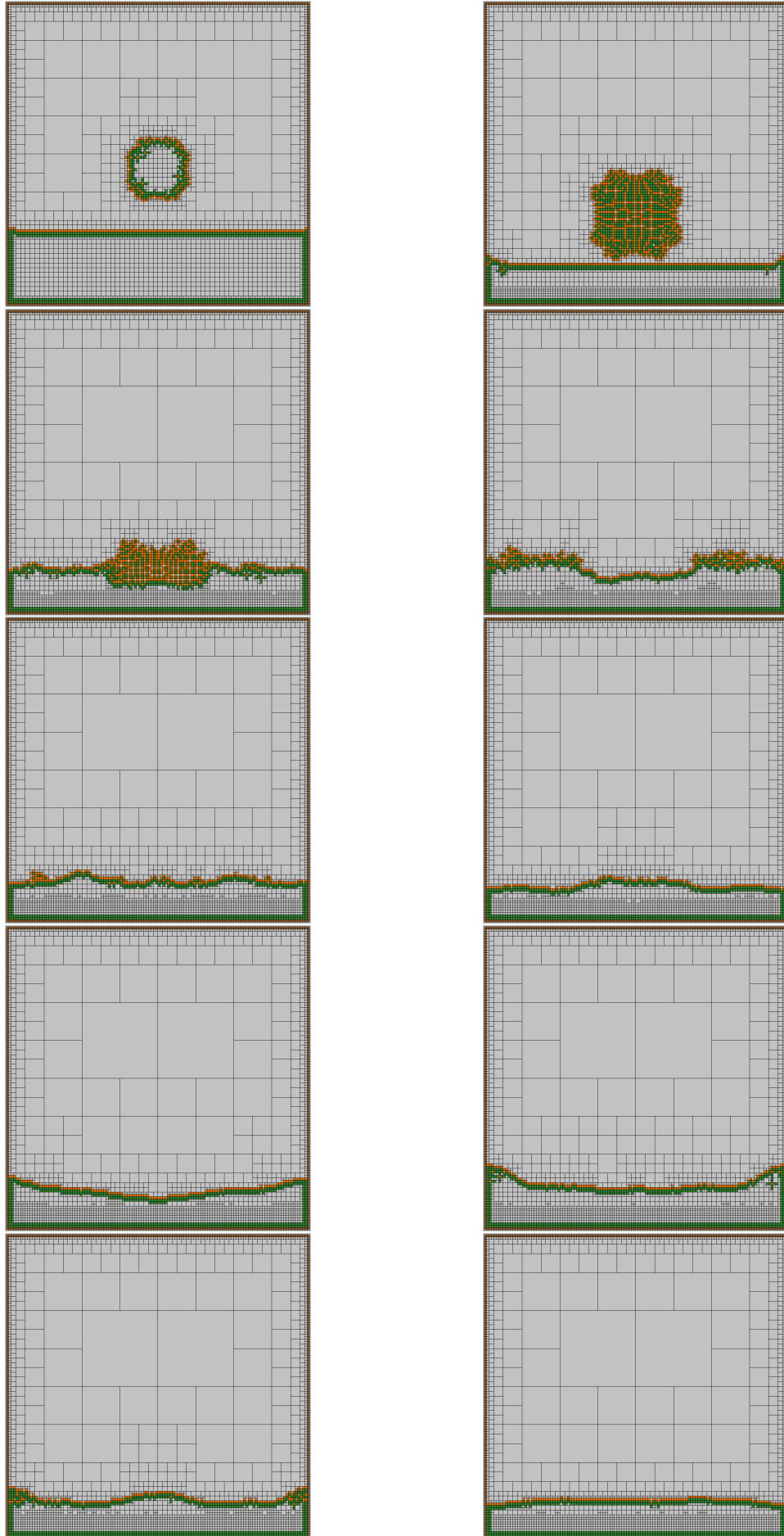
Figura 4.4: Simulação water drop para corpos granulares, ilustrada por 10 passos, escolhidos a cada 100 passos, iniciando no passo 100.
