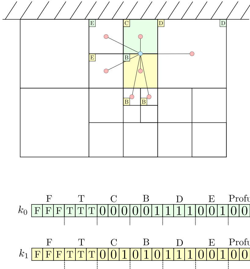
Figura 3.7: Exemplo de chave para um estêncil do operador gradiente em uma grade bidimensional.
