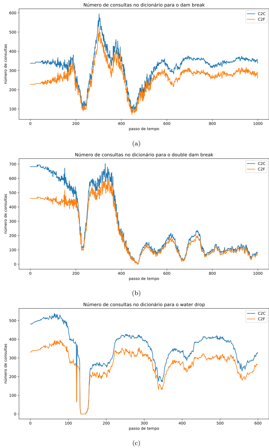
Figura 4.6: Número de consultas aos dicionários dos pesos do Laplaciano (C2C) e gradiente (C2F) em que há os pesos RBF-FD registrados para a chave consultada.
