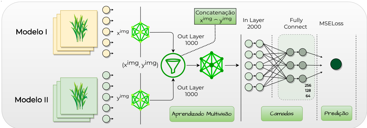
Figura 5.6: Modelo Deep4Fusion Multivisão utilizado neste trabalho.
