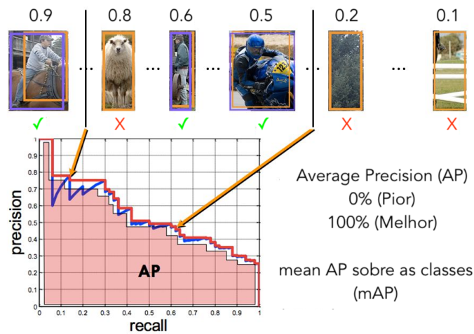
Figura 2.19: Métrica mAP. Adaptado de Lanqing (2019).
