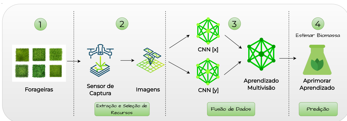
Figura 5.2: Visão geral do Aprendizado Multivisão aplicado à estimativa de massa de forragem.
