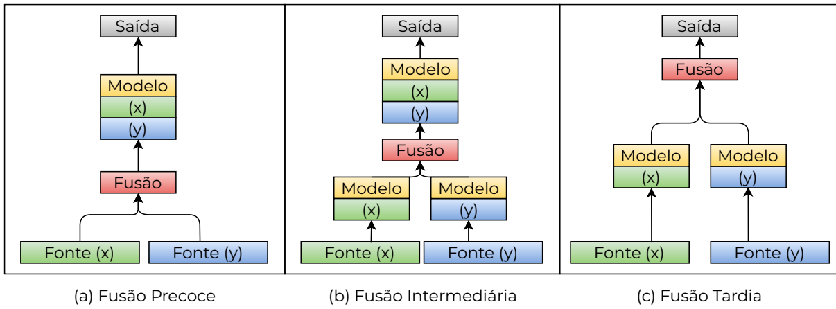
Figura 2.3: Tipos de Fusão Multimodal.
