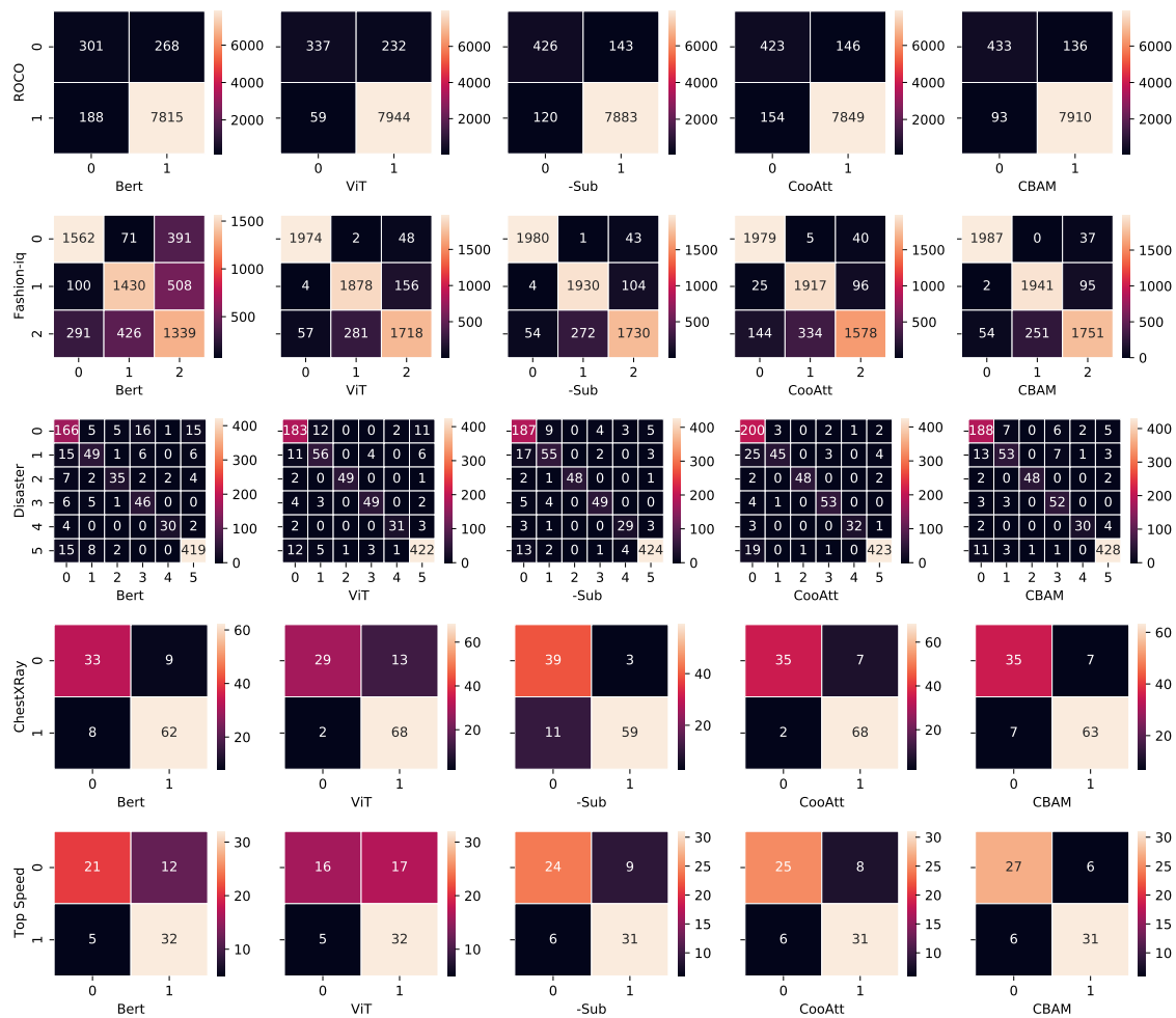
Figura 3.16: Matriz de Confusão - Resultados da classificação com os cinco conjuntos de dados avaliados neste experimento.
