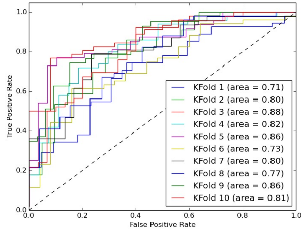
Figura 2.18: Gráfico ROC dataset diabetes (Asuncion and Newman, 2007).
