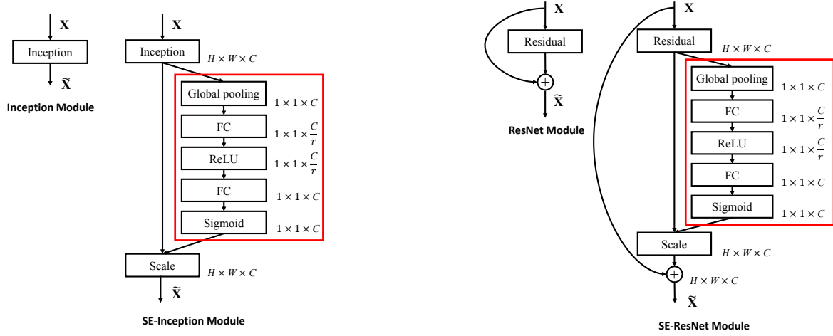
Figura 3.8: Operações em um bloco SE-Net . Fonte: (Hu et al., 2018).
