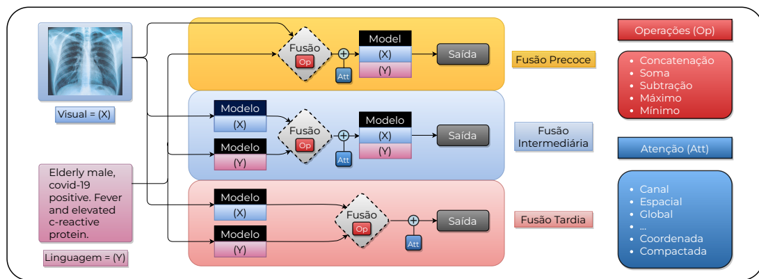
Figura 3.10: Modelos de Fusão para o Aprendizado Multimodal com Operações Aritméticas e Mecanismos de Atenção.
