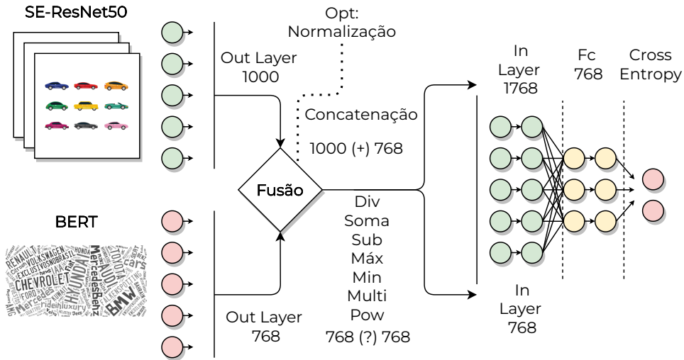
Figura 3.3: Modelo de Fusão - Representação gráfica do modelo multimodal com fusão tardia sobre dois modelos unimodais ( BERT e SE-ResNet50 ). Na etapa de fusão uma das oito operações aritméticas é seleccionada e em seguida uma camada totalmente conectada é aplicada na saída do modelo.
