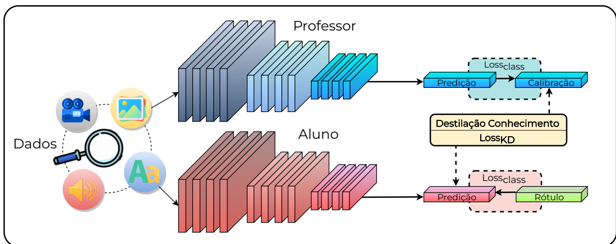
Figura 2.12: Arquitetura Multimodal Knowledge Distillation (MKD).
