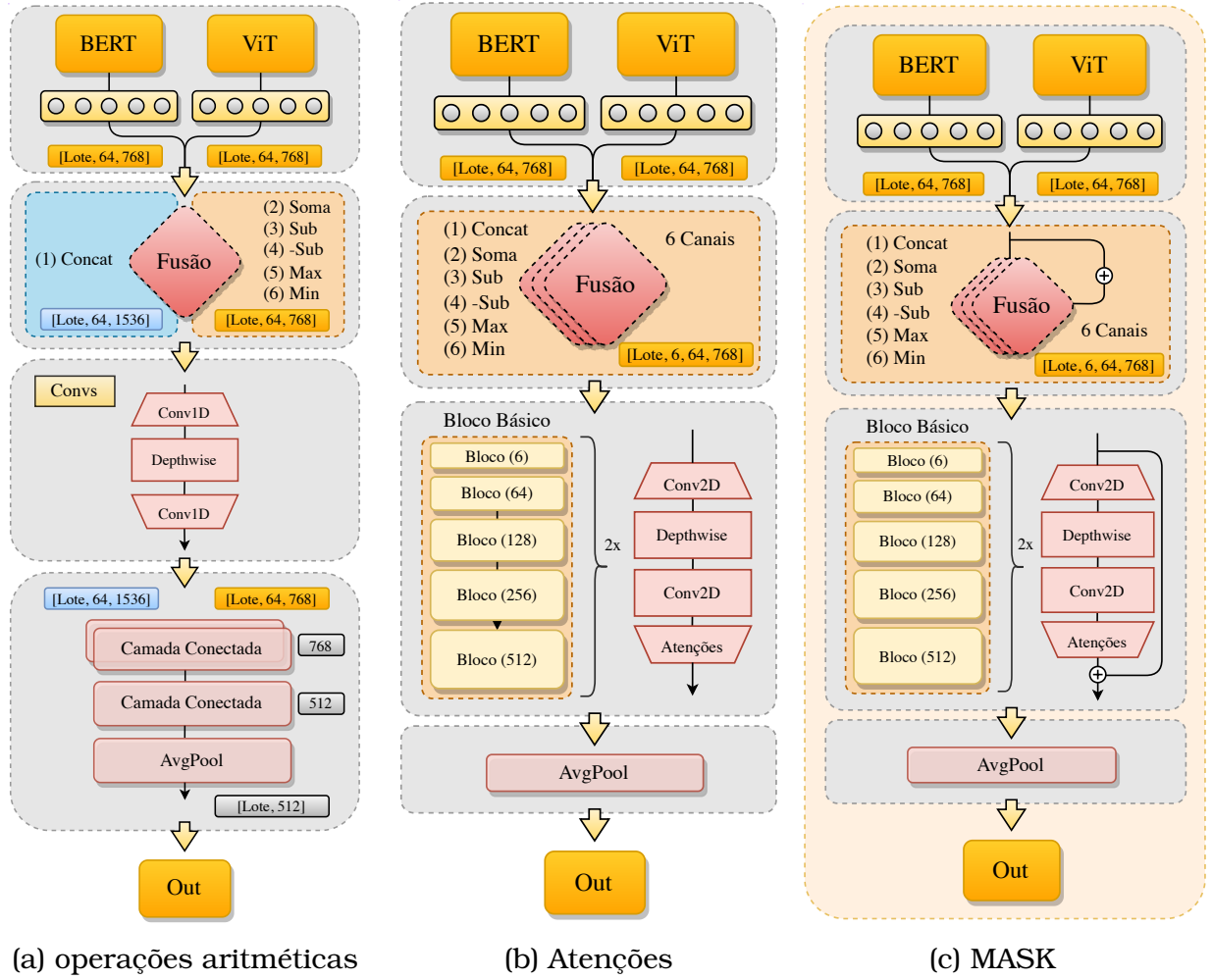
Figura 3.12: Modelos Multimodais: (a) Operações Aritméticas, (b) Mecanismos de Atenção, (c) Mecanismos de Atenção com Skip Connection .
