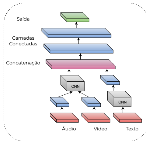
Figura 2.6: Fusão Lenta. Adaptado de Williams et al. (2018).
