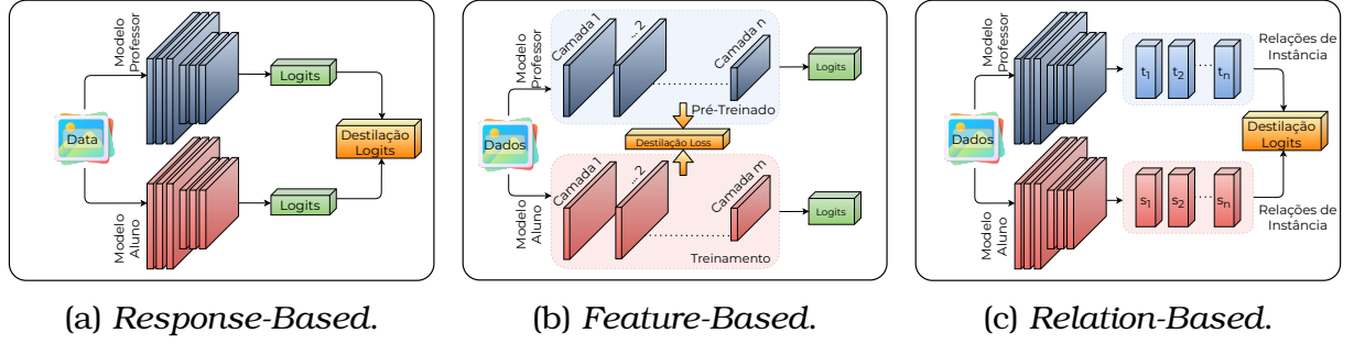
Figura 2.13: Métodos de Destilação de Conhecimento. Adaptado de Gou et al. (2021).
