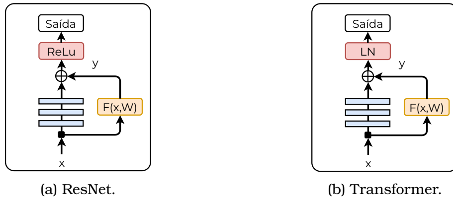
Figura 2.10: Representação do Skip Connection : (a) Unidade Residual Convencional (He et al., 2016), (b) Unidade Residual em Transformers (LN = Normalização de Camadas) (Vaswani et al., 2017). Adaptado de Liu et al. (2020) .
