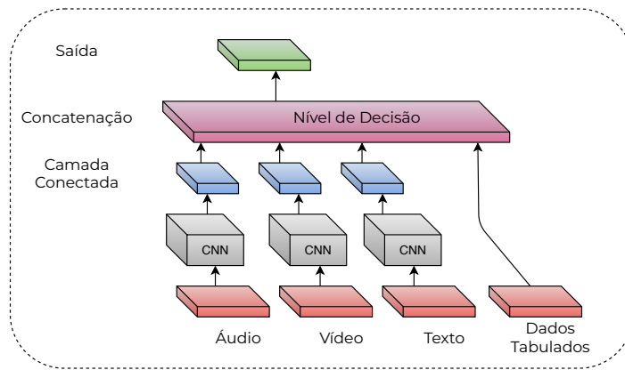
Figura 2.8: Fusão Tardia. Adaptado de Williams et al. (2018).
