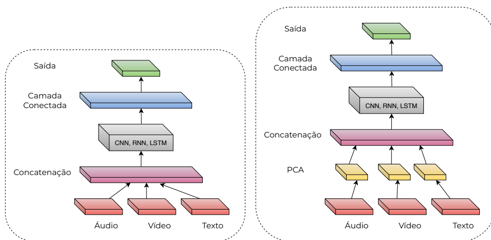
Figura 2.4: Fusão Precoce com e sem redução de dimensionalidade. Adaptado de Williams et al. (2018).
