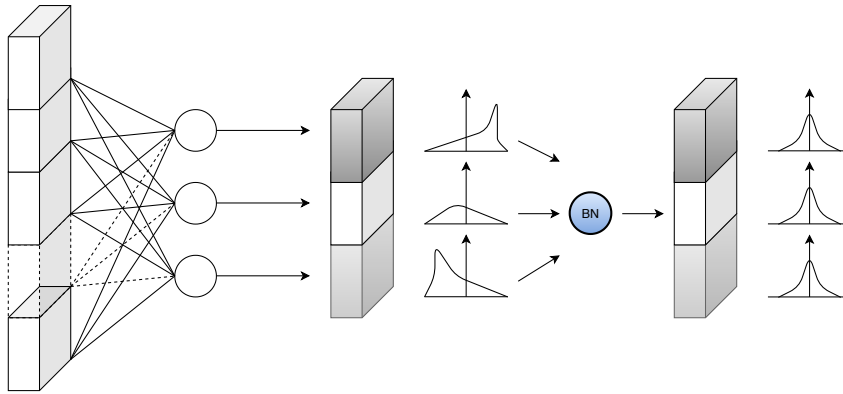
Figura 3.5: Sequência de passos para normalização das camadas em um rede neural.
