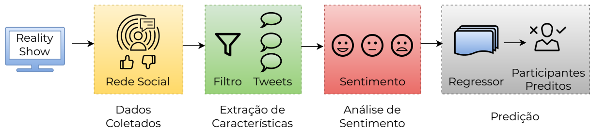
Figura A.3: Sequência de passos para predição de participantes eliminados.
