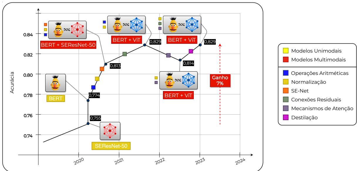
Figura 3.1: Evolução das técnicas do Aprendizado Multimodal realizados por este trabalho utilizando o conjunto de dados multimodal ( Top Speed ).
