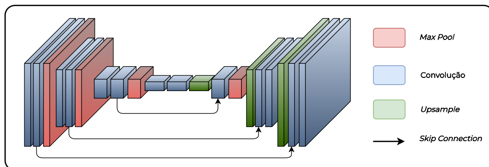
Figura 2.9: Arquitetura U-Net com uso de Skip Connection .
