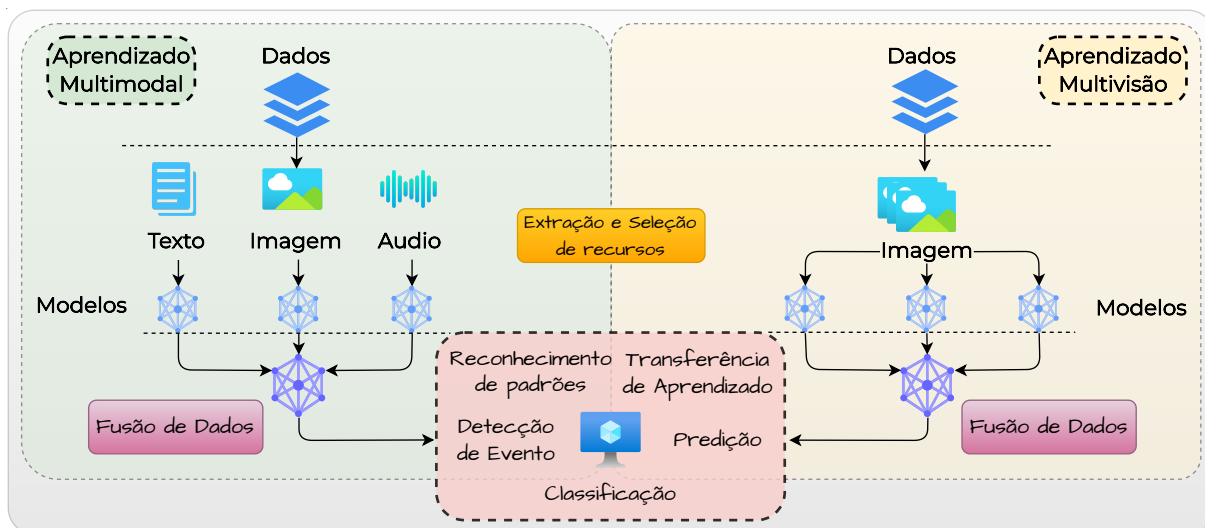
Figura 5.1: Aprendizado Multimodal versus Aprendizado Multivisão.
