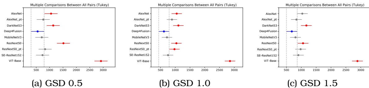
Figura 5.7: Média e intervalo de confiança de 95% para o teste pos-hoc Tukey HSD sobre a métrica MAE - TGMY.
