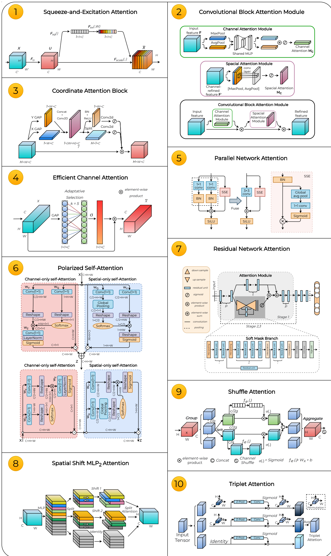
Figura 2.11: Estrutura dos Mecanismos de Atenção.
