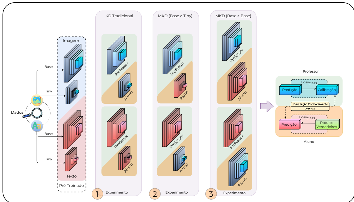
Figura 4.1: Arquitetura MKD - Pipeline.
