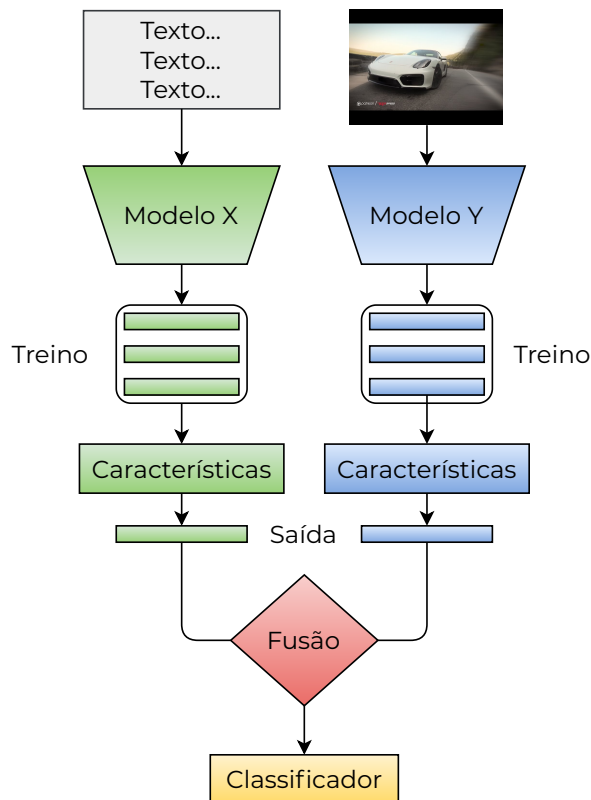
Figura 2.2: Visão geral do funcionamento de uma Rede Multimodal com Fusão Tardia.
