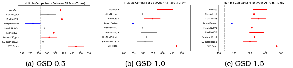
Figura 5.9: Média e intervalo de confiança de 95% para o teste pos-hoc Tukey HSD sobre a métrica MAE - TDMY.
