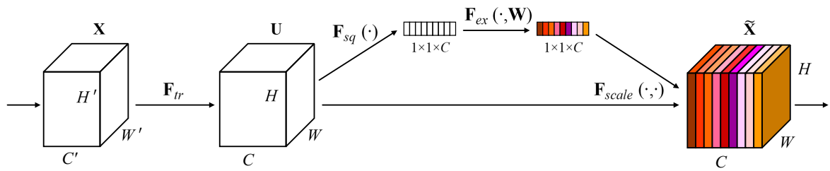
Figura 3.7: Bloco SE-Net . Fonte: (Hu et al., 2018)
