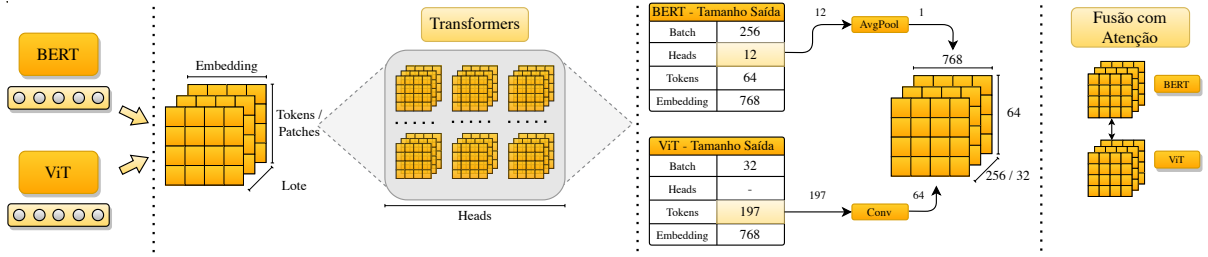
Figura 3.11: Configuração dos modelos BERT e ViT
