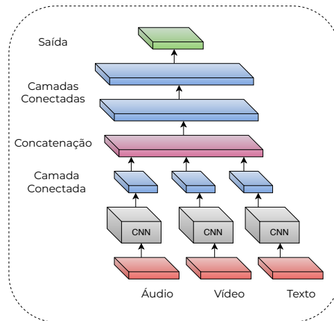
Figura 2.5: Fusão Intermediária. Adaptado de Williams et al. (2018).
