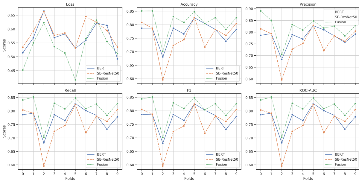
Figura 3.4: Loss , Accuracy , Precision , Recall , F1 e ROC-AUC para etapa de validação, com o número de 100 épocas para os modelos BERTimbau , SE-ResNet50 and Fusão = Subtração .
