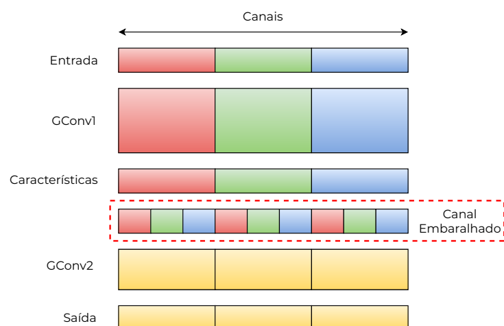
Figura 2.7: Arquitetura ShuffleNet . Adaptado de Zhang et al. (2018b).
