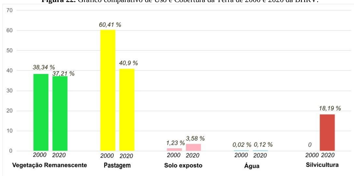
Figura 22. Gráfico comparativo de Uso e Cobertura da Terra de 2000 e 2020 da BHRV.
