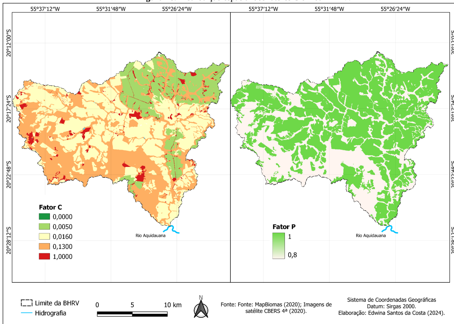
Figura 18. Distribuição espacial dos fatores C e P da BHRV.
