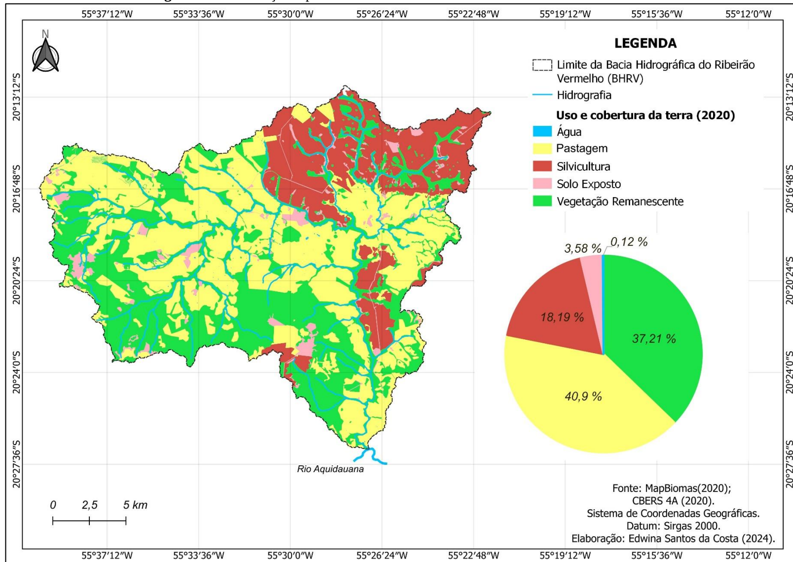
Figura 21. Distribuição espacial do uso e cobertura da terra do ano de 2020 na BHRV.
