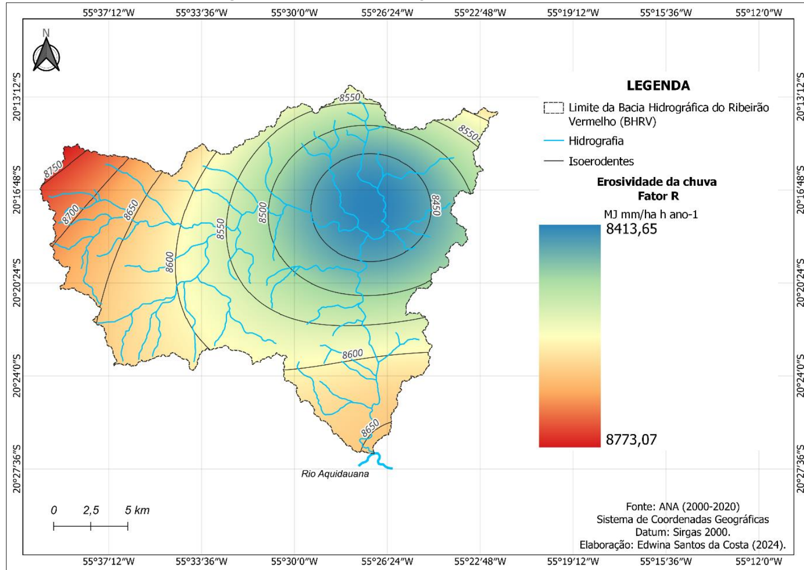
Figura 15. Fator R da bacia hidrográfica do Ribeirão Vermelho.
