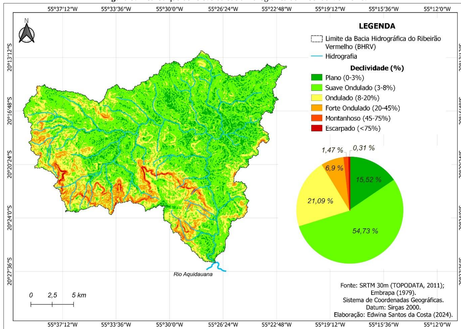
Figura 9. Distribuição do relevo da bacia hidrográfica do Ribeirão Vermelho.
