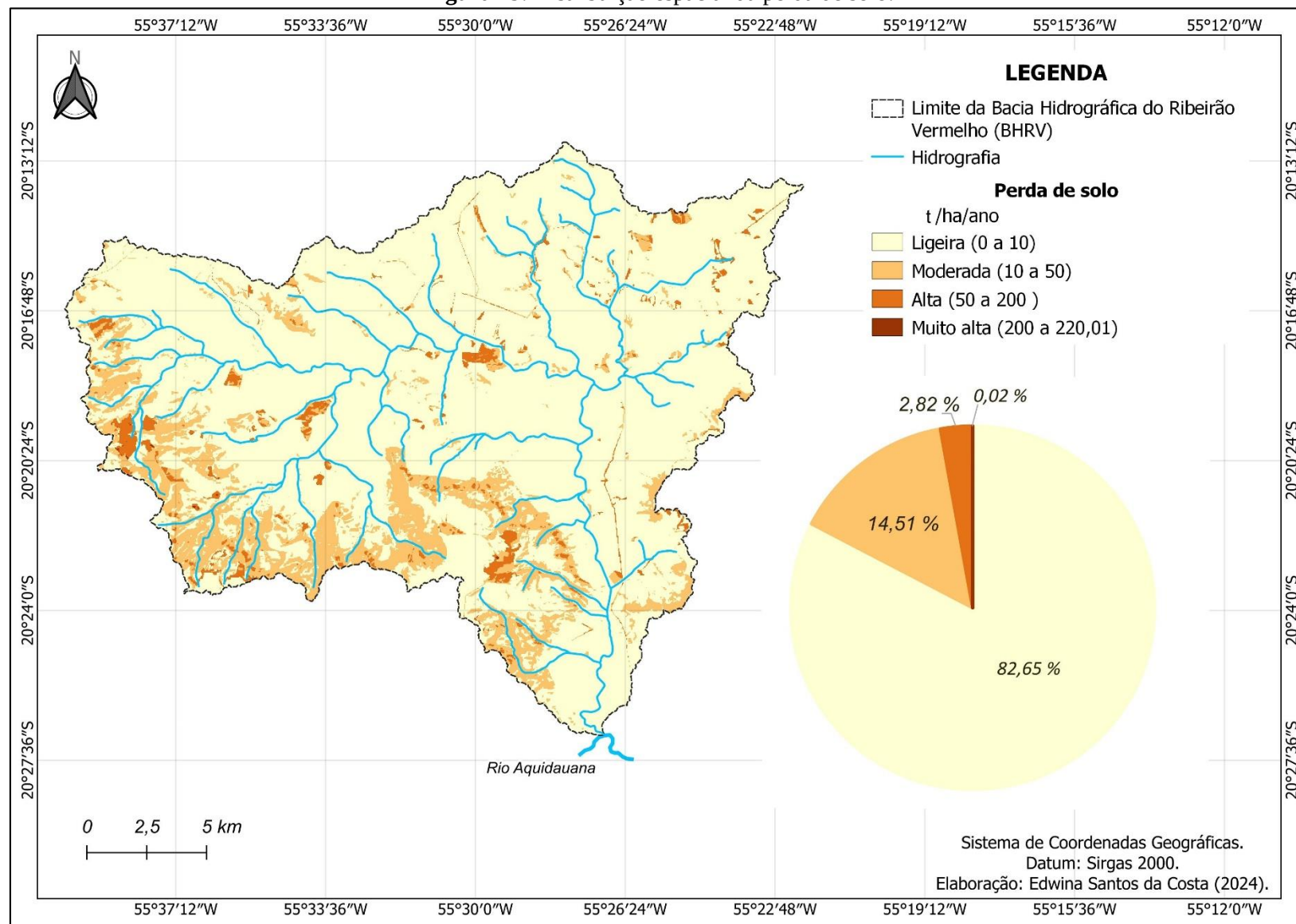
Figura 19. Distribuição espacial da perda de solo.
