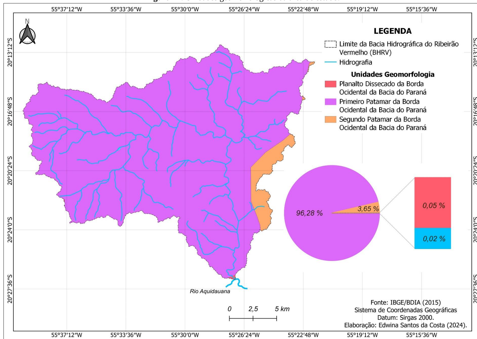
Figura 11. Unidades geomorfológicas da área de estudo.
