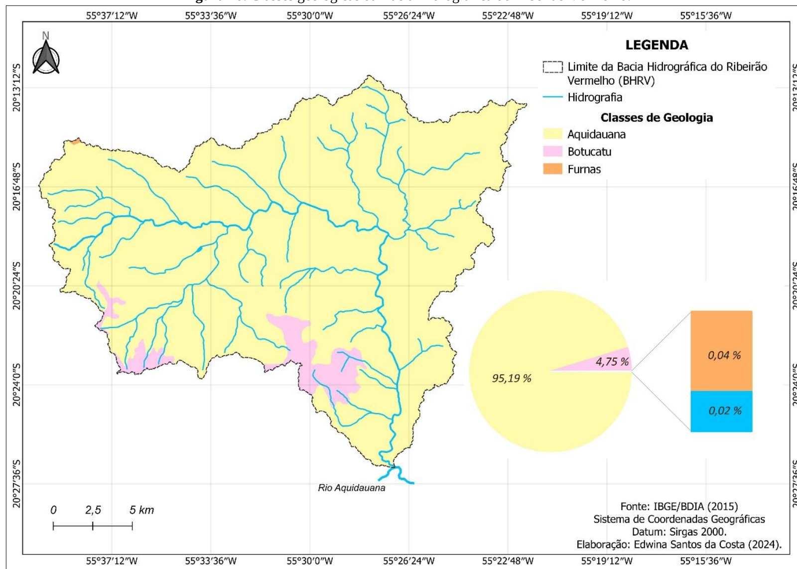
Figura 10. Classes geológicas da Bacia Hidrográfica do Ribeirão Vermelho.
