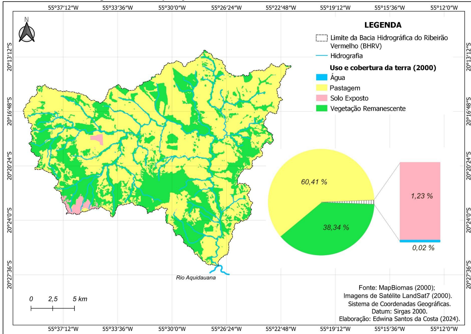
Figura 20. Distribuição espacial do uso e cobertura da terra do ano de 2000 na BHRV.
