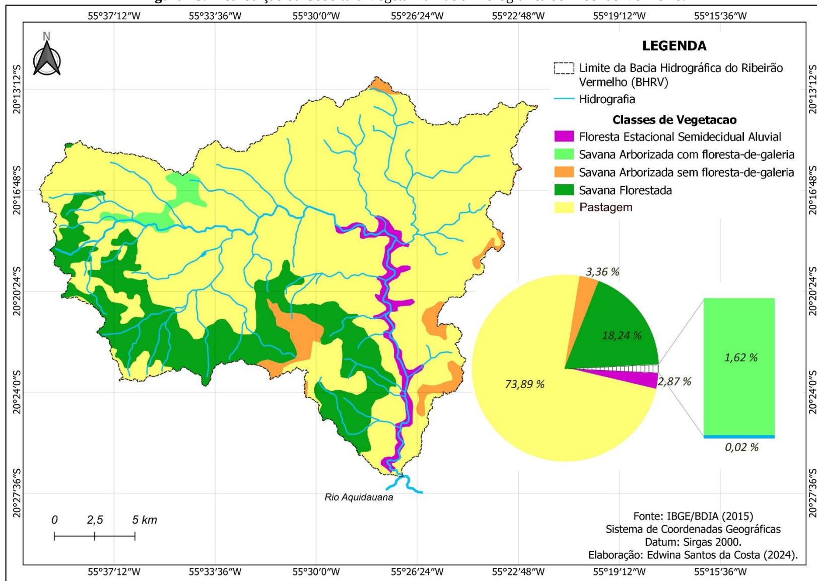
Figura 13. Distribuição da Cobertura Vegetal na Bacia Hidrográfica do Ribeirão Vermelho.
