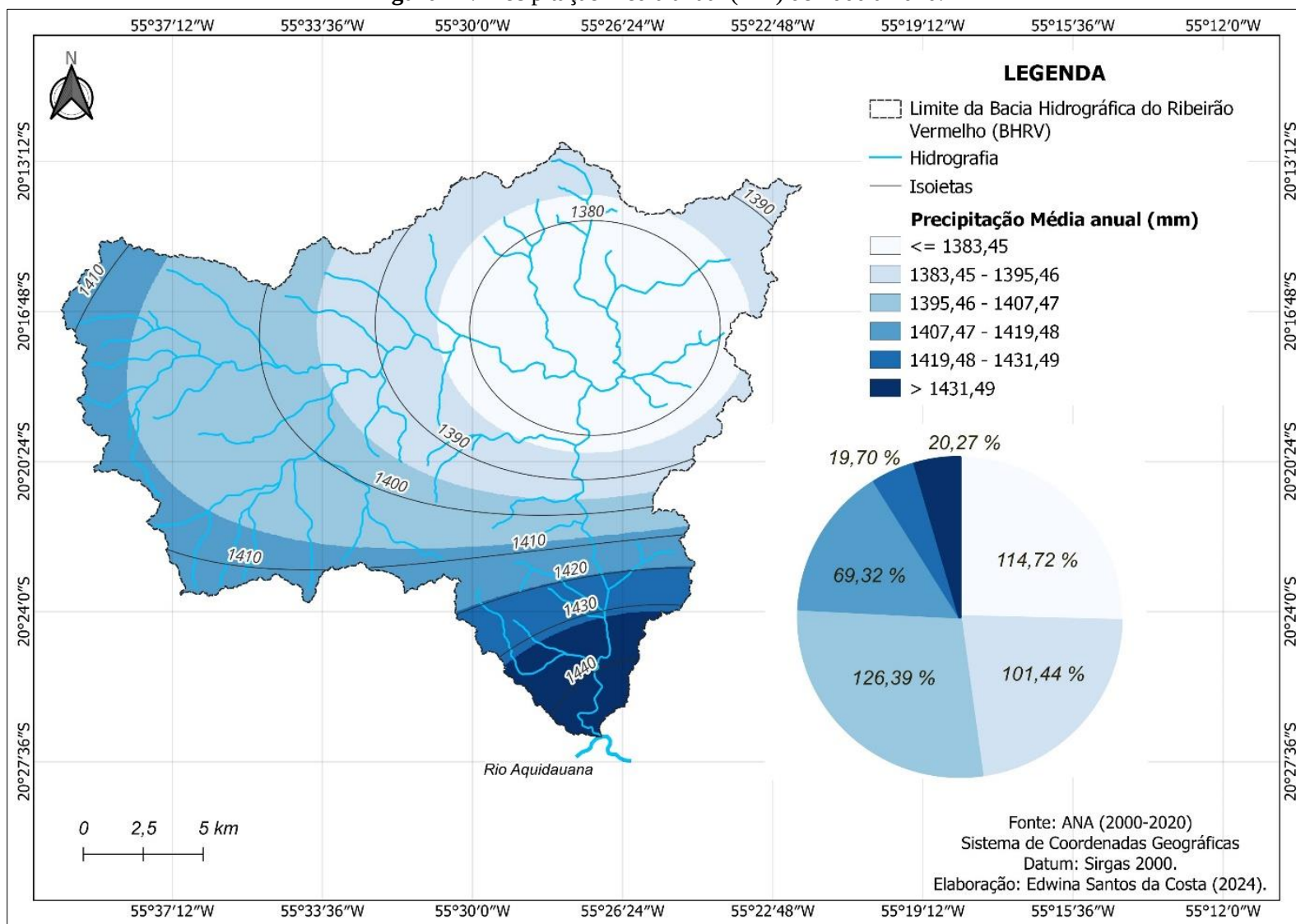
Figura 14. Precipitação média anual (mm) de 2000 a 2020.
