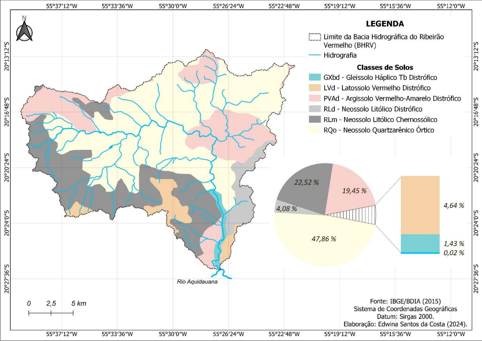
Figura 12. Distribuição dos solos na Bacia Hidrográfica do Ribeirão Vermelho.
