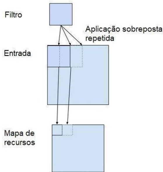
Figura 5 - Filtro Aplicado a uma Entrada Bidimensional para Criar um Mapa de Recursos
