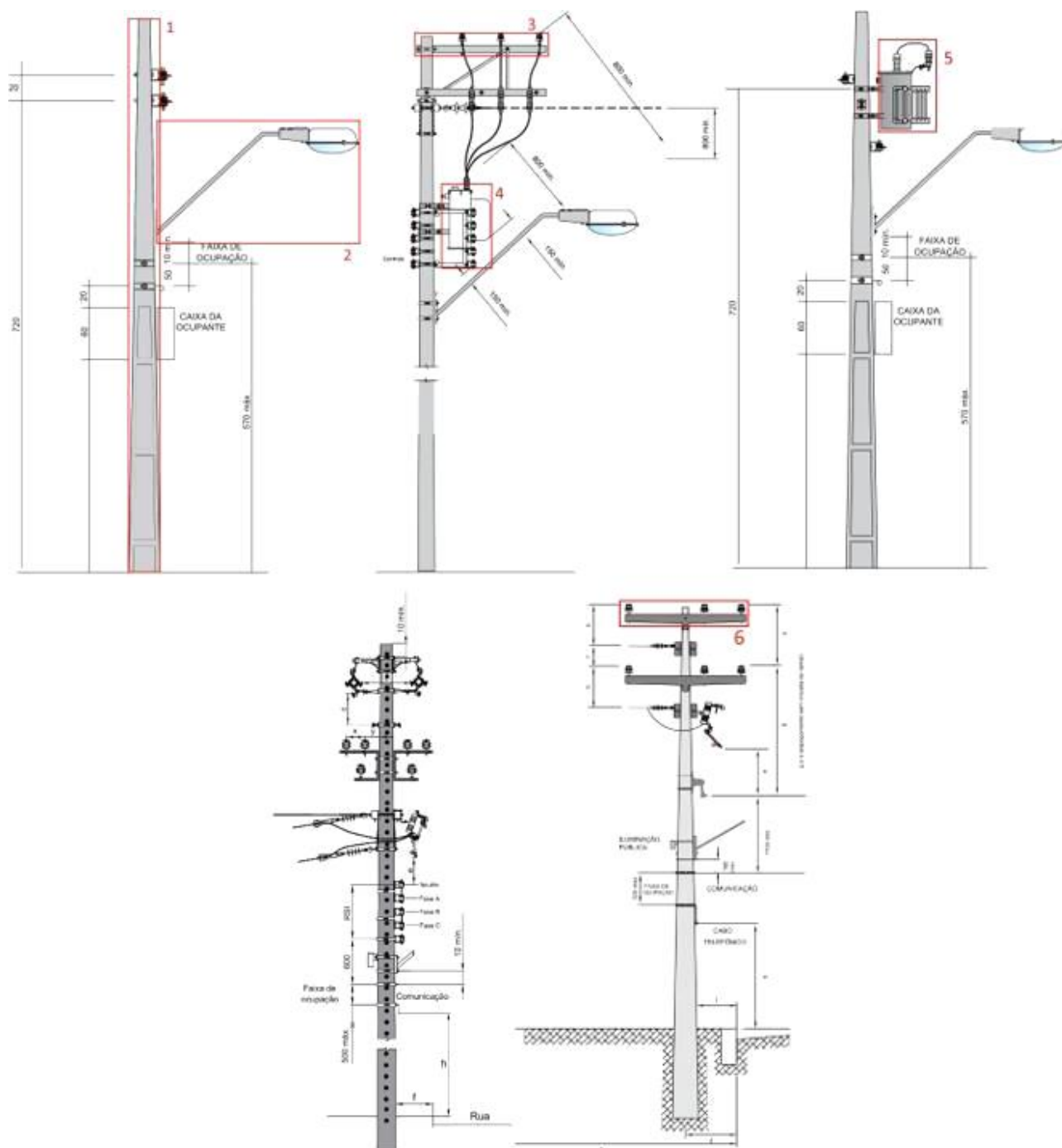
Figura 1 - Componentes dos tipos de postes em Campo Grande/MS.
