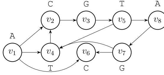
Figura 3.1: Exemplo de um grafo de sequência simples G .
