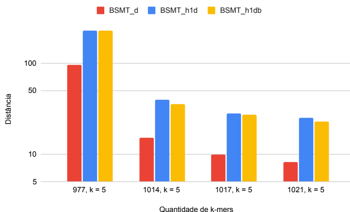
Figura 7.5: Média das distâncias: gráfico para a Tabela 7.5.
