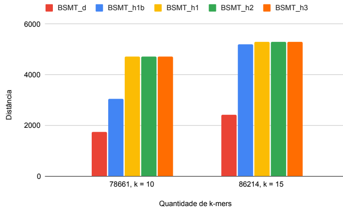
Figura 7.13: Média das distâncias: gráfico para a Tabela 7.13.
