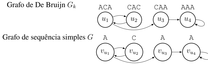
Figura 4.5: Exemplo da conversão de um grafo de De Bruijn G'_k (sem vértices com grau de entrada zero), onde k = 3 , para um grafo de sequência simples G . Neste exemplo, nenhum novo vértice é inserido, e os vértices têm seus rótulos alterados considerando o k -ésimo caractere de cada k -mer.
