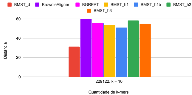
Figura 7.15: Média das distâncias: gráfico para a primeira linha da Tabela 7.15.
