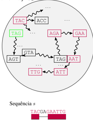
Figura 5.3: Passo 1 – quadrados roxos são sementes encontradas em G_k .
