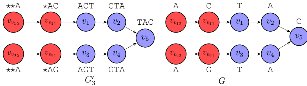
Figura 4.7: Exemplo de conversão de um grafo de De Bruijn G'_3 para um grafo de sequência simples G . Observe que essa conversão mantém a estrutura do grafo e apaga, de cada rótulo dos vértices, o prefixo de comprimento k - 1 .
