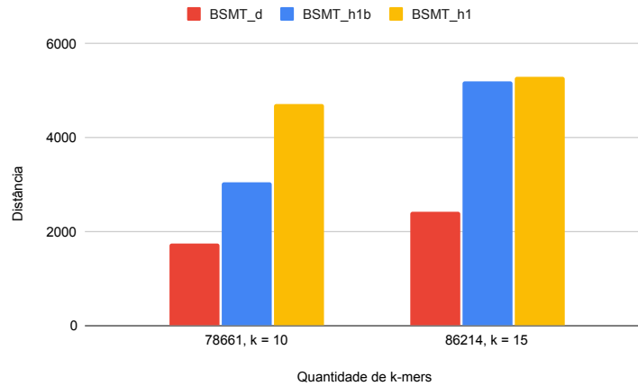
Figura 7.3: Média das distâncias: gráfico para a Tabela 7.3.
