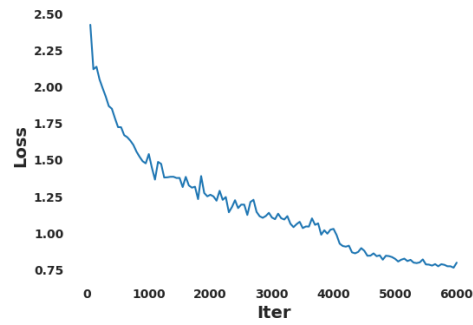
(d) ATSS
