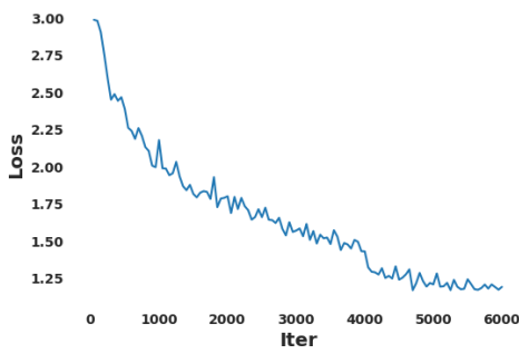
(a) Varifocal-Net
