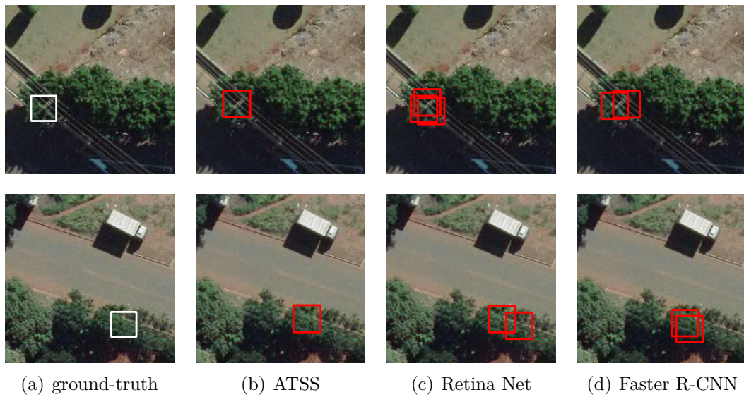
Figura 5 – Resultados obtidos pelos métodos quando localizando postes oclusos por topos de árvores: (a) ground-truth ; (b) ATSS; (c) RetinaNet; e (d) Faster R-CNN.
