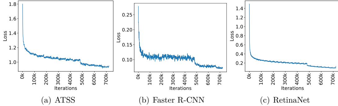
Figura 4 – Curva de erro durante o treinamento dos três métodos de detecção de objetos.
