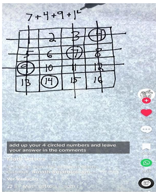
Figura 4.15 – Matriz mágica
