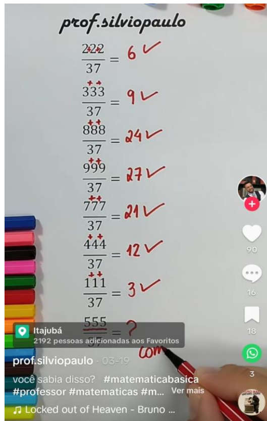
Figura 4.2 – O número 37
