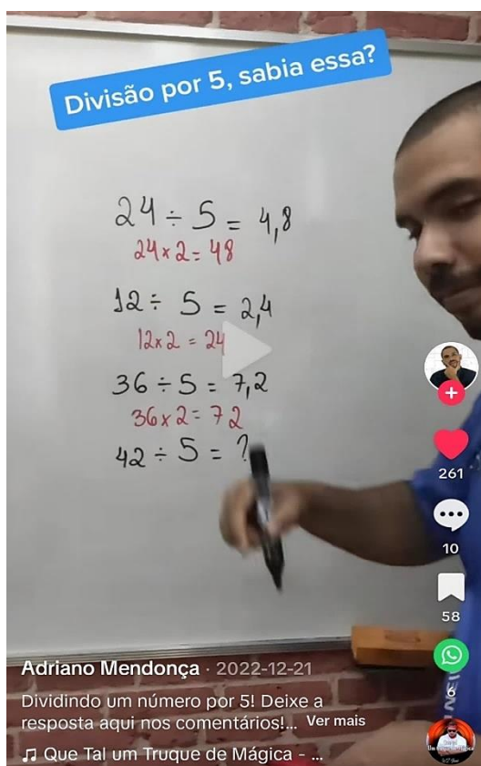
Figura 4.1 – Divisão por 5
