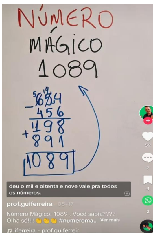
Figura 4.11 – O número 1089
