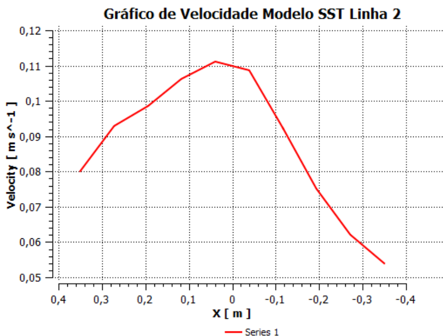
Figura 21: Curva comportamental de velocidade do Modelo SST Transition.
