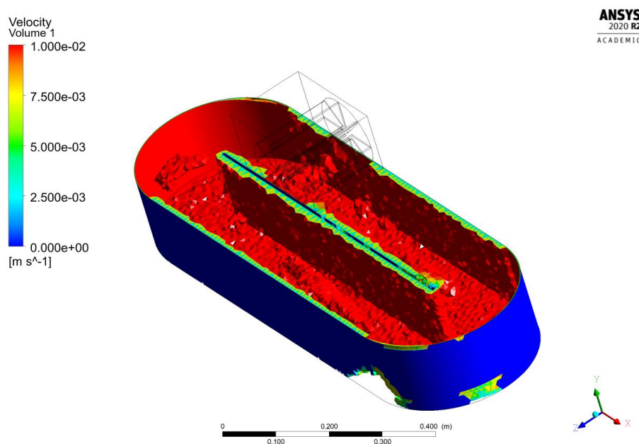
Figura 22: Volume morto com escala de velocidade até 0,01m/s.
