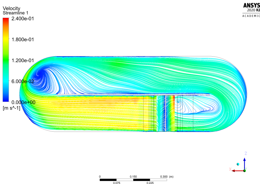
Figura 26: Linhas de velocidade na altura 0,135m, para fluxo inverso.
