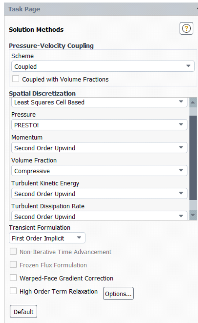
Figura 7: Imagem que mostra as resoluções usadas no método acoplado.
