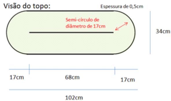
Figura 12: Geometria do tanque, planta.
