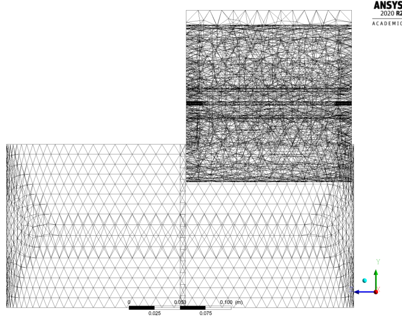
Figura 5: Malha completa, vista lateral esquerda.
