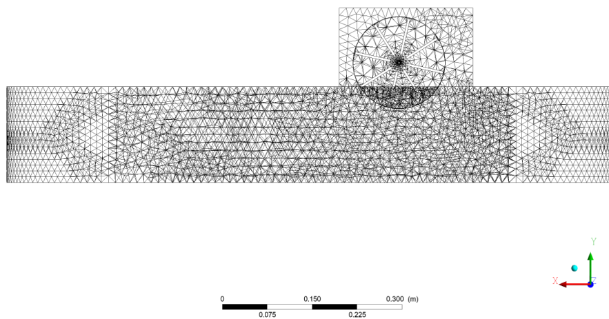
Figura 3: Malha completa, vista frontal.
