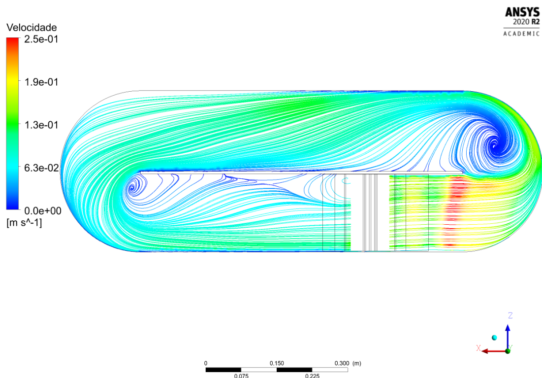
Figura 18:: Linhas de velocidade na altura de 0,135 m, representando o modelo Transition SST.
