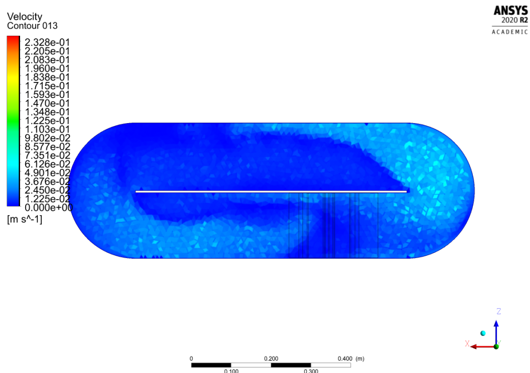
Figura 24: Velocidade de fundo do sistema.
