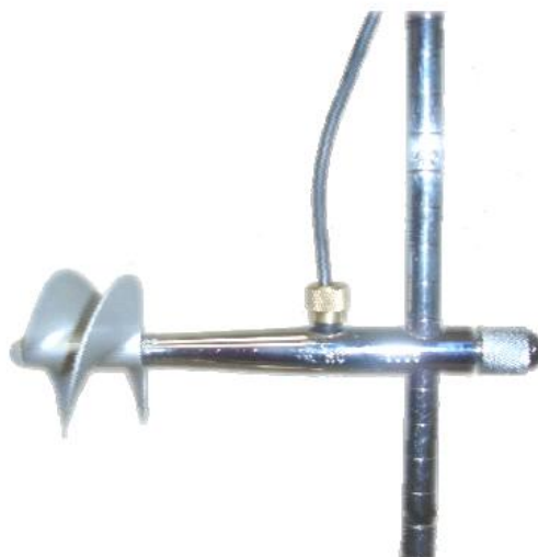
Figura 9: Equipamento de medição de vazão, micromolinete.
