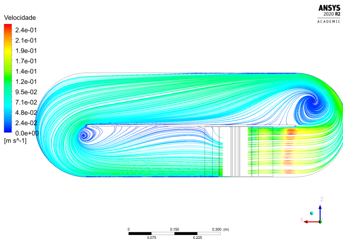
Figura 17: Linhas de velocidade na altura de 0,135 m, representando o modelo k-\varepsilon .
