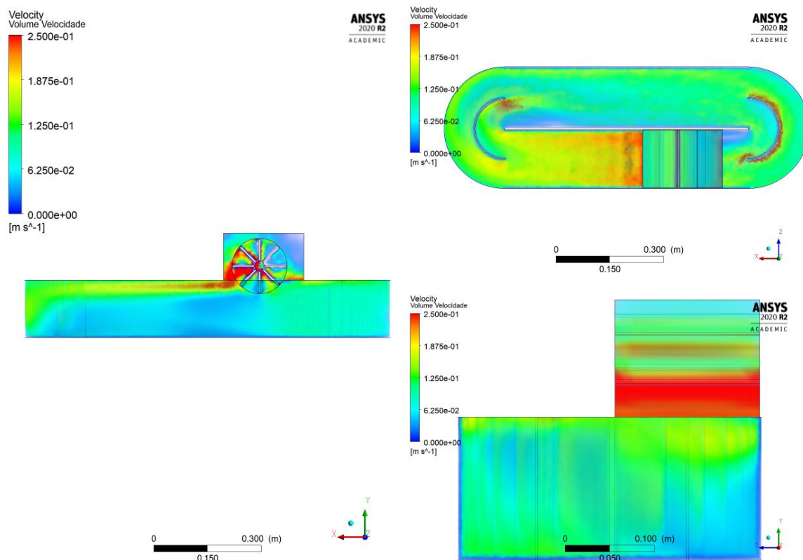
Figura 29: Velocidade do sistema com defletores de fluxo, vista em 3 perfis.
