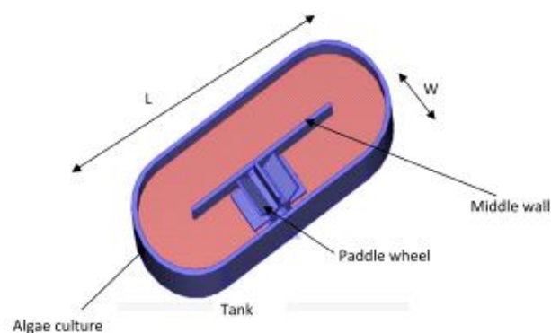
Figura 11: Design do tanque (Hadiyanto et al., 2013).
