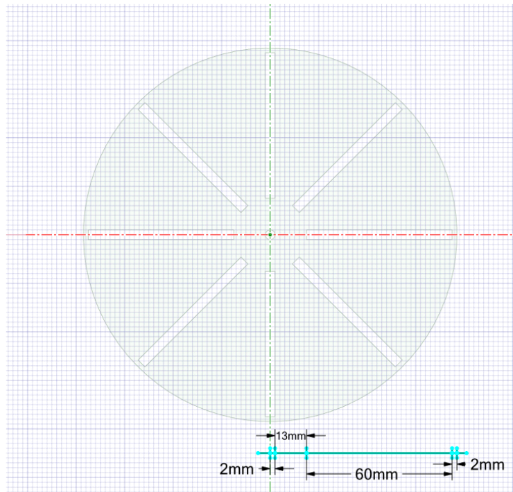
Figura 15: Eixo do paddlewheel com suas dimensões.
