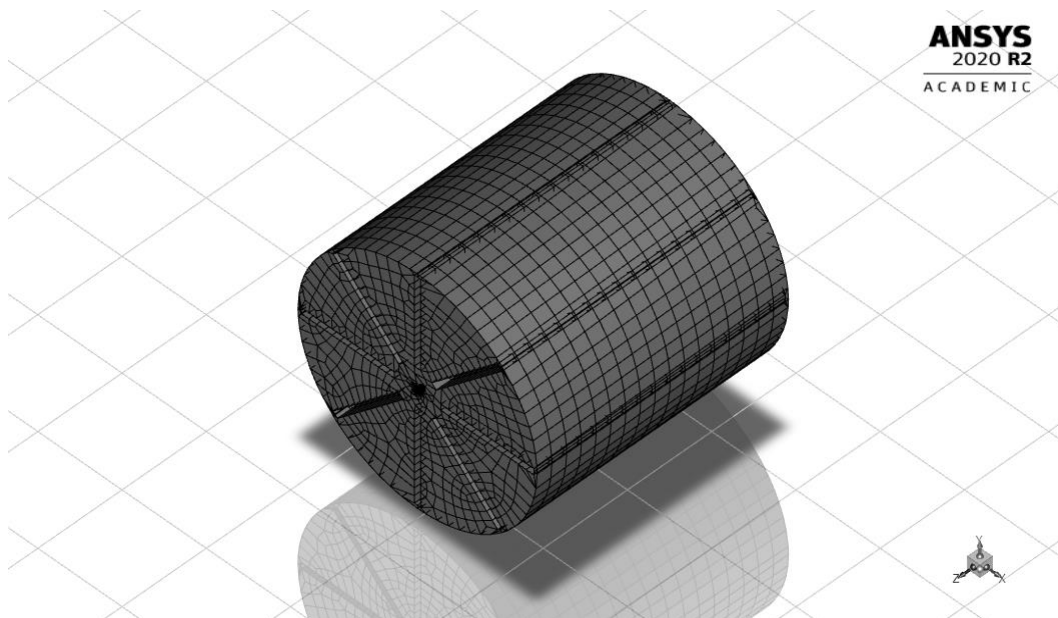
Figura 1: Malha 3D modelada para representar o paddlewheel .
