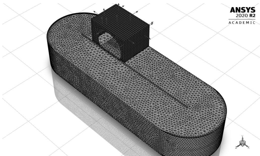
Figura 2: Malha 3D modelada para representar o fluido, sendo o bloco retangular a representação do ar atmosférico.
