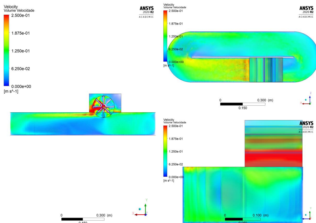
Figura 27: Velocidade do sistema de fluxo invertido, vista em 3 perfis.
