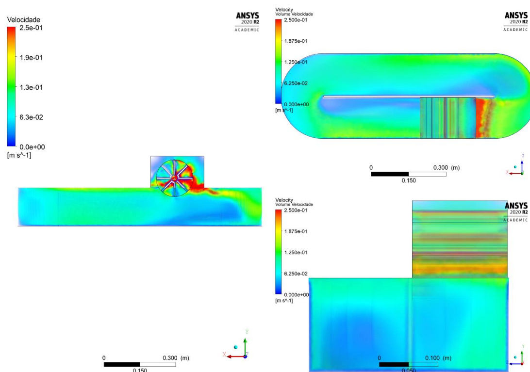
Figura 25: Velocidades do sistema vista em 3 perfis.
