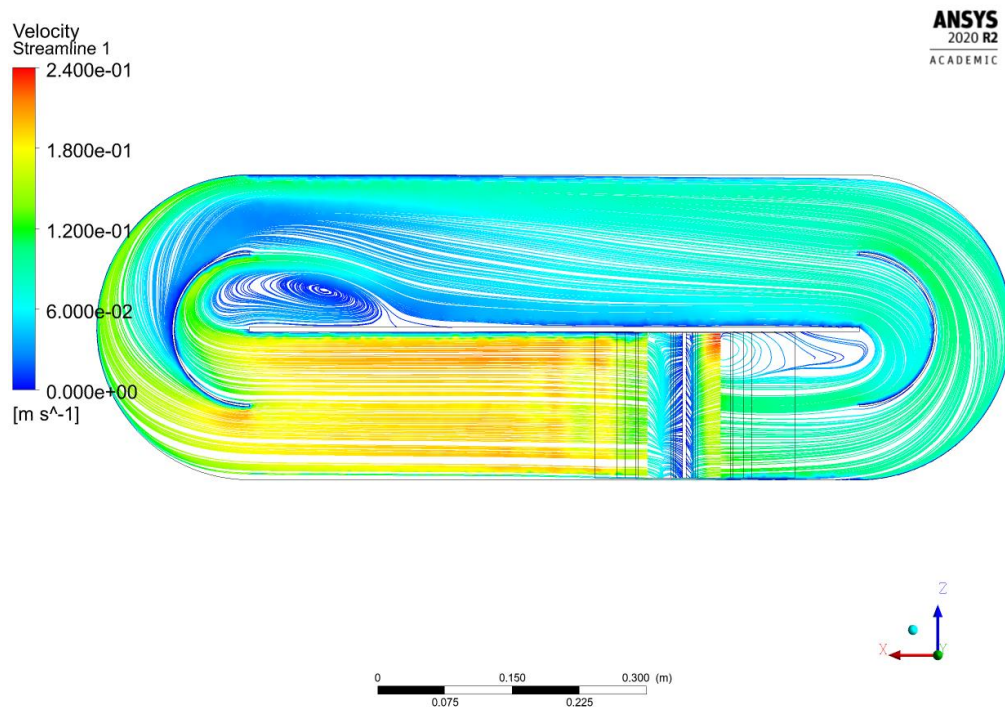
Figura 28: Linhas de velocidade na altura 0,135m, para defletores de fluxo.
