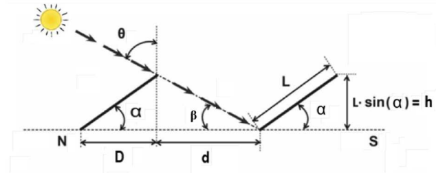
Figura 6 – Espaçamento entre as placas e sombreamento.
