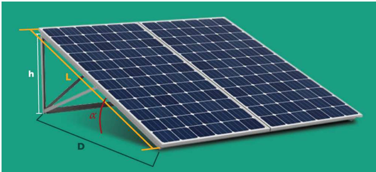
Figura 21 – Posicionamento de instalação de uma placa fotovoltaica.
