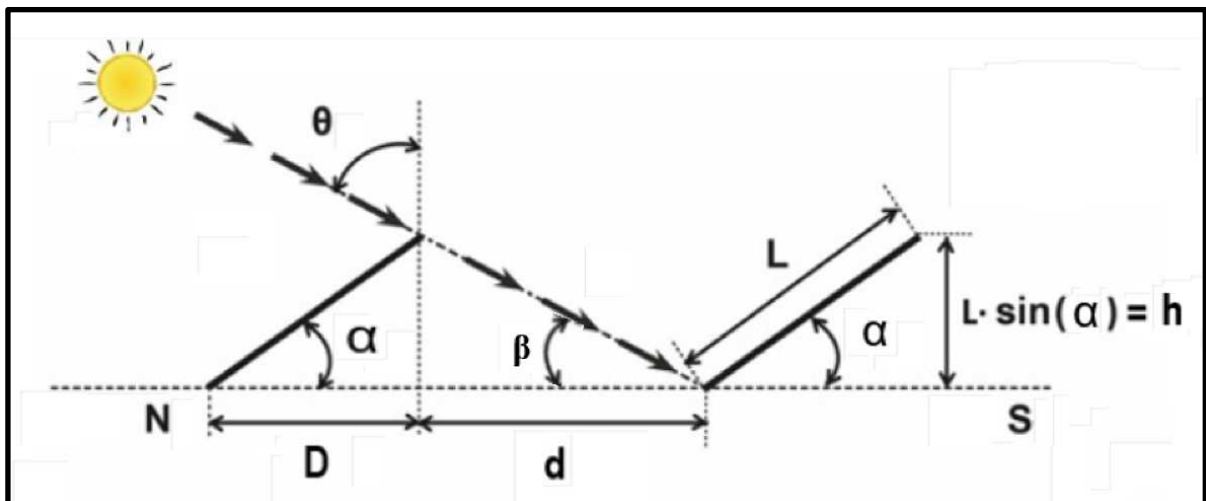
Figura 22 – Determinação do espaçamento entre as linhas das placas.
