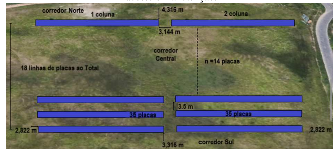
Figura 7 – Disposição das placas e espaçamentos dos corredores de acesso e manutenção.
