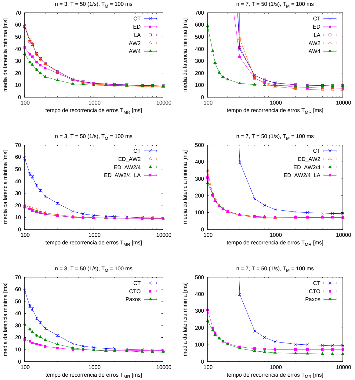
Figura A.7: Avaliação das otimizações. Latência vs. T_{MR} para \lambda = 0,1 ms.
