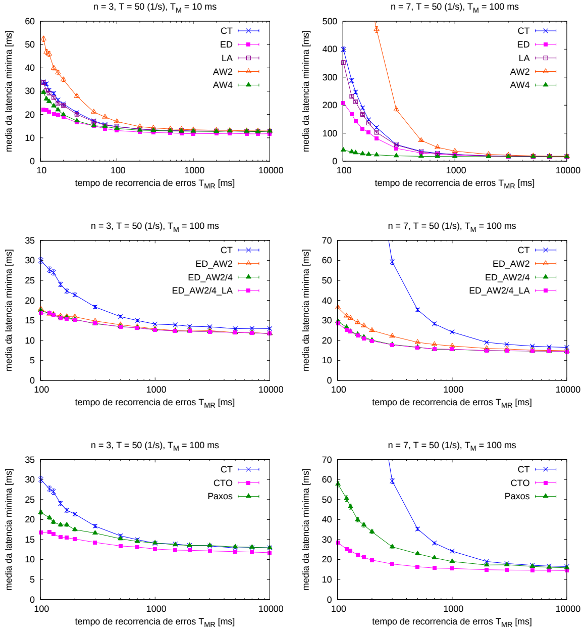
Figura A.9: Avaliação das otimizações. Latência vs. T_{MR} para \beta = 5 ms.
