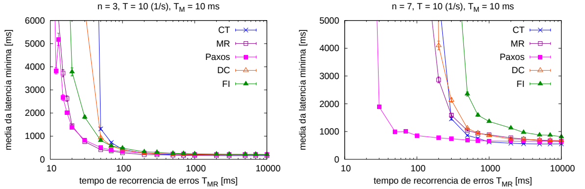
Figura 5.9: Comparação dos algoritmos. Latência vs. T_{MR} para \lambda = 10 ms.
