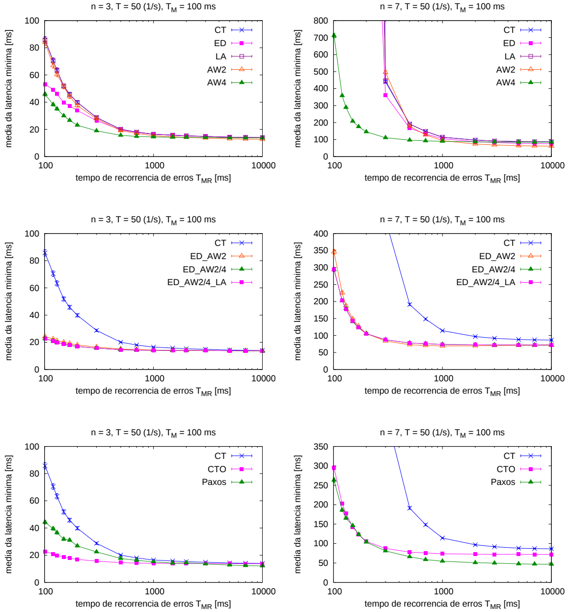
Figura A.6: Avaliação das otimizações. Latência vs. T_{MR} para \lambda = 1 ms.
