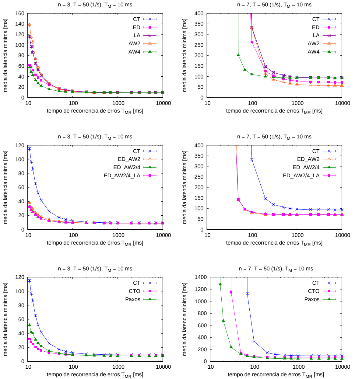
Figura A.1: Avaliação das otimizações. Latência vs. T_{MR} para \lambda = 0,1 ms.
