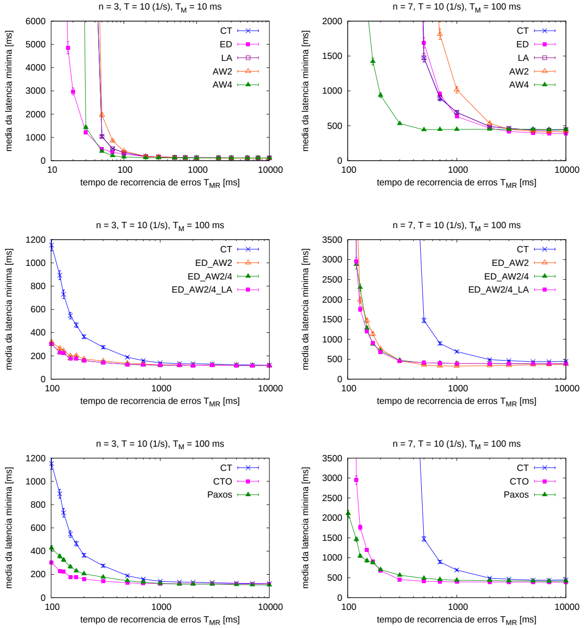
Figura A.8: Avaliação das otimizações. Latência vs. T_{MR} para \lambda = 10 ms.
