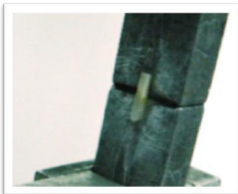
Figura 09- Dispositivo com o palito em posição na máquina de ensaio
