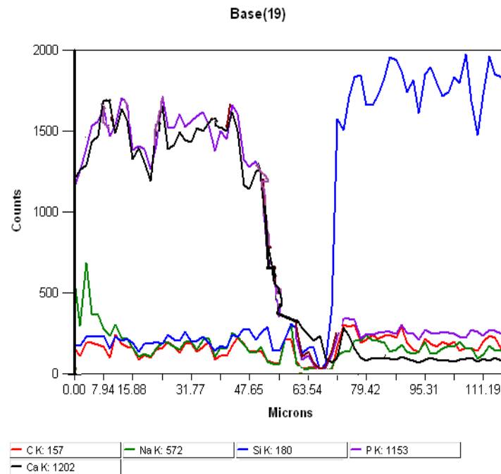
Figura 21- Gráfico 02- Microanálise do palito 10 (figura 23) pelo método de espectroscopia de energia dispersiva de Raios-X (EDX).
