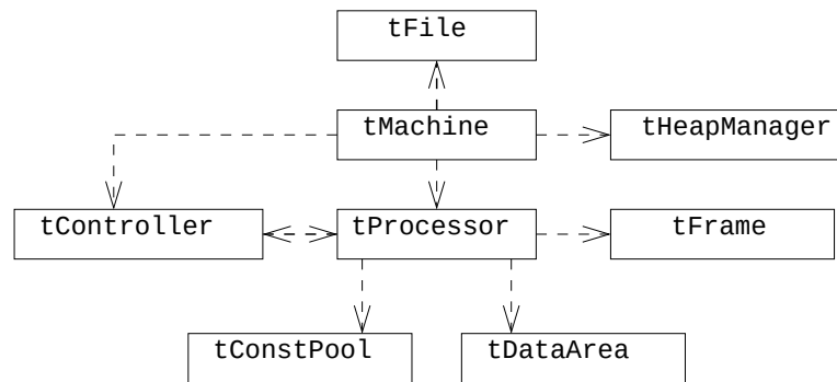
Figura 4.1: Arquitetura da MVL.
