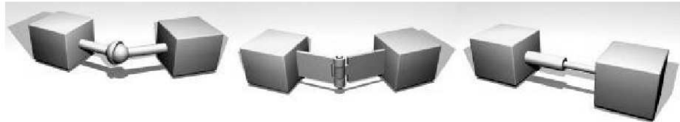
Figura 2.11: Exemplo de junções: esférica, de revolução e cilíndrica.
