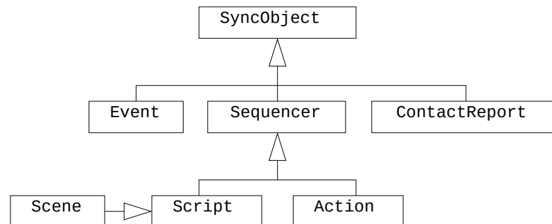
Figura 3.2: Classes de seqüenciadores e evento.
