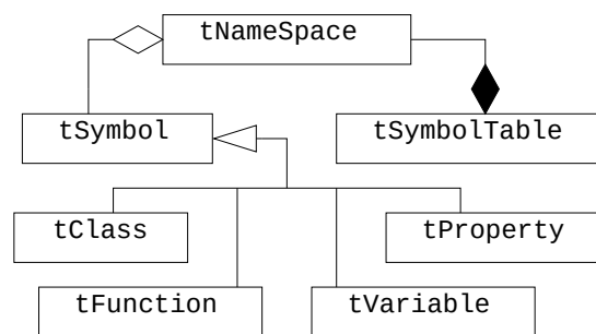
Figura 3.8: Classes da tabela de símbolos.
