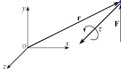
Figura 2.3: Torque sobre uma partícula.
