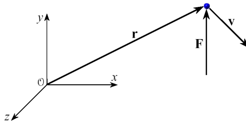
Figura 2.2: Resultante das forças que atuam numa partícula.
