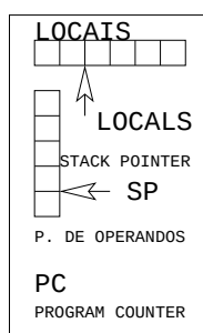
Figura 4.5: O formato de um frame comum.
