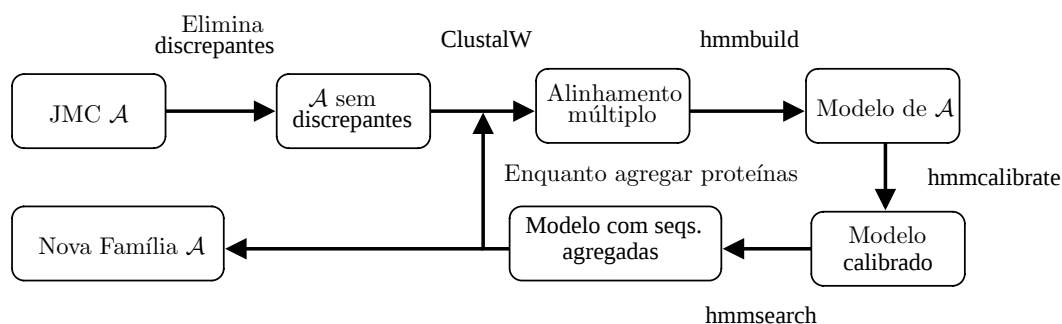
Figura 4.2: Fluxo de execução da fase Busca Homólogos
