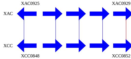
Figura 3.6: Representação gráfica do run do trecho de arquivo da Figura 3.5
