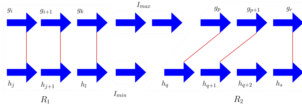
Figura 3.7: Exemplo de uma junção entre dois runs R_1 e R_2 .
