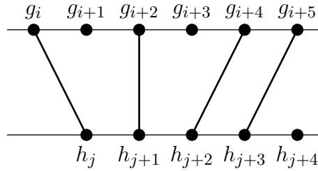
Figura 3.3: Representação de uma espinha dorsal de duas Regiões de Genes Consecutivos - RGCs.
