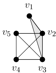
Figura 2.4: Exemplo de uma clique de tamanho 3 formada pelos vértices v_1, v_2 e v_3 .
