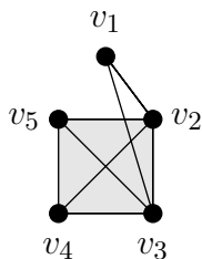
Figura 2.5: Exemplo de uma clique de tamanho 4 maximal formada pelos vértices v_2, v_3, v_4 e v_5 .
