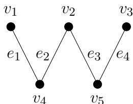
Figura 2.3: Exemplo de um grafo bipartido, tal que X = \{v_1, v_2, v_3\} e Y = \{v_4, v_5\} .
