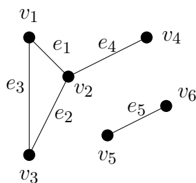
Figura 2.2: Exemplo de um grafo com seis vértices e cinco arestas.
