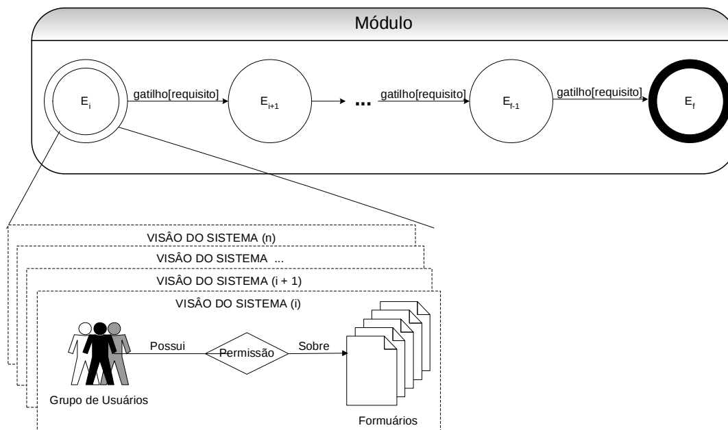
Figura 4.13: Estrutura de um Módulo.
