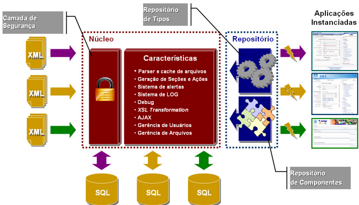
Figura 4.3: Arquitetura do framework Titan.
