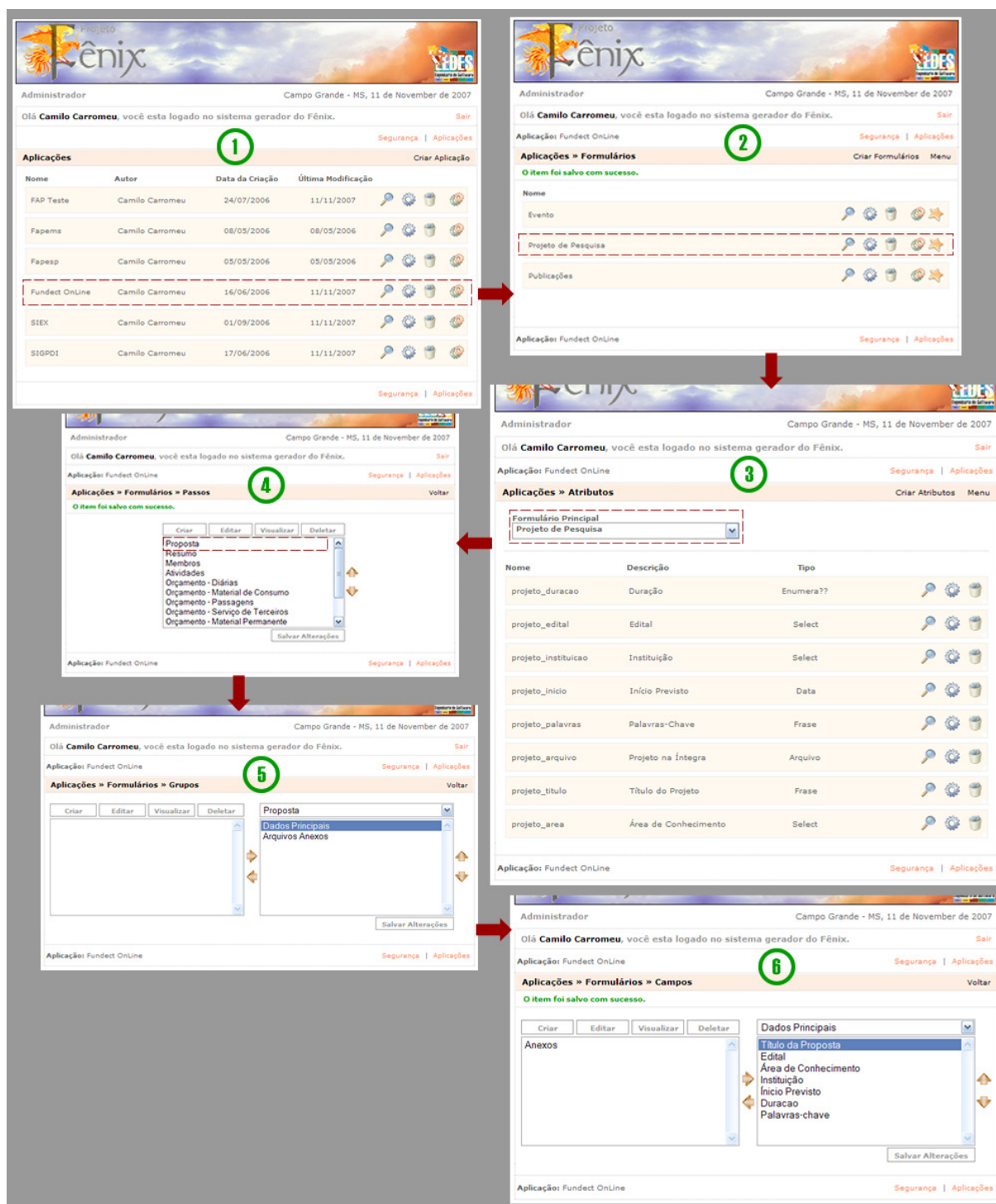
Figura 5.3: Criação de formulário eletrônico para a modalidade “Projeto de Pesquisa” e configuração do primeiro passo.
