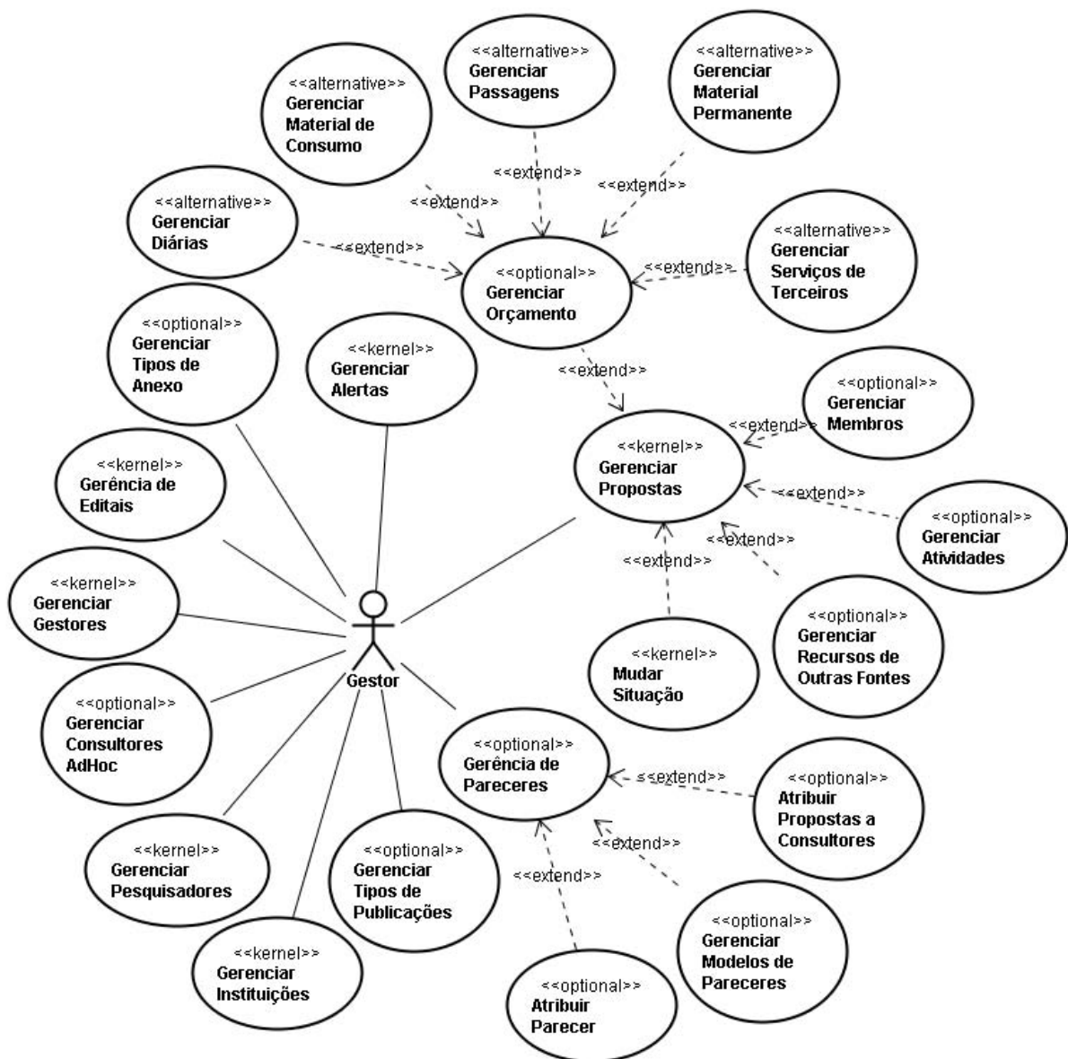
Figura 3.9: Diagrama de casos de uso para o ator Gestor.
