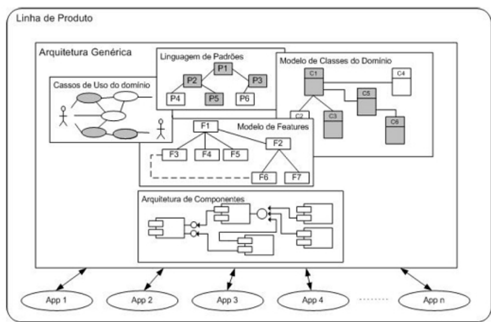
Figura 2.2: Representação de uma LPS ([3], p.12).
