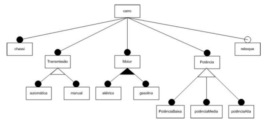
Figura 2.3: Exemplo de modelo de features ([64], p.3).
