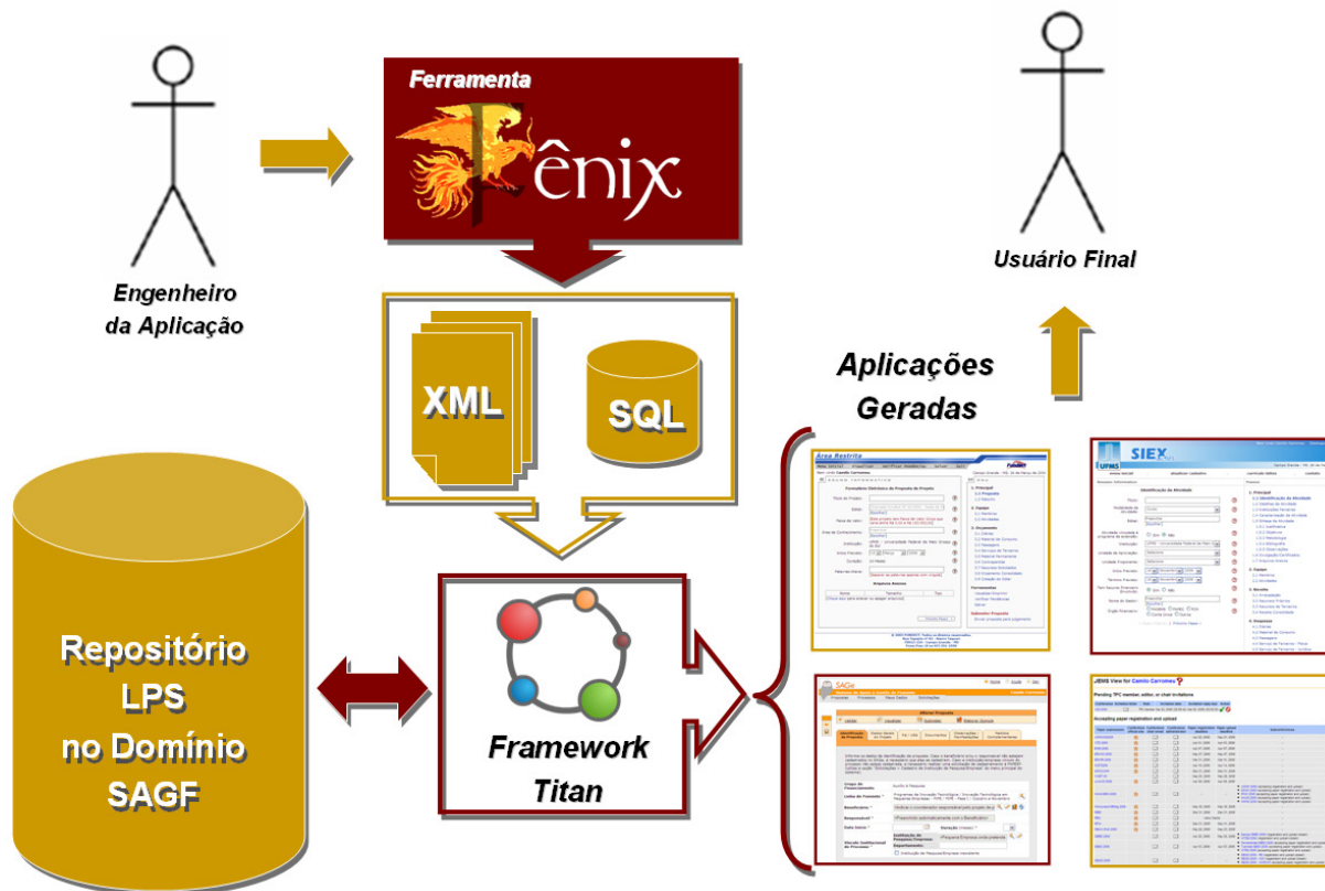
Figura 4.1: Ambiente de geração de aplicações.
