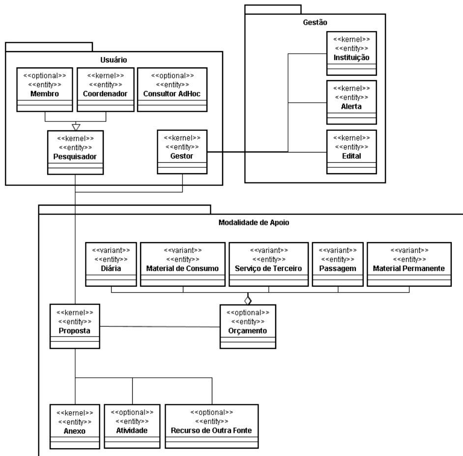
Figura 3.19: Arquitetura baseada em componentes da LPS de SAGF.
