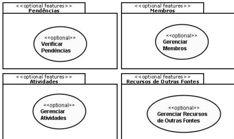
Figura 3.14: Pacotes de casos de uso para as features opcionais Pendências, Membros, Atividades e Recursos de Outras Fontes.
