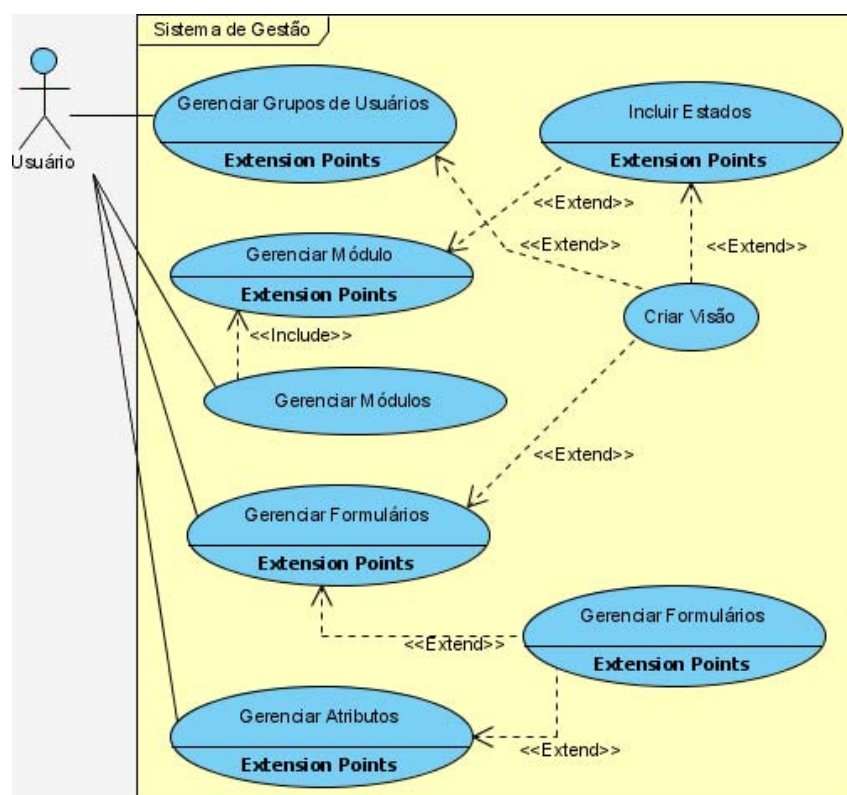
Figura 4.12: Diagrama de casos de uso para o Sistema de Gestão do Fênix.
