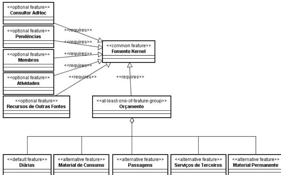
Figura 3.17: Dependências de features da Linha de Produto de SAGF.
