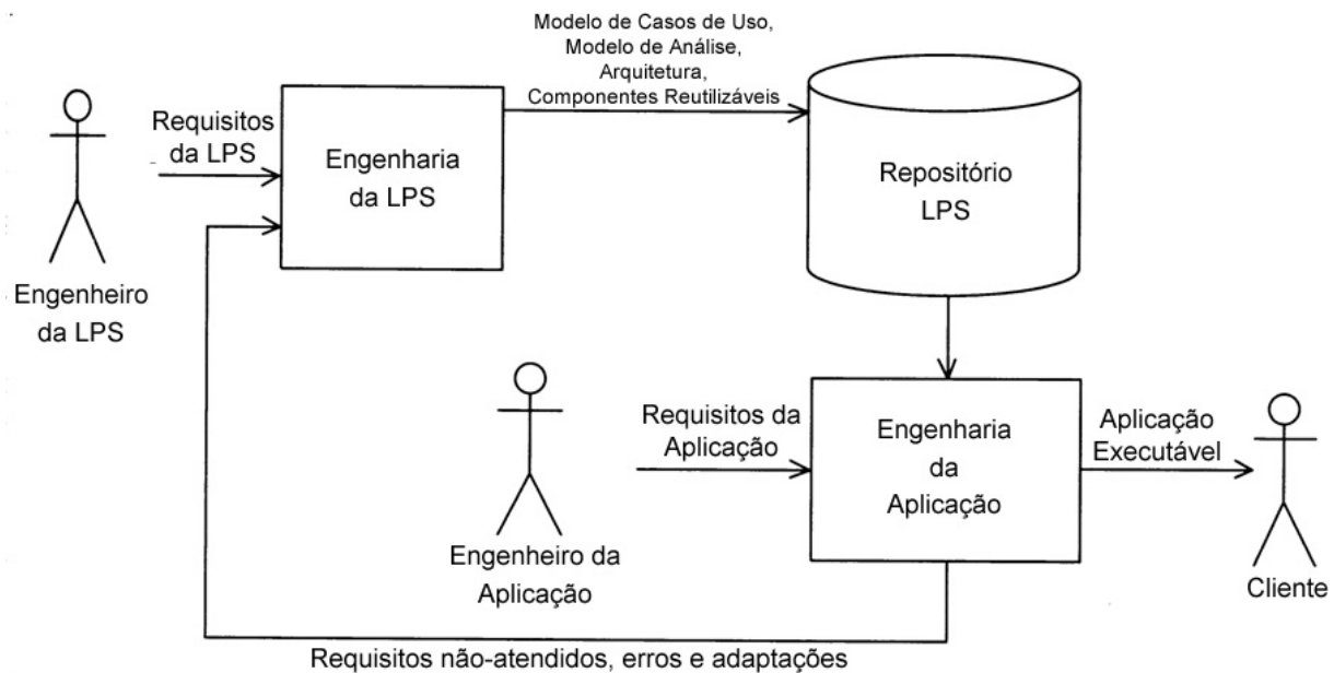
Figura 3.6: Ciclos do Processo ESPLEP ([56], p. 45).
