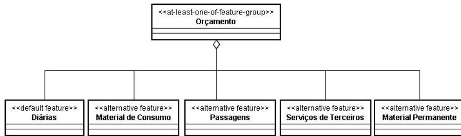
Figura 3.16: Dependências entre as features da variabilidade de Orçamento.
