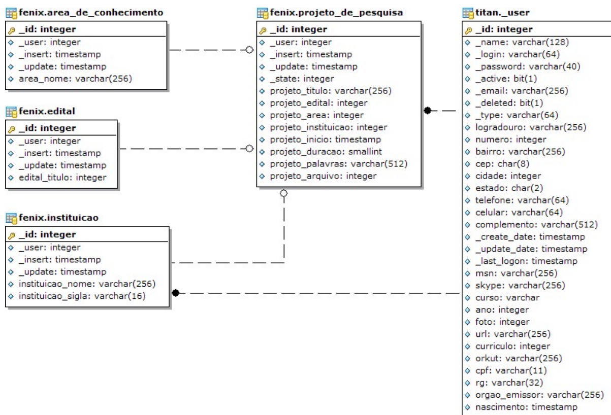
Figura 5.4: Diagrama entidade-relacionamento gerado para o formulário eletrônico da modalidade "Projeto de Pesquisa".
