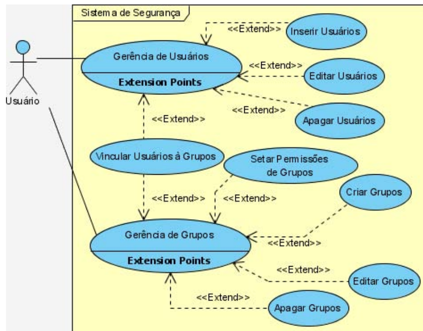
Figura 4.9: Diagrama de casos de uso do Sistema de Segurança do Fênix.
