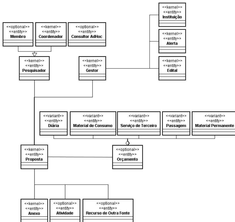
Figura 3.18: Modelo estático de classes de entidade.
