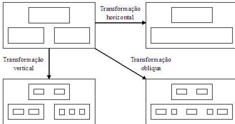
Figura 2.1: Transformações vertical, horizontal e oblíqua [34].
