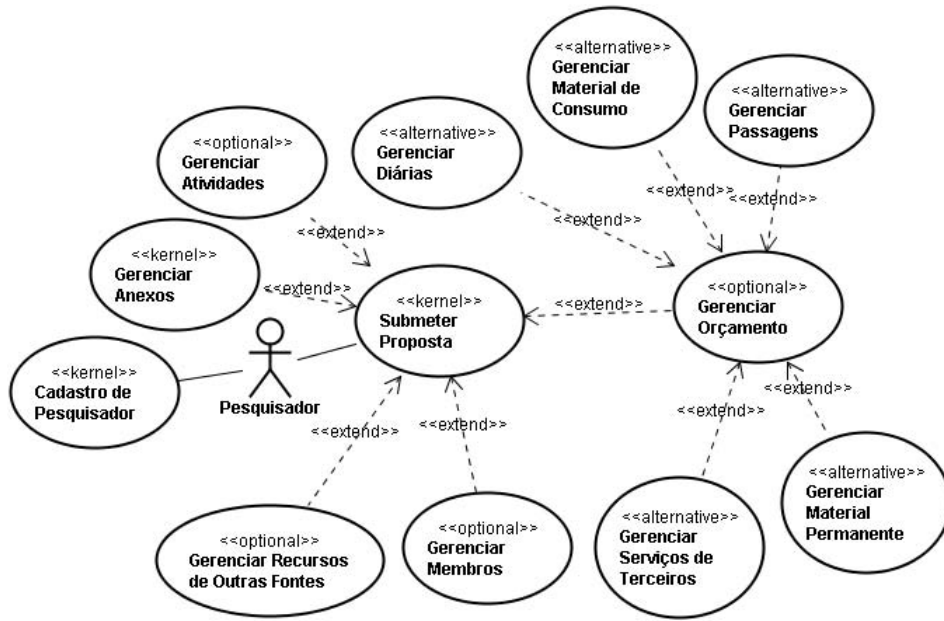
Figura 3.10: Diagrama de casos de uso para o ator Pesquisador.
