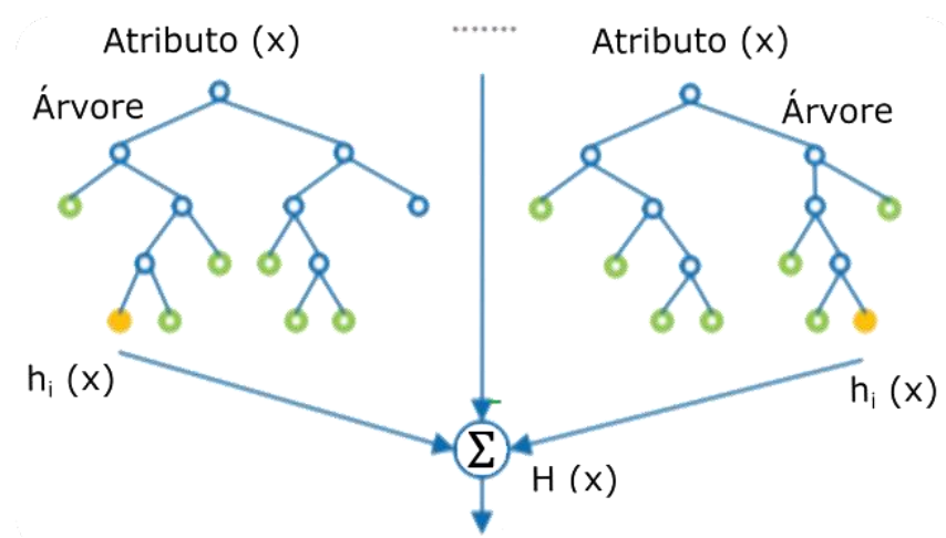
Figura 6. Método de Random Forest. Fonte: Zhao et al. (2017).
