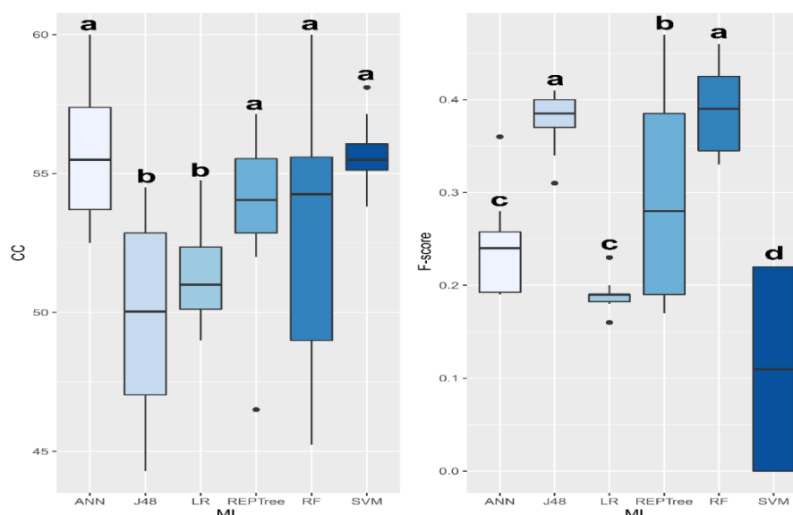
Figura 5. Boxplot para médias de classificações corretas (CC, %) e F-score considerando a análise de regressão logística (LR) e técnicas de AM: redes neurais (ANN), algoritmos de árvores de decisão J48 e REPTree, random forest (RF) e máquina de vetor de suporte (SVM). Grupos de médias com letras iguais não diferem entre si pelo teste de Scott-Knott a 5% de significância.
