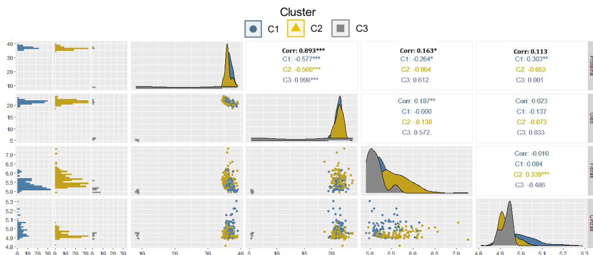
Figura 4. Gráfico de correlações e dispersão entre os clusters e as variáveis proteína, óleo, fibras e cinzas; ***, ** e *: significativo a 0,1%, 1% e 5% de probabilidade respectivamente pelo teste F.
