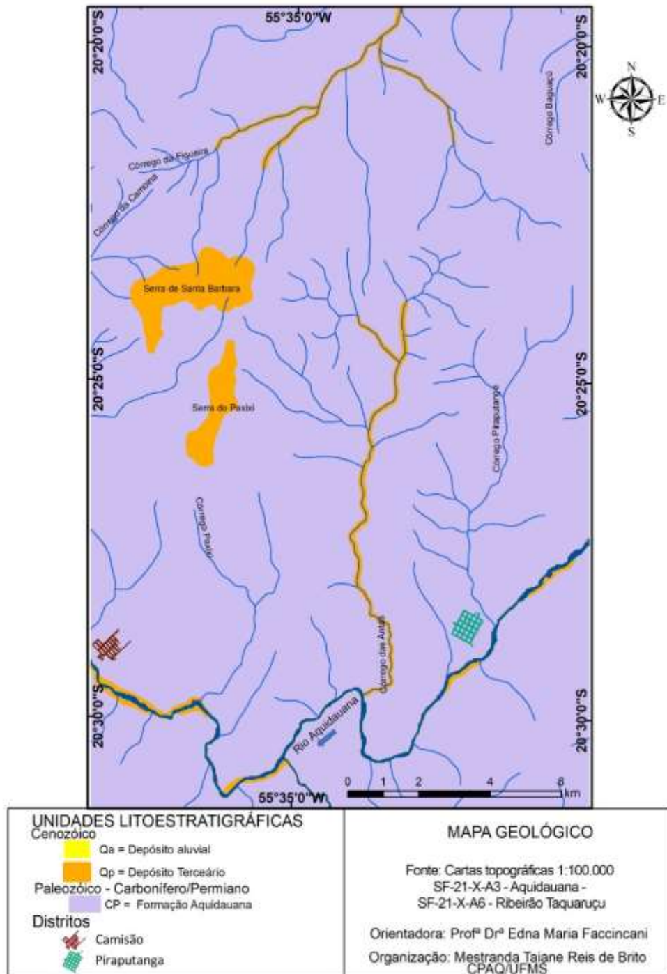
Figura 22. Mapa Geológico.
