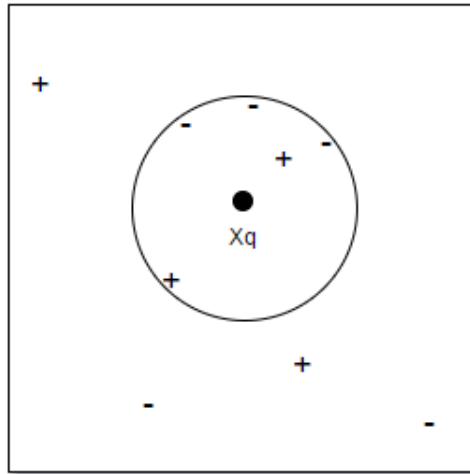
Figura 3.7: Na figura um conjunto de exemplos positivos e negativos, com um exemplo x_q a ser classificado. Para k = 1 , x_q será classificado com + , entretanto para k = 5 , x_q será classificado como - .
