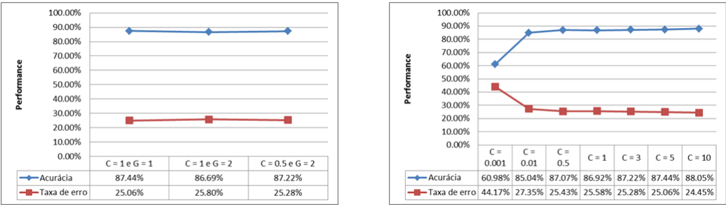
(a) Efeito dos parâmetros C e G sobre a performance do modelo LibSVM com o Kernel RBF (b) Efeito do parâmetro C sobre a performance do modelo LibSVM com o Kernel Linear
