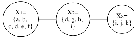
Figura 1.2: Uma decomposição em árvore para G .
