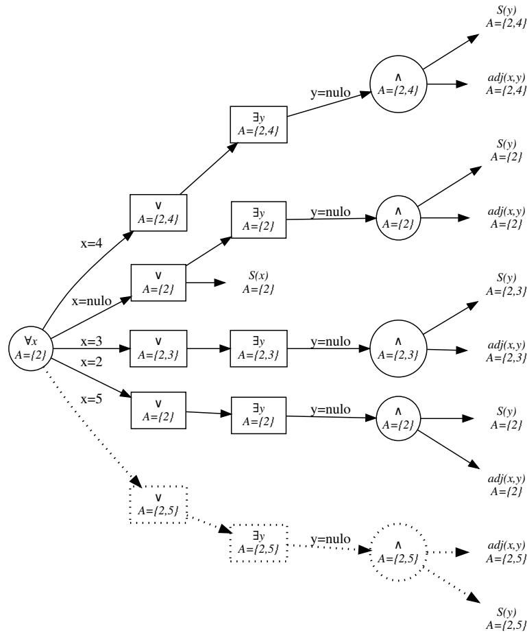
Figura 3.5: Jogo \mathcal{G} cuja estrutura é um caminho com 6 vértices tal que os vértices são rotulados de 0 a 5 de forma que (i, i+1) é uma aresta no caminho. Além disso, U = \{\} . Arestas pontilhadas denotam que não pertencem mais ao jogo.
