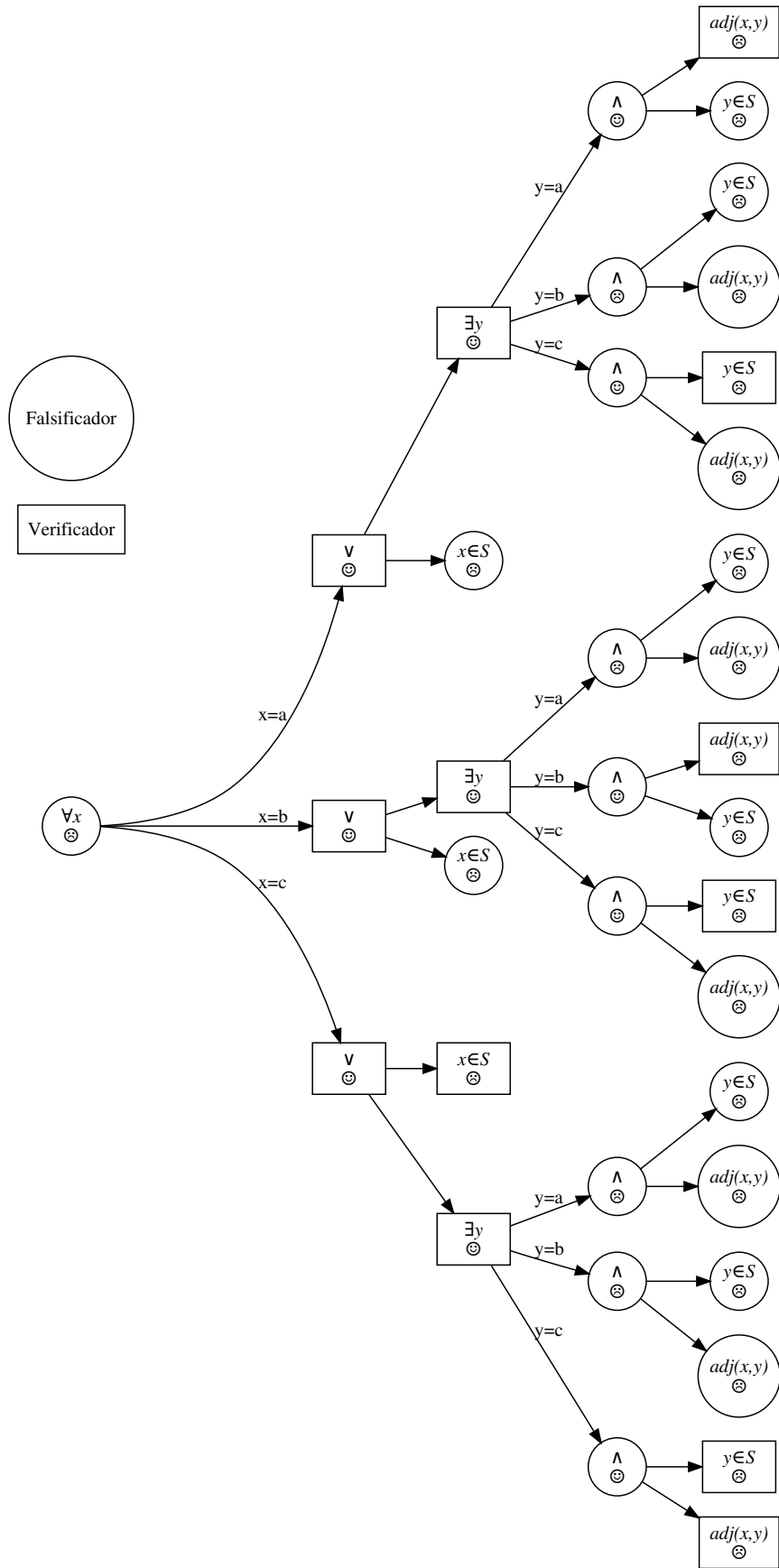
Figura 2.5: Jogo de avaliação da fórmula cd(S) .
