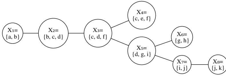
Figura 1.3: Outra possível decomposição em árvore para G .
