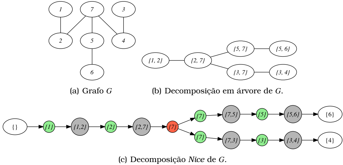
Figura 3.1: Exemplo de Decomposição em Árvore Nice.
