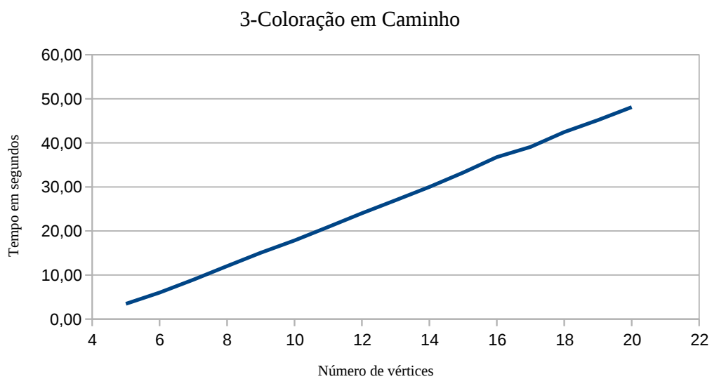
Figura 4.2: Gráfico de n para Tempo em Segundos .
