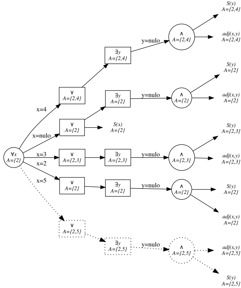
Figura 3.8: Jogo \mathcal{G}_1 retornado do Algoritmo 3.5, que teve como entrada o jogo \mathcal{G} da Figura 3.7 com x = 3 e U = \{\} . O grafo considerado aqui é um caminho com 6 vértices. Arestas pontilhadas denotam que não pertencem mais ao jogo.
