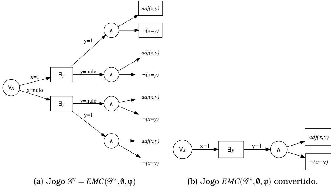
Figura 3.2: Um exemplo de entrada e saída do Algoritmo 3.1.
