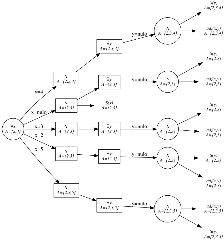
Figura 3.7: O jogo \mathcal{G} retornado da função combine(\mathcal{G}_1, \mathcal{G}_2) , tal que \mathcal{G}_1 e \mathcal{G}_2 são os jogos da Figura 3.6. O grafo considerado nesse jogo é um caminho com 6 vértices e U = \{\} .
