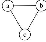
Figura 2.4: Um grafo G_2 .
