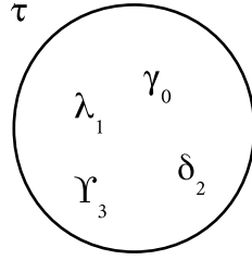
Figura 2.1: Ilustração de um vocabulário \tau .
