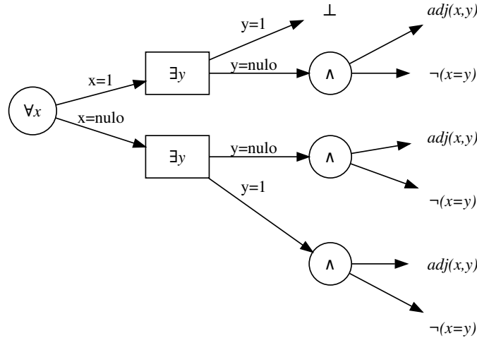
Figura 3.3: Jogo \mathcal{G}_1 = \text{avaliaEMC}(\mathcal{G}') para o jogo \mathcal{G}' da Figura 3.2(a).
