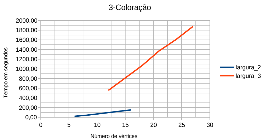
Figura 4.3: Gráfico de n para Tempo em Segundos utilizando grids . Cada reta é a representação do intervalo de valores para grids com a mesma largura de decomposição.
