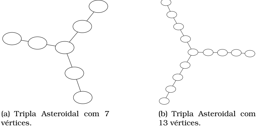
Figura 4.1: Exemplos de Triplas Asteroidais.
