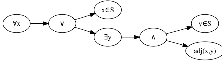
Figura 2.3: Árvore da fórmula cd(S) .
