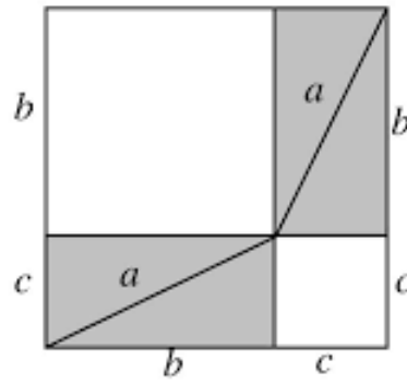
Figura 2.2: Quadrado de lados b + c (Parte 2).
