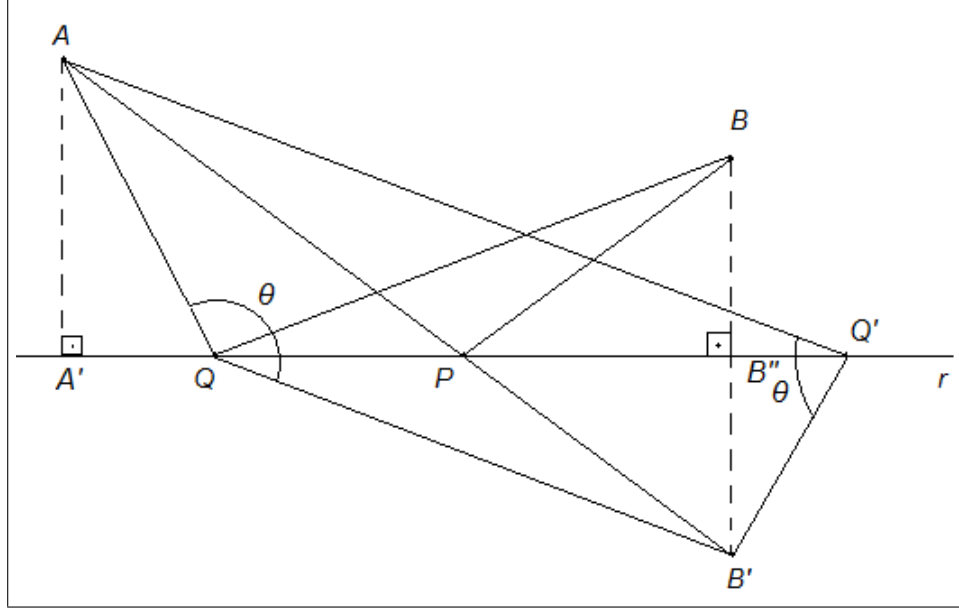
Figura 3.7: Caminho mínimo.
