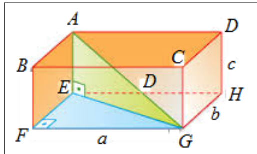
Figura 3.8: Paralelepípedo retângulo.
