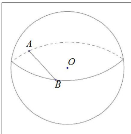
Figura 4.5: Corda de superfície.
