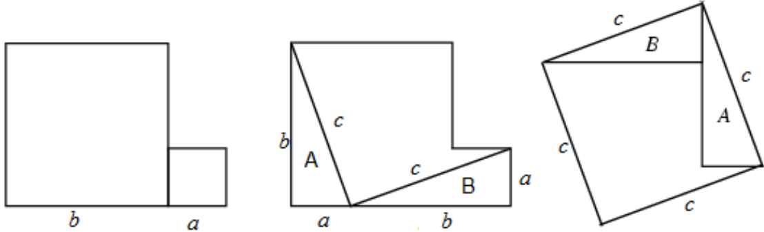
Figura 2.11: Thabit ibn-Qurra.
