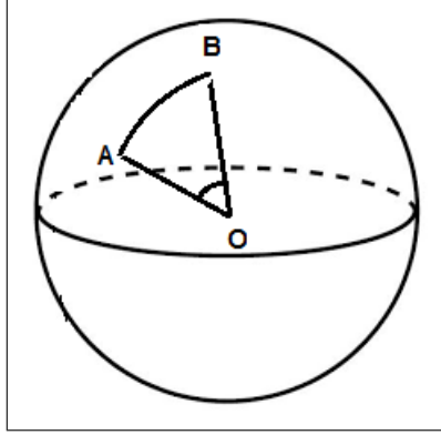
Figura 4.10: Curva geodésica.
