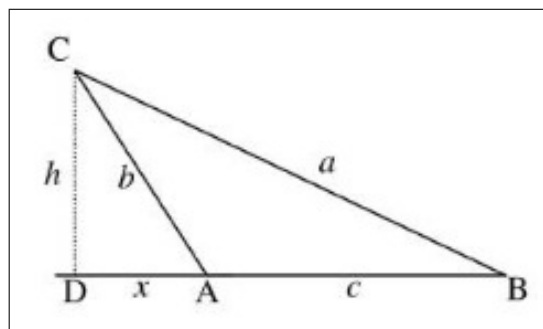
Figura 2.20: Recíproca do Teorema de Pitágoras.
