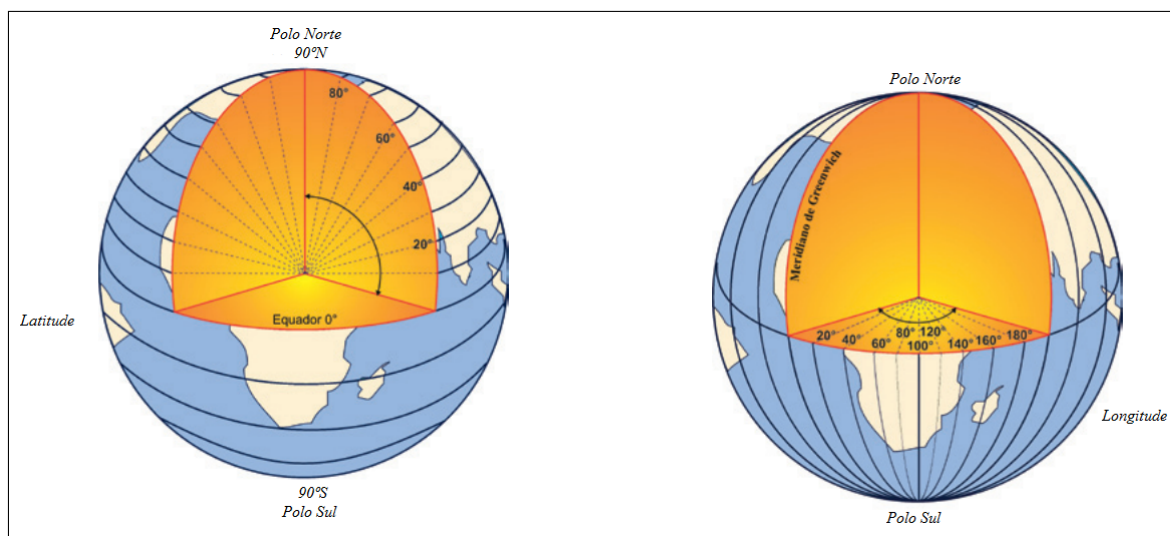
Figura 4.8: Latitude.
