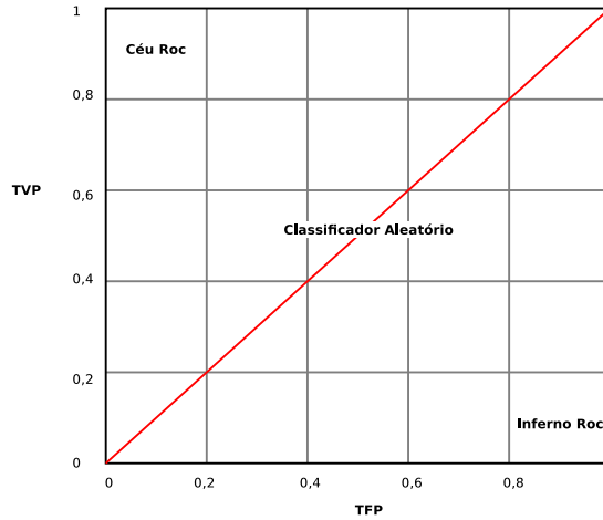
Figura 3.4: Gráfico ROC.
