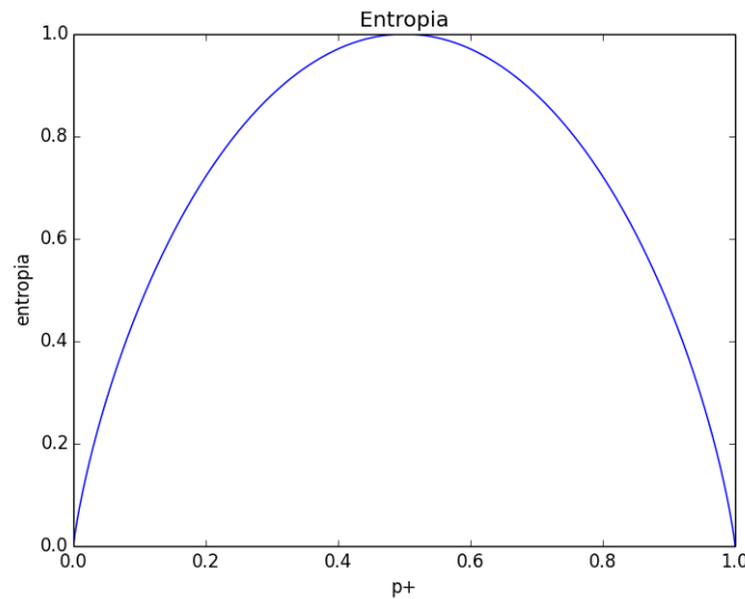
Figura 2.3: Cálculo de Entropia, (Shannon, 2001).
