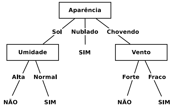
Figura 2.2: Previsão do Tempo, adaptado de: (Mitchell, 1997).
