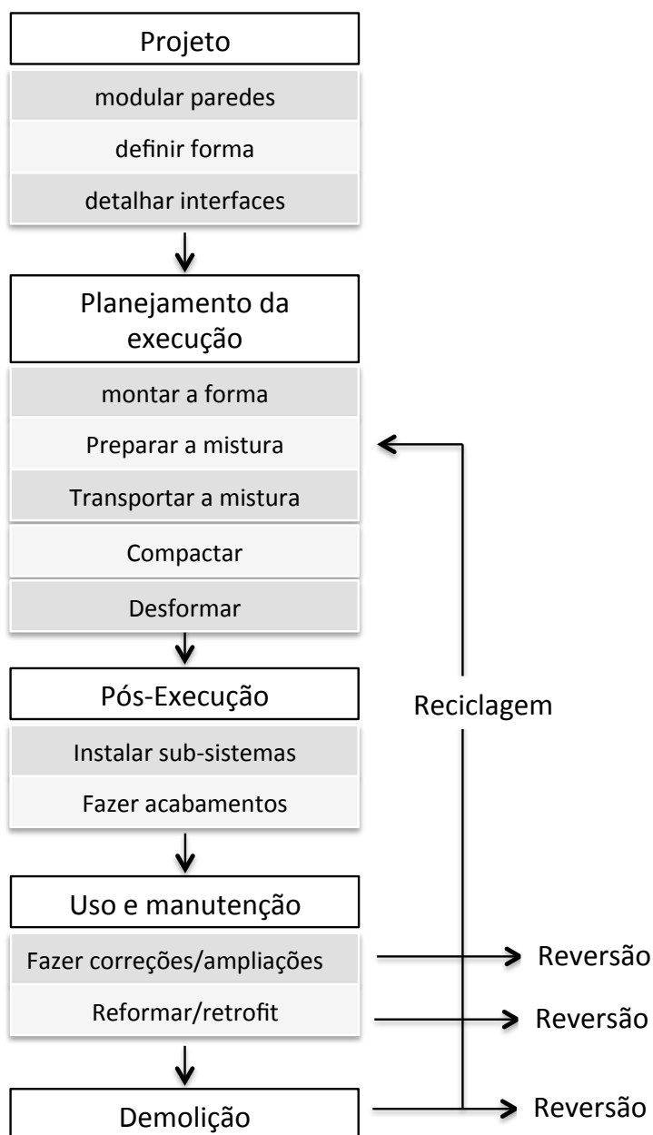
Figura 57: Processo de produção/ciclo de vida de paredes de taipa.
