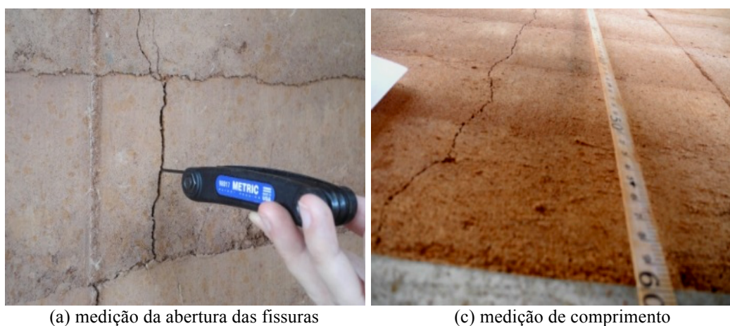
Figura 43: Etapas da medição das fissuras e trincas.
