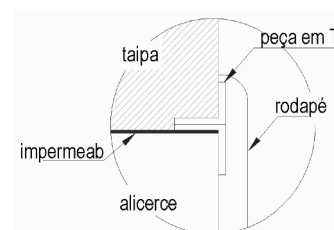
Remediação (corte)
