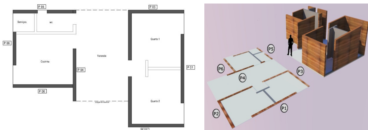
Figura 31. Ordem de execução das paredes do protótipo de habitação.
