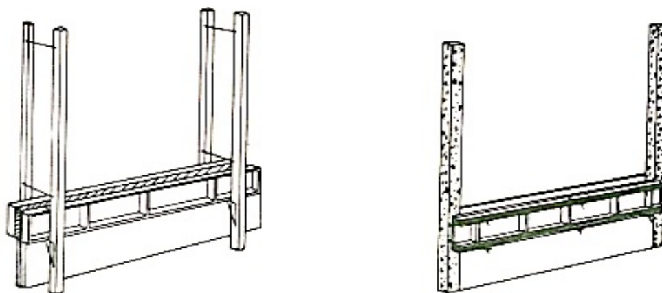
Figura 12: Sistema G-1 à esquerda e sistema G-2 à direita
