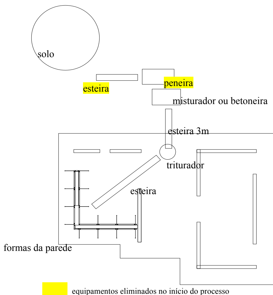
Figura 37: Layout do canteiro e conjunto de máquinas utilizadas na execução da parede 6.
