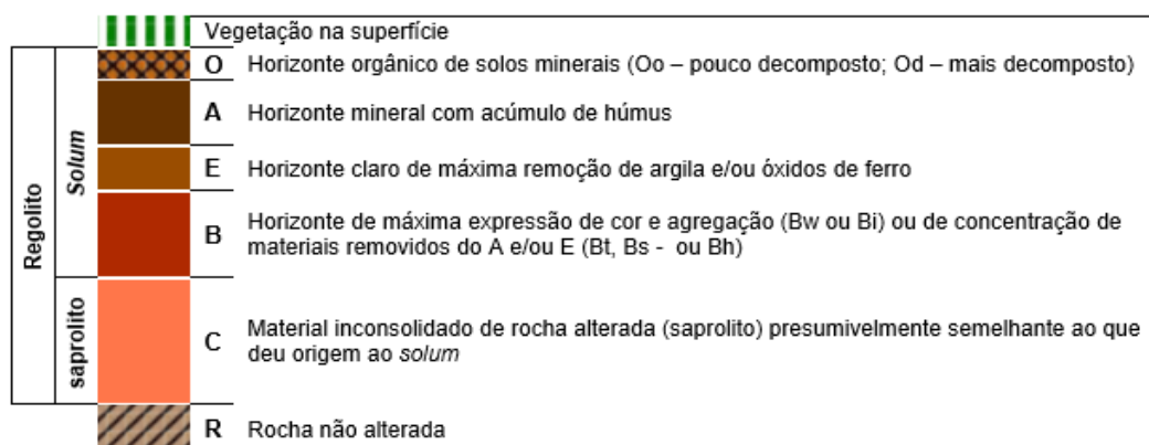
Figura 1: Horizontes principais do solo
