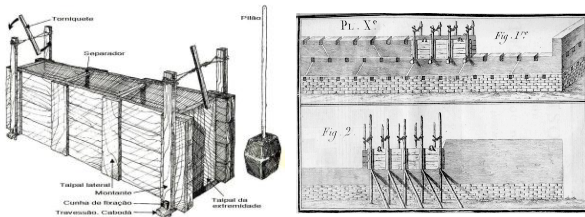
Figura 10: Sistemas de formas tradicionais
