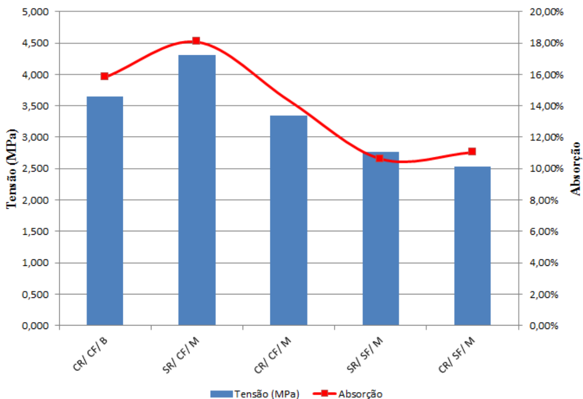
Figura 55: Valores de resistência à compressão simples dos corpos de prova e capacidade de absorção de água da mistura de solo-cimento e solo-cimento-fibras
