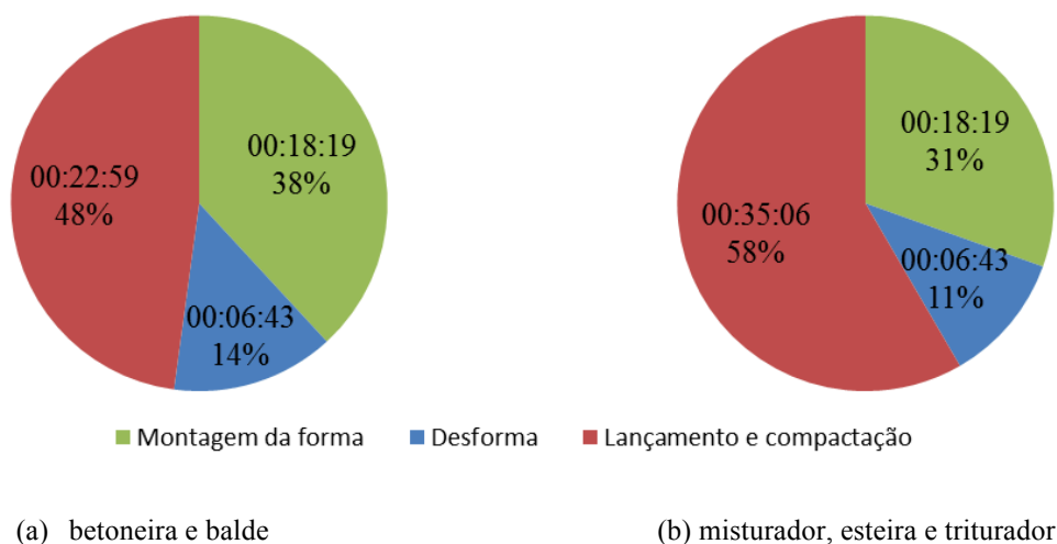
Figura 56. Comparação entre os processos construtivos.
