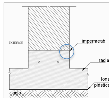
Proposta inicial (corte)
