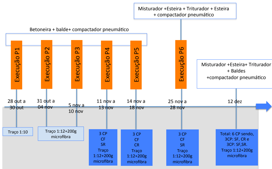
Figura 53: Linha do tempo referente a construção das paredes de taipa e moldagem dos mini-painéis
