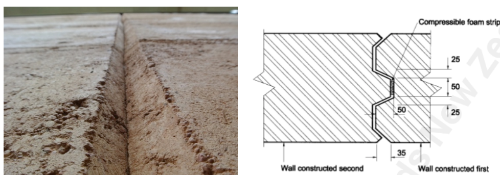
Figura 18: Detalhe de junta de controle e articulação entre paredes adjacentes
