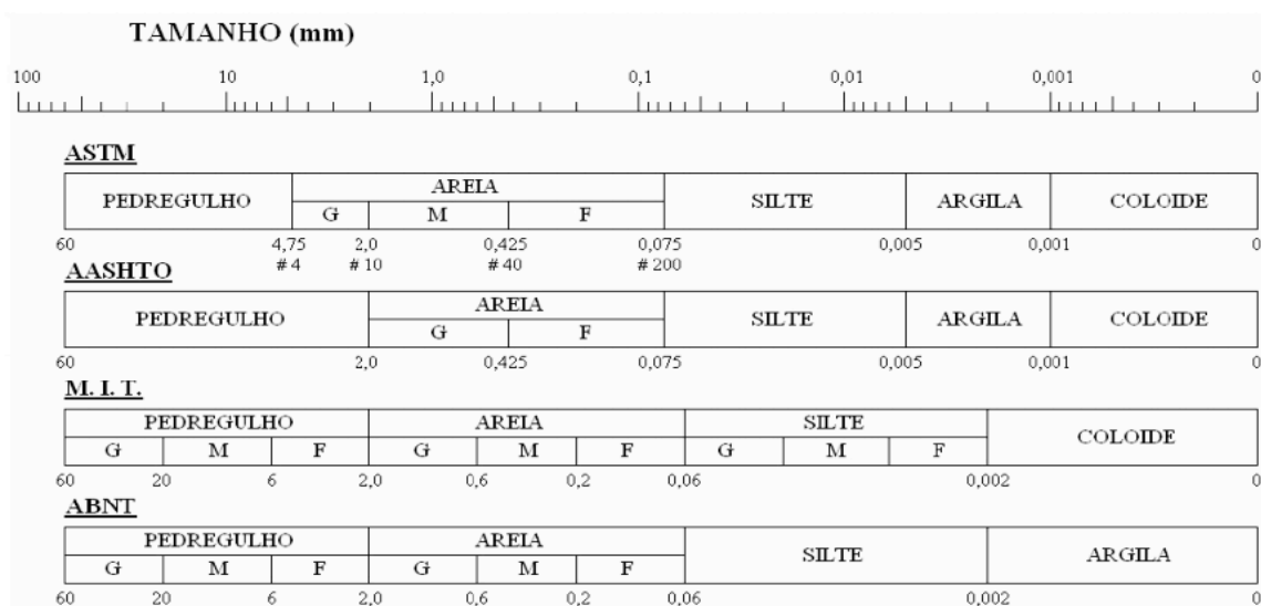
Figura 21: Escalas granulométricas adotadas pela A.S.T.M., A.A.S.H.T.O, M.I.T e ABNT
