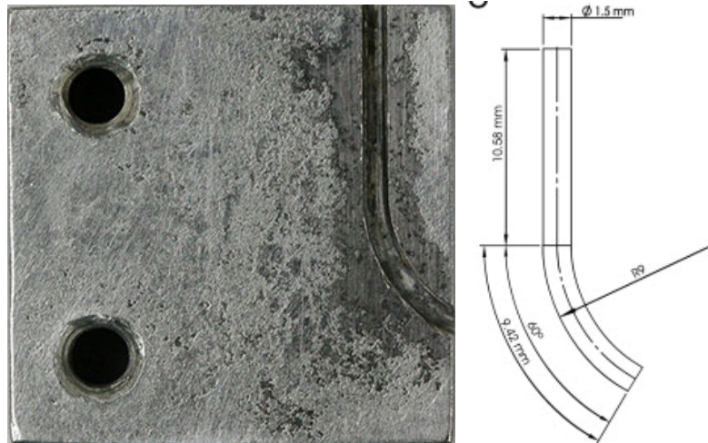
FIGURA 6 – Canal Simulado Raio 9mm, Arco 9,42mm
