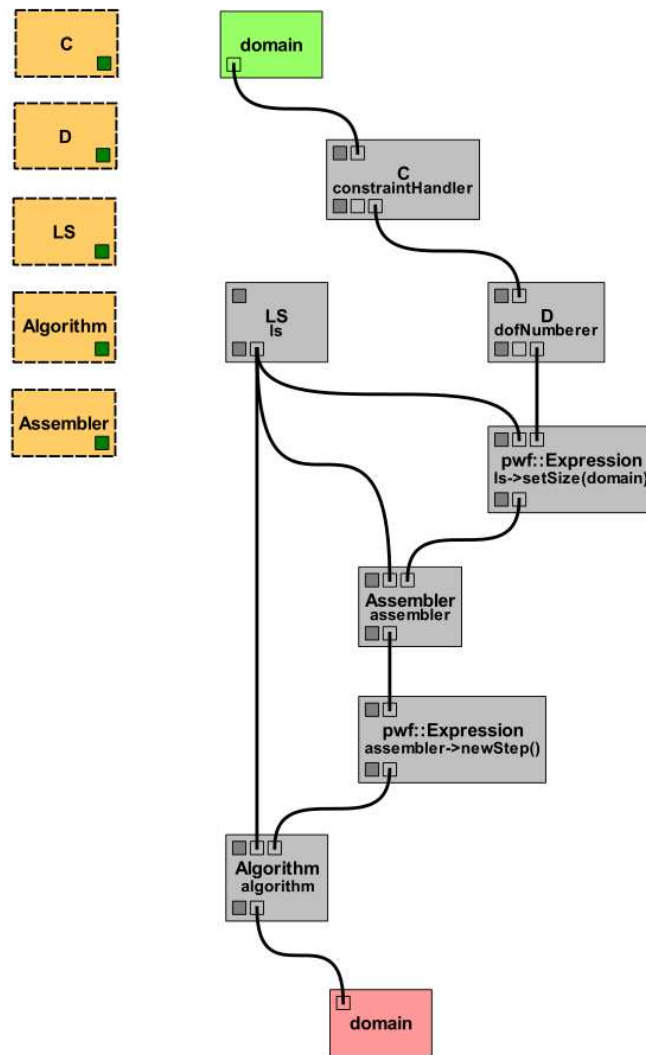
Figura 5.7: Atividade do tipo FemStaticAnalysis .
