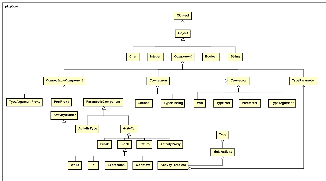
Figura 4.15: Diagrama de classes do modelo proposto.
