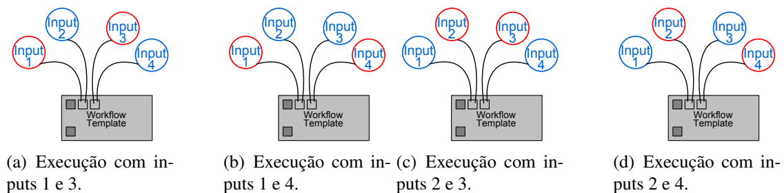
Figura 2.4: Produto cartesiano entre entradas de dados.
