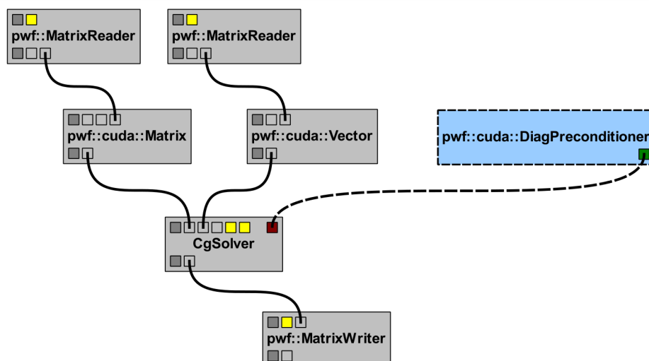
Figura 5.5: Instanciação de CGSolver para GPU.
