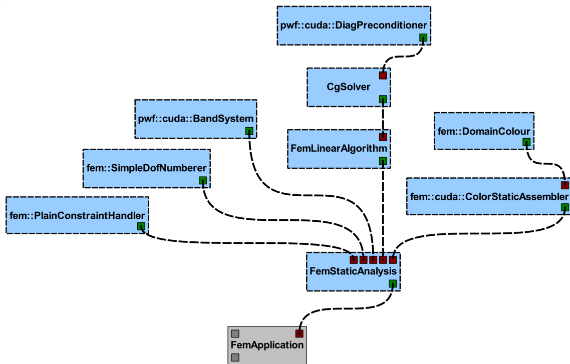
Figura 5.11: FEMMain para GPU.
