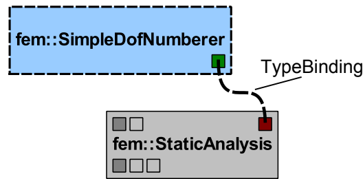
Figura 4.13: Instanciação de atividade paramétrica.
