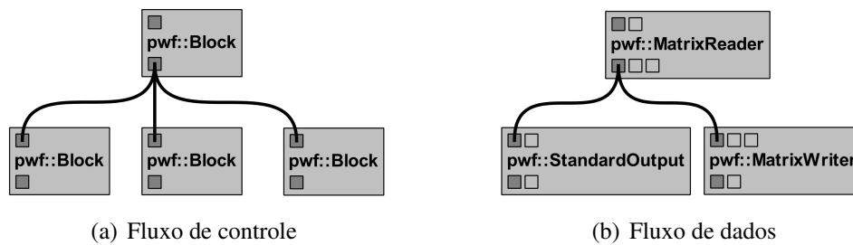
Figura 4.7: Paralelismo entre atividades.
