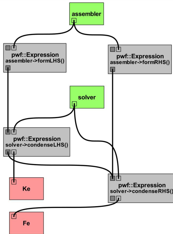
Figura 5.14: Bloco de FemSubdomainAnalysis que computa as contribuições do subdomínio.
