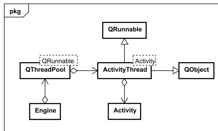
Figura 4.27: Diagrama de classes do motor de execução.
