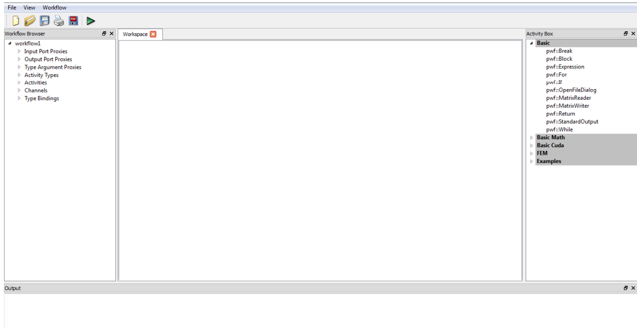
Figura 4.18: Interface Gráfica.
