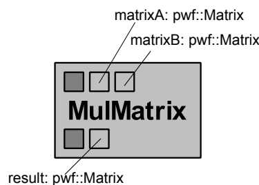
Figura 4.5: Atividade MulMatrix .
