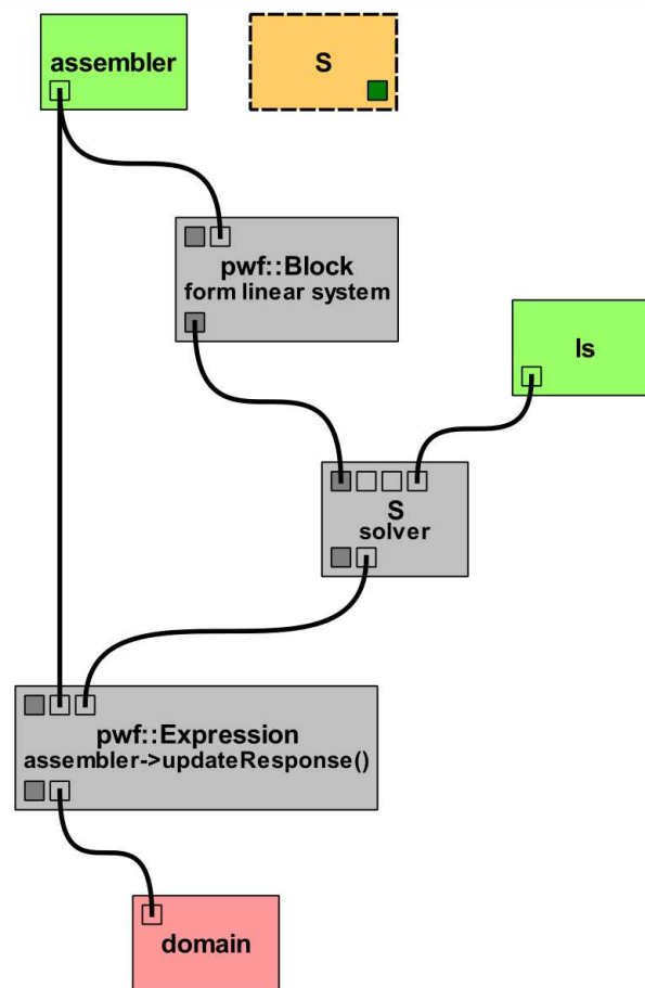
Figura 5.8: Atividade FemLinearAlgorithm.
