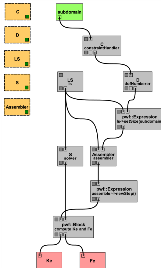
Figura 5.13: Atividade FemSubdomainAnalysis .
