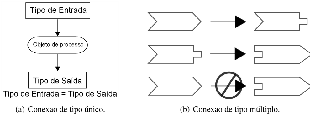
Figura 2.1: Compatibilidade de tipos para a realização de conexões.
