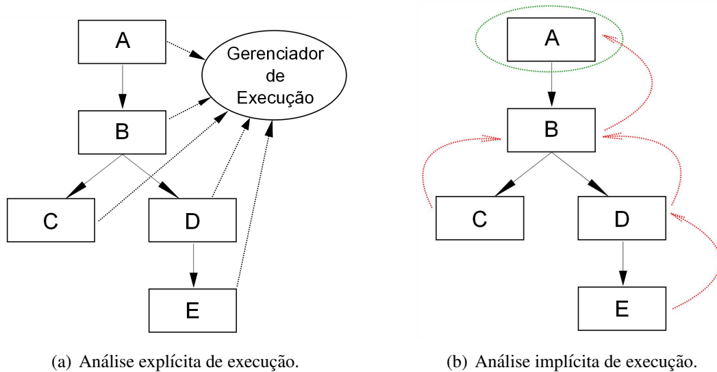
Figura 2.3: Abordagens para análise de execução de workflows.
