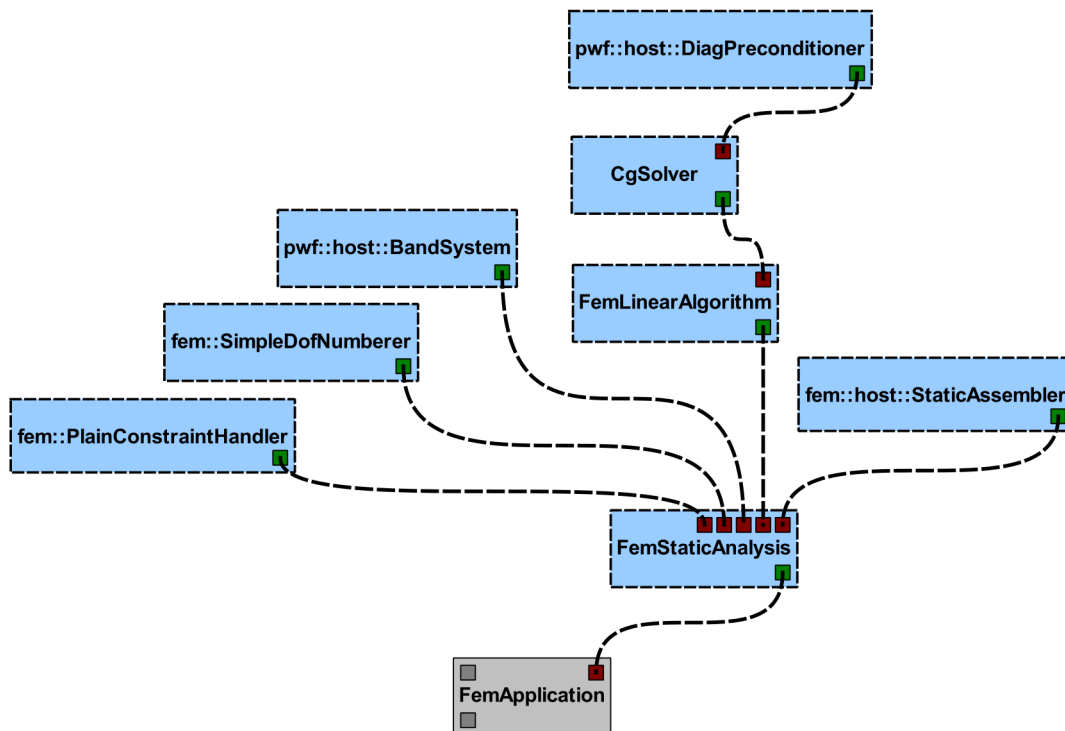
Figura 5.10: FEMMain para CPU.
