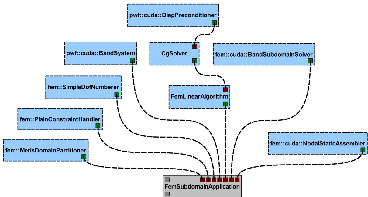
Figura 5.15: Análise com decomposição de domínio em GPU.
