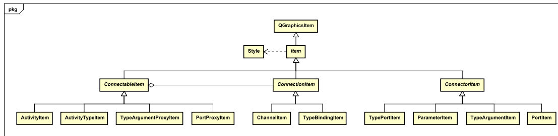
Figura 4.19: Diagrama de classes dos itens gráficos.
