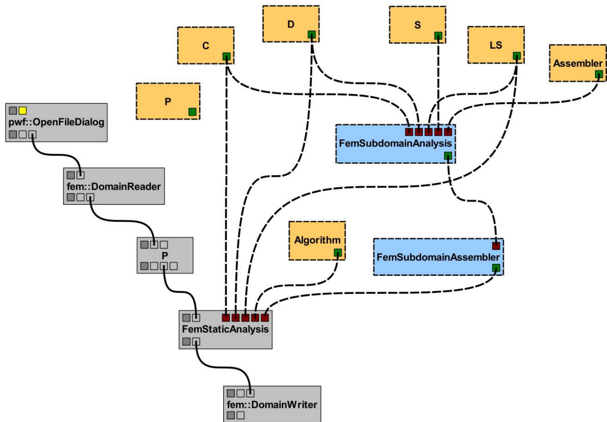
Figura 5.12: Aplicação do MEF para subdomínios.
