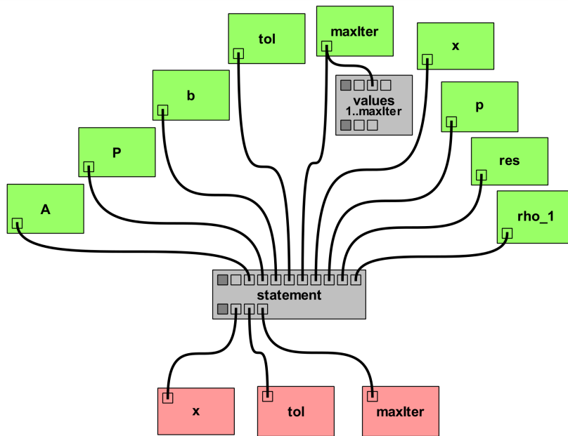
Figura 5.2: Atividade For 1..maxIter.
