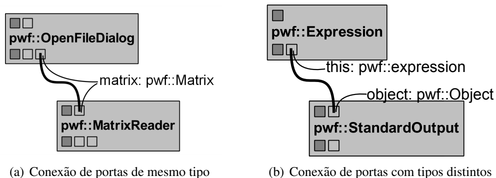
Figura 4.6: Conexões entre portas de tipos de dados compatíveis.
