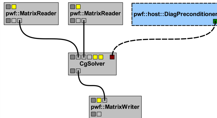
Figura 5.4: Instanciação de CGSolver para CPU.
