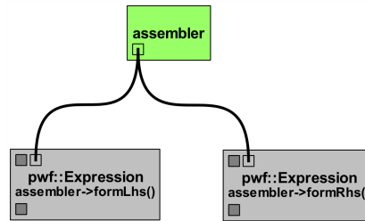
Figura 5.9: Bloco de formação do sistema na atividade FemLinearAlgorithm .
