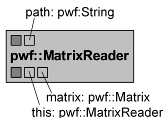
Figura 4.3: Atividade MatrixReader .
