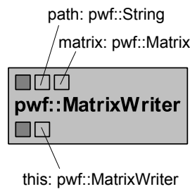
Figura 4.4: Atividade MatrixWriter .
