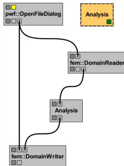
Figura 5.6: Atividade FEMMain .
