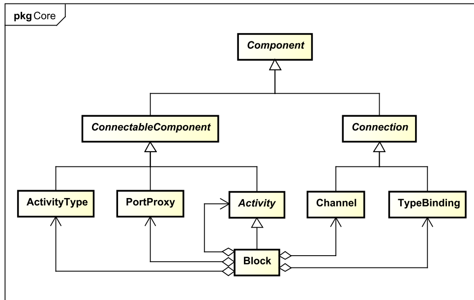
Figura 4.16: Composição de um bloco.
