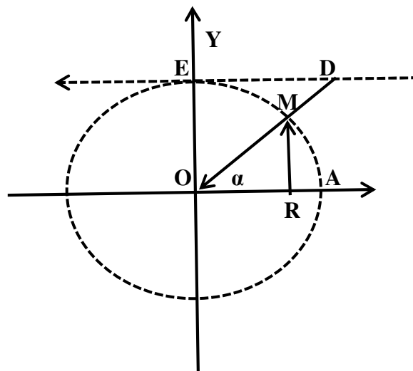
Figura 25: Cossecante
