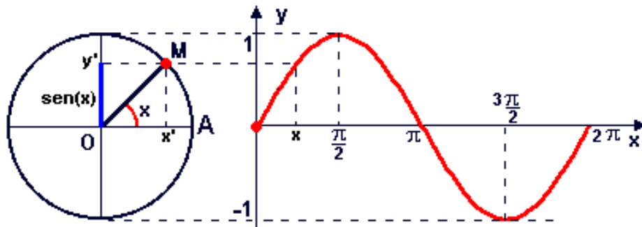
Figura 30: Gráfico Função Seno
