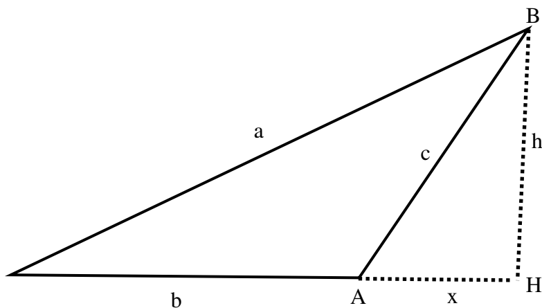
Figura 23: Lei dos Cossenos II
