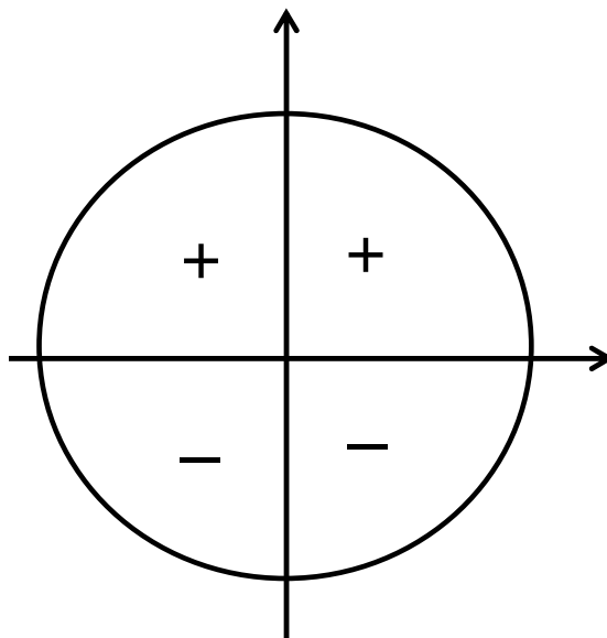
Figura 16: Sinais do Seno
