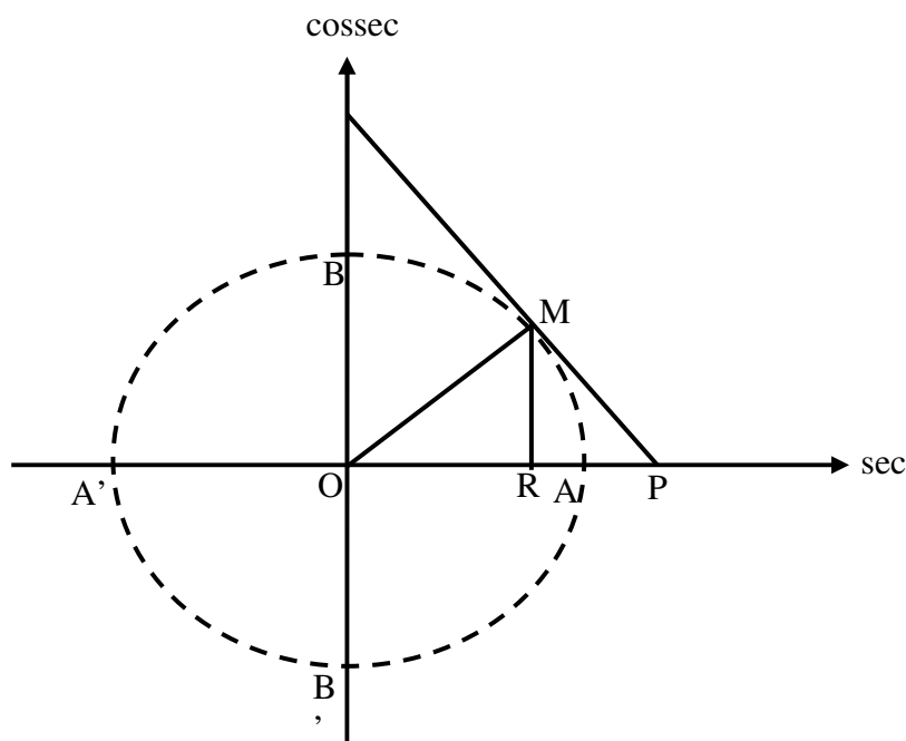
Figura 24: Secante
