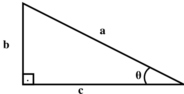
Figura 9: Triângulo Retângulo I
