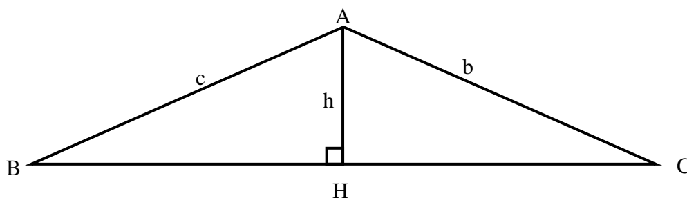
Figura 21: Lei dos Senos
