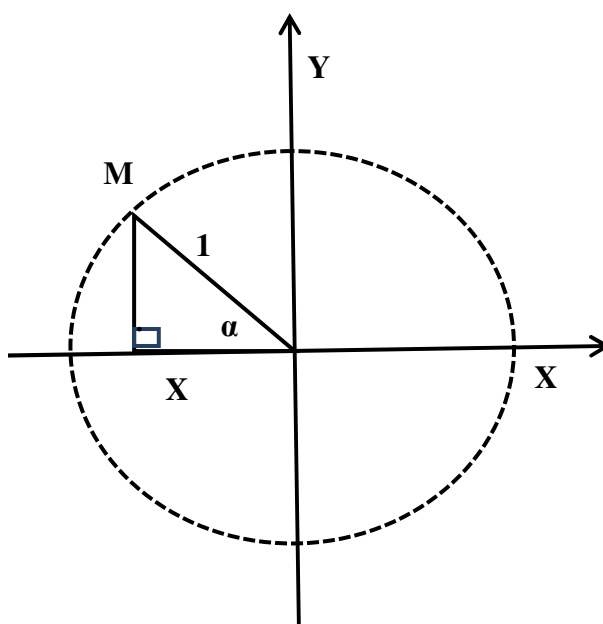
Figura 17: Eixo Cosseno
