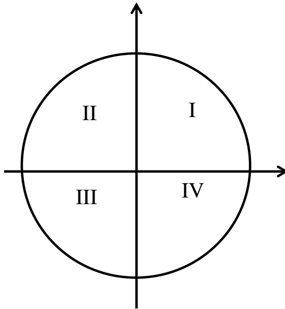
Figura 13: Ciclo trigonométrico I
