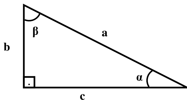
Figura 10: Triângulo Retângulo II
