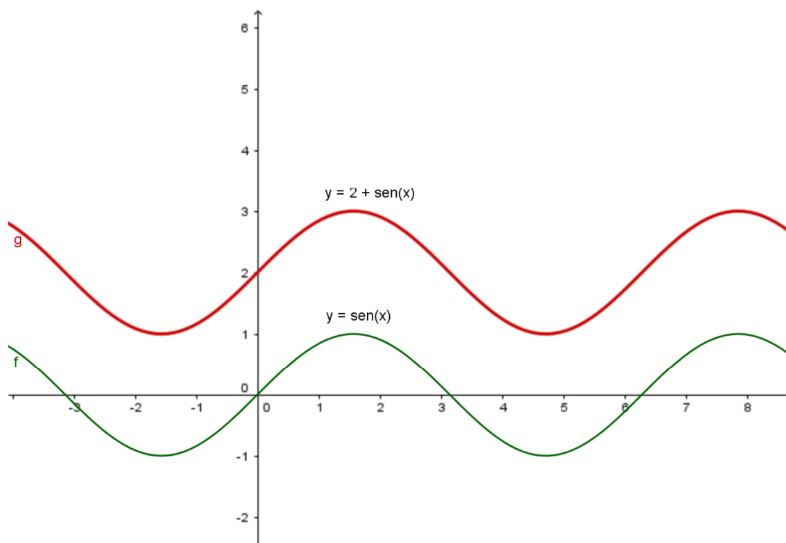
Figura 3: Gráfico de y = 2 + \text{sen}x
