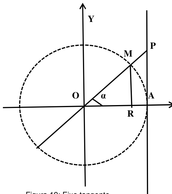
Figura 19: Eixo tangente
