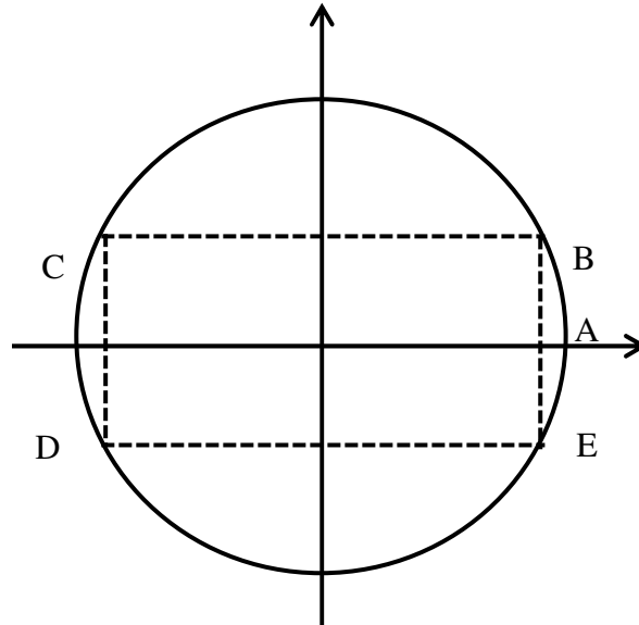
Figura 14: Ângulo Correspondentes
