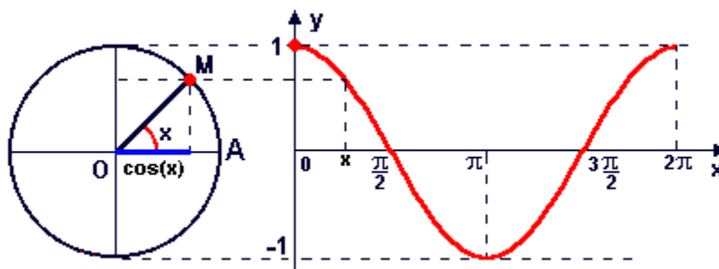
Figura 32: Gráfico Função Cosseno
