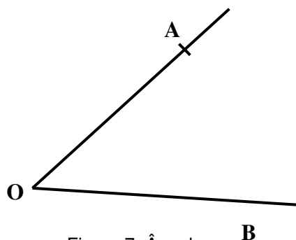
Figura 7: Ângulo
