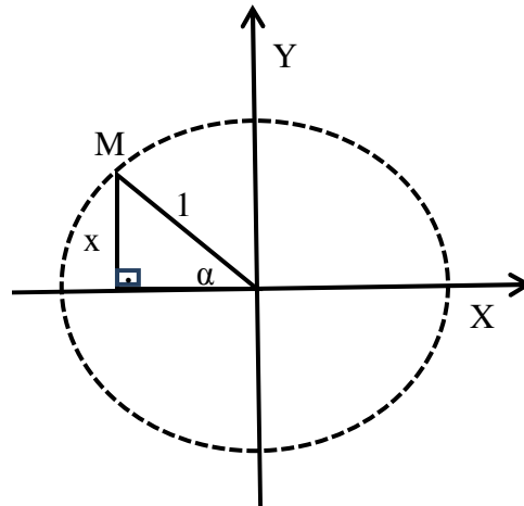
Figura 15: Eixo seno
