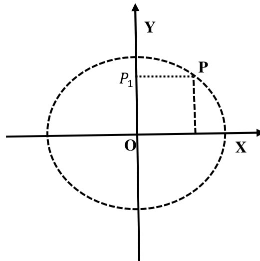
Figura 29: Função Seno I
