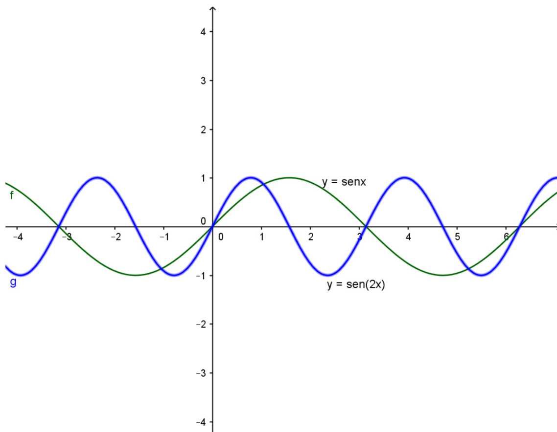
Figura 5: gráfico de y = \text{sen}(2x)
