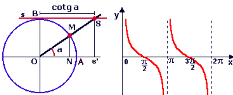
Figura 37: Gráfico da Função Cotangente
