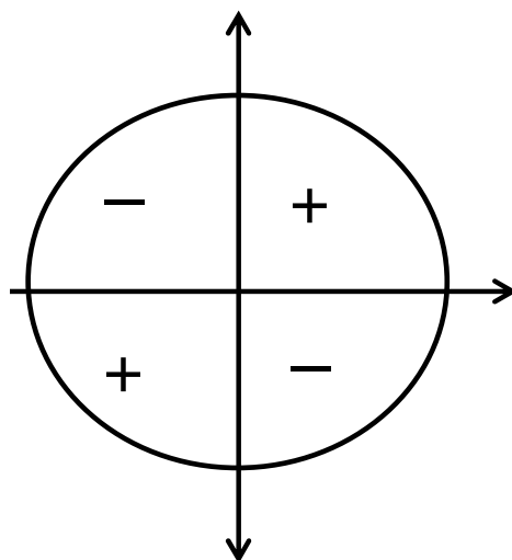
Figura 20: Sinais da Tangente
