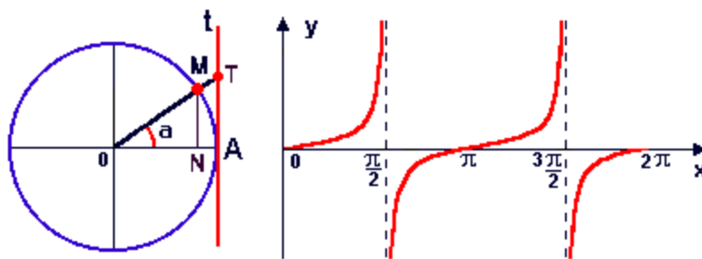
Figura 34: Gráfico Função Tangente
