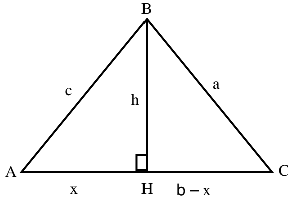
Figura 22: Lei dos Cossenos I
