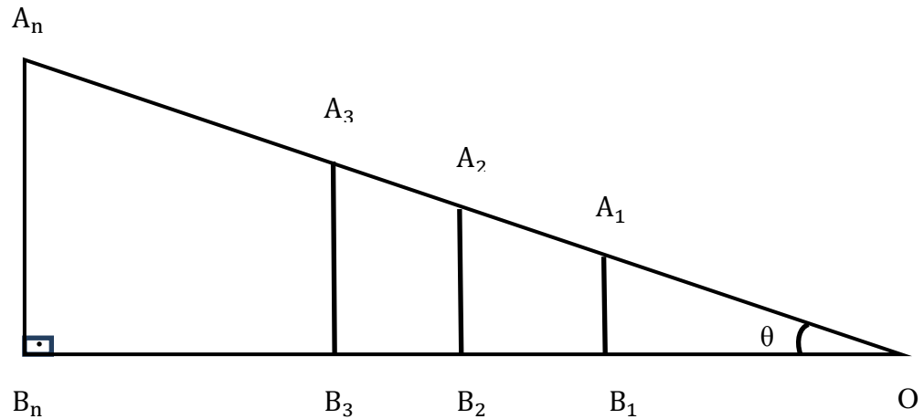
Figura 8: Triângulos Semelhantes
