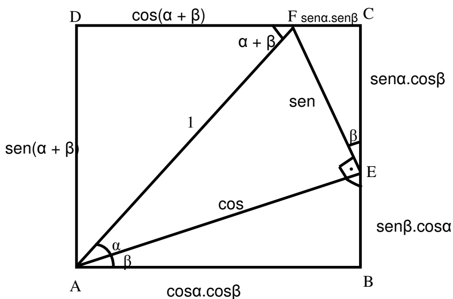
Figura 28: Arco Soma II
