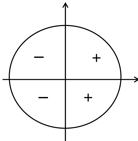
Figura 18: Sinais do cosseno
