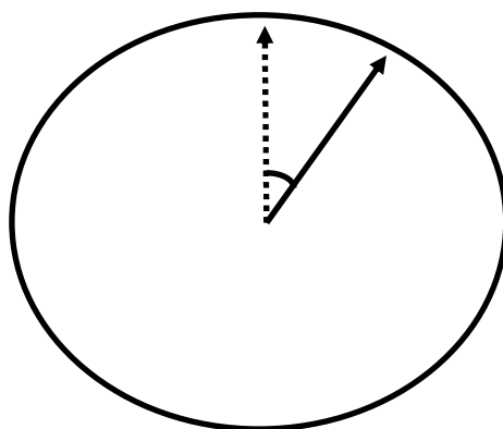
Figura 42: Relógio
