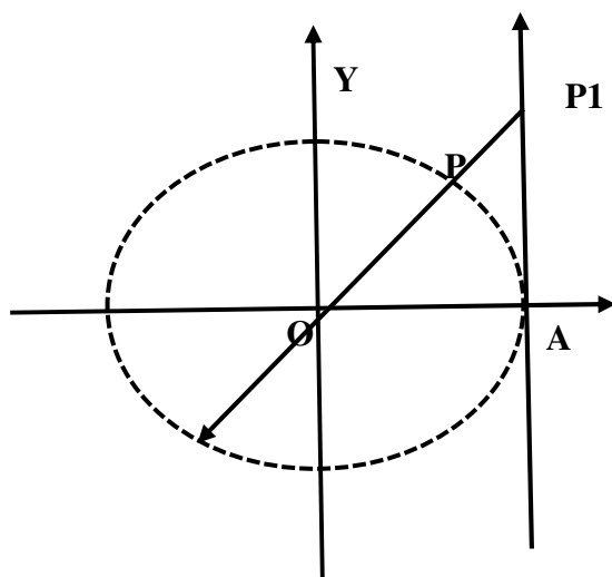
Figura 33: Função Tangente I
