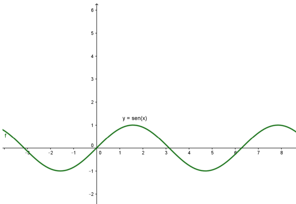
Figura 2: gráfico de \text{sen}x
