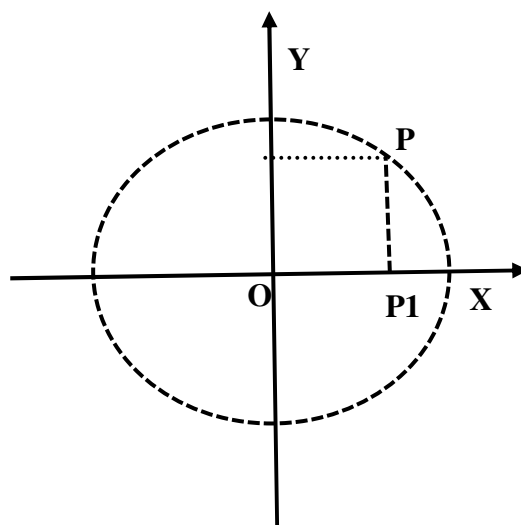
Figura 31: Função Cosseno I
