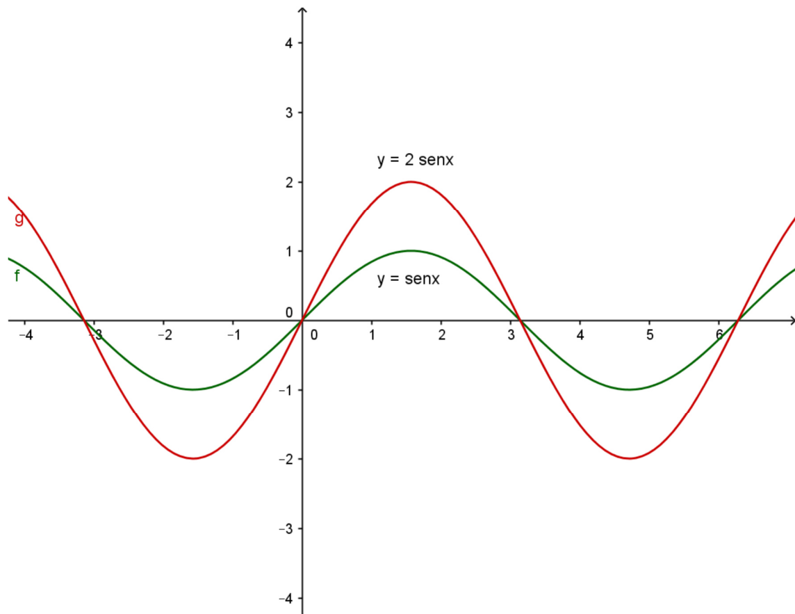
Figura 4: gráfico de y = 2\text{sen}x
