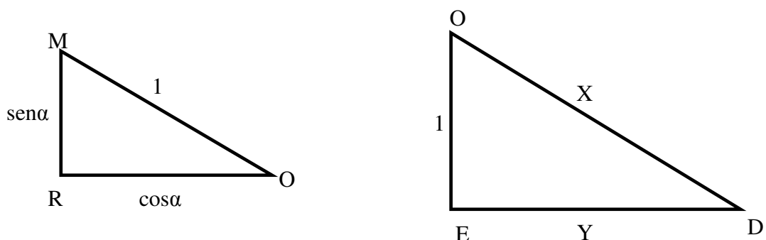
Figura 26: Cossecante I
