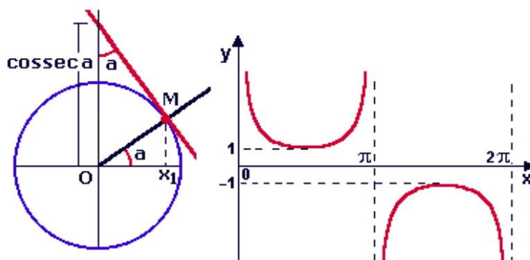
Figura 36: Gráfico da Função Cossecante
