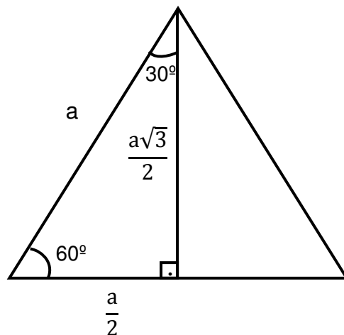
Figura 12: Triângulo Equilátero
