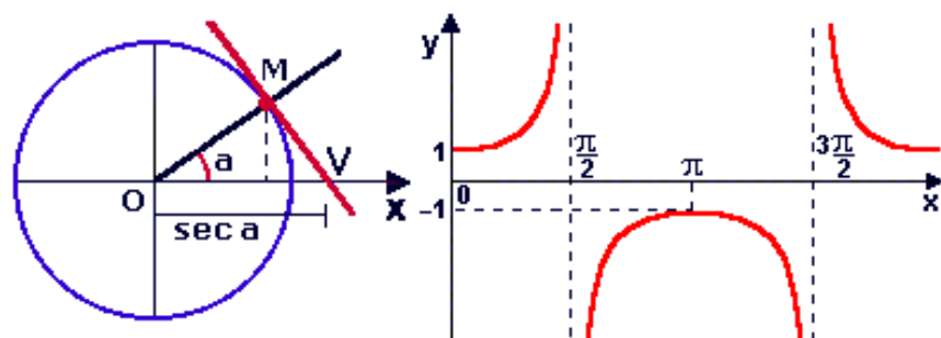
Figura 35: Função Secante
