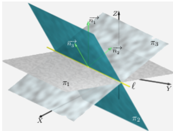
Figura 2.6.11: Os três planos são distintos e se intersectam segundo uma reta \ell
