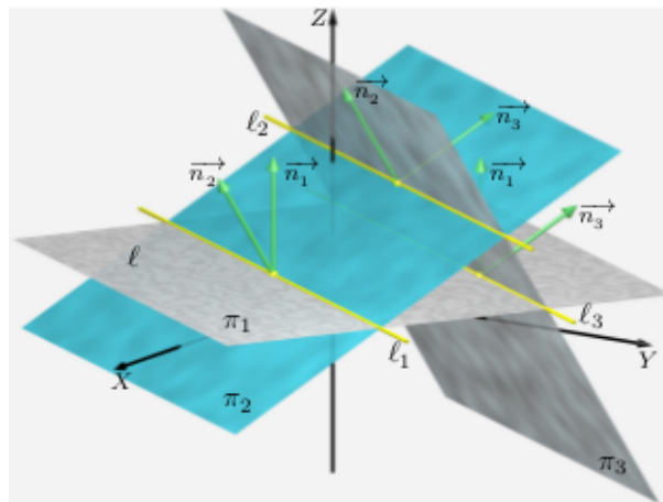
Figura 2.6.12: Os três planos se intersectam, dois a dois, segundo retas \ell_1 , \ell_2 , \ell_3
