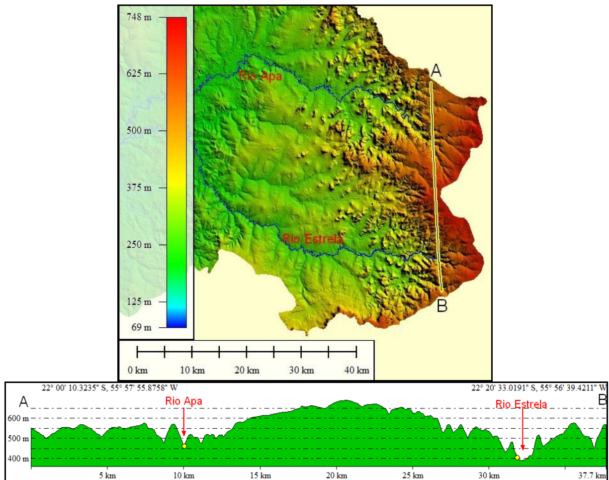
Figura 9. Perfil transversal (corte A – B) próximo as nascentes do rio Apa e rio Estrela.
