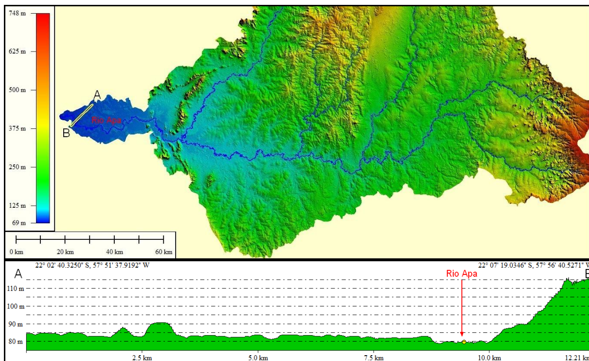
Figura 11. Perfil transversal (corte A – B) no baixo curso da bacia do rio Apa.
