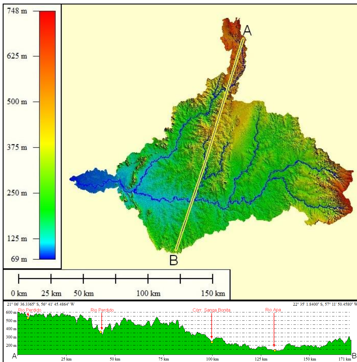
Figura 10. Perfil transversal (corte A – B) no médio curso da bacia do rio Apa.
