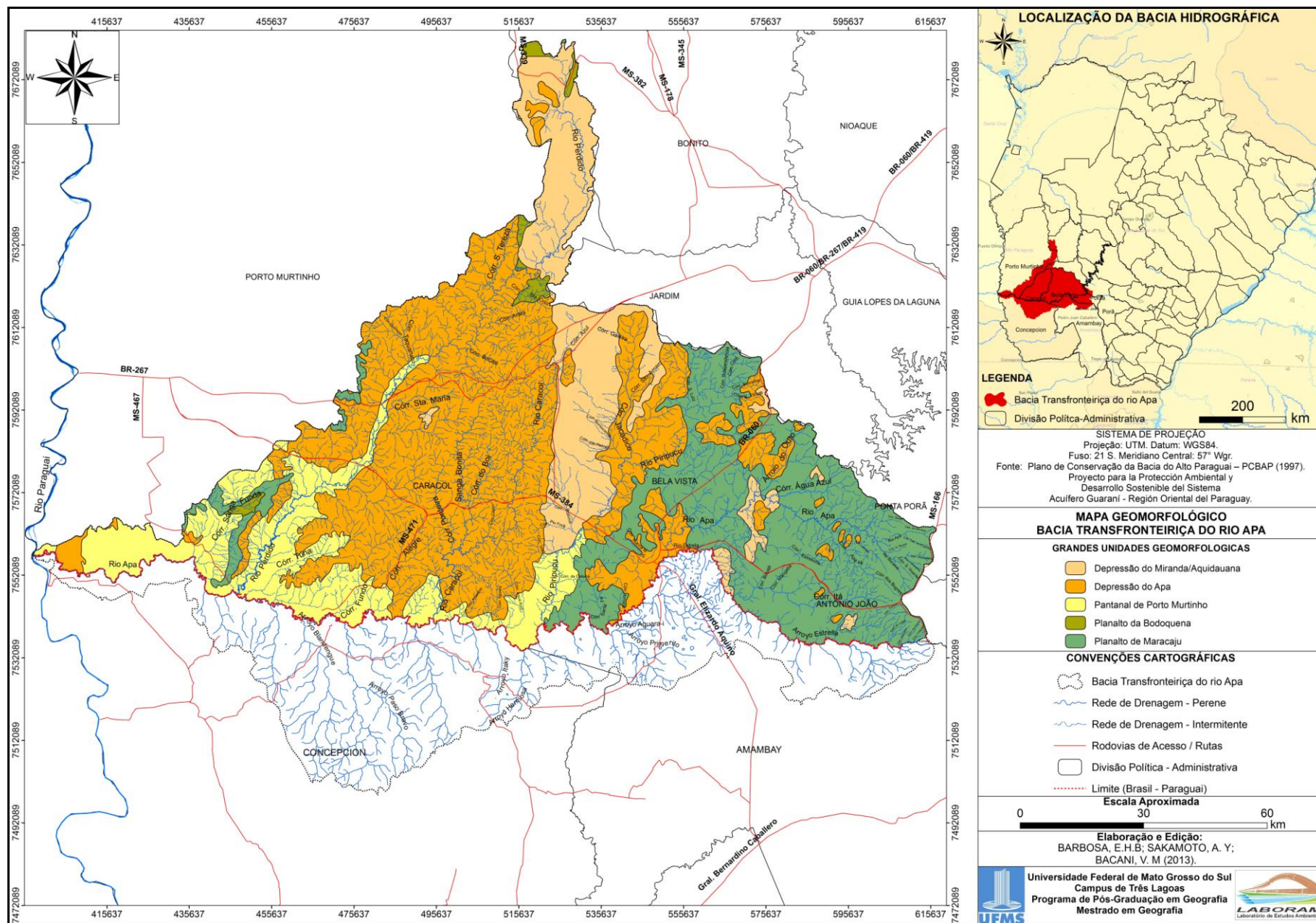
Figura 3. Mapa Geomorfológico, do lado brasileiro, da bacia transfronteiriça do rio Apa.
