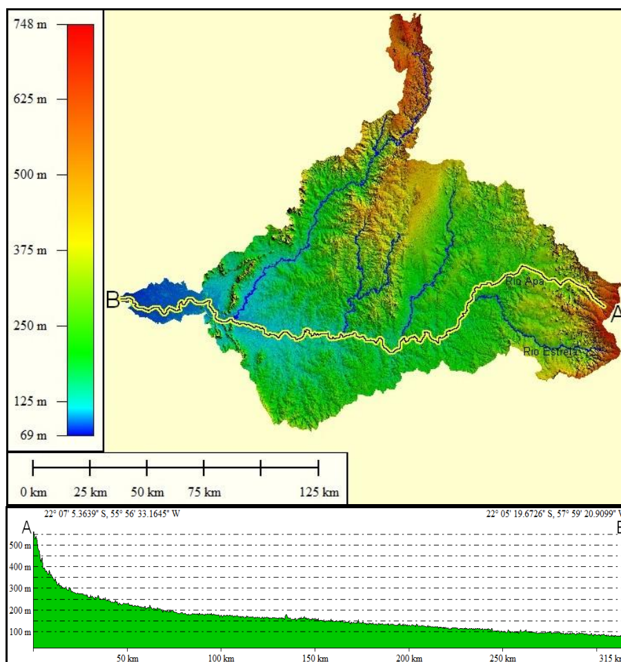
Figura 8. Perfil longitudinal (corte A – B) do rio Apa.
