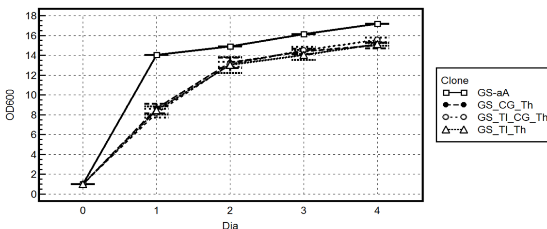
Figura 7. Crescimento médio ( OD_{600\text{ nm}} \pm desvio padrão) das 5 colônias de cada plasmídeo transformado, mostrando um desvio padrão muito baixo, o que significa que não houve diferença entre as recombinantes, a um nível de 99,9% de significância. GS-aA, GS_CG_Th, GS_TI_CG_Th e GS_TI_Th são os clones transformados com os plasmídeos pPICZalphaA, pPIC \alpha CG-Th, pPIC \alpha TI-CG-Th e pPIC \alpha TI-Th, respectivamente.
