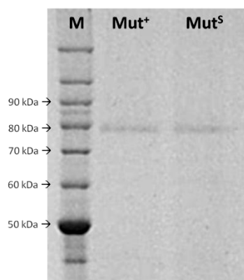
Figura 2. Expressão de rBm86-CG por P. pastoris . SDS-PAGE 7,5% da fração obtida pelo processo de cromatografia em coluna de níquel do sobrenadante da cultura dos clones Mut + e Mut S . M: Marcador BenchMark TM Loadler Protein que varia em peso molecular de 10-220 kDa. Mut + e Mut S : 10 \mu g por poço de rBm86-CG expressa pelos clones Mut + e Mut S .
