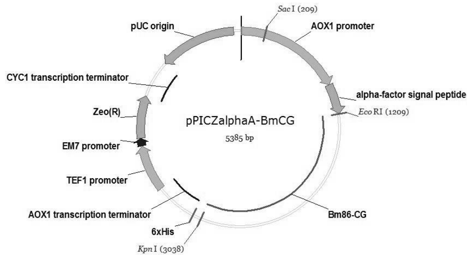
Figura 1. Mapa do plasmídeo pPICZ \alpha A-BmCG utilizado para transformar P. pastoris . O mapa foi criado no software Vector NTI 8; AOX1 promoter: promotor fortemente induzida por metanol; SacI: enzima utilizada para linearizar o plasmídeo antes da transformação em P. pastoris ; alpha-factor: sequência correspondente do peptídeo secretor de rBm86-CG; EcoRI: sítio de restrição utilizado para a clonagem na região 5'; Bm86-CG: gene parcial da Bm86-GC inserido no plasmídeo; KpnI: sítio de restrição utilizado para a clonagem na região 3'; AOX1 transcription terminator: sequência que determina o fim da transcrição; Zeo(R): gene de resistência à zeocina TM , permitindo a seleção de P. pastoris transformantes; pUC origin: origem de replicação de E. coli .
