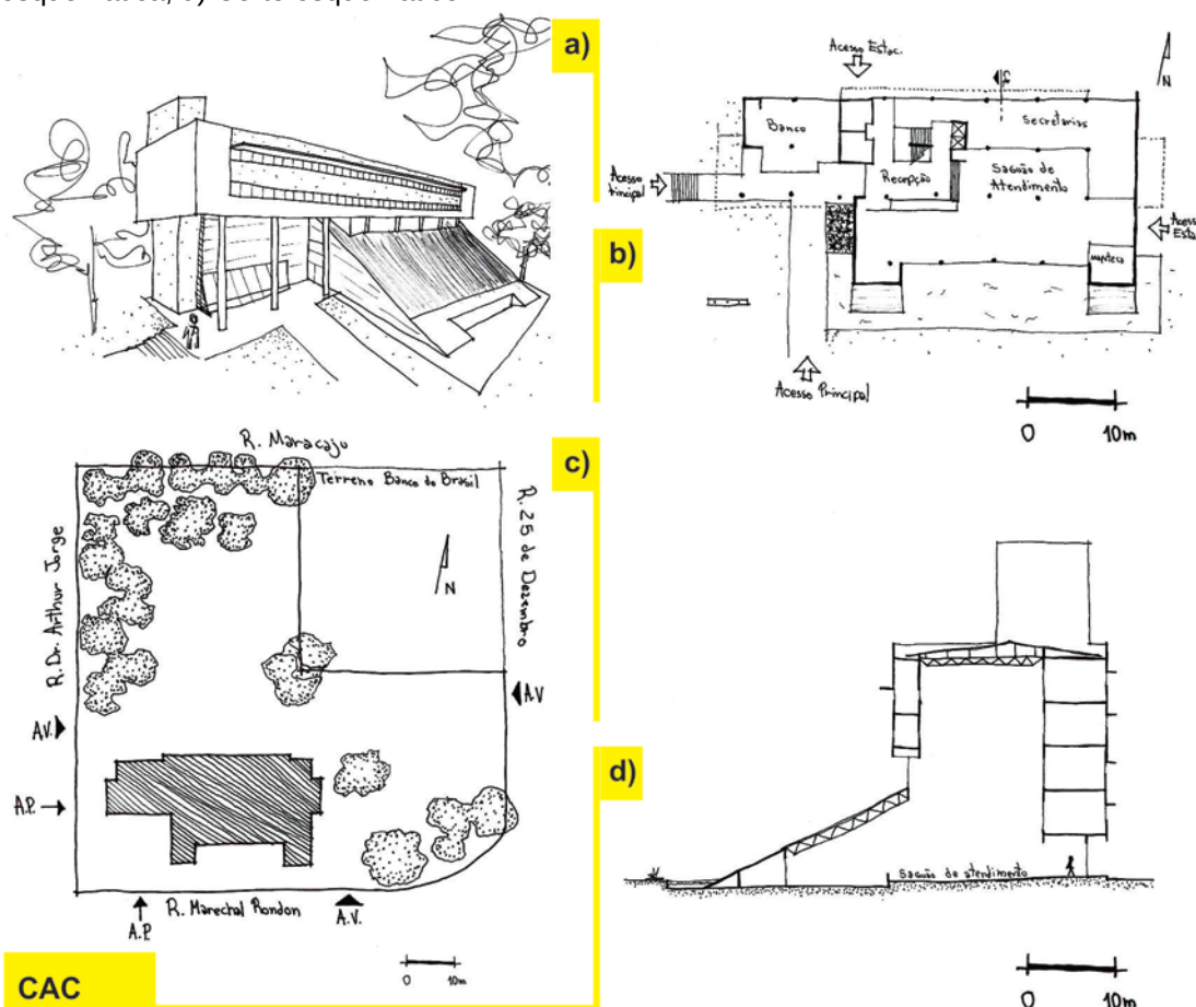
FIGURA 05 – Croquis da CAC: a) Vista geral; b) Planta esquemática; c) Implantação esquemática; d) Corte esquemático.
