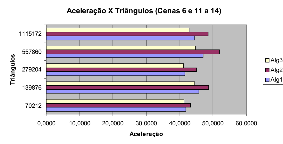
Figura 4.7: Traçado de raios: aceleração × número de triângulos (cenas 6 e 11 a 14).
