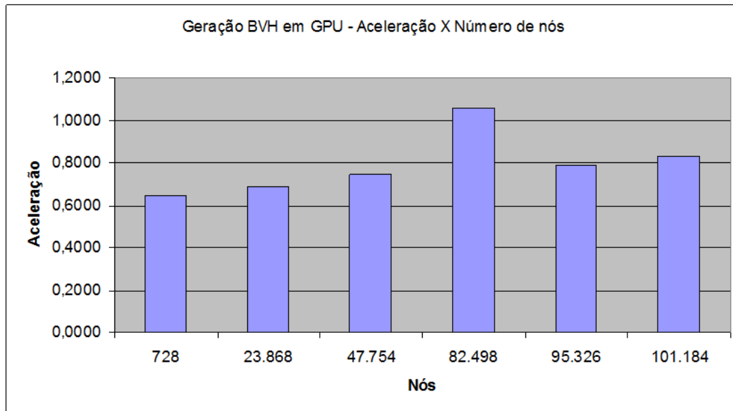
Figura 4.11: Geração BVH em GPU - Aceleração X número de nós.
