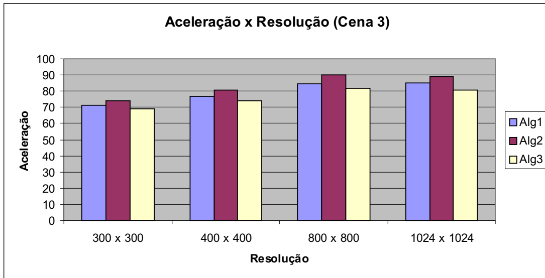
Figura 4.4: Traçado de raios primários: aceleração \times resolução das imagens (cena 3).
