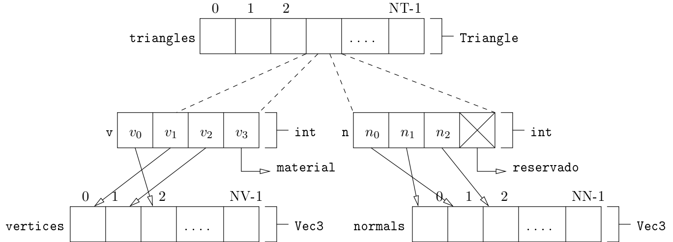
Figura 2.27: Estrutura de dados para malha de triângulos.
