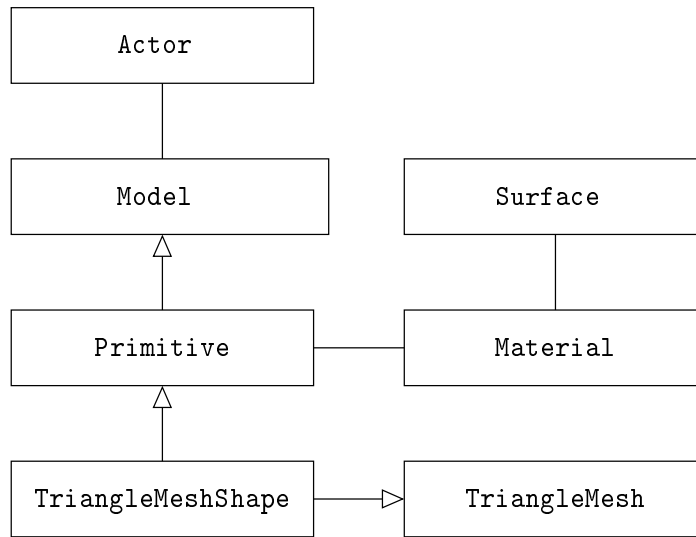
Figura 2.23: Diagrama da classe Actor.
