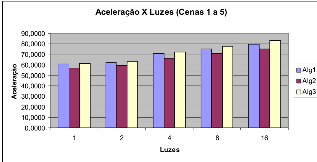
Figura 4.6: Traçado de raios: aceleração × número de luzes.
