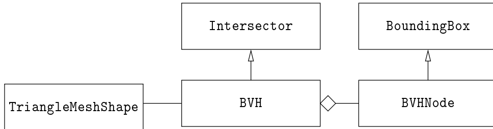
Figura 2.25: Diagrama da classe BVH.
