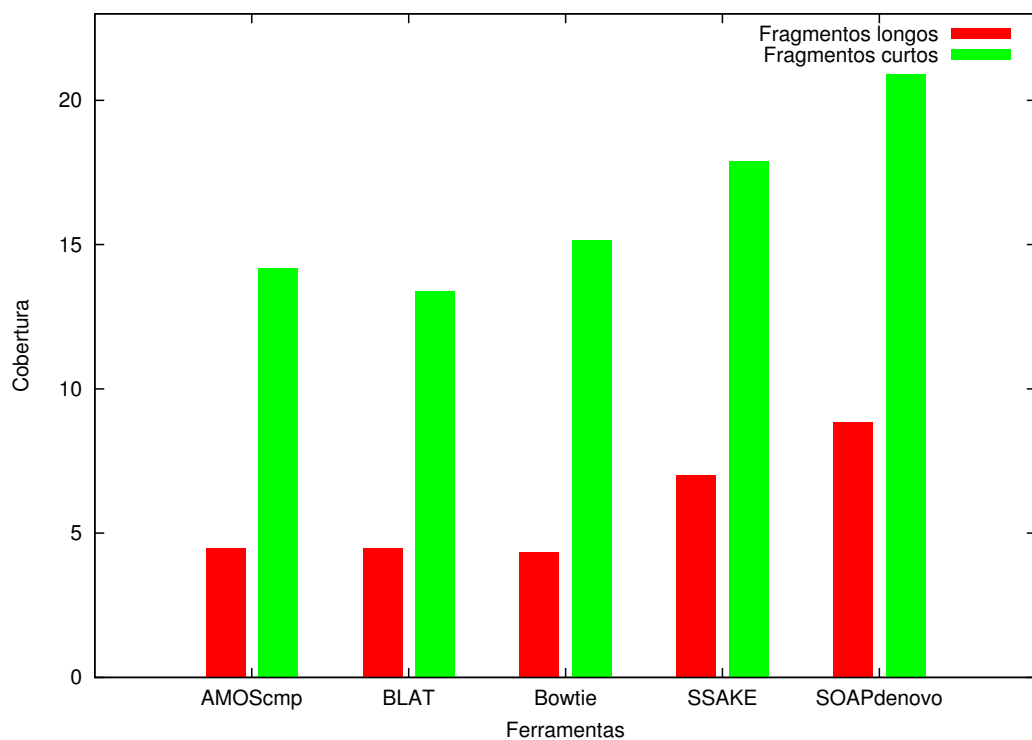
Figura 5.17: Média de coberturas dos contigs gerados para os fragmentos longos e curtos.
