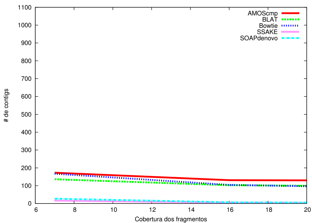
Figura 5.3: Variação na maior média de número de contigs para fragmentos de tamanho 120.
