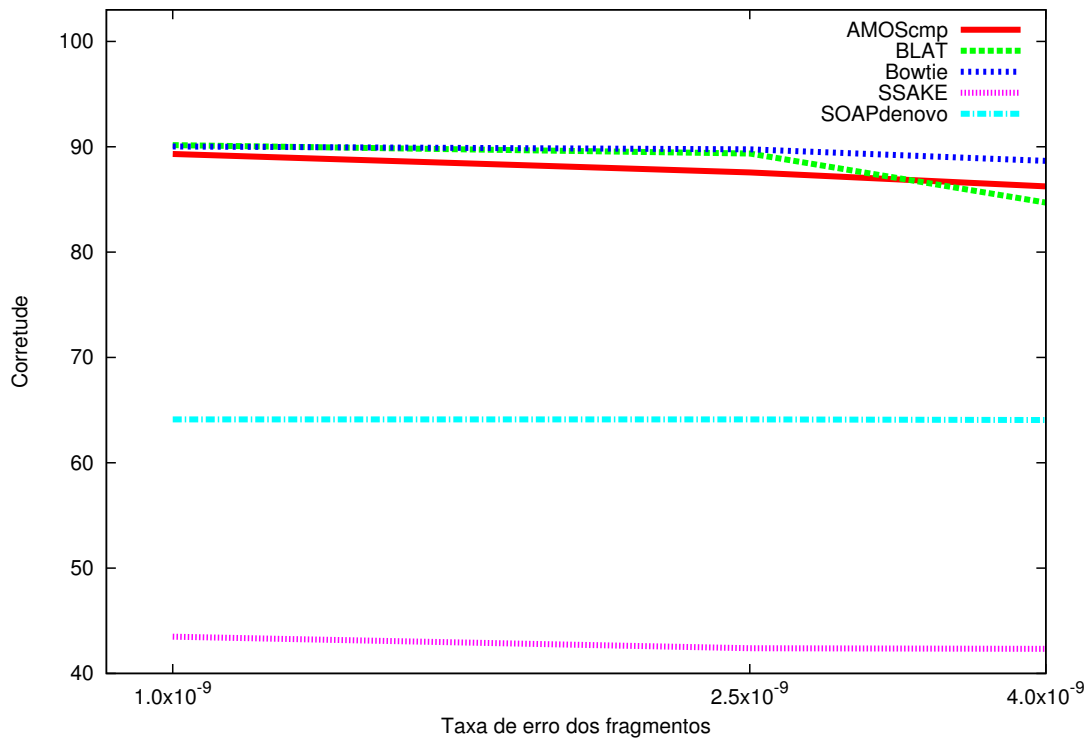
Figura 5.13: Porcentagem de médias de corretudes dos resultados para cobertura 16 e tamanho 50 dos fragmentos.
