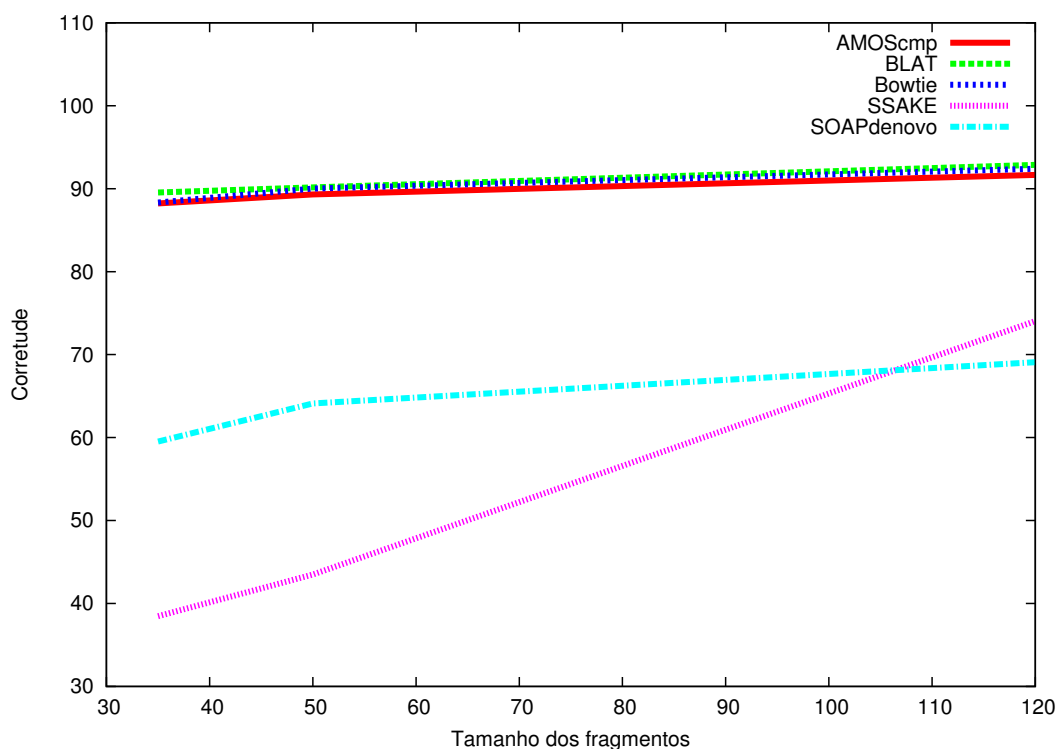
Figura 5.14: Porcentagens máximas de médias de corretudes dos resultados para cobertura 16.
