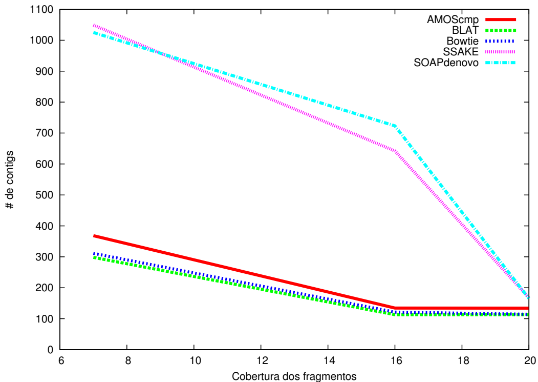
Figura 5.1: Variação na maior média de número de contigs para fragmentos de tamanho 35.
