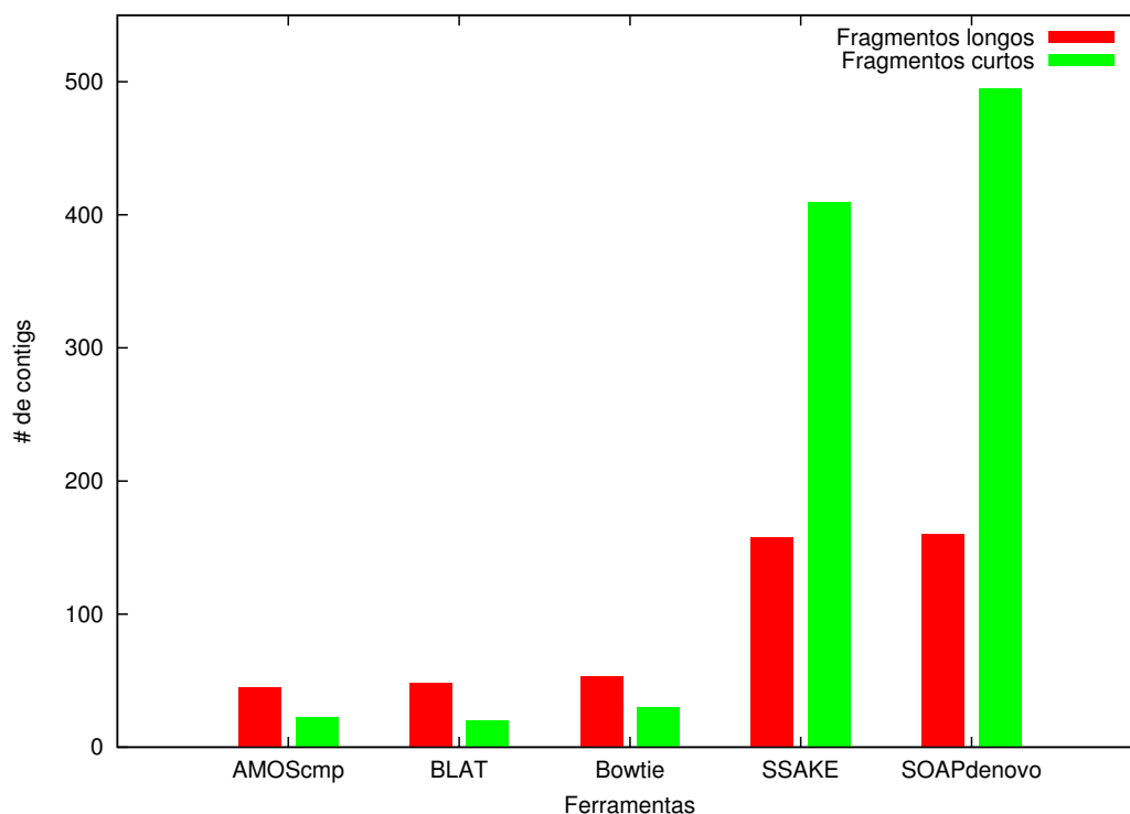
Figura 5.16: Média de contigs gerados para os fragmentos longos e curtos.
