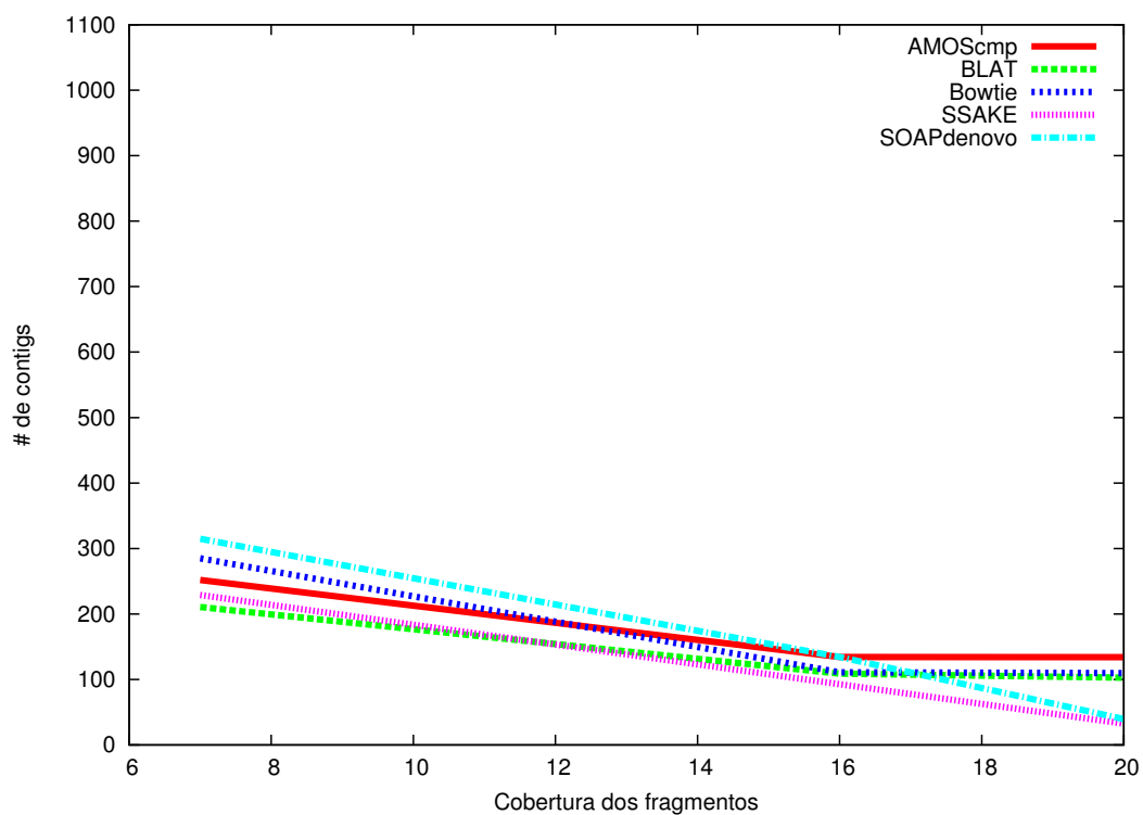
Figura 5.2: Variação na maior média de número de contigs para fragmentos de tamanho 50.
