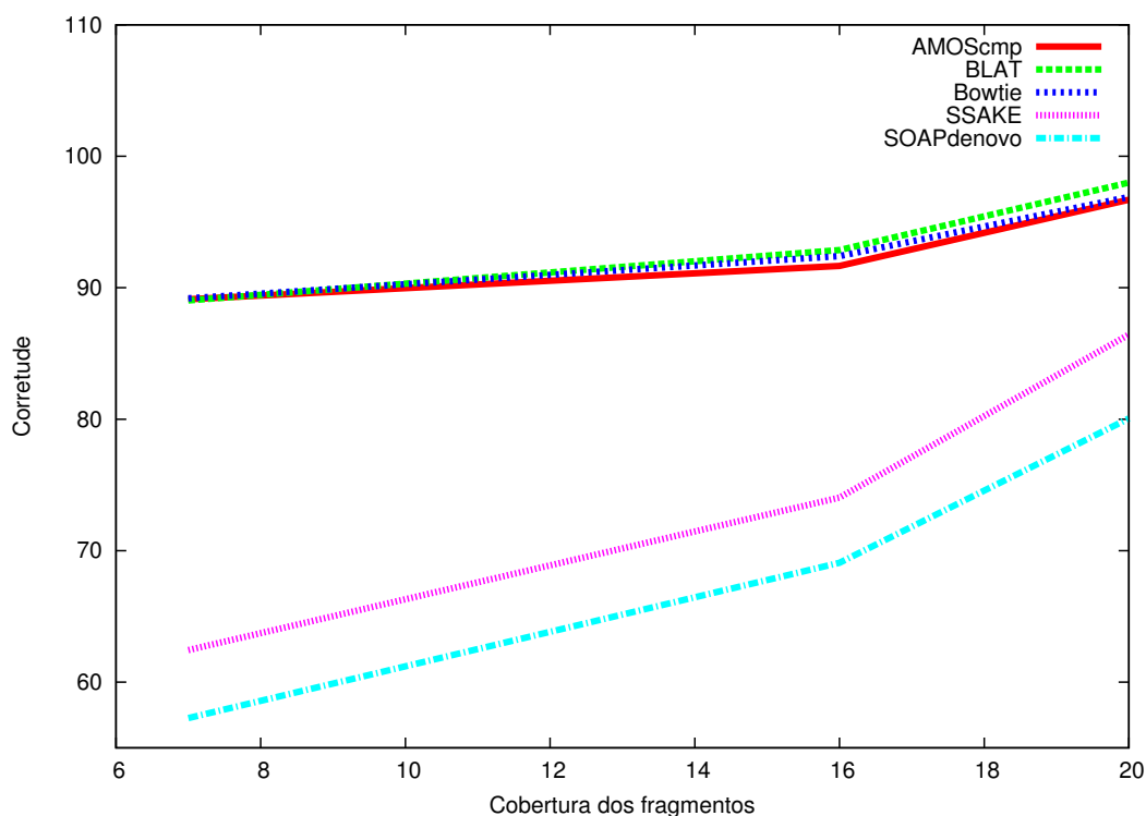
Figura 5.11: Porcentagens máximas de médias de corretudes dos resultados conforme a variação de cobertura dos fragmentos.
