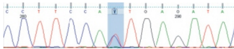
Figura 2.12: Sobreposição de curvas correspondentes a diferentes tipos de nucleotídeo no cromatograma. A linha azul corresponde ao nucleotídeo C e a linha vermelha corresponde ao nucleotídeo T. A área destacada no cromatograma mostra a sobreposição de picos impossibilitando a determinação do nucleotídeo sequenciado naquele ponto. Essa incerteza é representada, nesta figura, pelo caractere Y.
