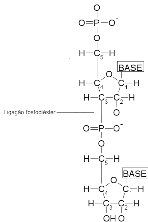
Figura 2.4: Dois nucleotídeos de uma mesma fita são ligados por uma ligação fosfodiéster.
