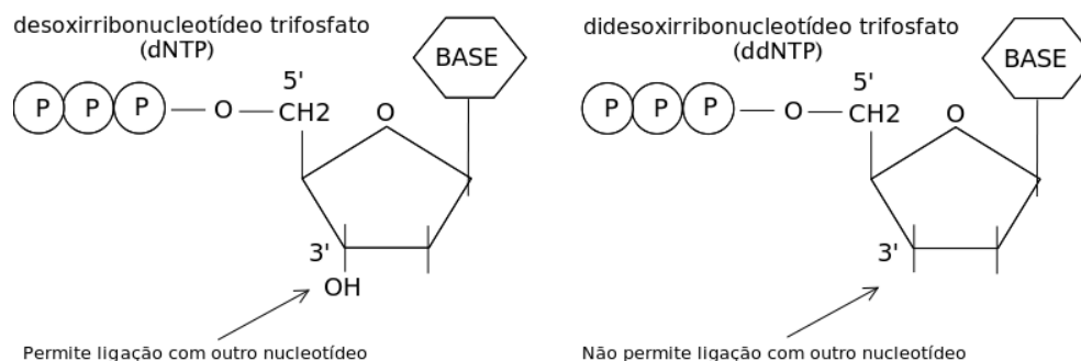
Figura 2.8: Diferença entre um ddNTP e um dNTP.
