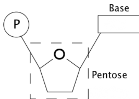
Figura 2.1: Visão geral da estrutura de um nucleotídeo.
