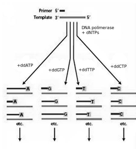
Figura 2.9: Conjunto de cadeias truncadas resultantes do processo de síntese. São realizadas 4 reações de síntese, uma para cada tipo de ddNTP, juntamente com os 4 dNTPs (dATP, dTTP, dCTP, dGTP). A partir do momento que a DNA polimerase insere um ddNTP, a síntese não é mais possível. Dessa forma, o conjunto de cadeias truncadas resultantes das 4 reações é formado por fragmentos que foram truncados em posições e tipos de nucleotídeos aleatórios em relação à cadeia original.
