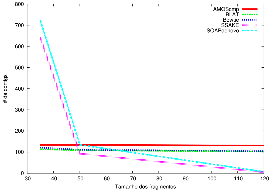
Figura 5.5: Variação na maior média de número de contigs para fragmentos de Cobertura 16.
