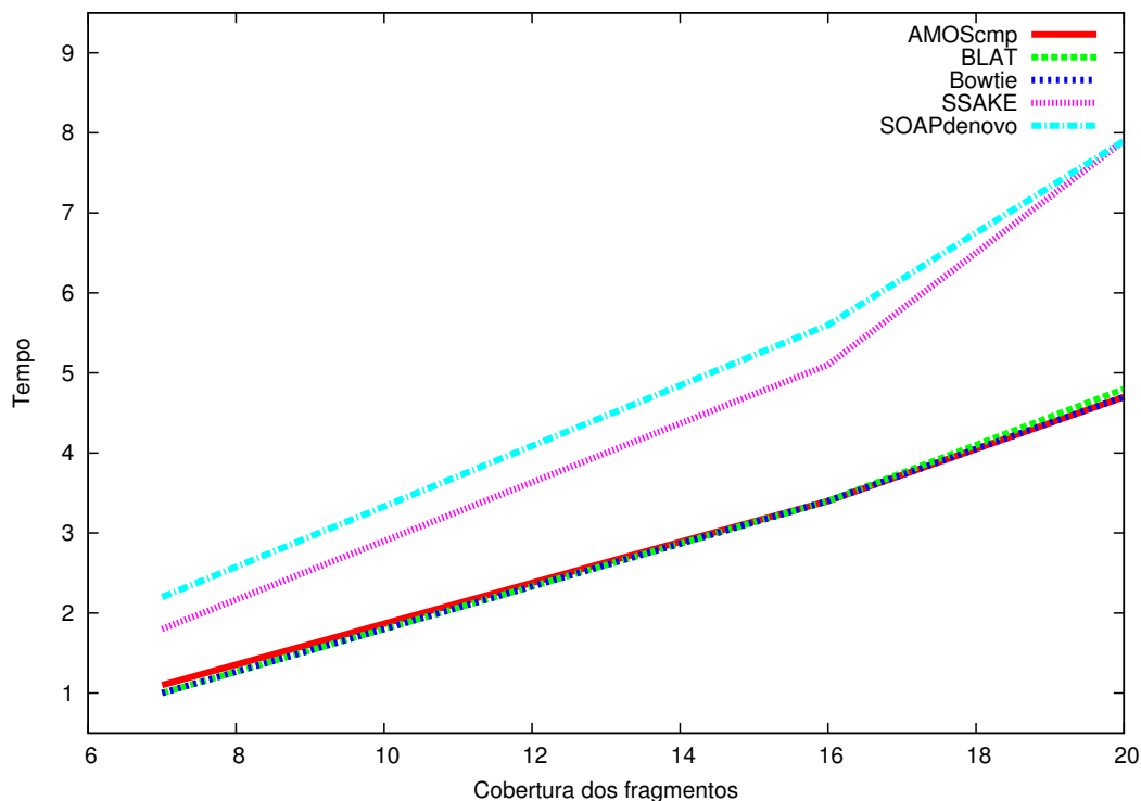
Figura 5.15: Variação em minutos no tempo de execução das ferramentas conforme valores das coberturas dos fragmentos.
