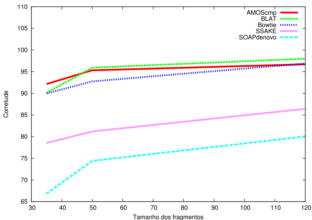
Figura 5.12: Porcentagens máximas de médias de corretudes dos resultados para cobertura 20.
