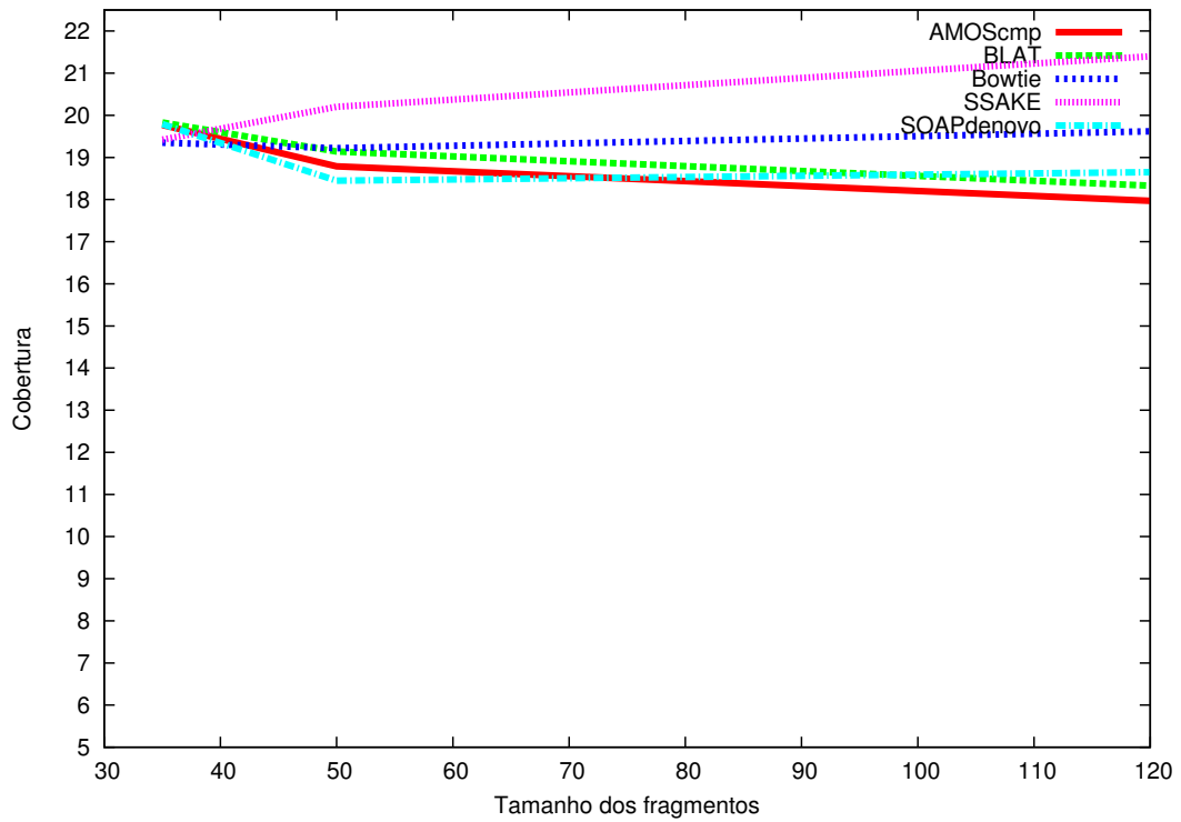
Figura 5.9: Variação na média de coberturas dos resultados de remontagem para fragmentos de cobertura-genfrag 20.
