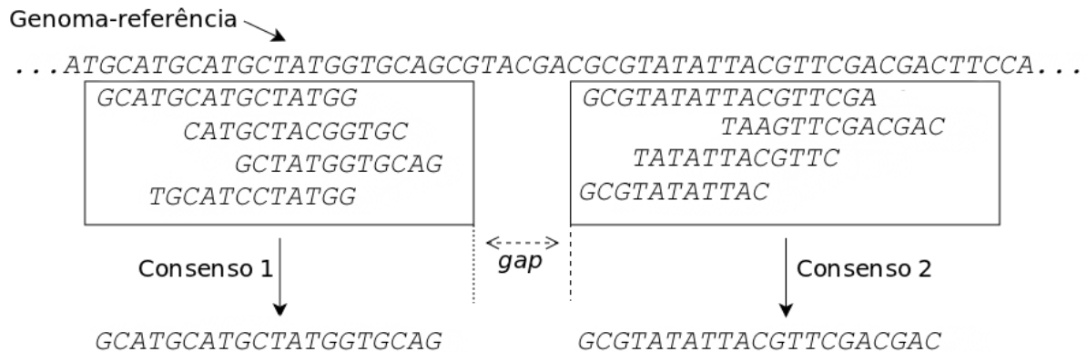
Figura 3.4: Obtenção da sequência consenso de cada contig resultante do mapeamento dos reads .
