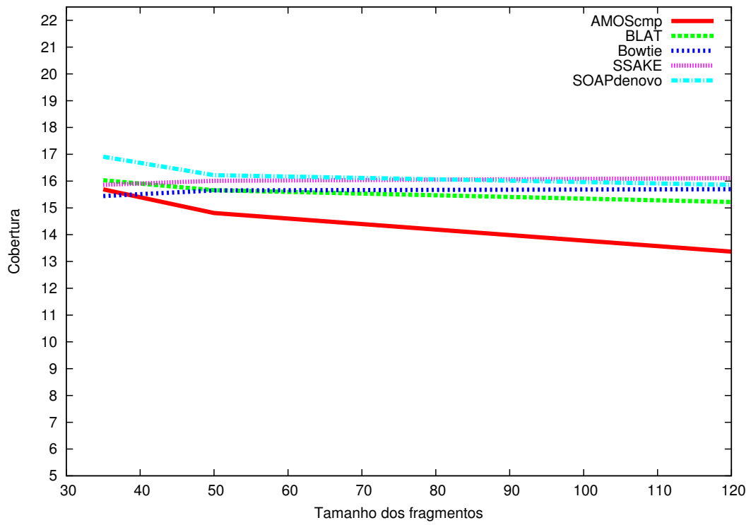
Figura 5.8: Variação na média de coberturas dos resultados de remontagem para fragmentos de cobertura-genfrag 16.
