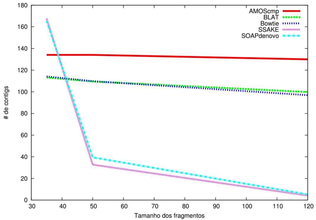
Figura 5.6: Variação na maior média de número de contigs para fragmentos de Cobertura 20.
