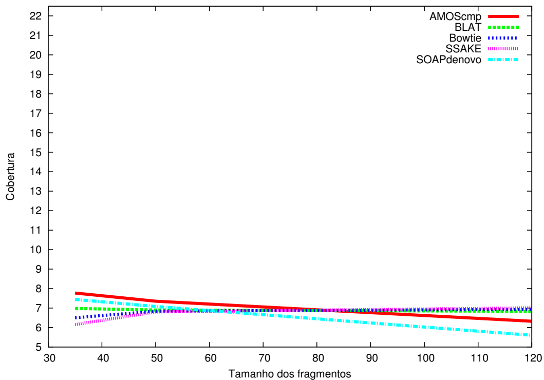
Figura 5.7: Variação na média de coberturas dos resultados de remontagem para fragmentos de cobertura-genfrag 7.
