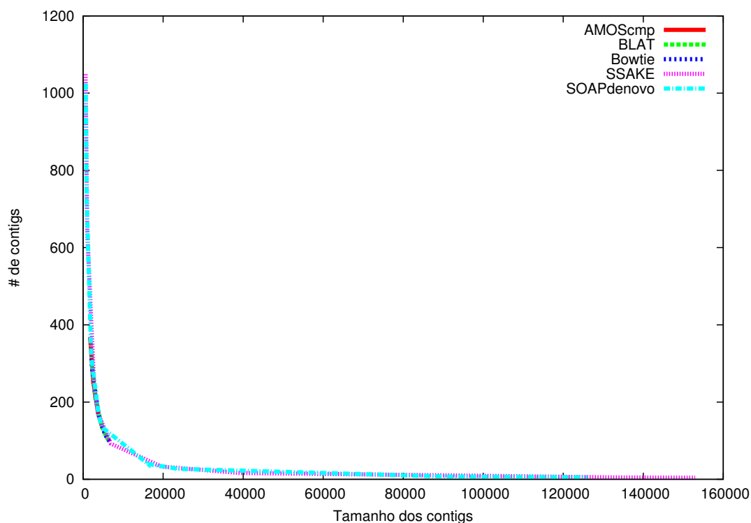
Figura 5.10: Proporção entre o número médio de contigs gerados e o tamanho médio de contigs .
