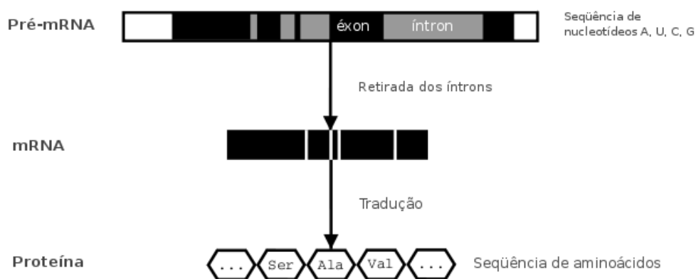
Figura 2.7: Síntese de proteínas.
