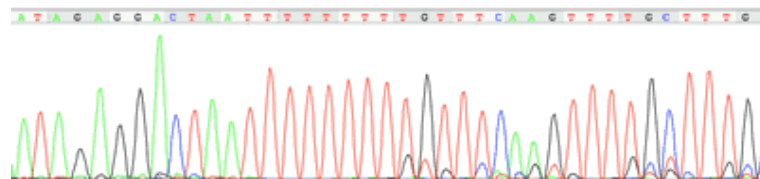
Figura 2.13: Picos consecutivos no cromatograma correspondentes ao mesmo tipo de nucleotídeo.
