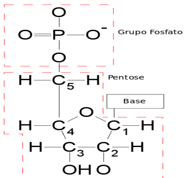
Figura 2.3: Visão detalhada da estrutura de um nucleotídeo.
