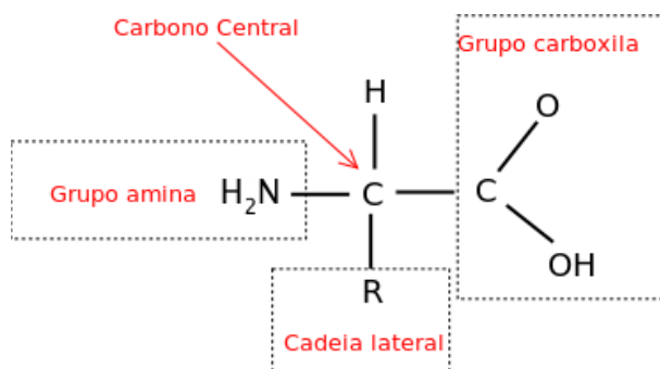
Figura 2.6: Estrutura esquemática de um aminoácido.
