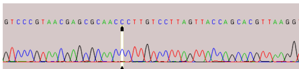
Figura 2.10: Exemplo de Cromatograma. Para representar os nucleotídeos A, C, T, G são usadas, respectivamente, as cores verde, azul, vermelha e preta. A linha branca indica um pico de curva azul e, logo, a base C é a base correspondente à posição indicada.
