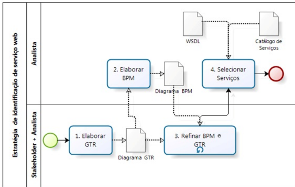
Figura 2.5: Processo de Engenharia de Aplicação [Silva, 2011]
