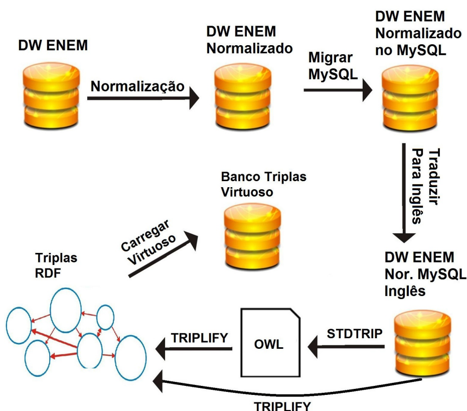
Figura 4.1: Processo utilizando Stdtrip, Triplify e Virtuoso no DW ENEM.
