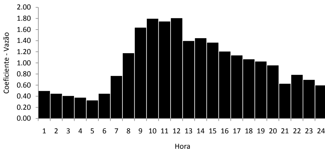
Figura 5.13 - Padrão de demanda observado (Setor A).
