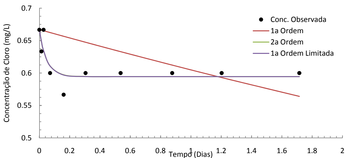
Figura 5.21 - Modelos de decaimento de cloro.
