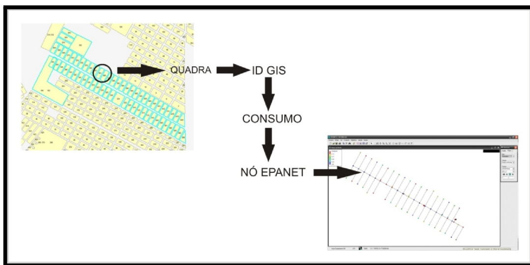
Figura 4.10 - Ilustração do procedimento de alocação de demandas.
