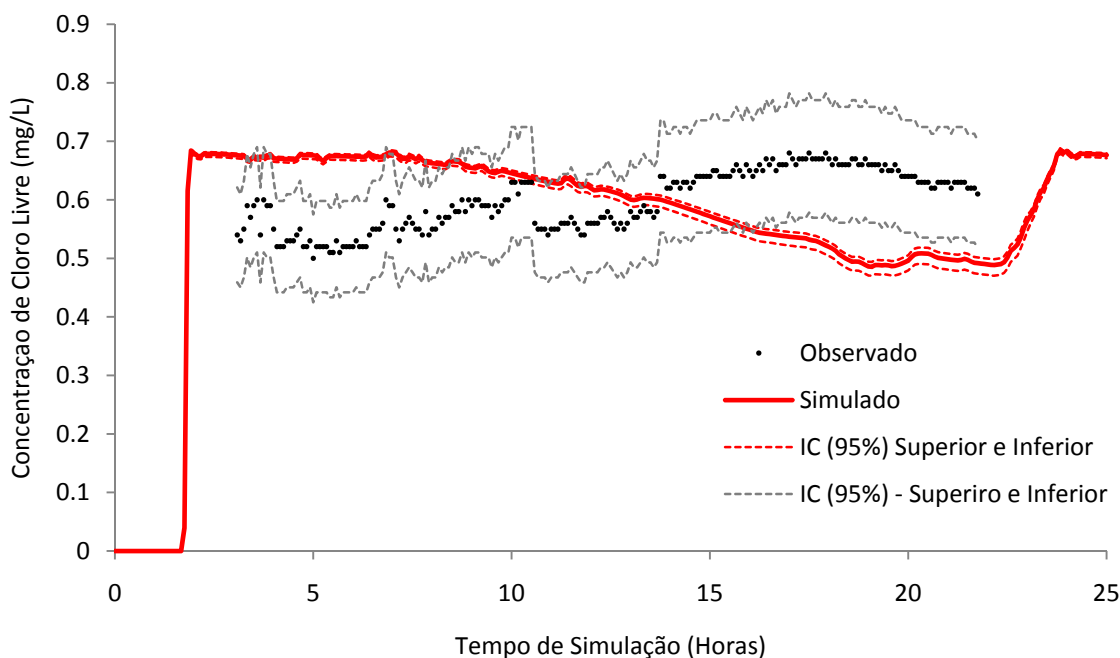
Figura 5.18 - Valores simulados e observados (Setor A).
