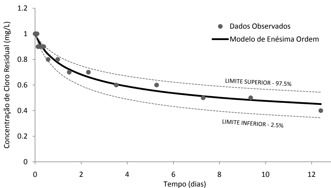
Figura 5.6 - Intervalo de confiança (modelo de enésima ordem) - Setor A.
