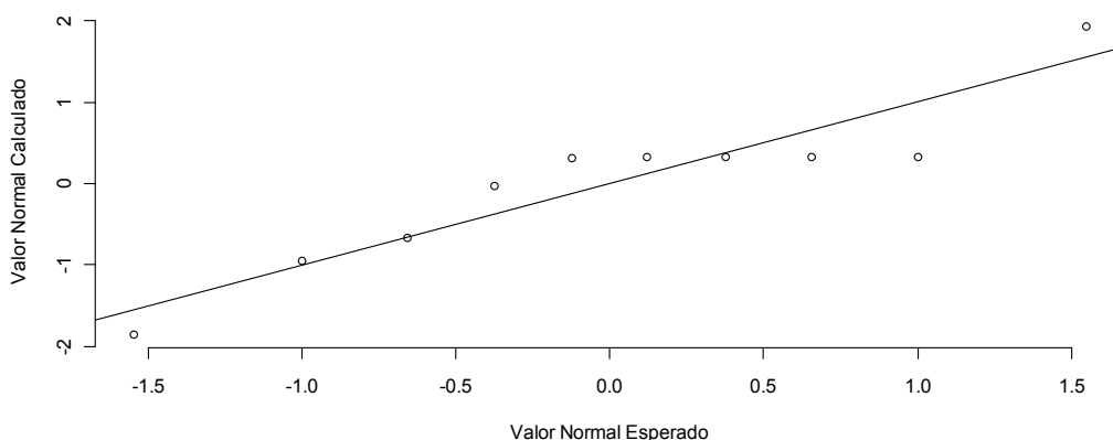
Figura 5.24 - Gráfico de probabilidade normal (Setor B).
