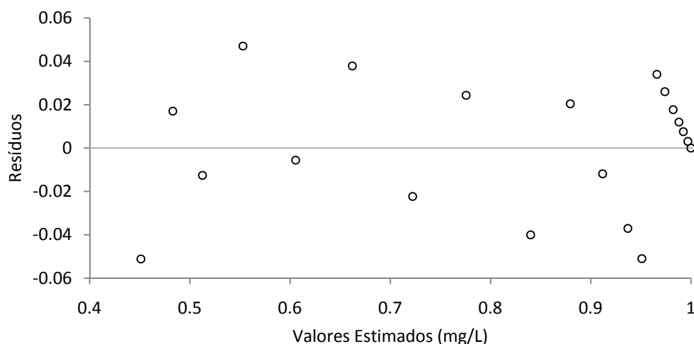
Figura 5.2 – Diagrama de dispersão dos resíduos (Setor A).
