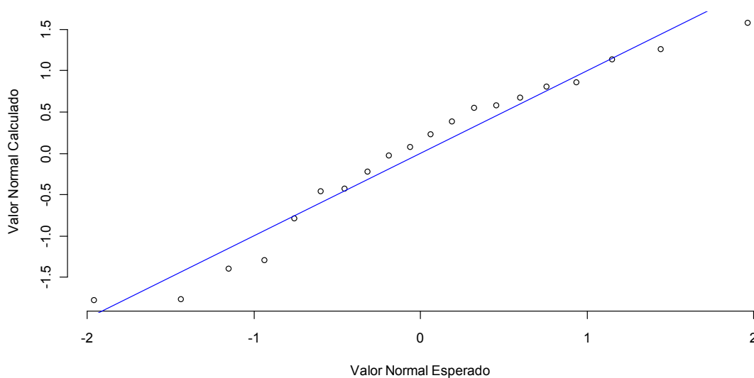
Figura 5.4 - Gráfico de probabilidade normal (Setor A).
