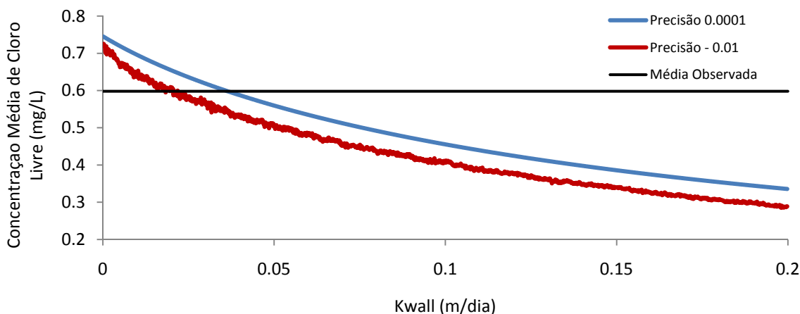
Figura 5.17 - Relação k_{wall} com concentração média de cloro.
