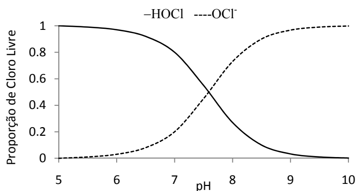
Figura 3.1 - Efeito do pH na quantidade relativa de HOCl e \text{OCl}^- . (Fonte: Hass, 1990 - Adaptado de Morris, 1951).
