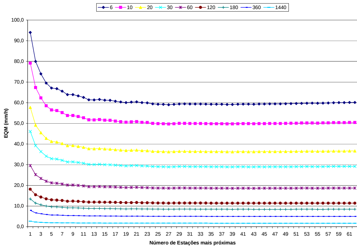
FIGURA 5.20. EQM das Intensidades Pluviométricas, utilizando o Método do Inverso da Distância, em relação ao número de Estações mais próximas e da duração da precipitação para T = 50 anos.
