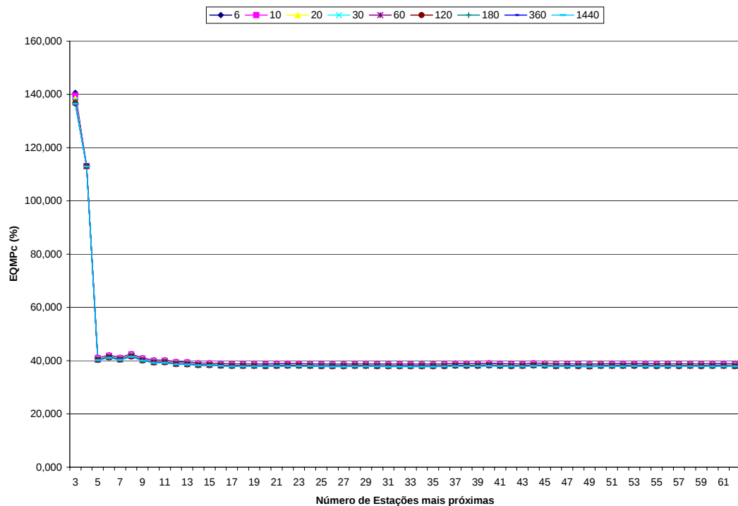
FIGURA 5.10. EQMPc das Intensidades Pluviométricas, utilizando o Método da Superfície Spline, em relação ao número de Estações mais próximas, para T = 50 anos e t variável de 6 min a 1440 min.
