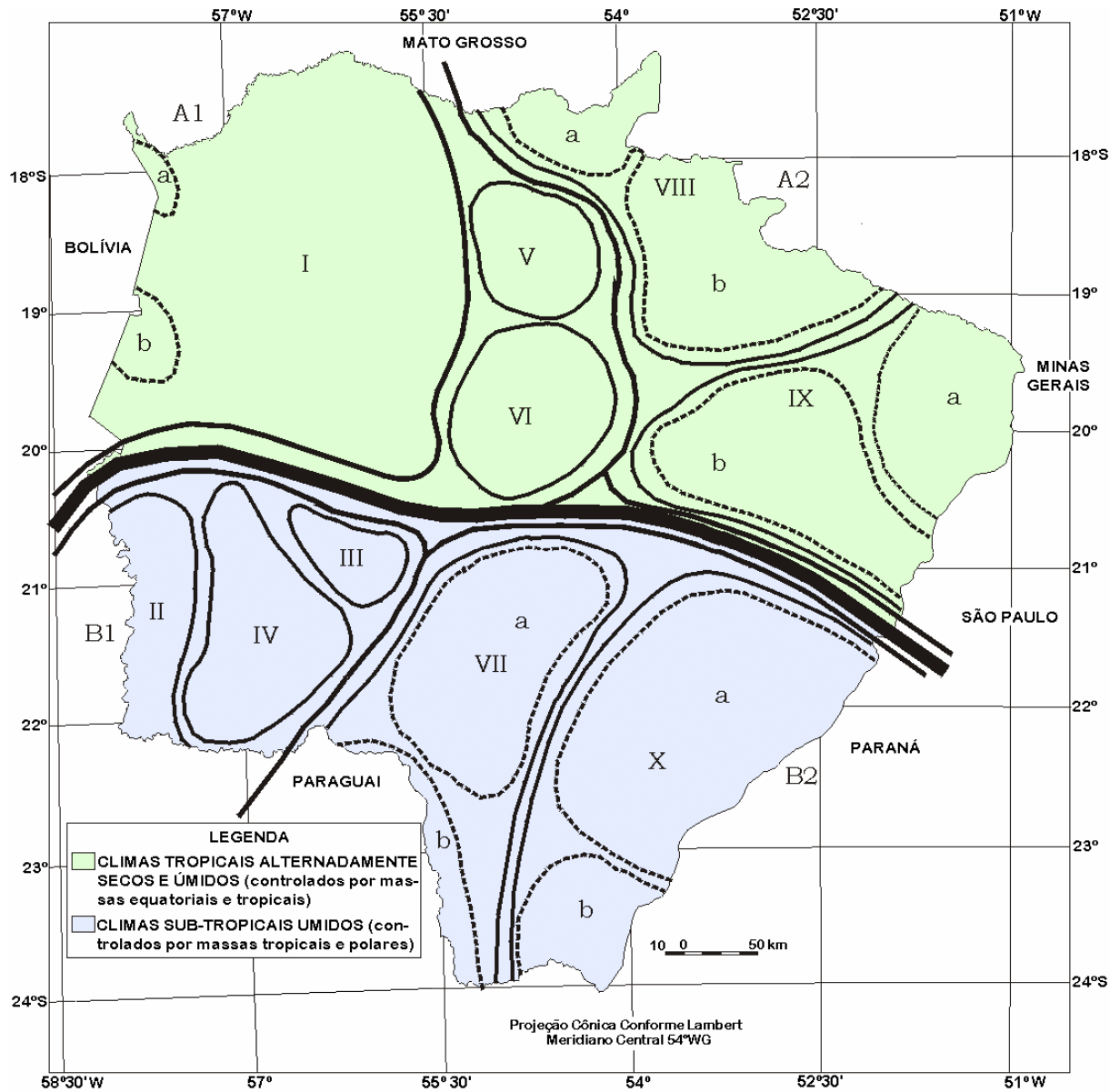
FIGURA 1.2. Proposta de Classificação Climática para o Mato Grosso do Sul, modificado de ZAVATINI (1992) e UNIDERP (2001).
