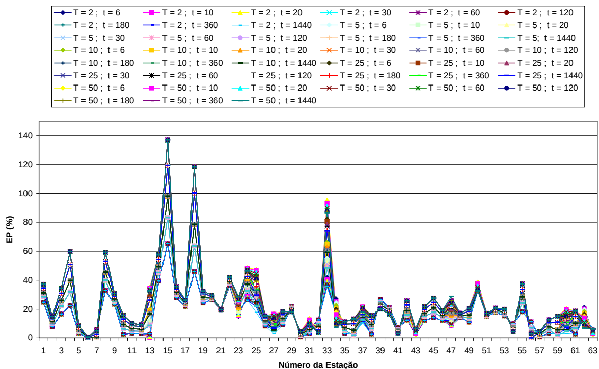
FIGURA 5.21. EP das Intensidades Pluviométricas das 63 Estações, utilizando o Método dos Polígonos de Thiessen (Vizinho Mais Próximo) para 45 combinações entre períodos de retorno e durações de chuva.
