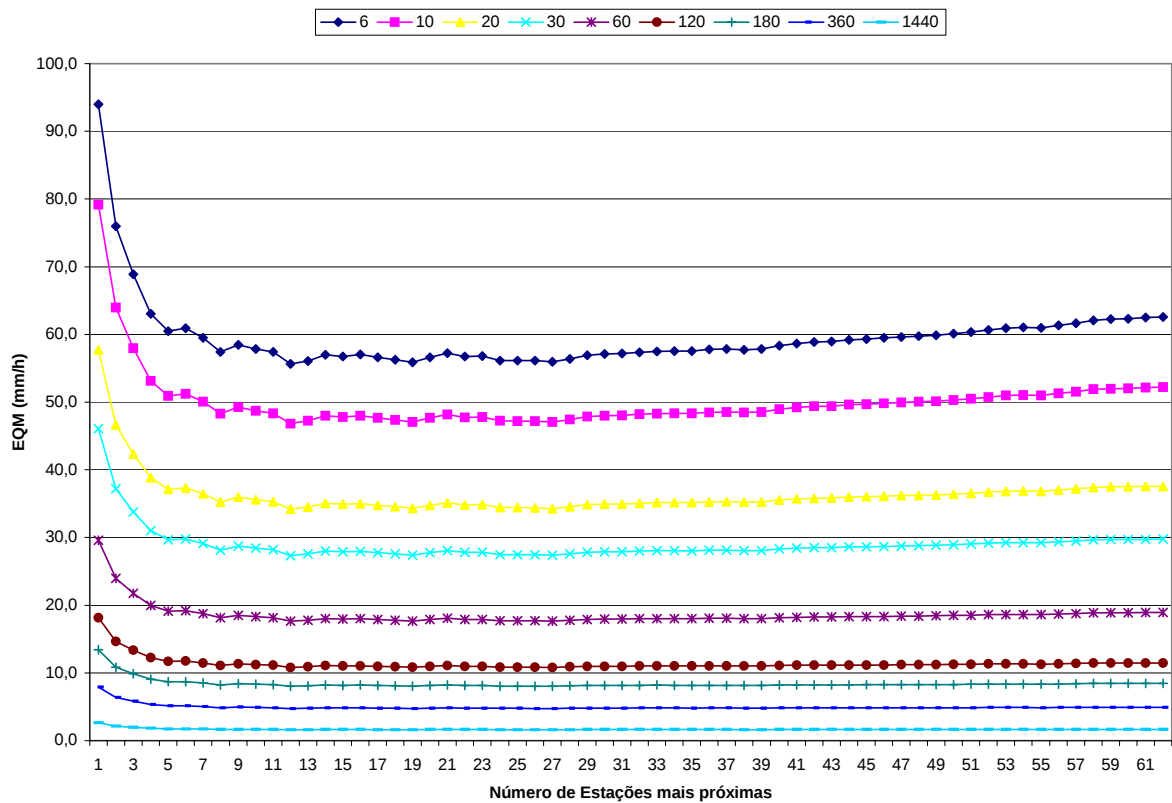
FIGURA 5.15. EQM das Intensidades Pluviométricas, utilizando o Método dos Vizinhos Mais Próximos, em relação ao número de Estações mais próximas, para T = 50 anos e t variável de 6 min a 1440 min.
