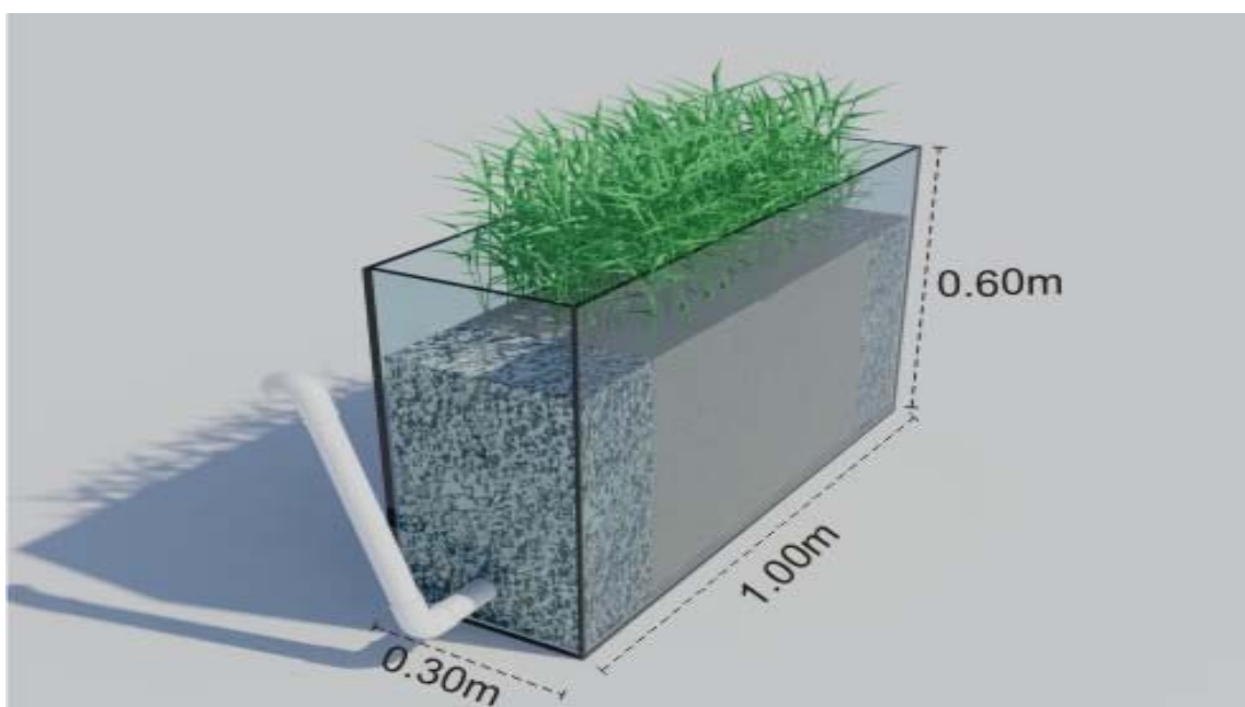
Figura 1 – Perspectiva das wetlands construídas - vegetadas
