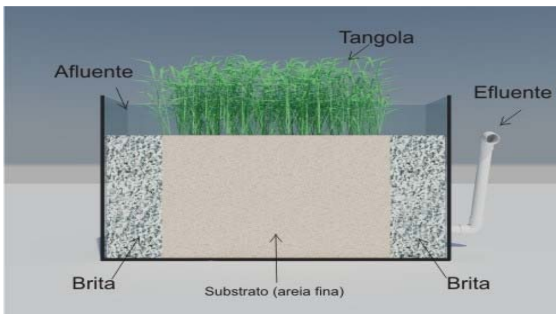
Figura 2 – Corte longitudinal das wetlands construídas - vegetadas
