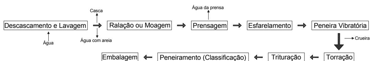
Figura 2 - Fluxograma geral de uma farinheira
