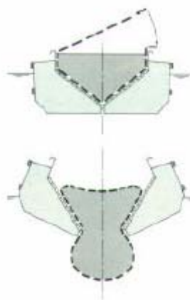
Figura 3.9. Desenho esquemático de uma comporta de fundo em dois momentos, ora fechada durante preenchimento do geotubo e depois aberta para disposição do mesmo no local.
