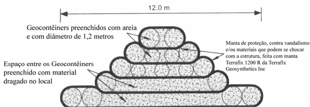
Figura 3.10. Corte esquemático da disposição dos geocontainers no quebra-mar “Kirra”, na costa dourada da Austrália.
