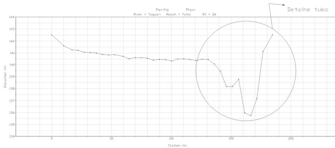
Perfil Seção Transversal
