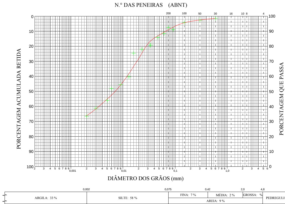
Figura 5.3. Curva granulométrica conjunta – amostra A4: profundidade de 1,20 m da superfície.
