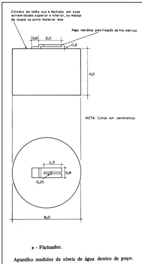
Figura 3.14 - Flutuador.
