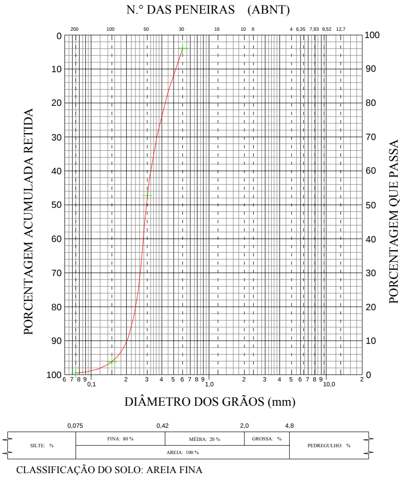
Figura 5.5. Curva de ensaio de peneiramento – amostra 01: profundidade de 0,50 m da superfície.
