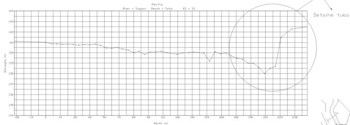
Perfil Seção Transversal
