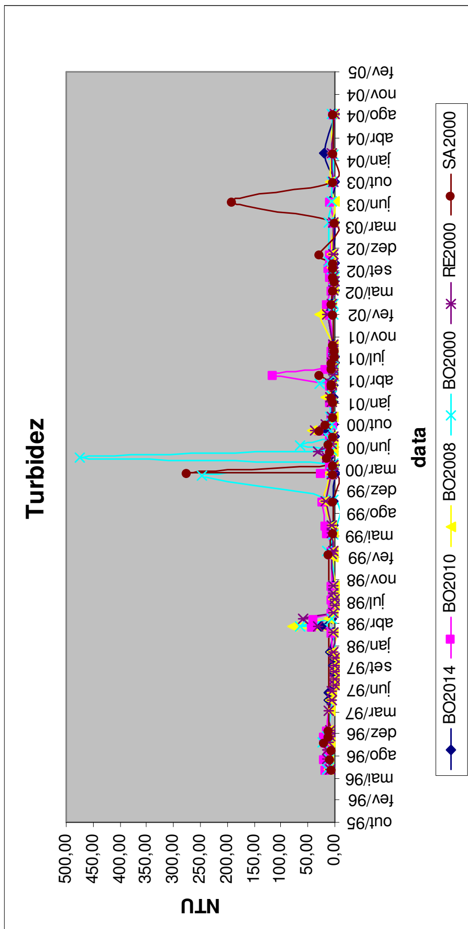
Figura 20 – Variação espaço temporal da turbidez nas águas da bacia do córrego Saladeiro.
