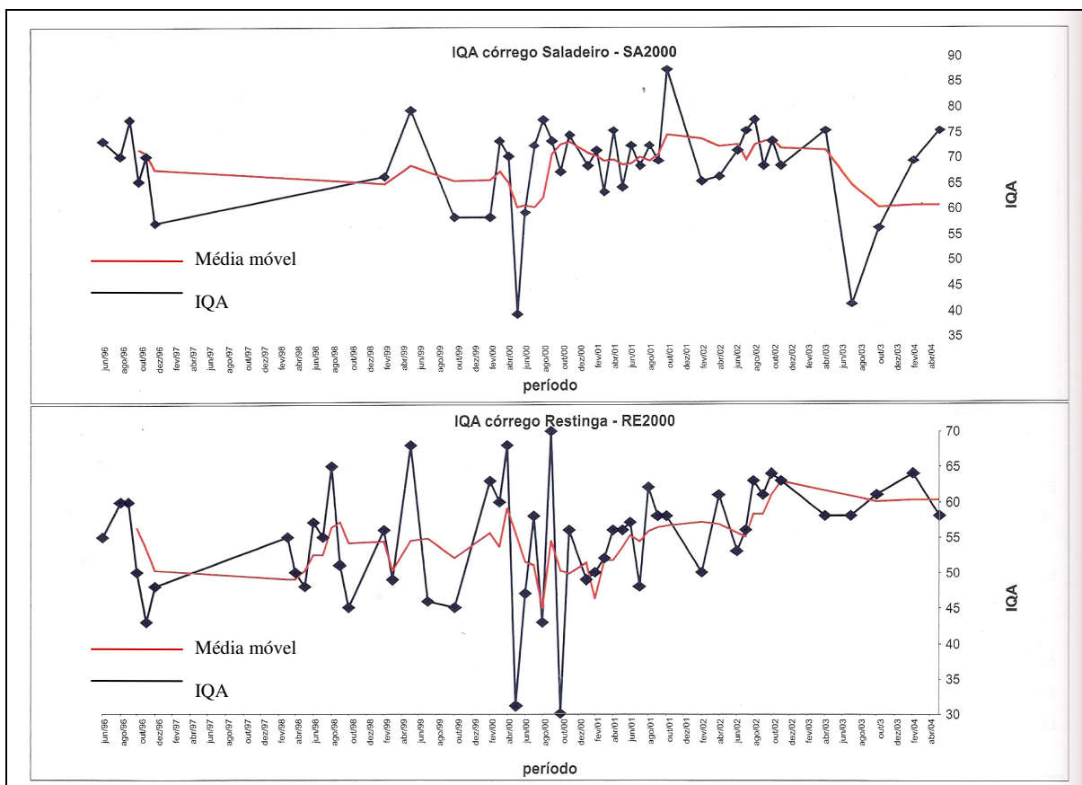
Figura 7 – Variação espacial longitudinal da qualidade da água dos córregos Saladeiro e Restinga e a tendência da qualidade medida pela média móvel. Fonte: MATO GROSSO DO SUL (2005)
