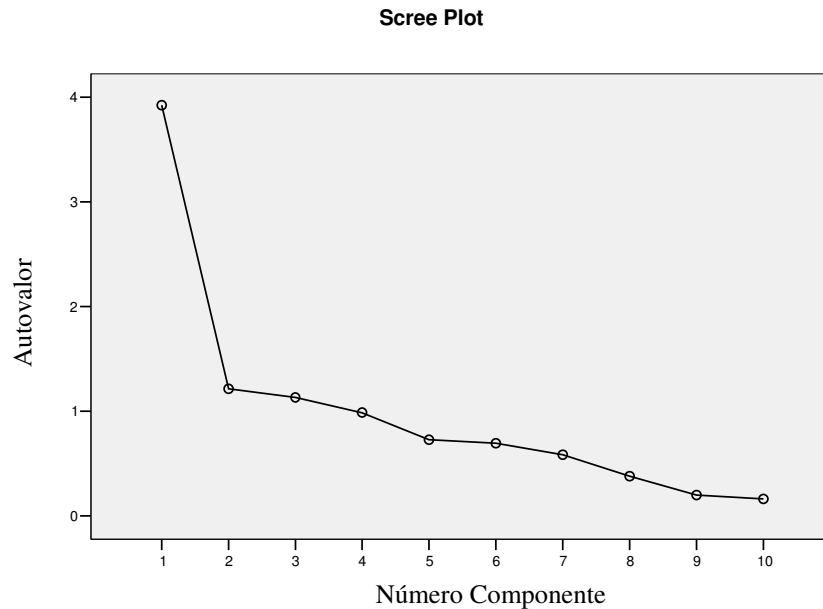
Figura 35 – Scree Plot da resultante da análise das 10 variáveis.
