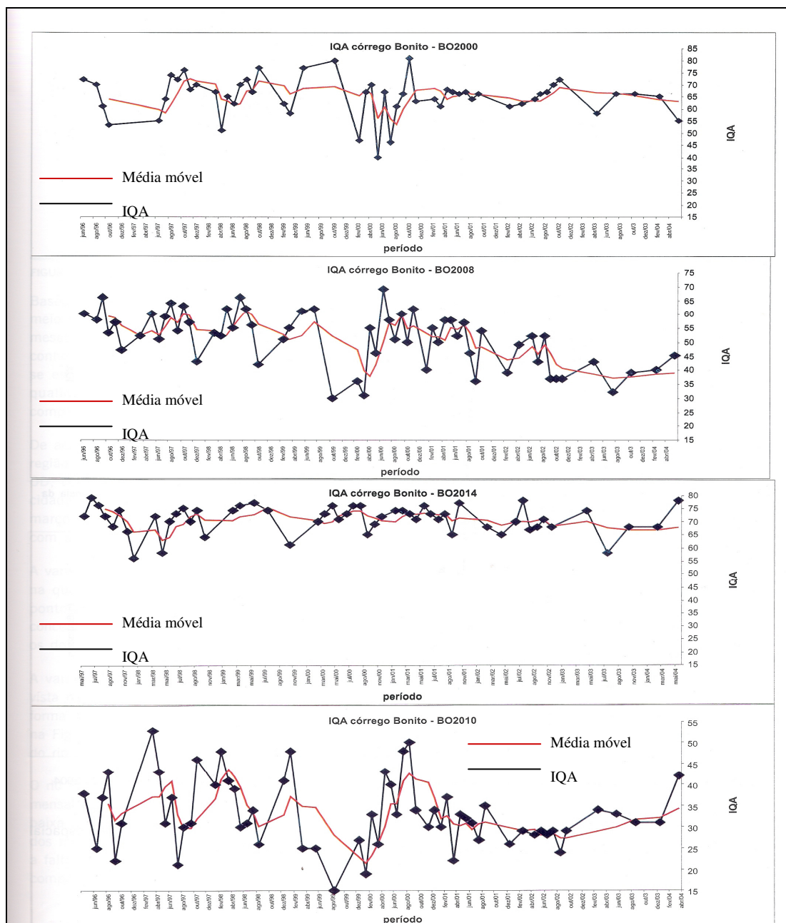
Figura 6 – Variação temporal e espacial longitudinal da qualidade da água do córrego Bonito e a tendência da qualidade medida pela média móvel.
