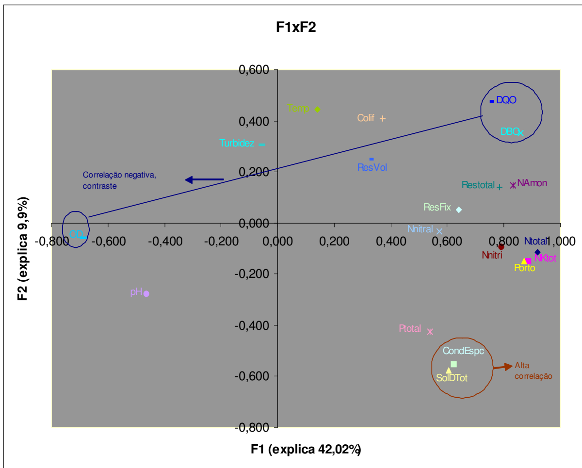
Figura 33 – Relação das duas primeiras componentes principais, F1 e F2, resultante da análise das 19 variáveis.
