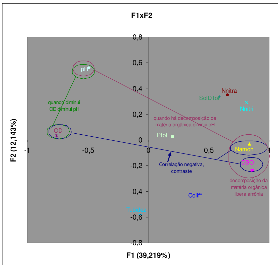
Figura 36 – Relação das duas primeiras componentes principais, F1 e F2, resultante da análise das 10 variáveis.
