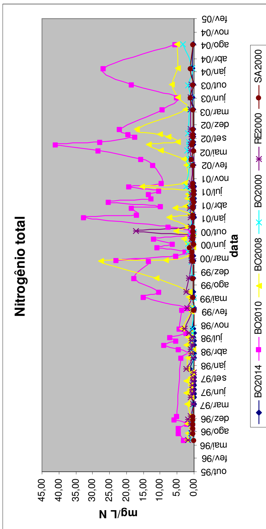
Figura 17 – Variação espaço temporal do nitrogênio total nas água da bacia do córrego Saladeiro.
