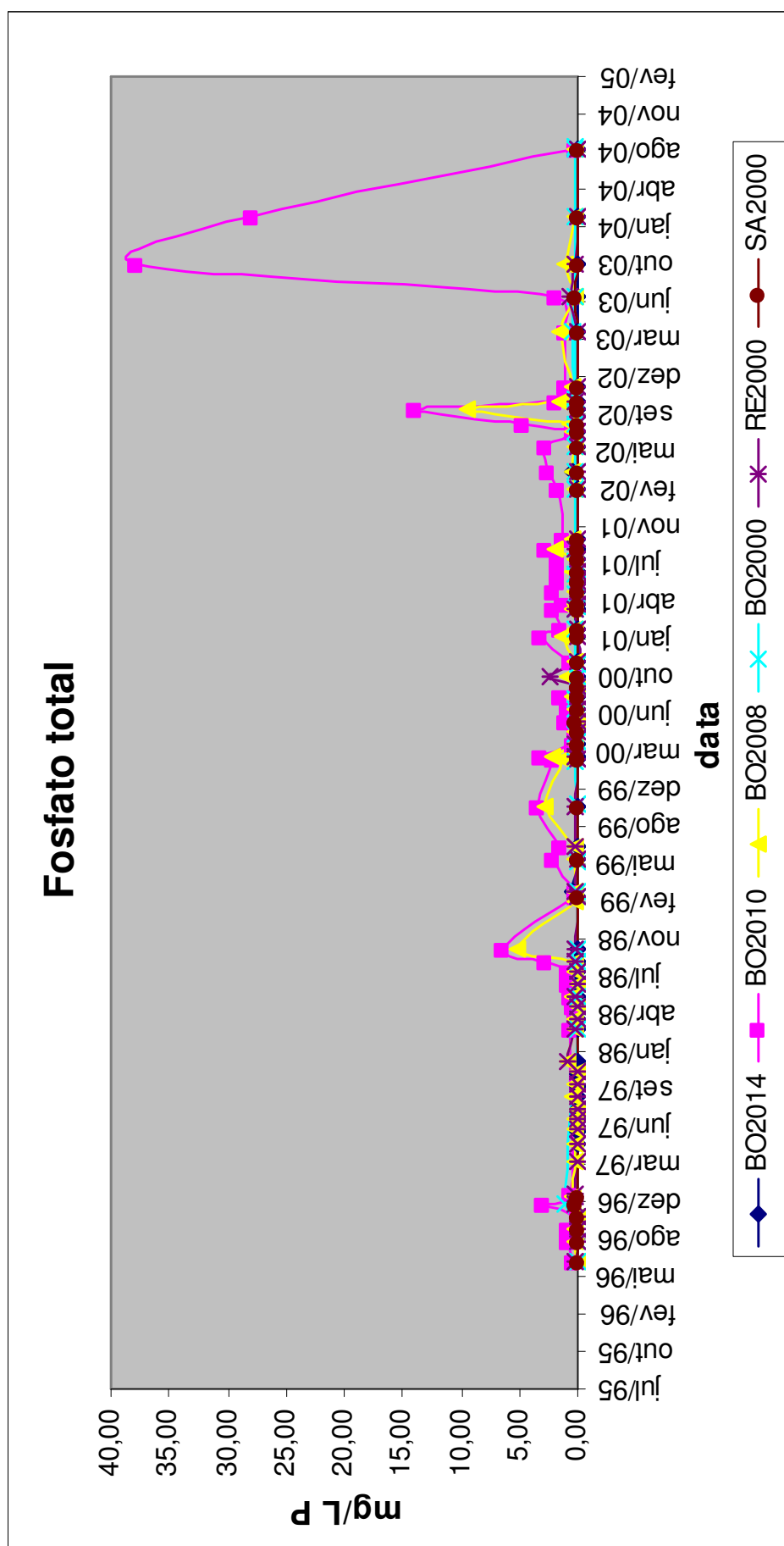
Figura 18 – Variação espaço temporal do fosfato total nas águas da bacia do córrego Saladeiro.
