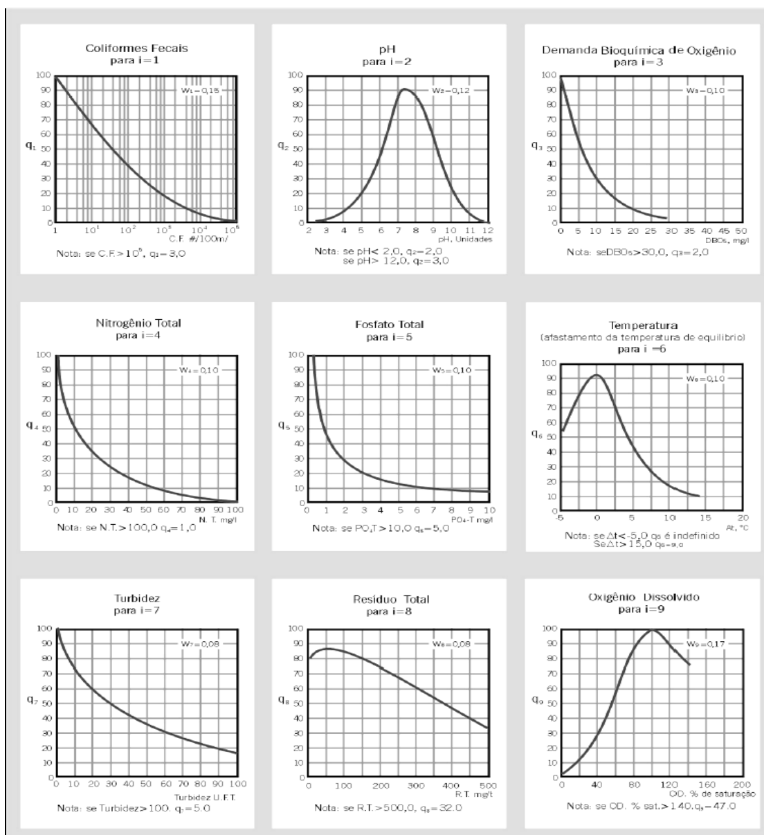
Figura 3 - Curvas Médias de Variação de Qualidade das Águas Fonte: MATO GROSSO DO SUL (2004).
