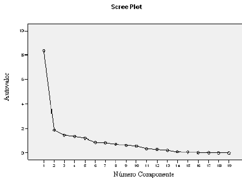
Figura 32 – Scree Plot resultante da análise das 19 variáveis.
