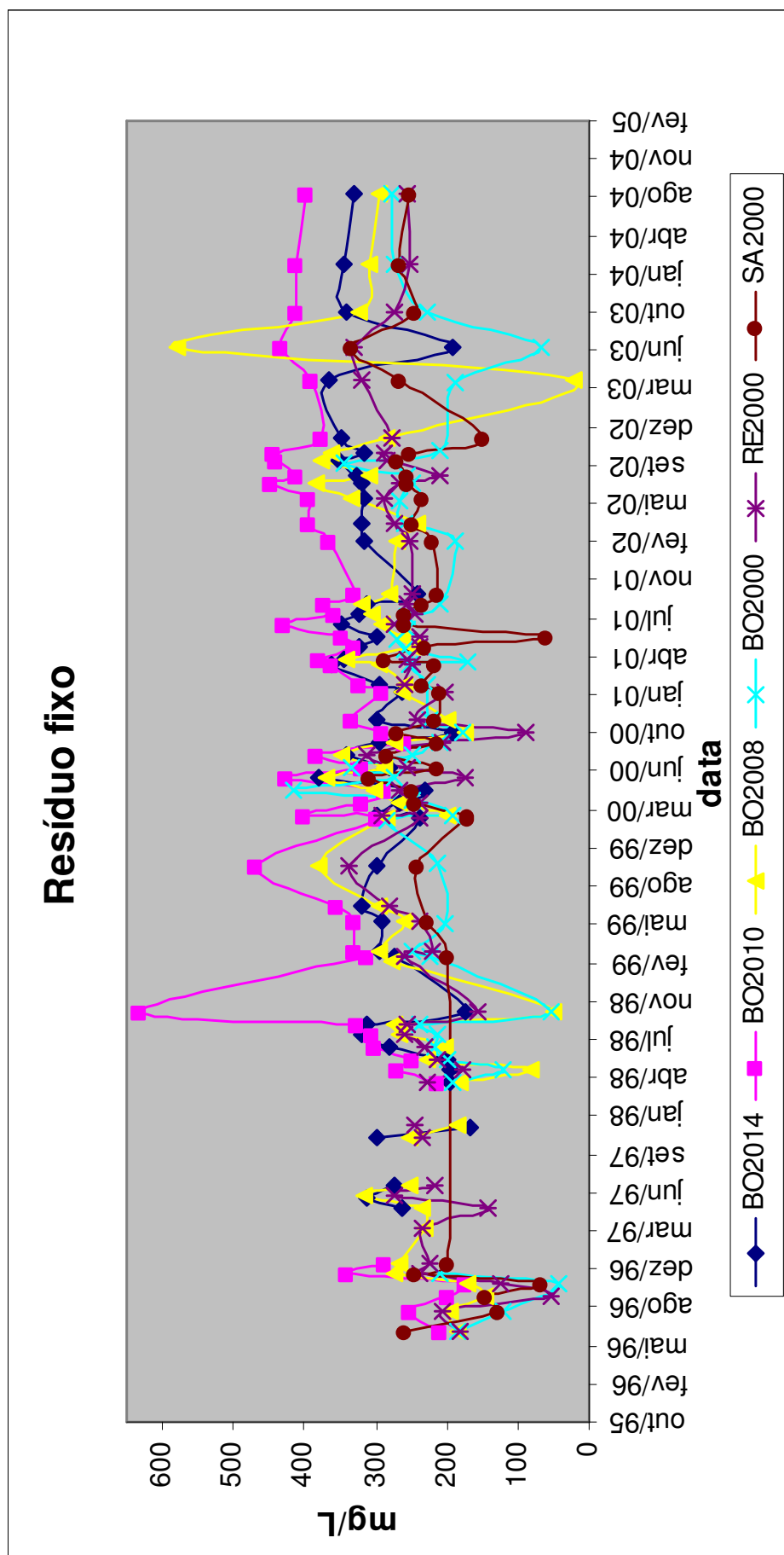
Figura 28 – Variação espaço temporal do resíduo fixo nas águas da bacia do córrego Saladeiro.
