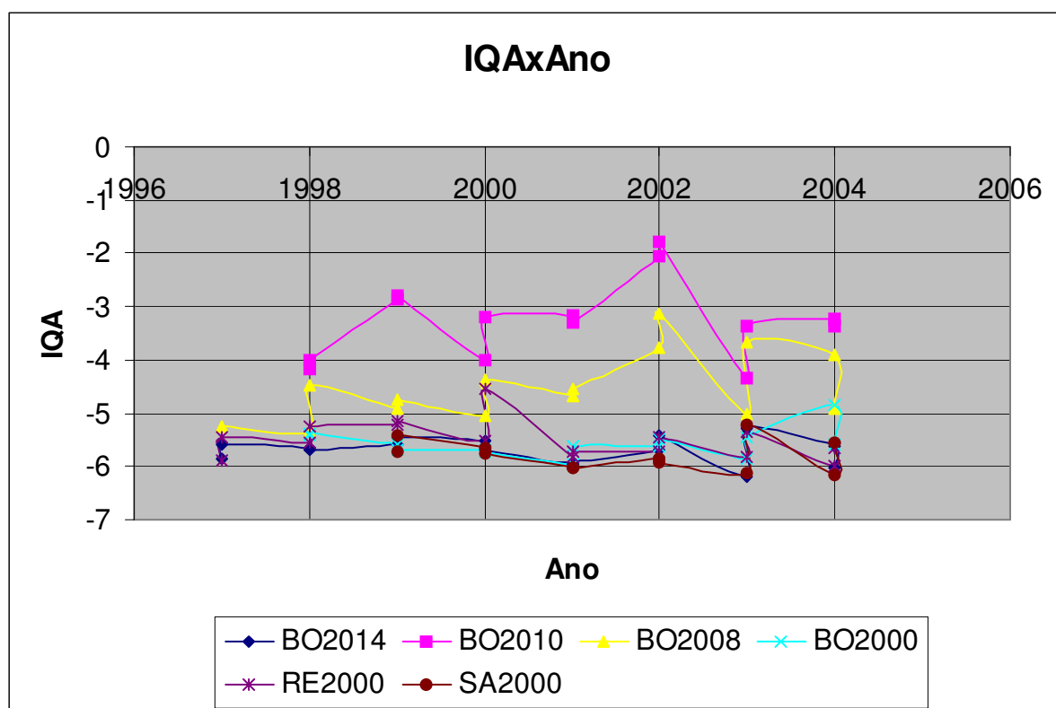
Figura 37 – IQAxAno, variação da qualidade da água de diversos pontos da bacia do córrego Saladeiro ao longo do tempo, resultante da análise das 10 variáveis.
