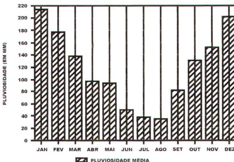
Figura 06 – Pluviosidade Média do Município de Aquidauana-MS, período de 1931 a 1990. Fonte: PINTO (1998).
