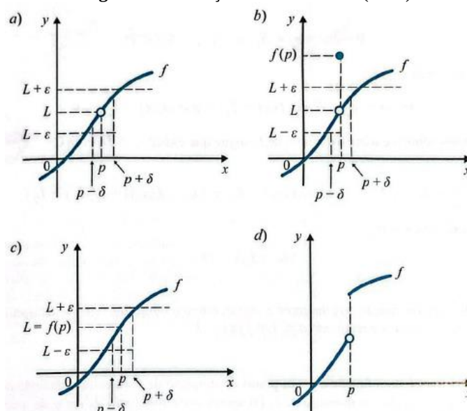
Figura 31 - Situações em Guidorizzi (2018)
