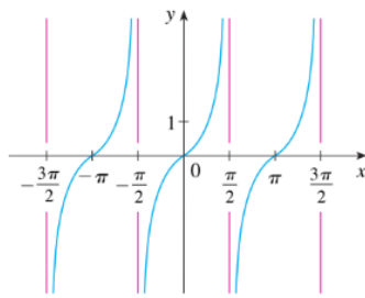
FIGURA 16 y = \operatorname{tg} x
