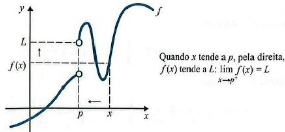
Figura 39 - Definição de limite lateral no gráfico no Guidorizzi (2018)
