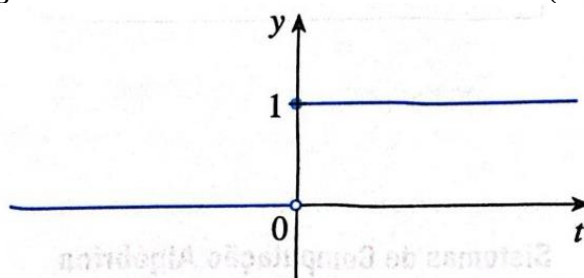
Figura 24 - Limites laterais na Heaviside em Stewart (2017)
