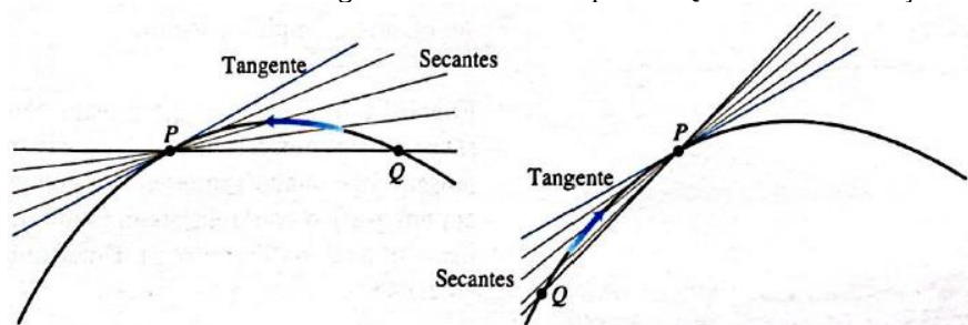
FIGURA 2.3 A tangente à curva em P é a reta que atravessa P cujo coeficiente angular é o limite dos coeficientes angulares das secantes quando Q \rightarrow P de ambos os lados.
