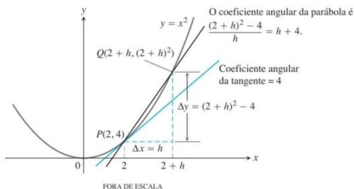
Figura 7 - Coeficiente angular no gráfico (Thomas, 2012)
