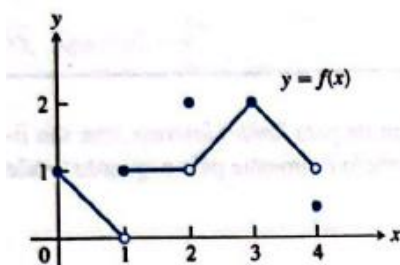
Figura 13 - Limite lateral no gráfico em Thomas (2012)
