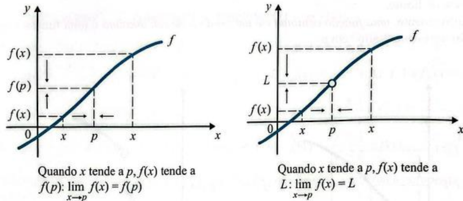
Figura 28 - Gráficos representando a definição intuitiva
