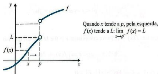
Figura 40 - Definição de limite lateral pela esquerda no Guidorizzi (2018)
