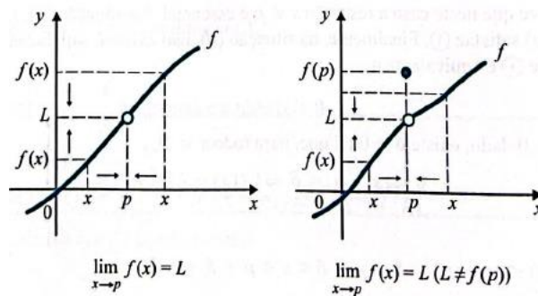
Figura 32 - Limites no gráfico em Guidorizzi (2018)
