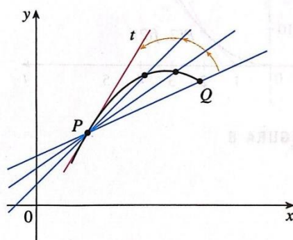
Figura 18 - retas secantes aproximando-se da reta tangente
