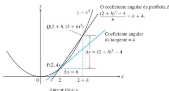
FIGURA 2.4 Determinação do coeficiente angular da parábola y = x^2 no ponto P(2, 4) como o limite de coeficientes angulares das secantes (Exemplo 3).
