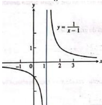
Figura 15 - Limites laterais no gráfico de f em Thomas (2012)
