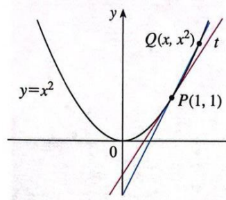
Figura 20 - inclinação da reta secante em Stewart (2017)
