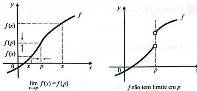
Figura 33 - Análise dos limites no gráfico em Guidorizzi (2018)
