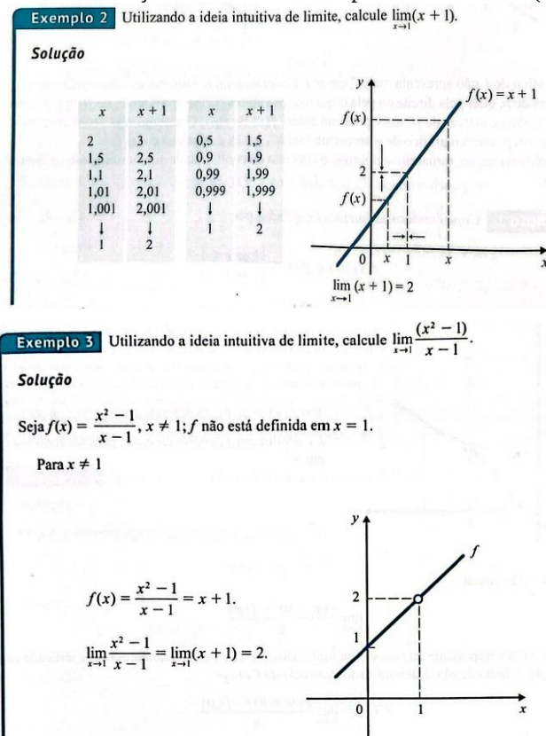
Figura 29 - Definição intuitiva nos exemplos no Guidorizzi (2018)
