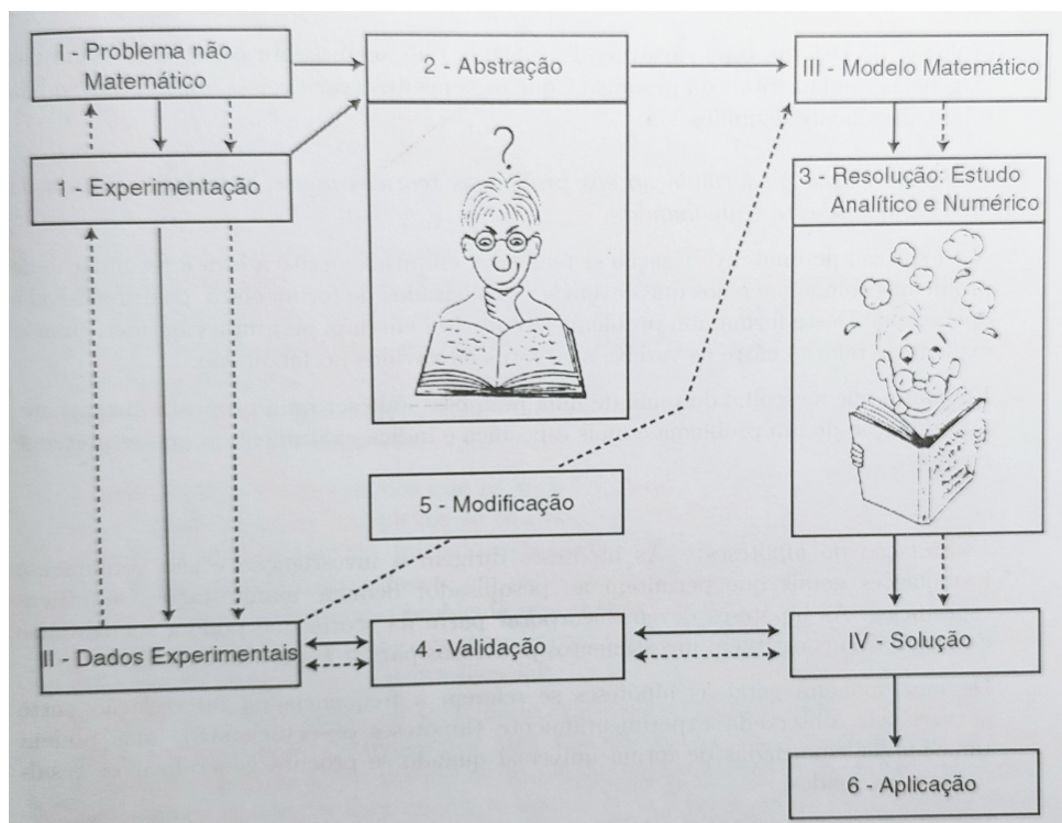
Figura 2.1: Esquema de uma modelagem: as setas contínuas representam a primeira aproximação. As setas pontilhadas surgem na busca de um modelo matemático para o problema, tornando o processo dinâmico.
