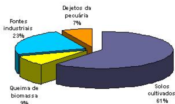
Figura 4.3 - Principais fontes antrópicas de emissões de óxido nitroso (N 2 O) para a atmosfera
